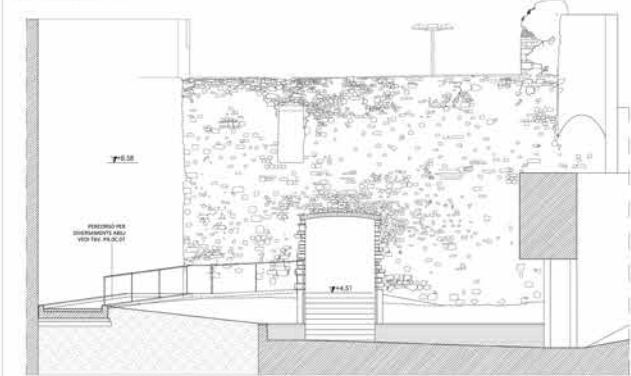
PROGETTO - SEZIONE B-B'
