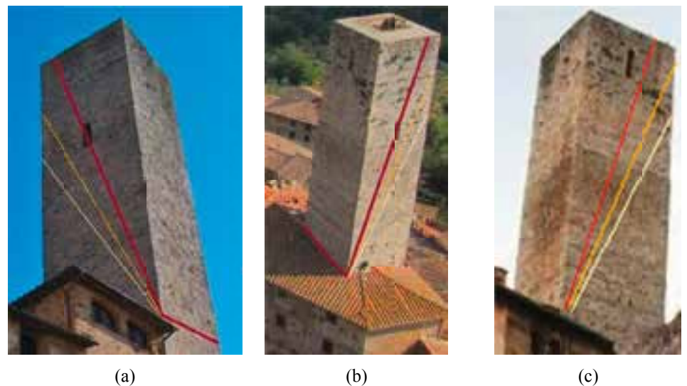
Figura 8 - Ribaltamento composto: (a) parete Sud (E); (b) parete Nord (F); (c) parete Ovest (G). Inclinazione del cuneo: 15°(rosso), 22°(arancione) e 30°(giallo).
