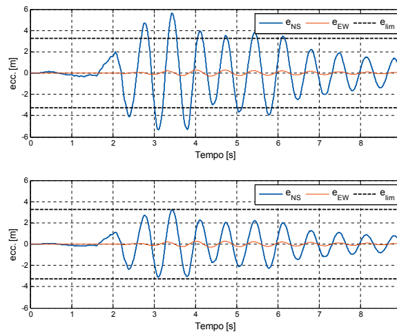
Figura 11 – Input 2 / TH6: Evoluzione temporale di ez,t.
