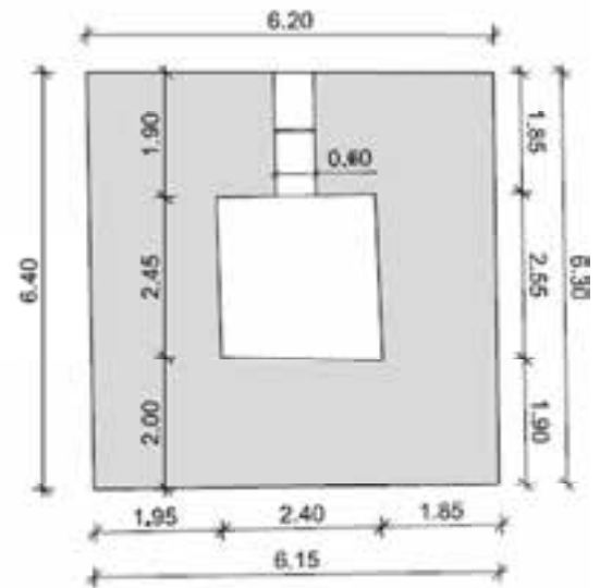
Figura 4 - Sezione quota + 35 m (S7). Misure in metri.
