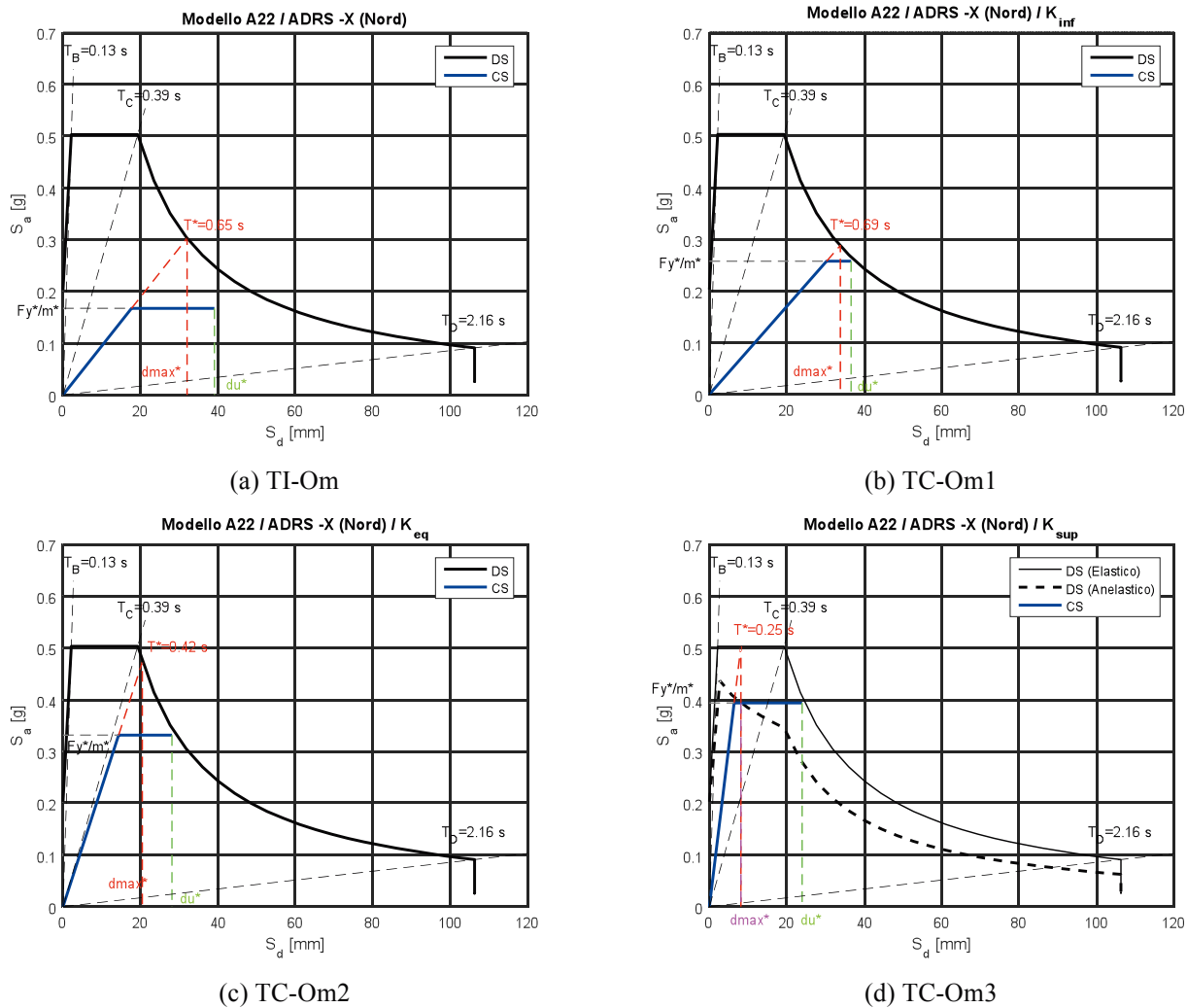
Figura 19. Confronto tra capacità e domanda mediante il metodo N2 per la direzione Nord (-X): influenza della rigidezza dei vincoli (modello di torre con paramenti omogeneizzati e parametri meccanici del caso A22).
