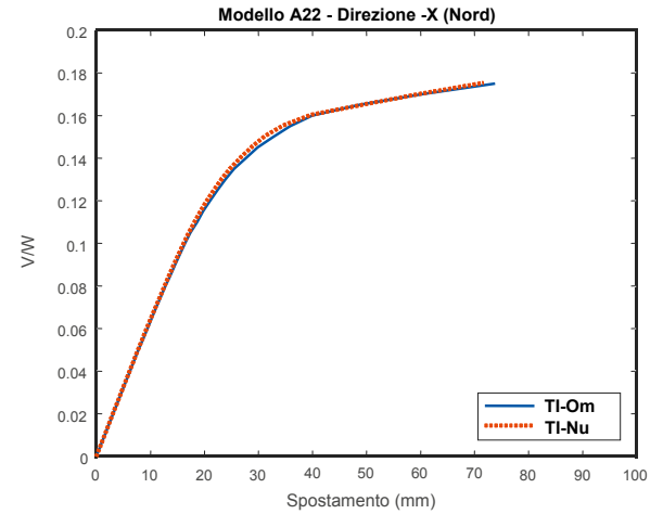
Figura 14. Confronto tra le curve di capacità del modello meccanico A22 in direzione -X (Nord) per i modelli TI-Om (paramenti omogeneizzati) e TI-Nu (paramenti distinti).
