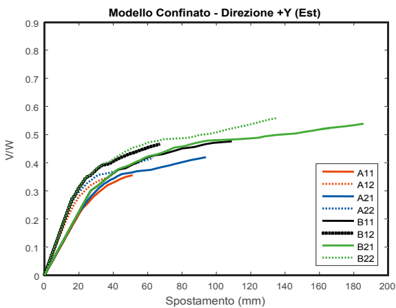
Figura 16. Modello di torre confinata. Curve di capacità nelle direzioni \pm X e +Y al variare dei parametri meccanici in ingresso, fissato il grado di vincolo offerto dagli edifici adiacenti ( K=K_{eq} ).
