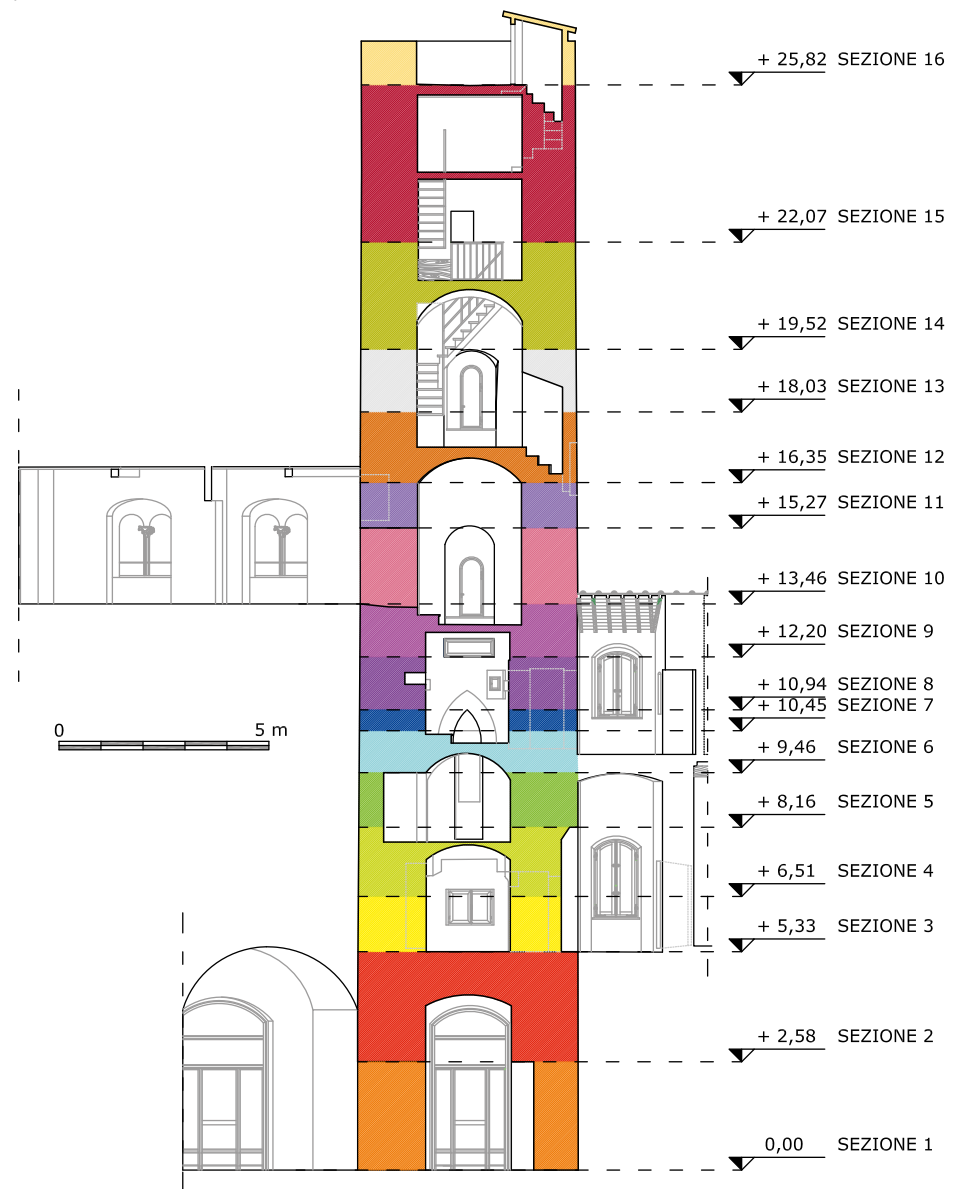
Figura 7. Sezioni dei concii individuati nella schematizzazione a mensola.
