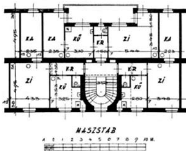
WOHNHAUSANLAGE XIX. BEZ. HEILIGENSTÄDTERSTRASSE BAUBLOCK I WOHNUNGSTYP
