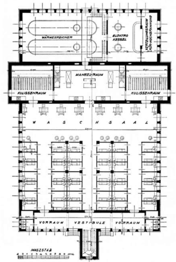
WOHNHAUSANLAGE - XIX. BEZ. HEILIGENSTÄDTERSTRASSE WÄSCHEREI-UND-BADEANLAGE ERDGESCHOSS
