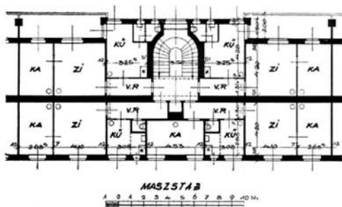
WOHNHAUSANLAGE - XIX. BEZ. HEILIGENSTÄDTERSTRASSE WOHNUNGSTYP
