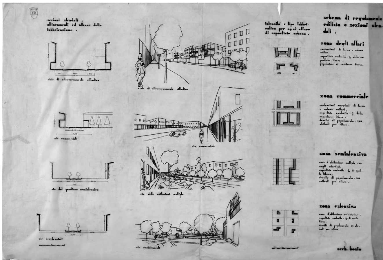
Gherardo Bosio, Piano Regolatore di massima, schema di regolamento edilizio e sezioni stradali, 1937. China su lucido
