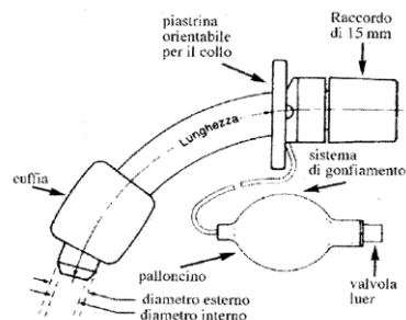
Figura 10 – Componenti della cannula tracheostomica. [Fonte: Linea Guida per la gestione del Paziente con Trachotomia nell'ambito riabilitativo, Clinica Hildebrand, Brissago, 7, I-cure-030.
