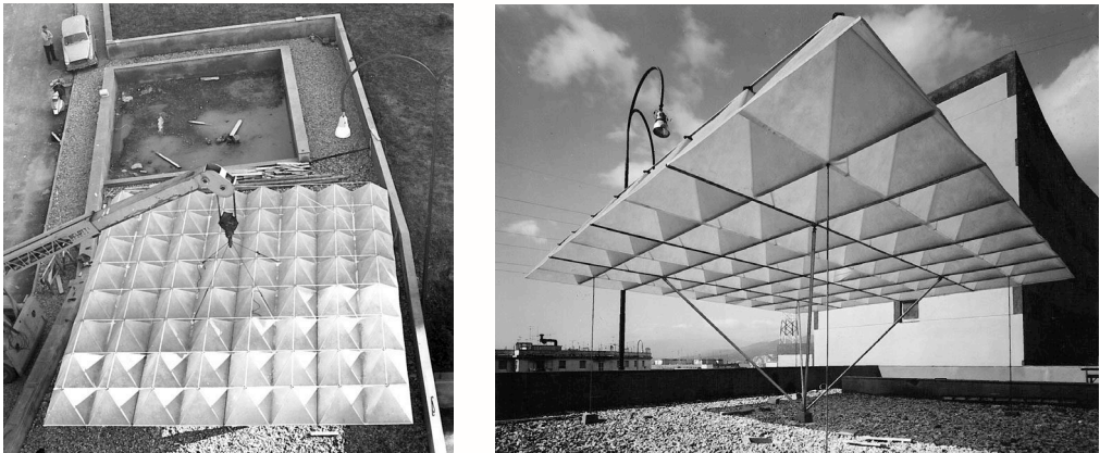
Figure 3, 4. Reinforced polyester space frame, Genoa, 1965. Renzo Piano. (Fondazione Renzo Piano)
