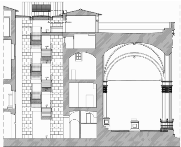
Sezione BB Section BB
