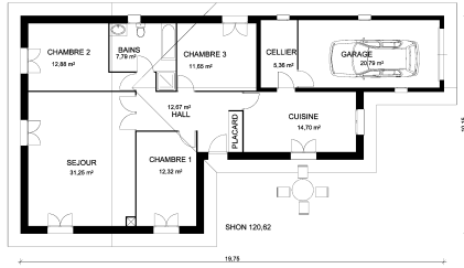
Plan du Rez de Chaussée 42446 11/06/2018 10h 10m pour 110 dém. mesurer 20/08/2018 4 p.10
