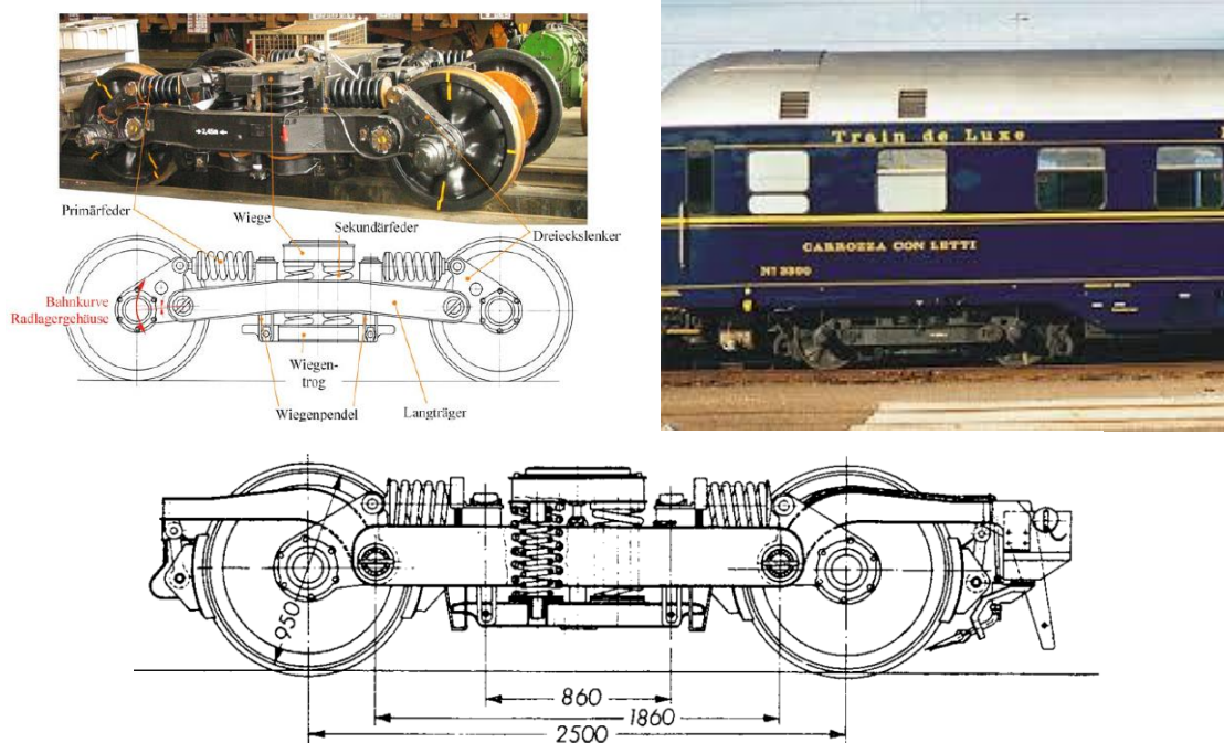
Fig. 5 Top: the Wegmann-Kassel (also know as the München-Kassel) bogie, with swinging arms and horizontal primary suspension (from J. Ihme – Schienenfahrzeugtechnik - Springer Vieweg Verlag 2016, pp. 183-184). Bottom: drawing taken from K. Sachs – Elektrische Triebfahrzeuge, Springer Verlag, 1973.
