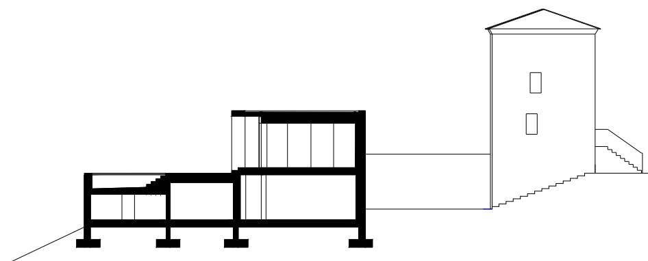
Sezione B-B
