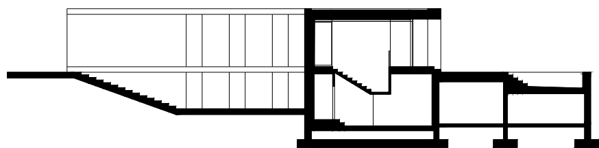
Sezione A-A
