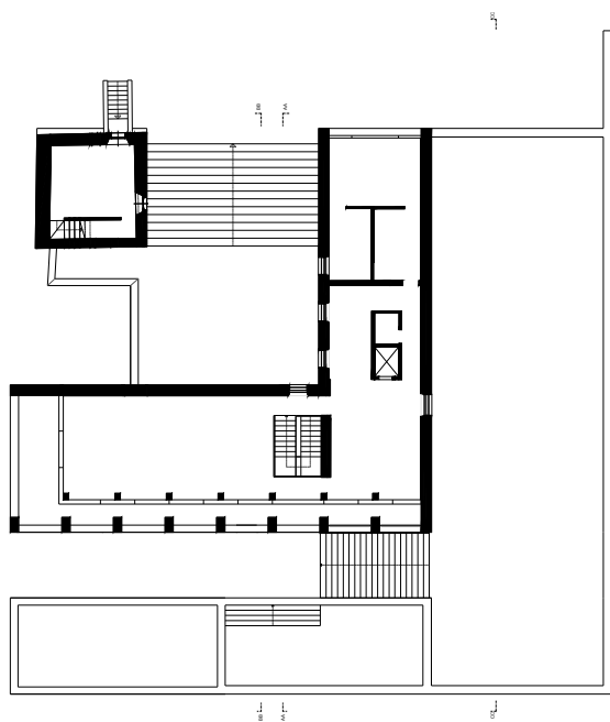
Piano livello 1
