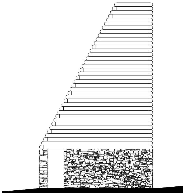
prospetto
