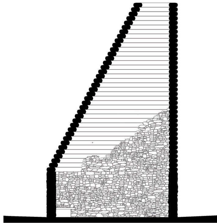
sezione
