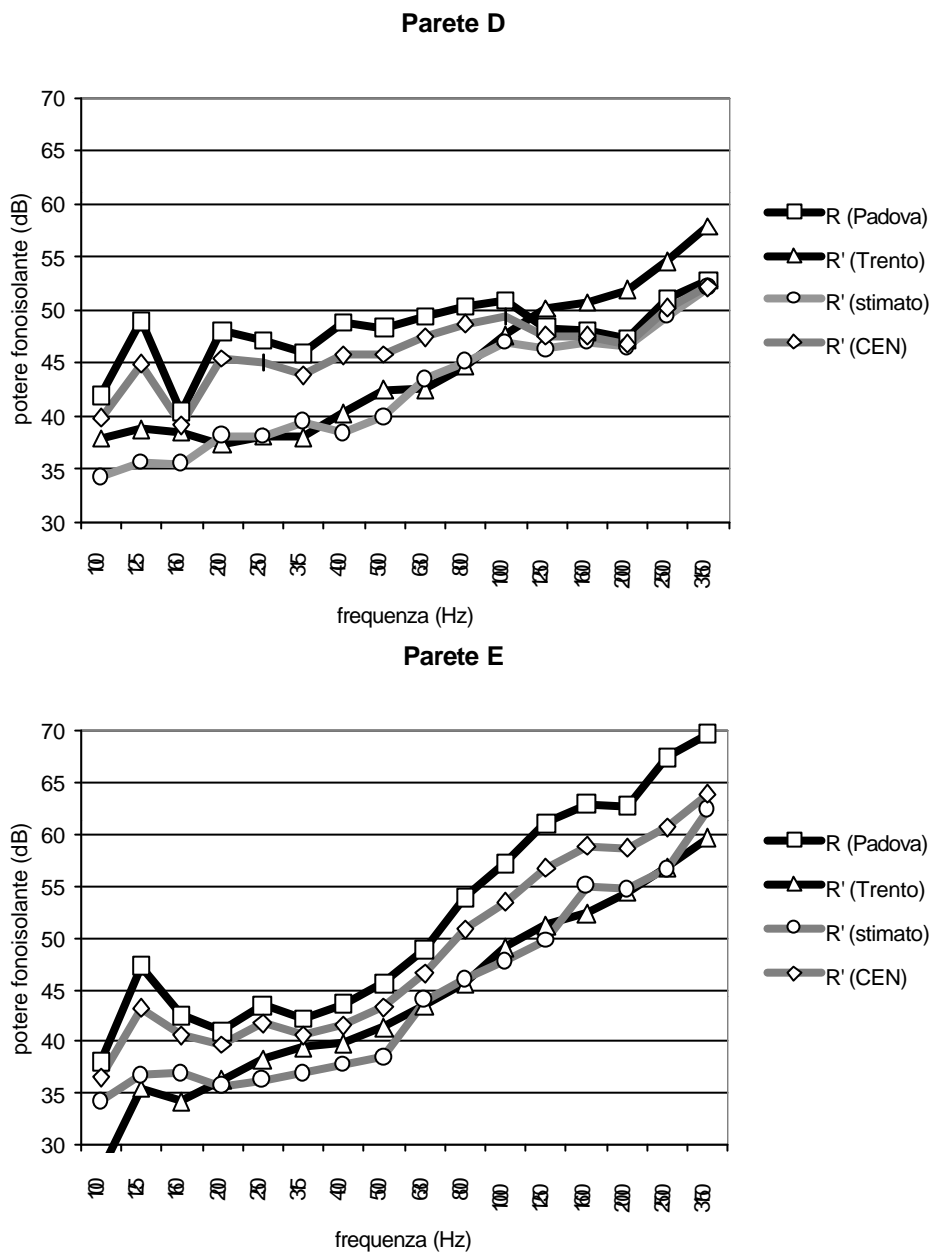
Fig. 5 - Dati sperimentali (△) e teorici (○,◇) del potere fonoisolante apparente R', al confronto con il valore del potere fonoisolante R (□)
