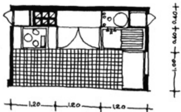
Figura 7. Servizi della zona giorno: elemento impianti e servizi della cucina.
