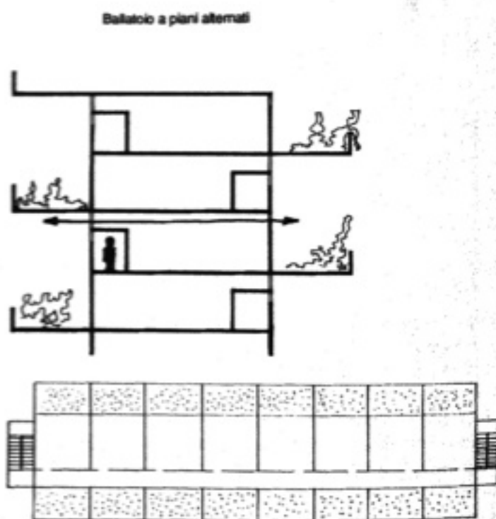
Figura 24. Schema associativo a ballatoio.
