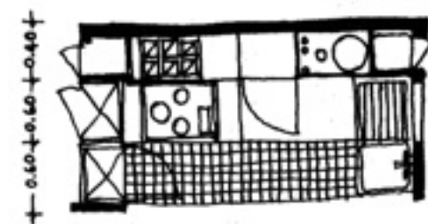
Figura 8. Servizi della zona giorno: elemento impianti e servizi della cucina.
