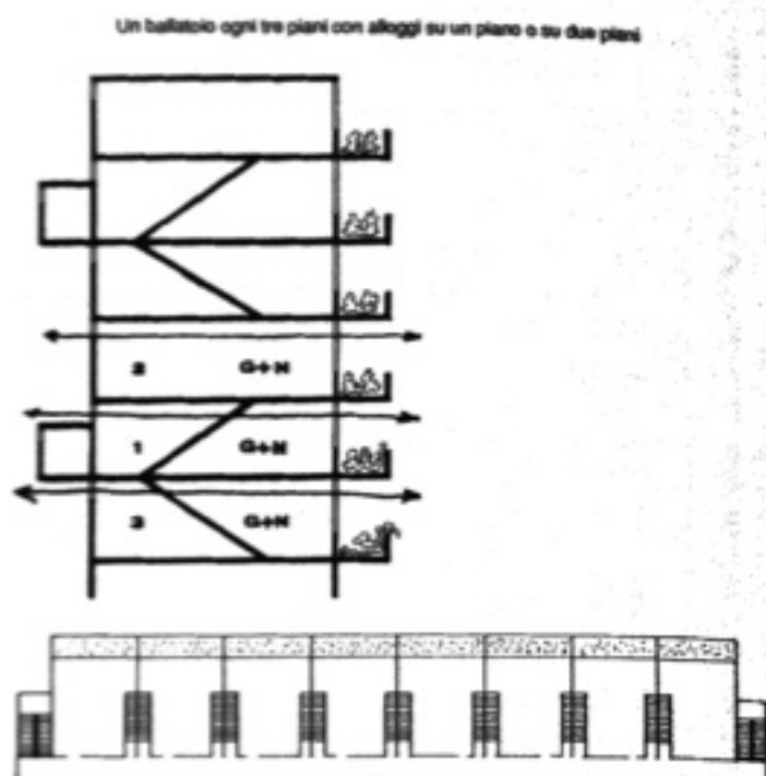
Figura 23. Schema associativo a ballatoio.
