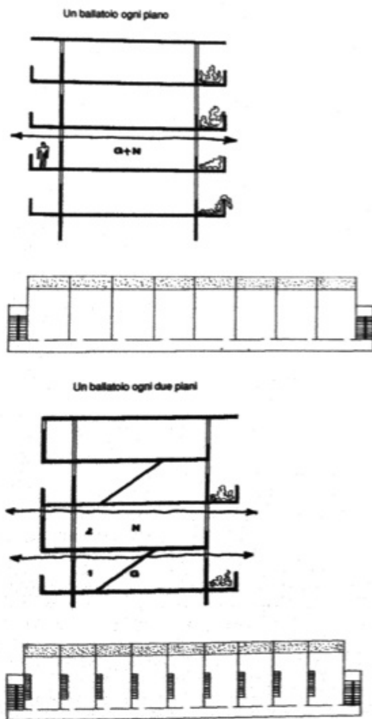
Figura 22. Schema associativo a ballatoio.
