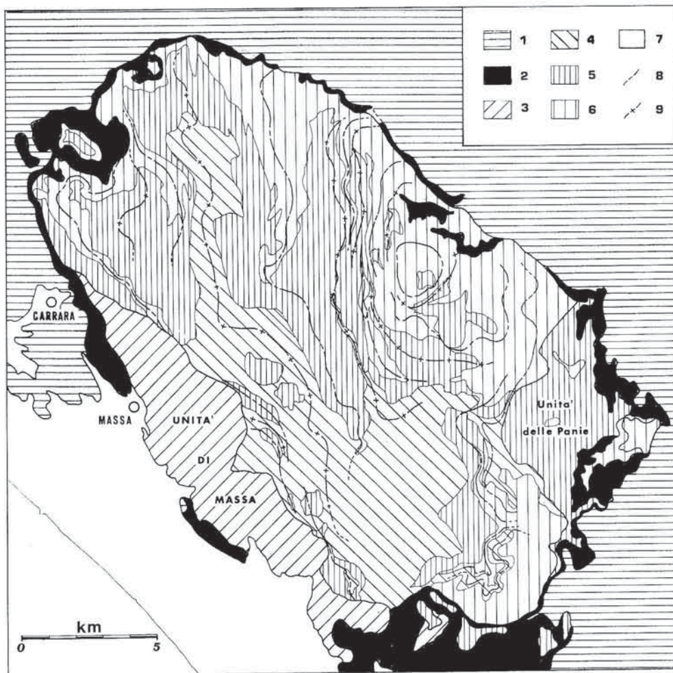
Fig. 4 - Schema geologico-strutturale della finestra tettonica delle Alpi Apuane: 1) Falda Toscana e Unità Liguri; 2) Breccie Poligeniche e "Calcare Caveroso" s.l.; 3) Unità di Massa; 4) Basamento paleozoico dell'Unità delle Alpi Apuane; 5) Formazioni di piattaforma carbonatica dell'Unità delle Alpi Apuane (Norico-Lias inferiore); 6) Formazioni (emi) e flysch dell'Unità delle Alpi Apuane (Lias-Oligocene); 7) Depositi alluvionali attuali e recenti; 8) Tracce dei piani assiali delle principali sinclinali di prima fase; 9) Tracce dei piani assiali delle principali anticlinali di prima fase (da CARMIGNANI e GIGLIA, 1984, ridisegnato e semplificato).
