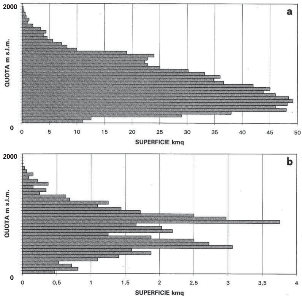
Fig. 11 - Grafici a barre relativi allo sviluppo areale per fasce di quota (a) e allo sviluppo areale delle superfici con pendenza < 33% (b) dell'area apuana.
