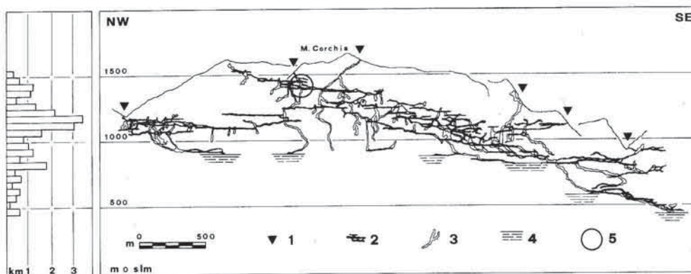
Fig. 12 - Sezione longitudinale schematica del Complesso Carsico del Monte Corchia. 1) Posizione delle principali ingressi del sistema; 2) Condotti di origine prevalentemente freatica; 3) Condotti di origine prevalentemente vadosa (pozzi e forre); 4) Livello attuale della zona saturata; 5) Zona di ritrovamento dei ciottoli arenacei. A sinistra: Grafico dello sviluppo planimetrico per fasce di quota dei condotti freatici del Corchia.
