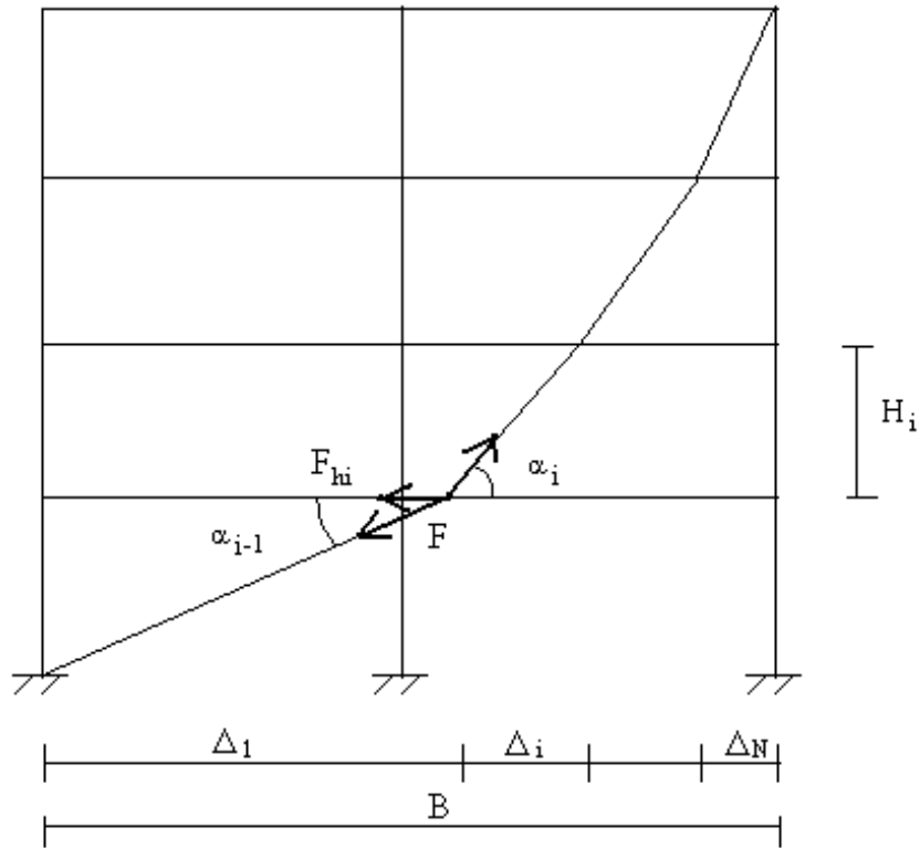
Fig. 3.1.4. Cable layout
