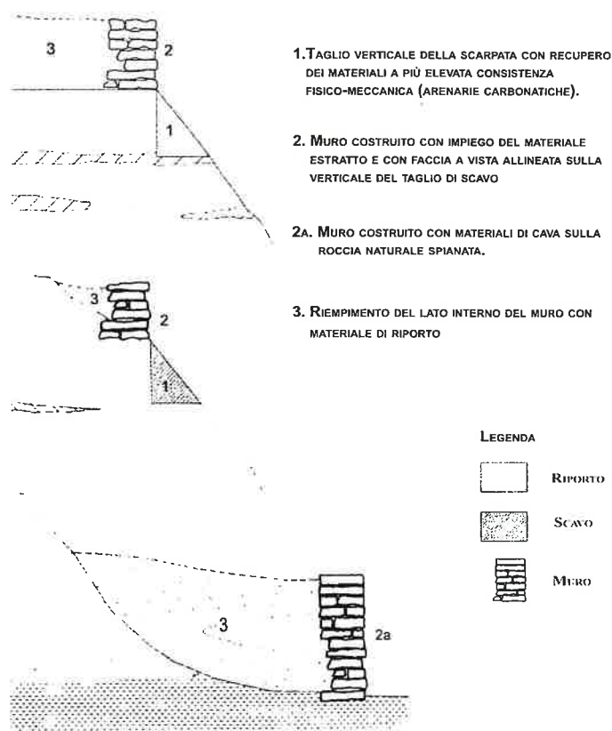
FIG. 8. Schemi di edificazione delle mura etrusche.
