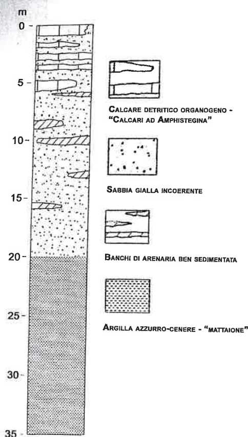
Fig. 7. Schema litostratigrafico del colle volterrano.
