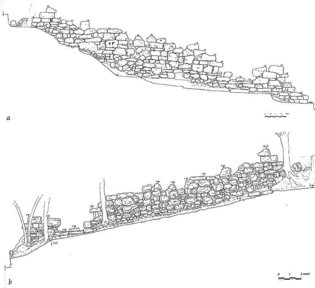
FIG. 10. Volterra. Località S. Andrea, muro etrusco. a) Prospetto principale; b) Prospetto tergale.
