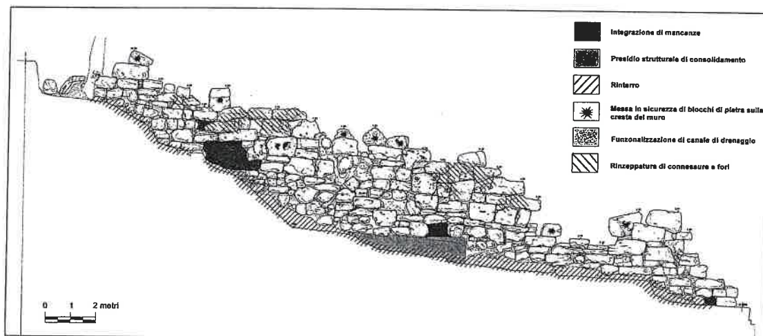
FIG. 13. Volterra. Località S. Andrea, muro etrusco: prospetto principale con proposta di interventi.
