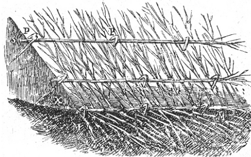
Fig. 6 – Brush mattress [Viappiani 1923]
