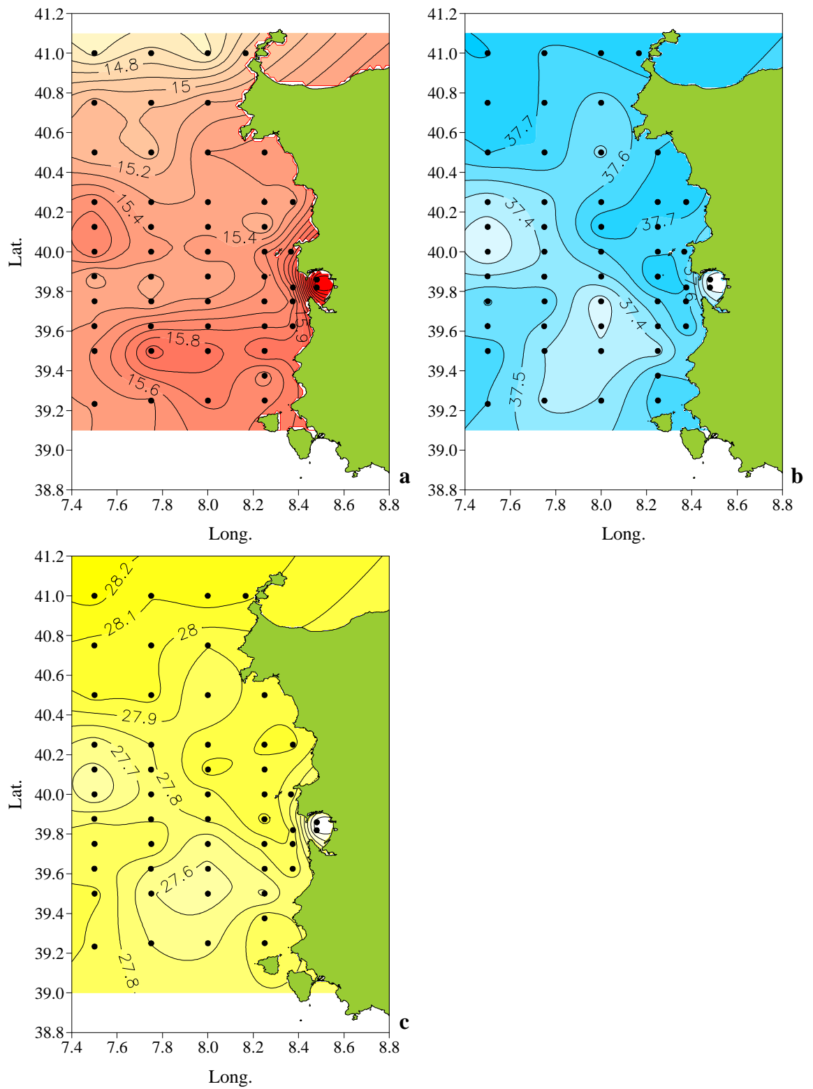
Fig.5 - Mar di Sardegna, aprile 2001. Distribuzione superficiale di: a) temperatura (°C); b) salinità, ‰; c) densità, kg m -3 .
