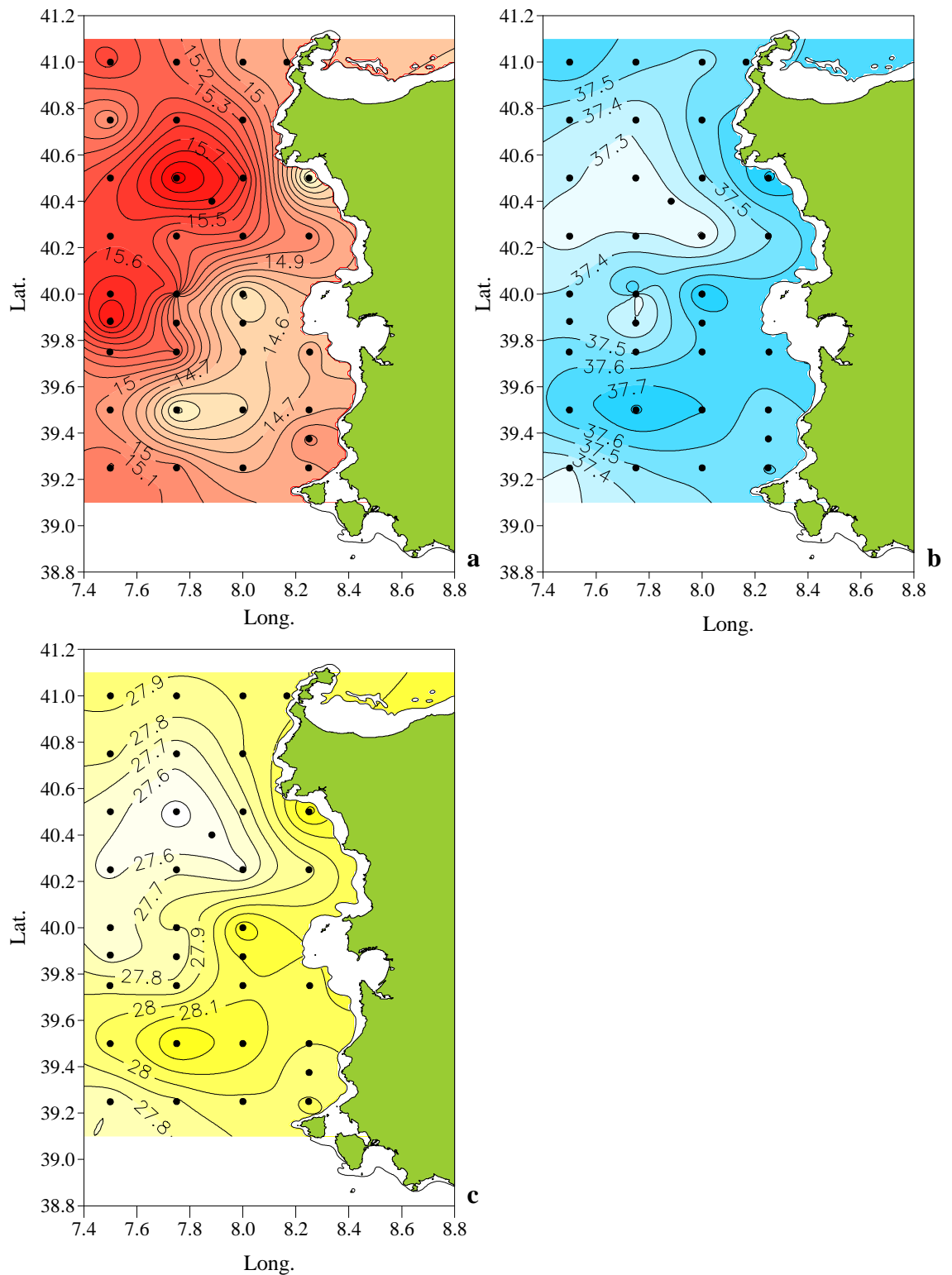
Fig. 12 - Mar di Sardegna, maggio 2002. Distribuzione a 50 m di: a) temperatura, °C; b) salinità, ‰; c) densità, kg m -3 .
