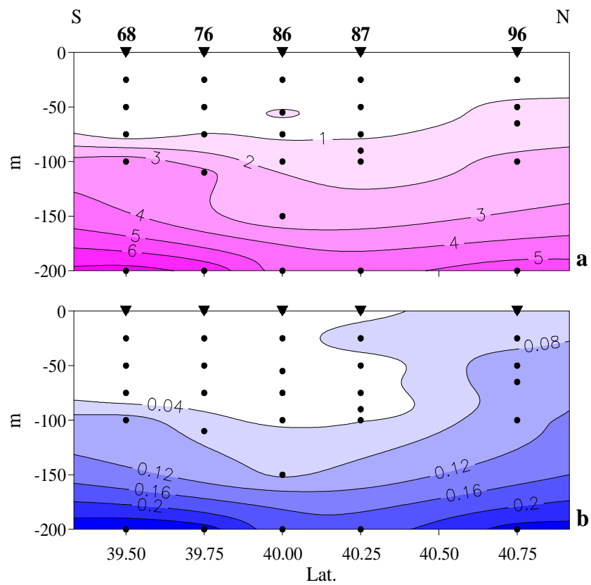
Fig. 15 - Mar di Sardegna, maggio 2002. Distribuzione verticale alla long. 7°5'E delle concentrazioni ( \mu\text{M} ) di: a) DIN; b) DIP.
