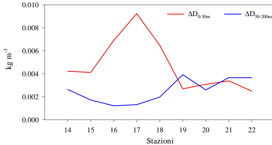
Fig. 20 - Mar Tirreno Centrale, maggio 2004. Variazione degli indici di stabilità, \Delta D_{0-50m} e \Delta D_{50-200m} , lungo la sezione verticale alla lat. 41°0'N.
