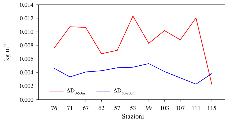
Fig. 8 - Mar di Sardegna, Aprile 2001. Variazione degli indici di stabilità, \Delta D_{0-50\text{ m}} e \Delta D_{50-200\text{ m}} , alla longitudine 7°5'E.
