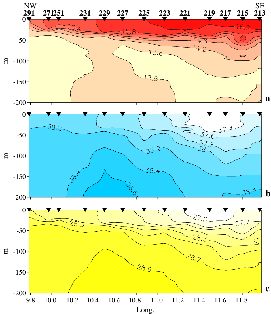
Fig. 23 - Mar Tirreno Meridionale, maggio 2004. Distribuzione verticale lungo il transetto A di: a) temperatura, °C; b) salinità, ‰; c) densità, kg m -3 .
