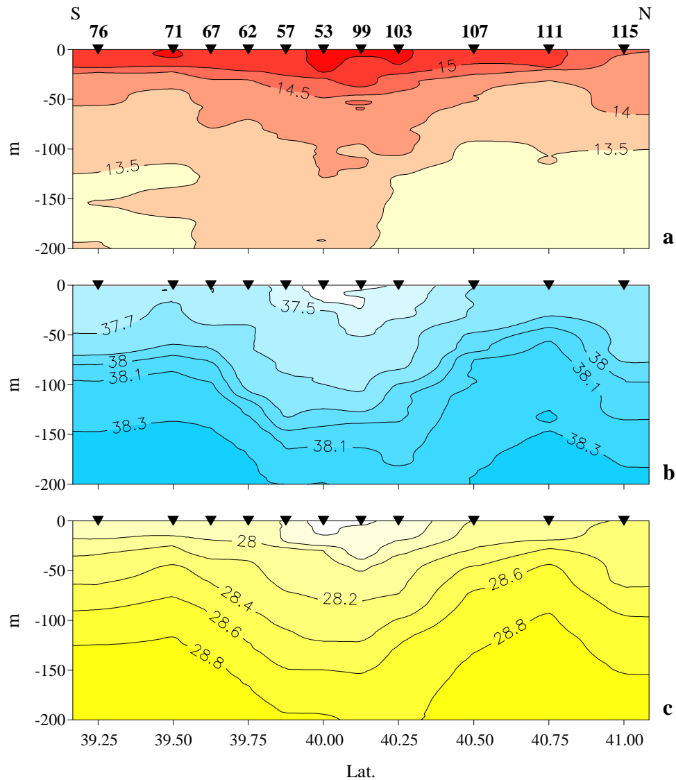
Fig. 7 - Mar di Sardegna, aprile 2001. Distribuzione verticale alla long. 7°5'E di: a) temperatura, °C; b) salinità, ‰; c) densità, \text{kg m}^{-3} .
