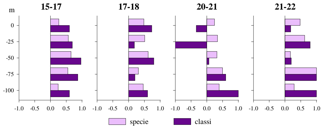
Fig. 43 - Mar Tirreno Centrale, maggio 2004. Coefficiente di correlazione \tau tra le stazioni alla lat. 41^{\circ}0'N a parità di strato.
