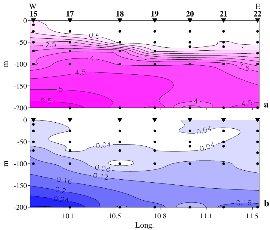
Fig. 21 - Mar Tirreno Centrale, maggio 2004. Distribuzione verticale alla lat. 41°0'N delle concentrazioni ( \mu\text{M} ) di: a) DIN; b) DIP.
