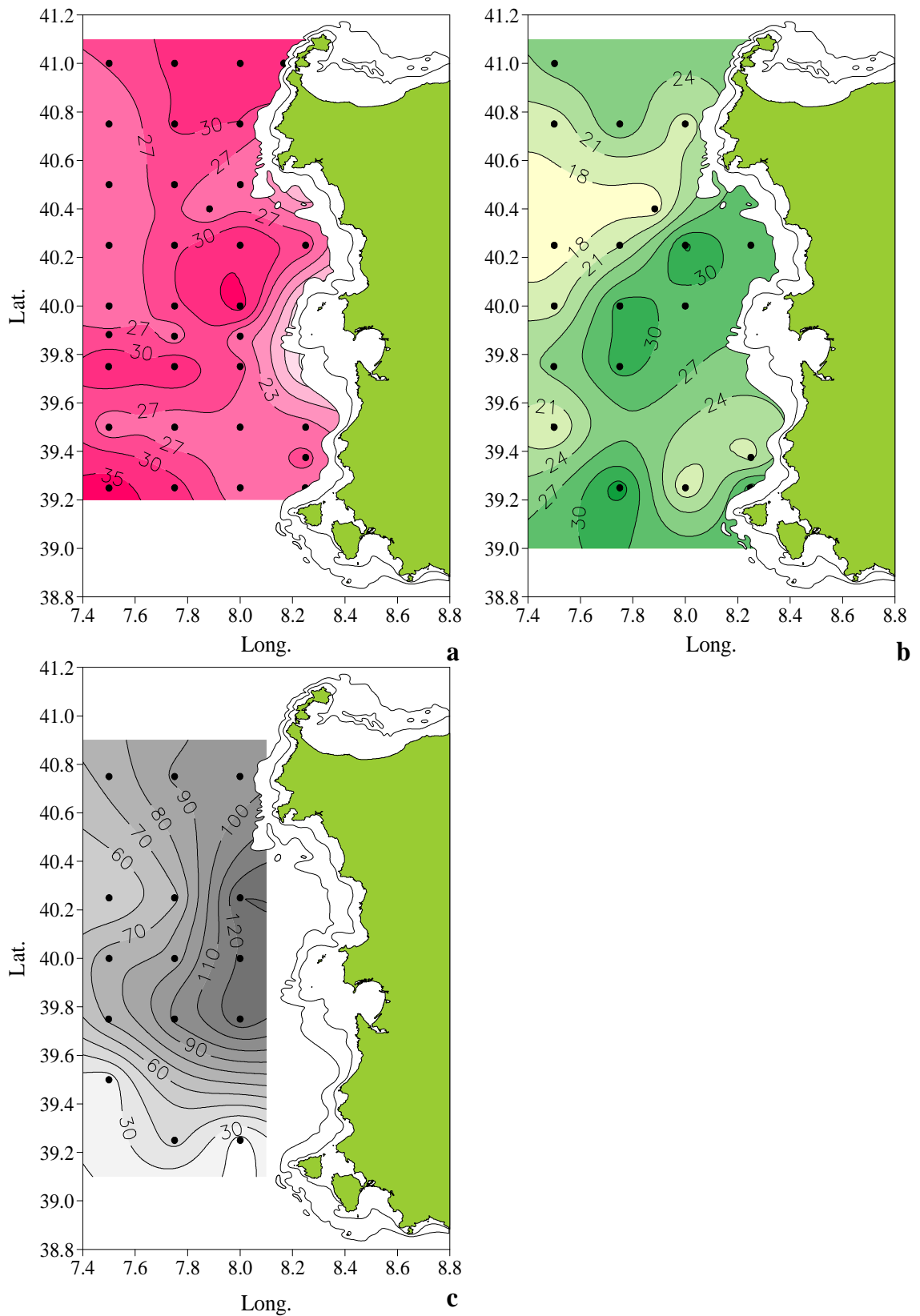
Fig. 30 - Mar di Sardegna, maggio 2002. Distribuzione dell'integrale tra 0 e 100 m ( \text{mg m}^{-2} ) di: a) fluorescenza corretta; b) clorofeopigmenti; c) densità cellulare ( \times 10^6 \text{cell m}^{-2} ).
