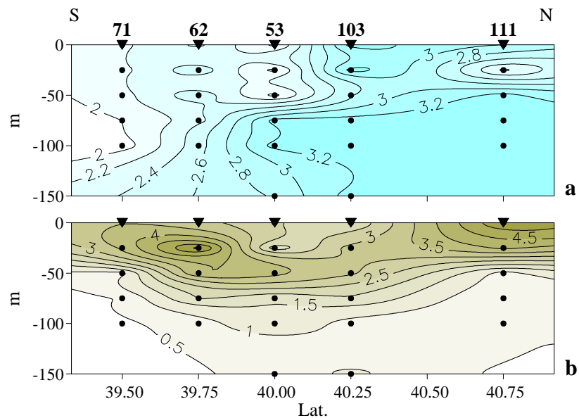
Fig. 10 - Mar di Sardegna, aprile 2001. Distribuzione verticale alla long. 7°5'E di: a) concentrazioni ( \mu\text{M} ) dell'azoto ammoniacale; b) rapporto tra azoto ammoniacale e DIN.
