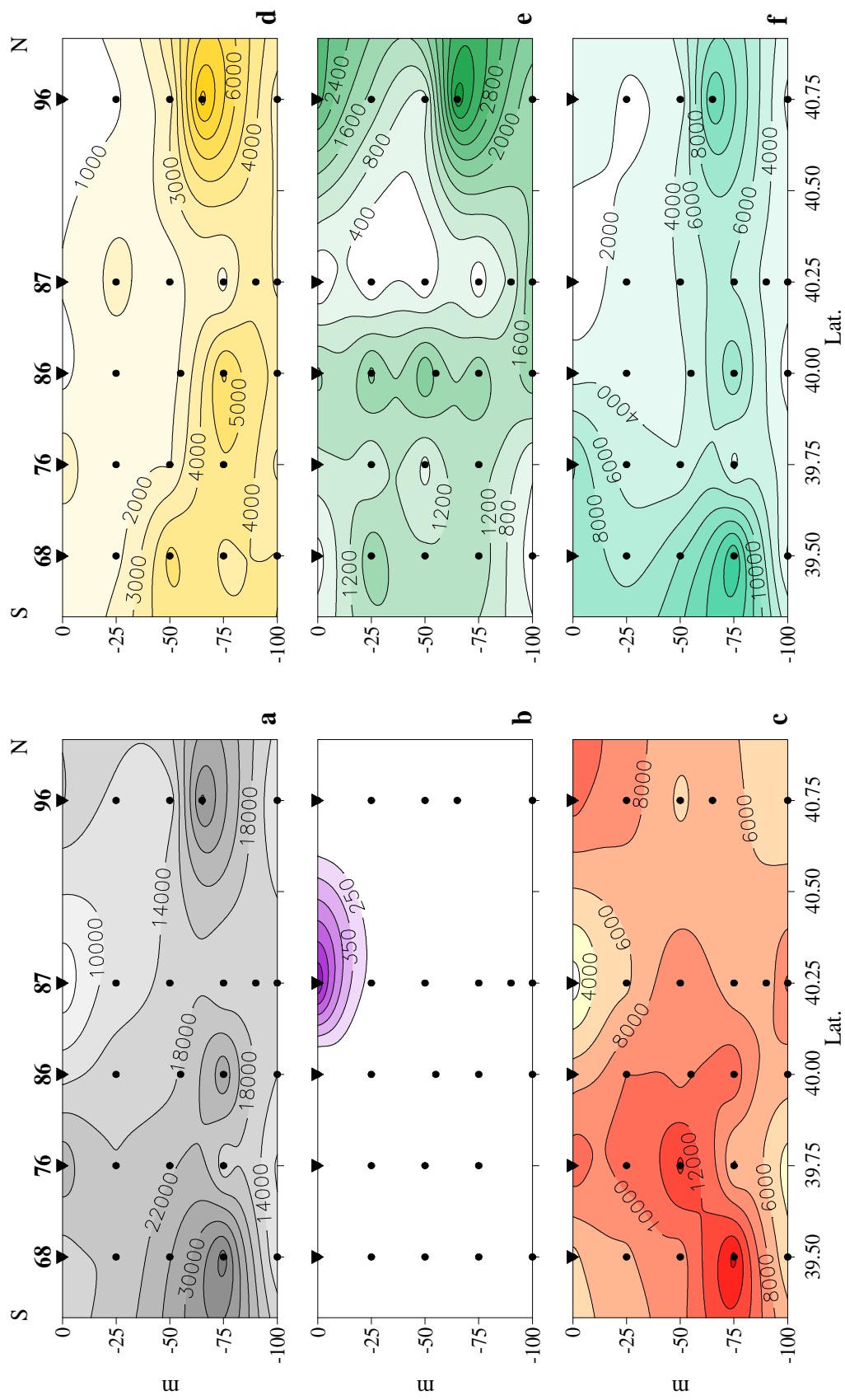
Fig. 34 - Mar di Sardegna, maggio 2002. Distribuzione verticale delle densità fitoplanctoniche (cell L -1 ): a) totale; b) diatomee; c) dinoflagellati; d) coccolitoforidee; e) Cryptomonadaceae ; f) flagellati nanoplanctonici.
