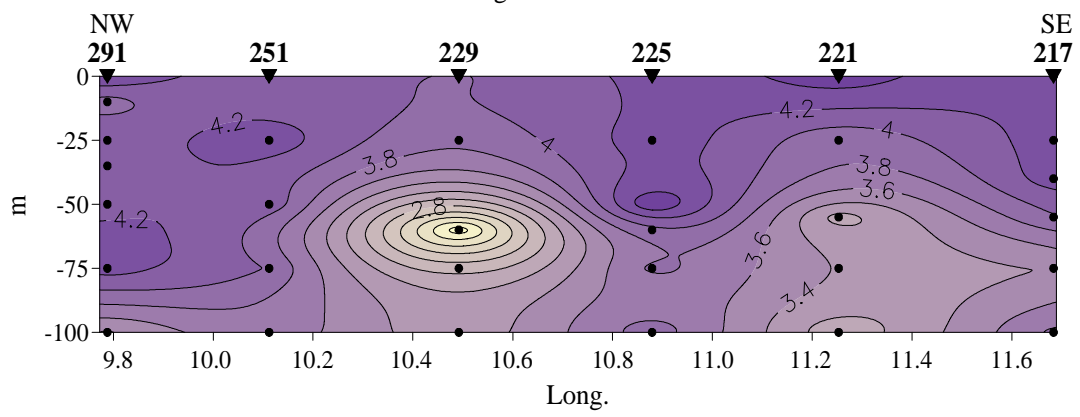
Fig. 37 - Distribuzione verticale della diversità specifica H' (Shannon): a) Mar di Sardegna, aprile 2001; b) Mar di Sardegna, maggio 2002; c) Mar Tirreno Centrale, maggio 2004; d) Mar Tirreno Meridionale, maggio 2004.
