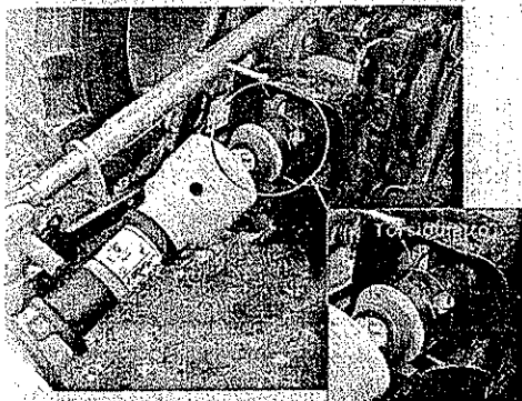
► Fig. 3 - Torsiometro interposto fra cardano e presa di potenza.
