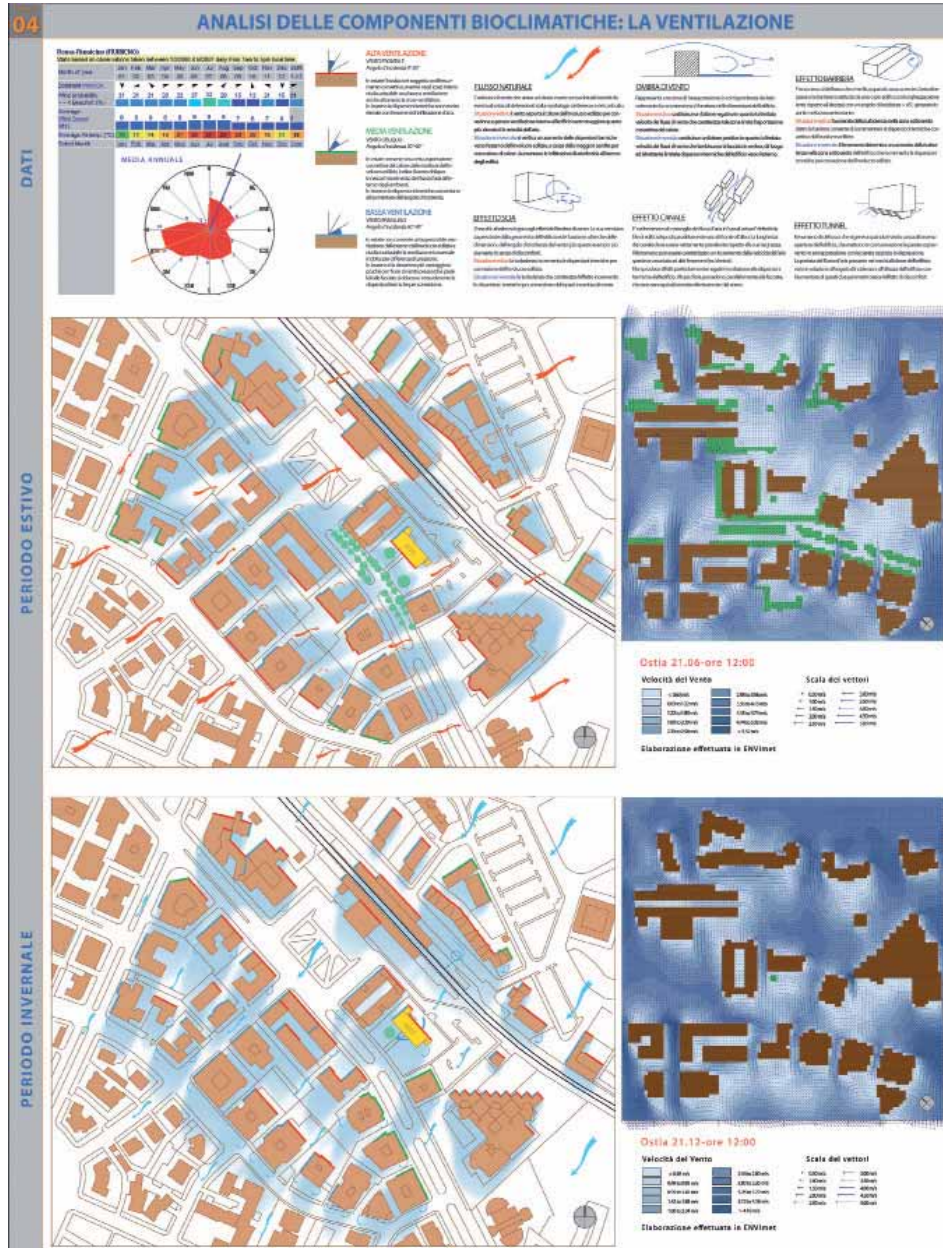
Fig. 1.10 Master di Il Livello, Architettura Bioecologica e Tecnologie Sostenibili per l’Ambiente, 2007. Analisi e valutazione delle condizioni di Ventilazione (Software Envimet) nell’ambito del progetto di recupero dell’Asilo nido “Il Sagittario”, Roma. Arch. Mario Piccirillo.
