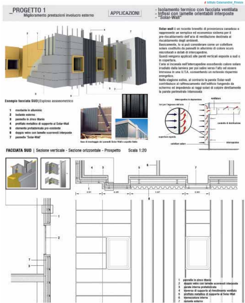
Fig. 1.15 Master di II Livello, Architettura Bioecologica e Tecnologie Sostenibili per l'Ambiente, 2008. Adeguamento energetico e ambientale del complesso "Casa dello studente" a Scandicci, Firenze. Arch. Spaziani.
