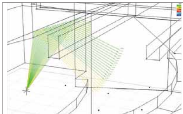
Fig. 7 Analisi acustica sul riverbero dei suoni in un interno. (Fonte Autodesk).
