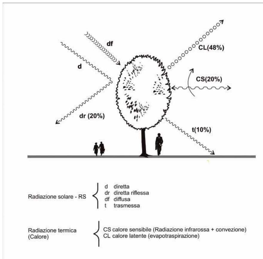
Fig. 2.17 Flussi energetici intorno ad un albero.
