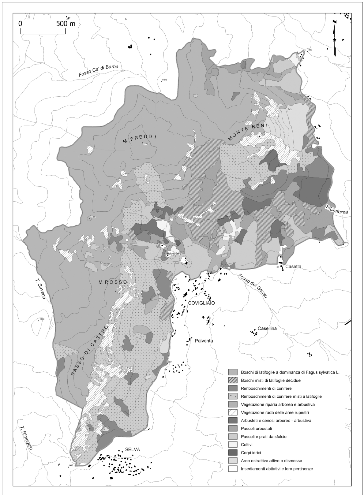
Fig. 3 - Carta della vegetazione fisionomico-floristica del SIC/SIR «Sasso di Castro e Monte Beni».
