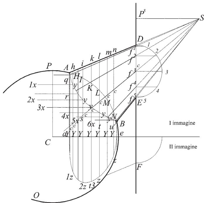
Fig.120c. Determinazione della proiezione orizzontale dello spigolo superiore interno del lunotto.
