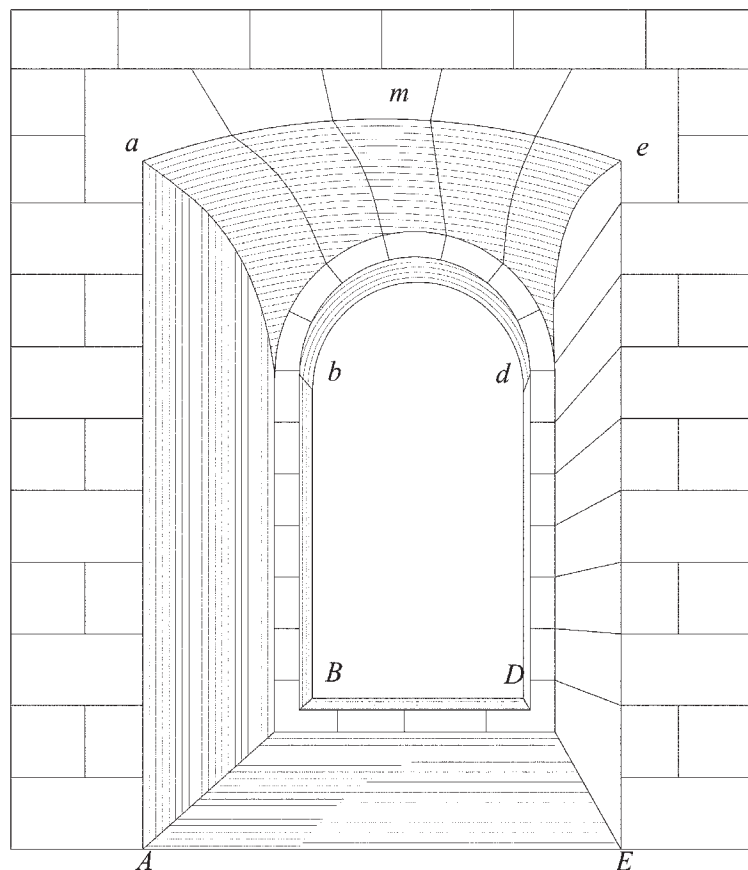
Fig. 235 L'arrière-voussure de Marsiglia ordinaria.
