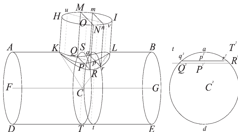
Fig. 59 L'incontro dei due cilindri, retti e ineguali, forma la figura non piana KQLR detta Cicloimbre.
