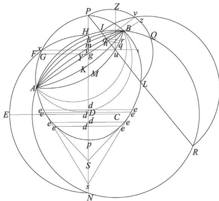
Fig. 101 Si può considerare uno sferoide come un'infinità di piccoli tronchi di cono ed è proprio su questo presupposto che si basa la teoria del taglio delle pietre.
