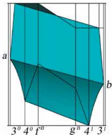
Fig. 227 a Cuneo concavo convesso sul lato del Nocciolo alla cui formazione si perviene in modo analogo al cuneo concavo della fig. 229. Vista ortogonale al piano d'intradosso.
