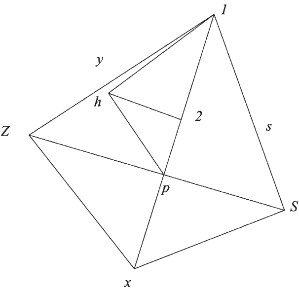
Fig. 92 Rappresentazione dell'angolo ZxS trovato per assemblare gli intradossi piani
