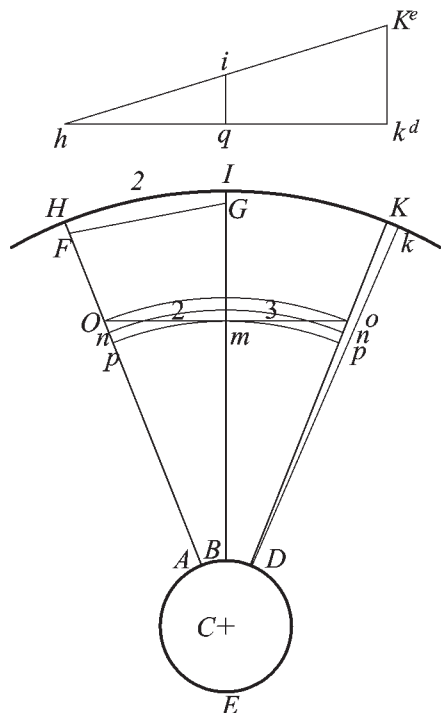
Fig. 180 Costruzione di gradini per una scala a chiocciola a nocciolo pieno
