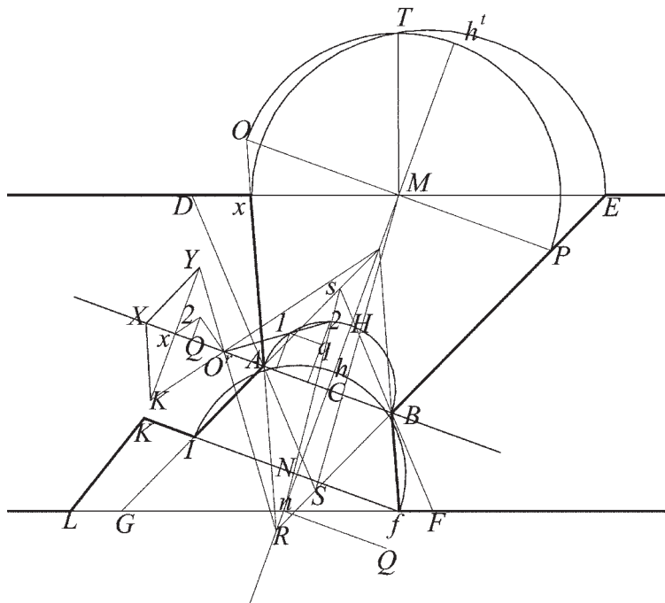
Fig. 105: Costruzione di un'Embrasure sbieca voltata, realizzata in un muro avente la parete esterna a scarpa e quella interna a piombo. O in 1-2, si prolungherà la corda 1-2 dal Collet, fino all'intersezione col diametro AB, che questa incontrerà in O', per il quale e per i vertici dei conici s, R, si traceranno delle linee sO'K, RO'V, che saranno le sezioni Nota 4: Per la costruzione dei due tronchi di cono, profili esterno ed interno dell'Embrasure, vedi il Tomo Secondo, pag. 222.
