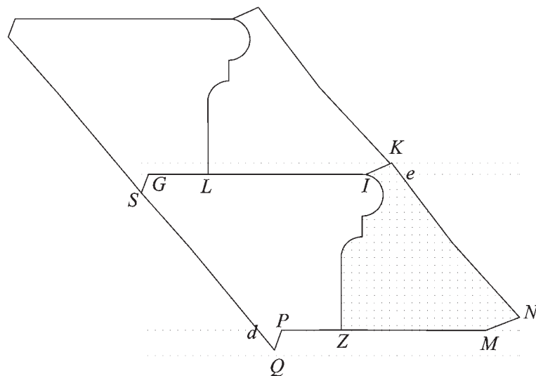
Fig. 192 Sezione in prossimità della testa, che mostra la sovrapposizione di due conci, 19 Nella Fig. 192 si è aggiunta la lettera K mancante.
