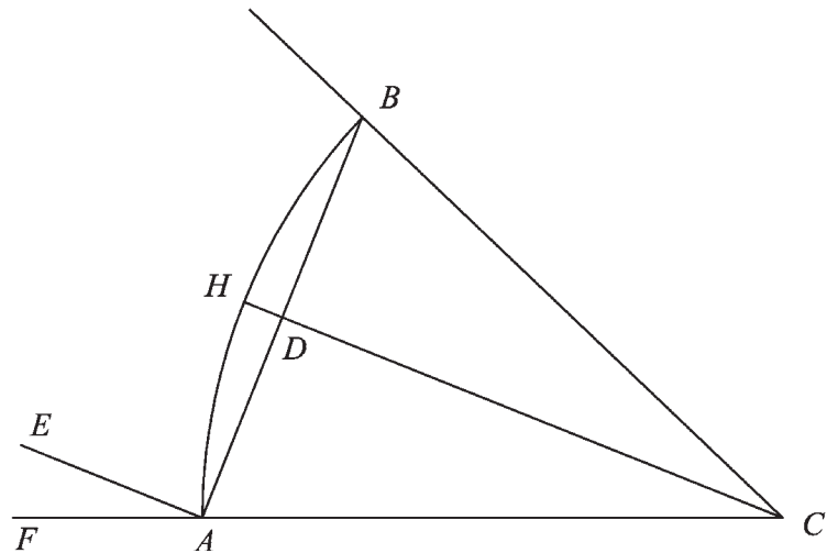
Fig. 56 La figura mostra il rapporto di proporzione che intercorre tra gli angoli e le corde di un arco di circonferenza.
