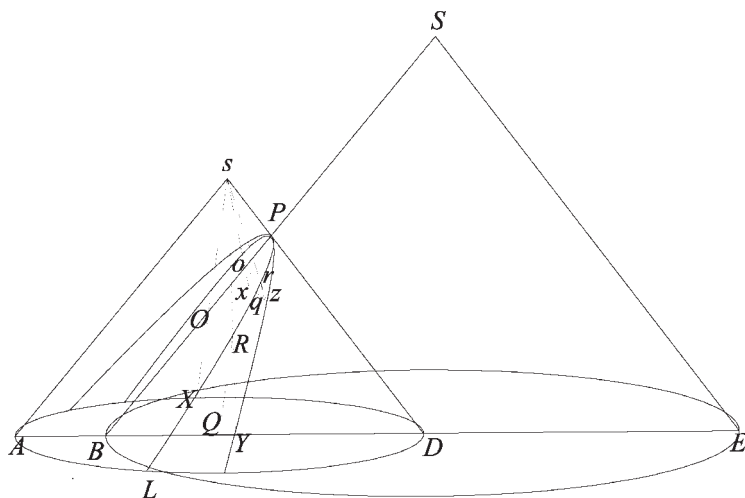
Fig 85. Sezione data dall'intersezione di due coni diversi ma simili in cui assi e lati sono paralleli
