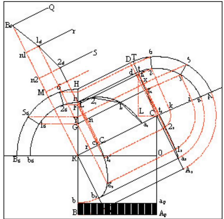
Fig 86. Discesa retta a scarpa sul davanti e a piombo sul di dietro
