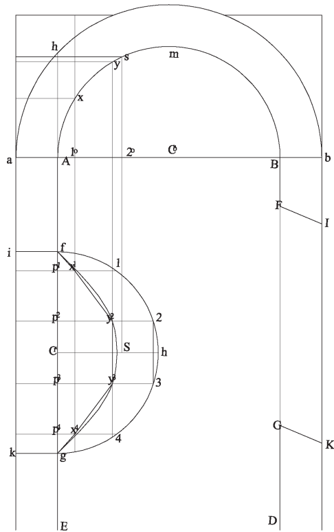
Fig. 30.2 Lunetta diritta tracciata seguendo il procedimento utilizzato per la lunetta di sbieco come indicato da Frézier.
