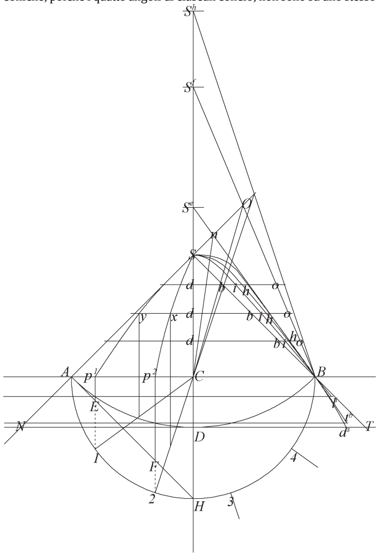
Fig.134 b Costruzione del ribaltamento delle linee di giunzione e loro proiezione orizzontale
