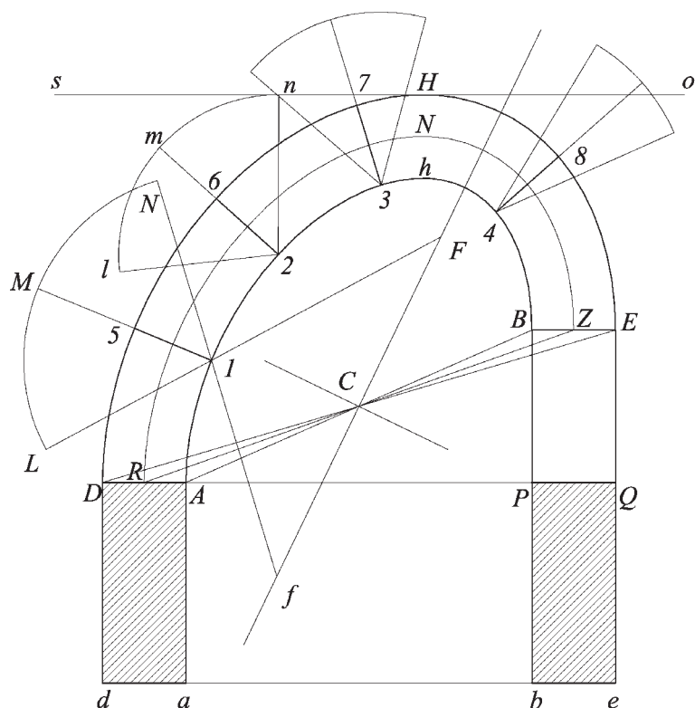
Fig. 61 La figura mostra i rapporti geometrici in una Volta a Botte Rampante. Fig. 60 o rampante come in Fig. 61 . Essendo la curvatura divisa nei suoi conci e la direzione determinata come nel metodo visto precedentemente, si tireranno le corde degli archi A1, 12, 13 ecc, e data la lunghezza del piedritto sarà tracciato tutto il disegno in scala.
