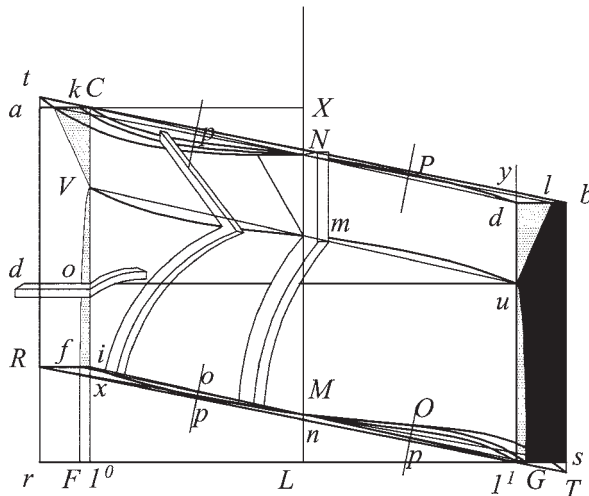
Fig. 229 Cuneo concavo del lato della Torre con i diversi calandrini necessari alla sua formazione. Vista ortogonale al piano d'intradosso. Le curve sulle corde, eliche, sono esasperate per visualizzare la concavità e la convessità rispetto le corde per tre punti che altrimenti sarebbe minima.
