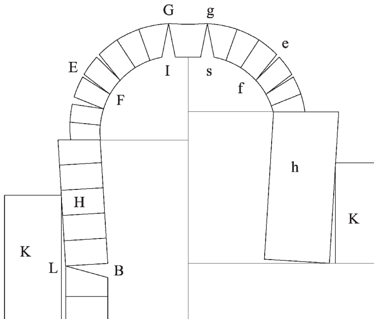
Fig. 236 Rappresentazione di una piccola volta in gesso a tutto sesto, composta da 5 pietre.
