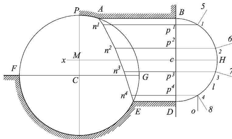
Fig. 89a Proiezione dello spigolo di volta
