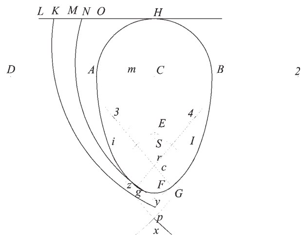
Fig.158: Costruzione attraverso archi di cerchio dell'ovale appuntito, chiamato in architettura Ove; è una figura a cui v'è venuto spesso l'occhio nelle cornici, come quando, in quattro parti, & si prolunghi questo diametro da una parte & dall'altra, di tre quarti della sua lunghezza in modo che DA & B2 siano
