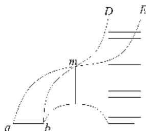
Fig. 194 Proiezione orizzontale della staffa
