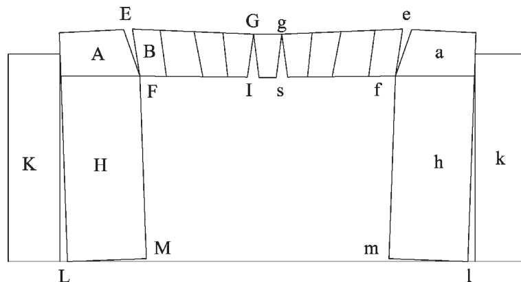
Fig. 240 Rappresentazione di una piatta banda di 9 chiavi di volta
