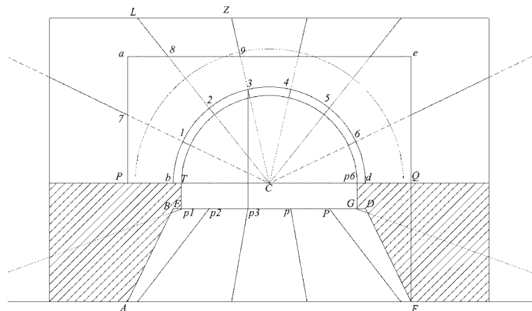
Fig. 261A - Costruzione della volta di Montpellier attraverso il primo metodo sopradescritto in cui le facce dei conci sono perpendicolari alla circonferenza del battente.
