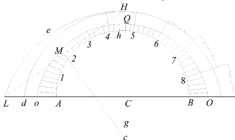
Fig. 48 Costruzione di un arco di cerchio con raggio Qo, che sarà utile dare l'istrutto per i centri del mezzo cerchio interno e di 120°.
