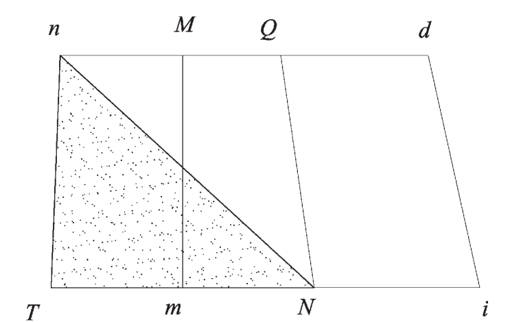
Fig.90 Rappresentazione del concio della volta sferica
