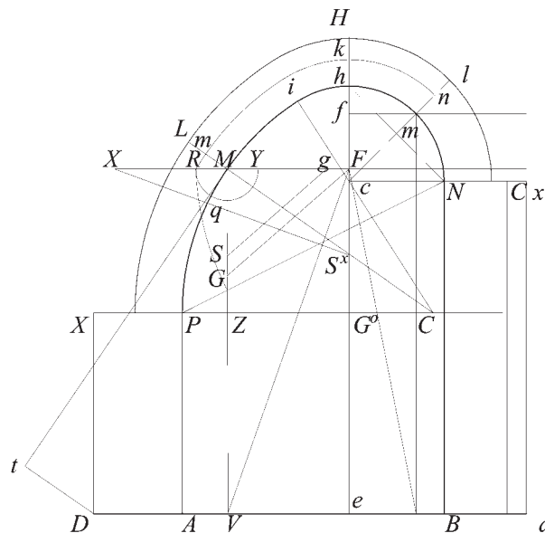
Fig. 217 Costruzione di una volta ellittica a sesto rampante.
