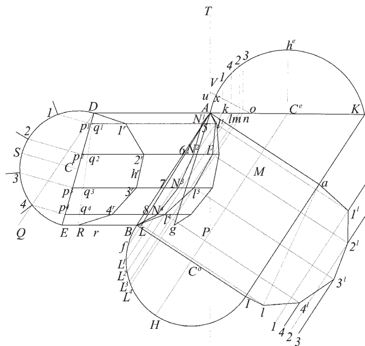
Fig.54 sviluppo dell'incrocio che la volta in pendenza fa penetrando
