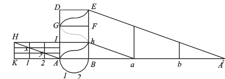
Fig. 281b Sviluppo di un'ellisse su una superficie cilindrica o conica
