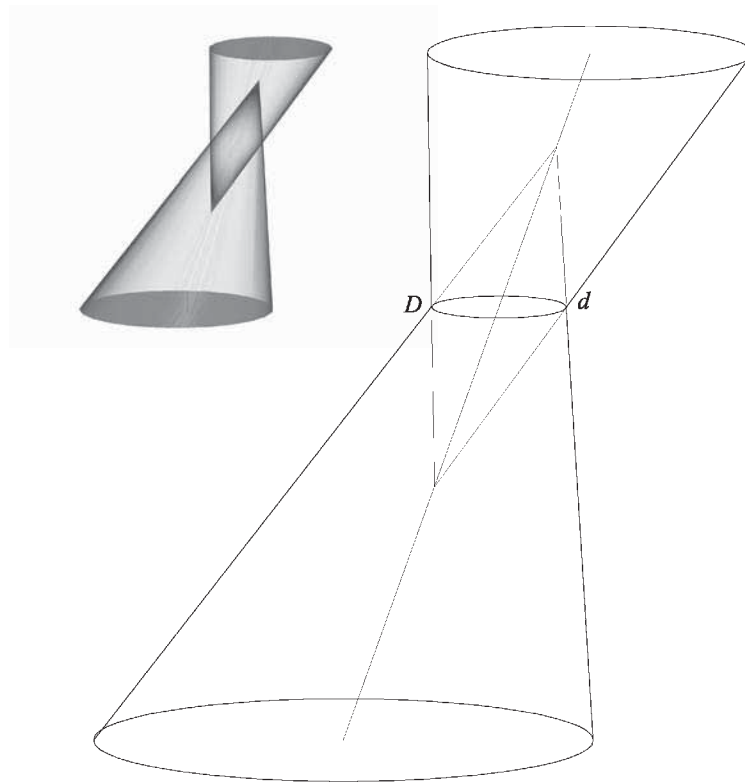
Fig 84. Intersezione di coni in cui gli assi si confondono e le basi sono parallelamente lontane
