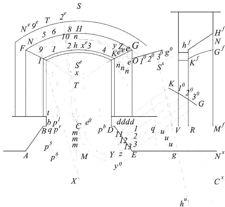
Il piano orizzontale del vano da voltare supposto come nel disegno Fig. 138b , e l'arco di taglio dato HNK , il cui centro è C , precedente della Fig. 138b , e l'arco di taglio dato HNK , il cui centro è C ,
