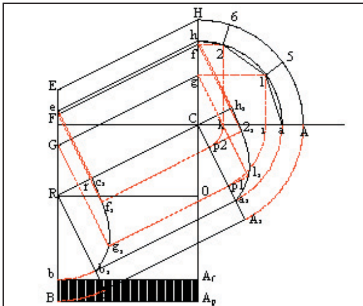
Fig 84. Proiezione dell'arco-retto ribassato
