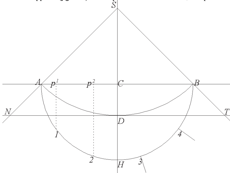
Fig. 134 a Proiezione dello sbalzo ( ADB ) della torre e ribaltamento ( AHB ) della sezione di torre tagliata con un piano passante per A e B
