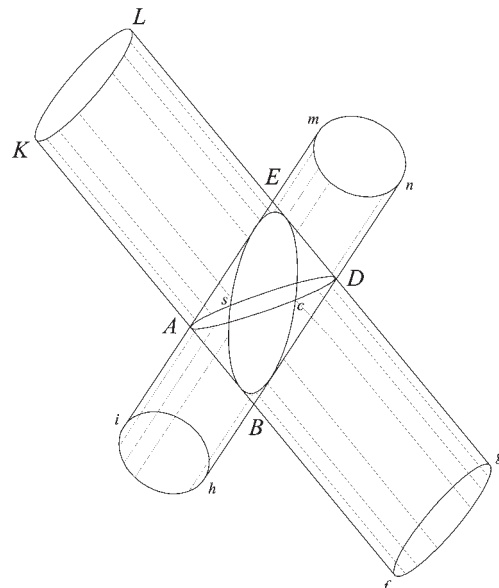
Fig. 58 I due ellissi AD e BE sono formati dall'incrocio dei due cilindri ineguali ma di ugual diametro.
