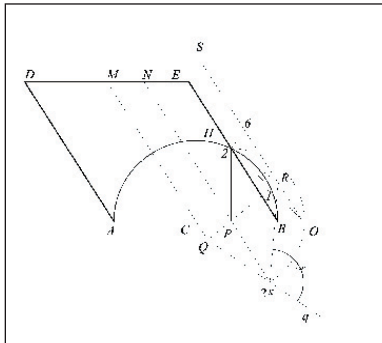
Fig.318 L'angolo del calandrino cercato è 105°
