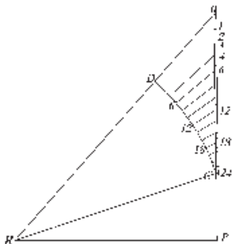
Fig. 138 Allungare o accorciare il contorno della spirale.
