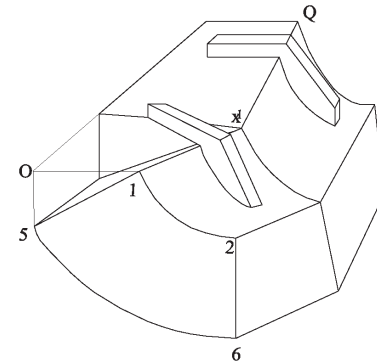
Fig. 31 Taglio di un concio.
