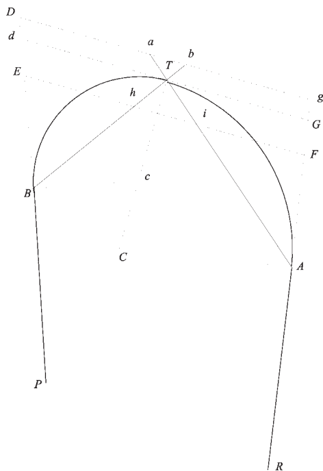
Fig.154: Imitazione di un'ellisse costruita da archi di circonferenza i cui raggi non appartengono alla stessa retta
