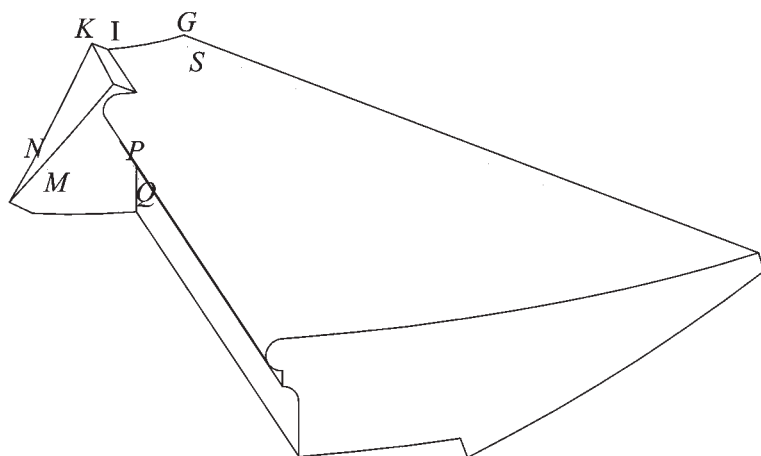
Fig. 191 Sezione in prossimità dell'incastro, che mostra la sovrapposizione di due conci e la parte di pietra da asportare dal pannello di partenza evidenziata dalla rigatura verticale.
