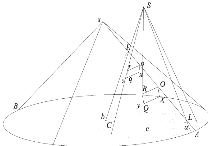
Fig 86. Sezione fatta dall'incontro di due coni con assi paralleli e con due lati che si
