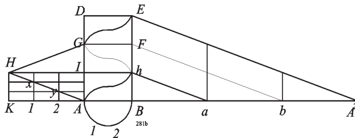
Fig. 281c Sviluppo se si esegue una rivoluzione intera
