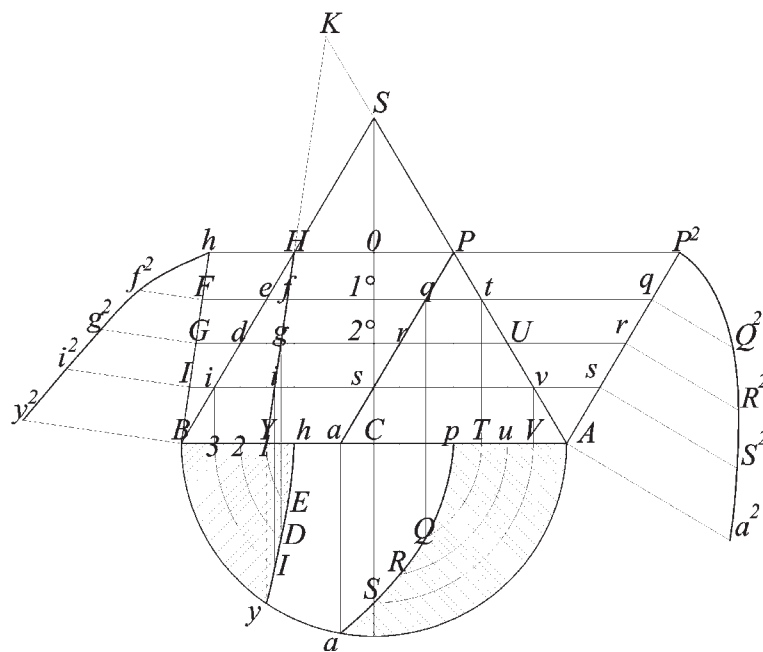
Fig. 184 d Sezione del cono: iperbole
