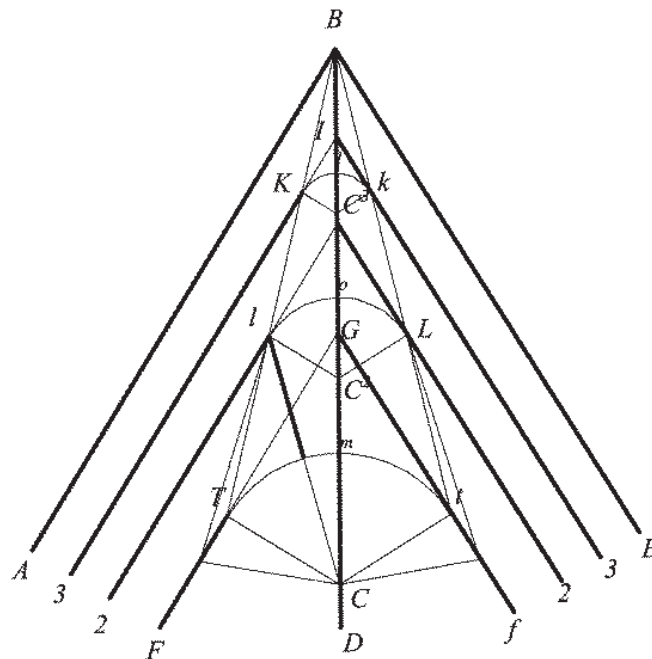
fig. 28 arrotondamento conico del cono retto della base TC , tC , si avrà sulla diagonale Cb i punti c^2 e c^3 che saranno i centri dell'arrotondamento dei letti di ogni base, i cui raggi saranno le
