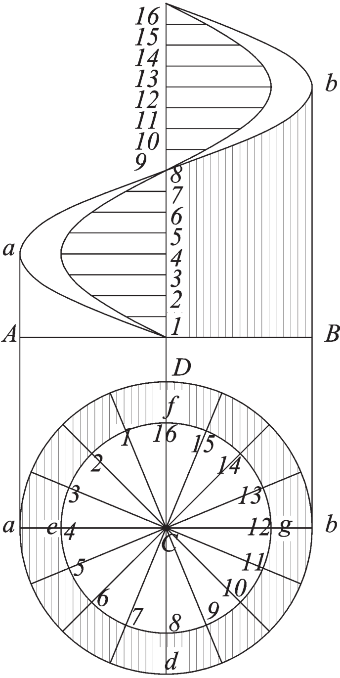
Fig. 249. 2 Rappresentazione della scala dentro la torre
