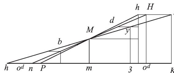
Fig. 183 Proiezione dell'inclinazione della scala
