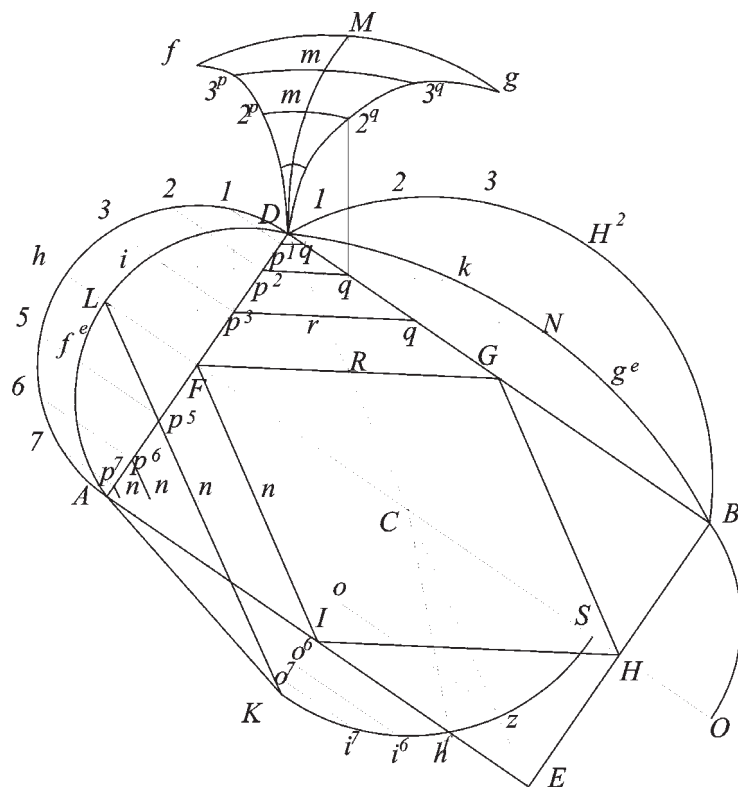
Fig. 213d Sviluppo dei pennacchi.
