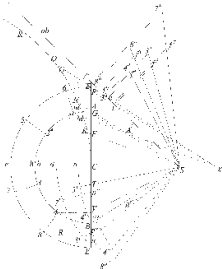
Fig. 83d due intradossi sullo spigolo come nel Disegno citato.
