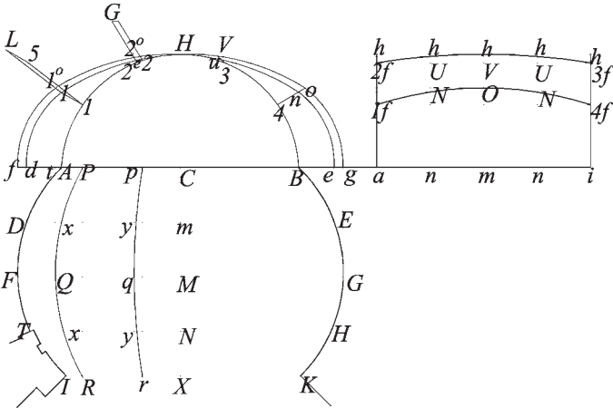
Fig.251b proiezione orizzontale e verticale dei giunti all'intradosso della volta
