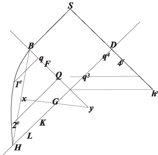
Fig.122b.Costruzione per trovare i giunti di letto
