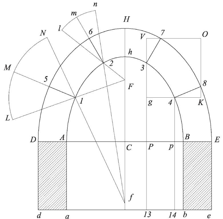
Fig. 60 Rapporti geometrici in una Volta a Botte a Sesto Rialzato.
