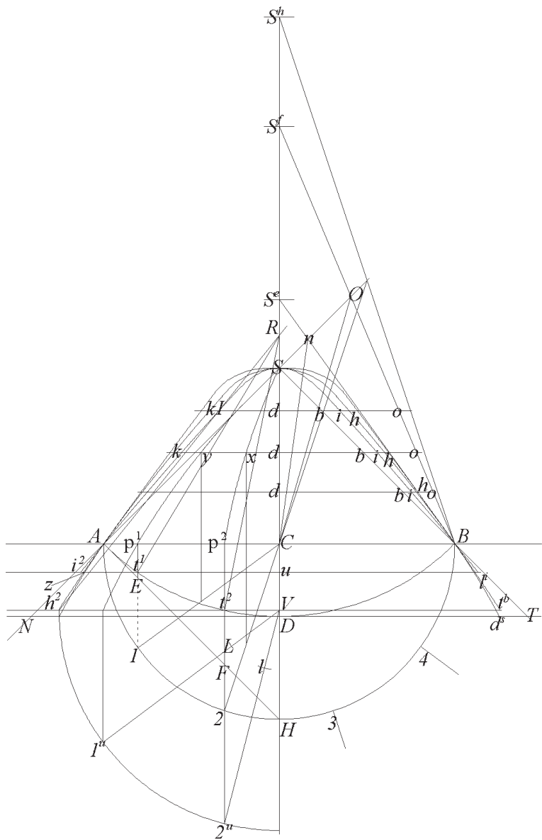
Fig.134 c Costruzione delle piramidi con facce piane dalle quali, sottraendo pietra, si ricaveranno i conchi
