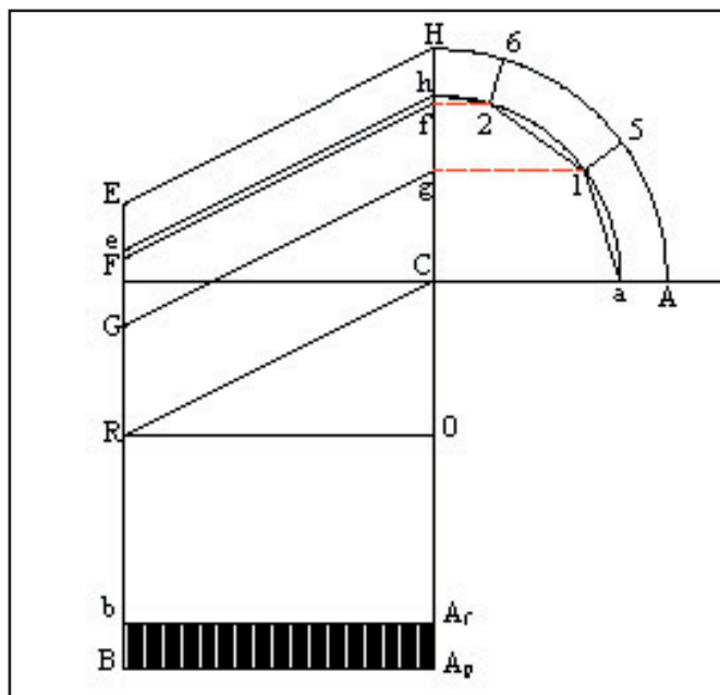
Fig 84. Linea di rampa, quarto di cerchio d'intradosso e d'estradosso diviso in due conci e mezzo, e profilo della volta
