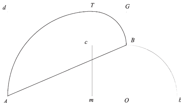
Fig.155: Costruzione di un arco rampante in cui i piedritti sono paralleli e la linea di sommità dG è orizzontale
