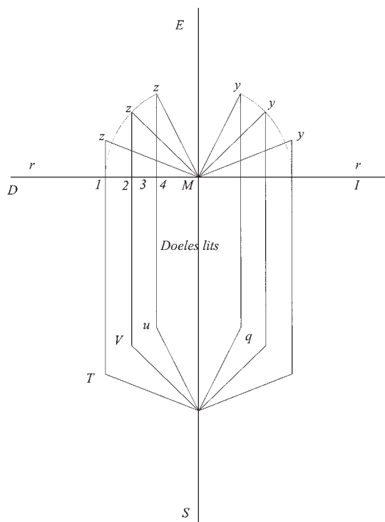
Fig.98 costruzione per evidenziare le doeles e i lits.
