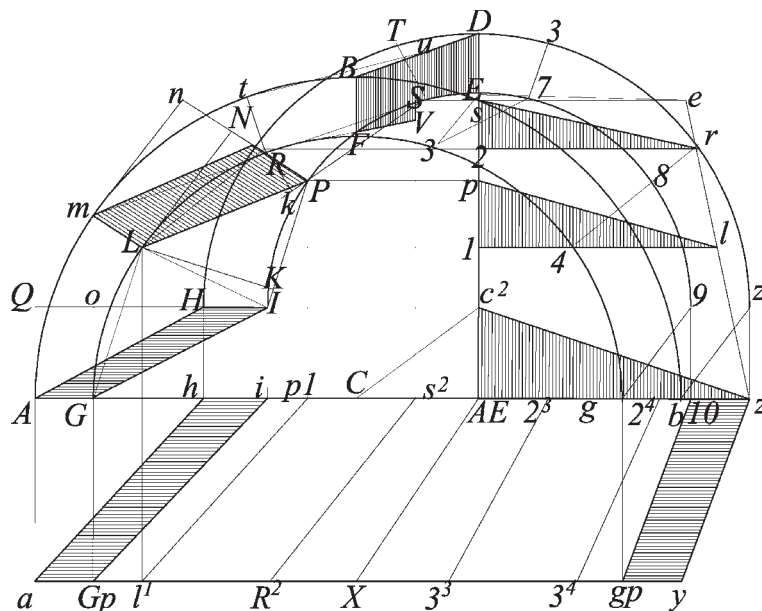
Fig.285 Proiezione orizzontale della volta e proiezione verticale con i joins de lit in vera grandezza e i panneaux de lit e di testa
