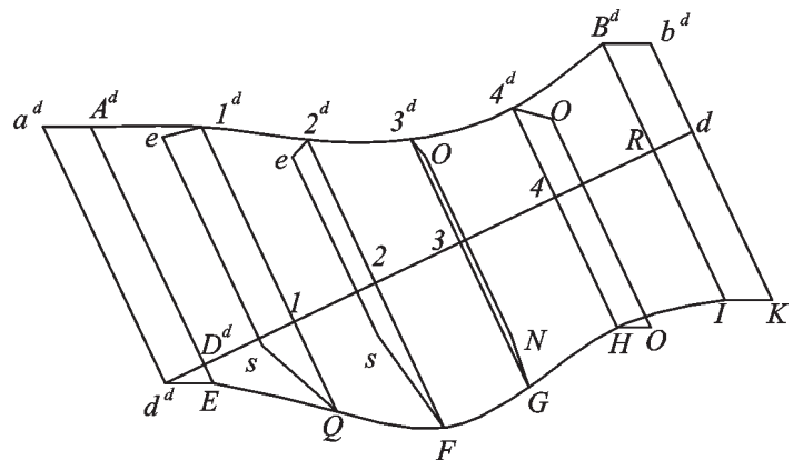
Fig. 280b Le linee curve sono lo sviluppo dello spigolo d'intradosso della faccia anteriore e posteriore.
