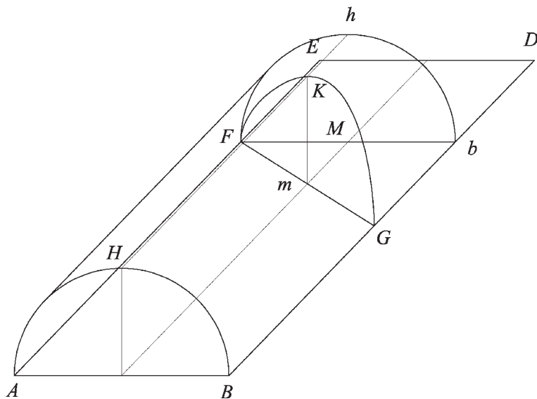
Fig. 58 In una Volta a Botte Sbieca a faccia circolare, ogni sezione formante con la faccia un angolo pari a quello con cui è ruotata la faccia è pure circolare.
