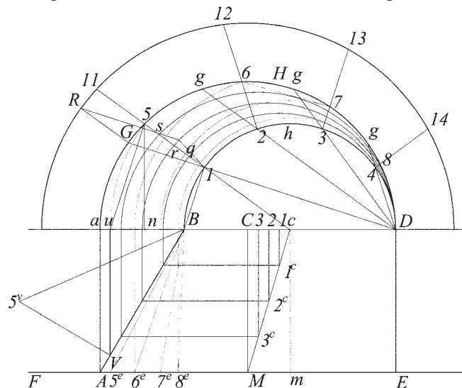
Fig. 132c Procedimento finale del nuovo metodo, invece delle curve, poiché diventano allora delle sezioni triangolari dei piani che si incrociano tutti sull'asse CD del cono scaleno, del quale la sezione orizzontale è rappresentata nella Fig. 135 dal triangolo ASD , che si può vedere solo in elevazione, o in proiezione verticale, i punti EDS si riuniscono in uno solo: D ; poiché la rappresentazione di una perpendicolare al piano di proiezione si riduce a un solo punto come è stato detto a pag. 208 del 2° libro.
