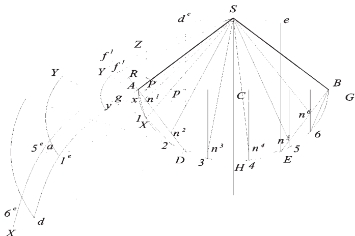
Fig. 127 Prime fasi della costruzione geometrica, proiezione sul piano orizzontale della “TROMPE” piatta.
