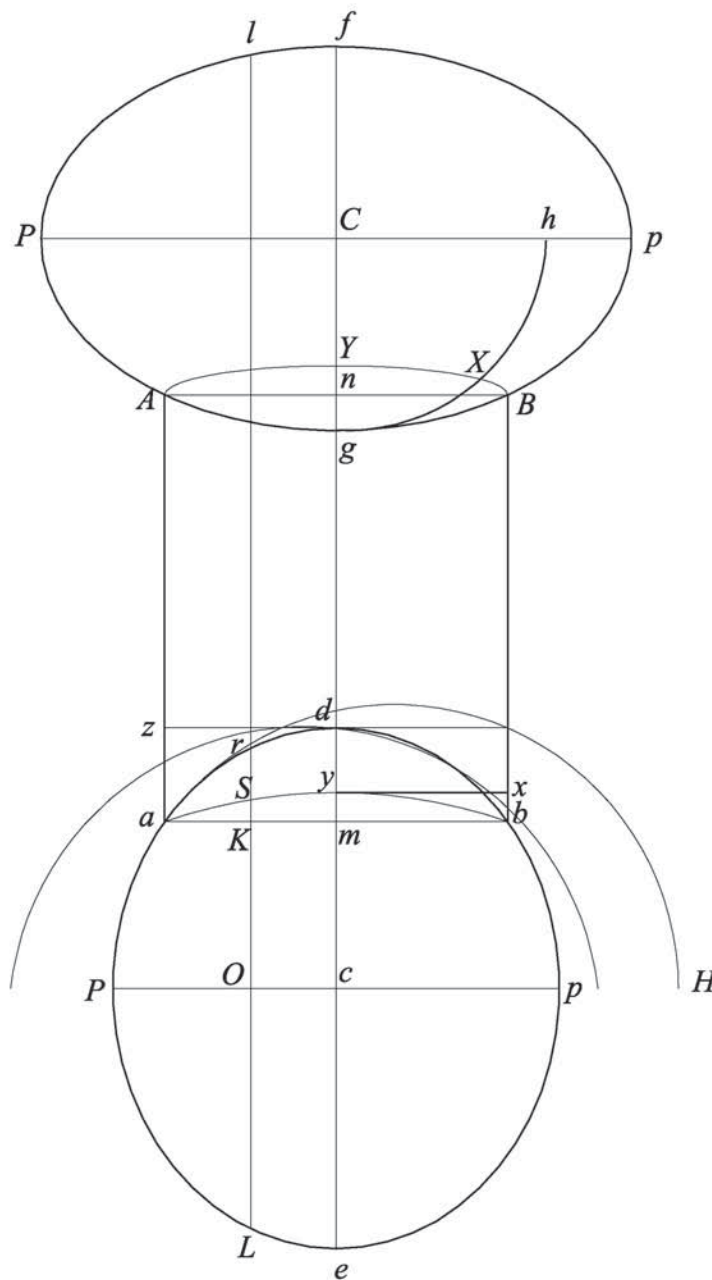
Fig. 99 La sezione fatta dall'incontro tra un cilindro retto e uno sferoide, i cui assi sono perpendicolari, è un "cicloimbre".
