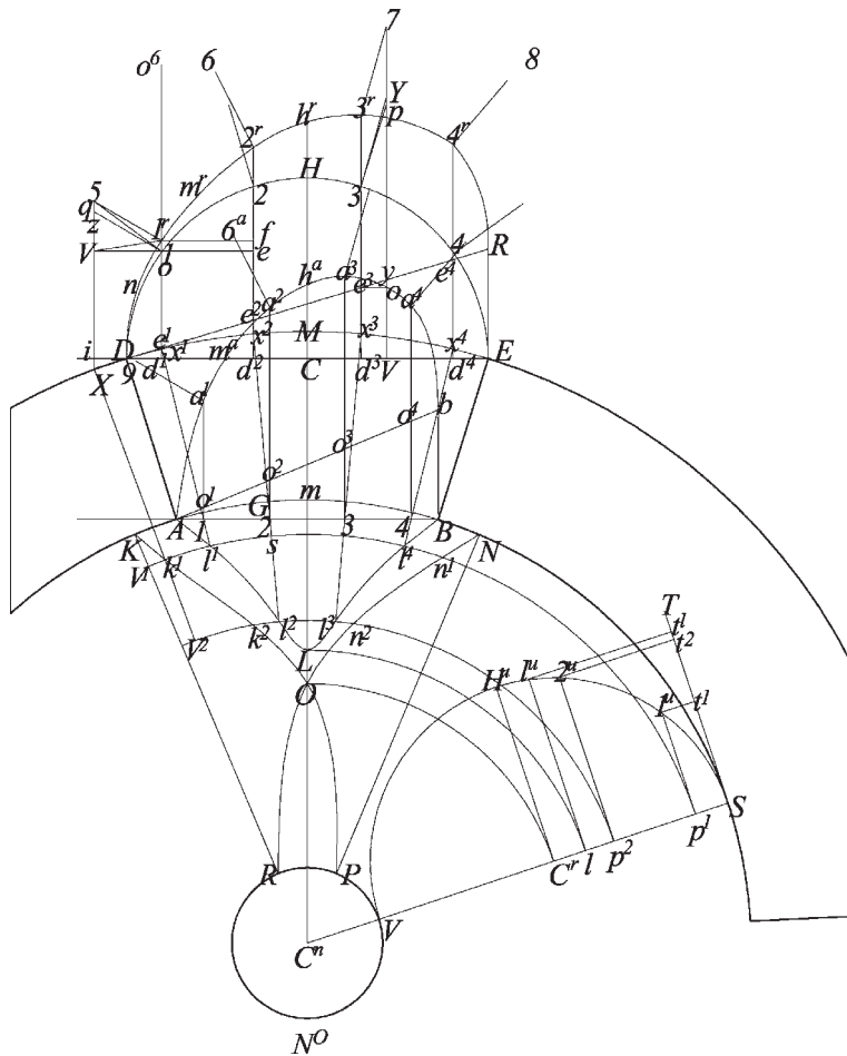
Fig.171 Disegno conclusivo della lunetta strombata dentro una volta a crociera tornante e rampante
