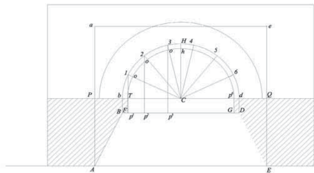
Fig. 261E - Costruzione della volta di Montpellier attraverso il terzo metodo sopradescritto in cui le le direzioni dei giunti delle facce di letto sono fatte su dei piani verticali diretti ad un punto S.
