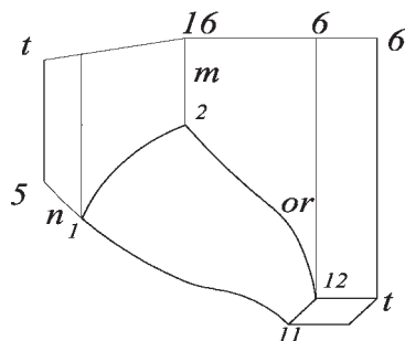
Fig. 129 L'arco AB sembrerebbe diviso in conci di uguale misura, questo porterebbe a un disegno diverso dei giunti di letto in facciata da quello presentato nella Fig.45
