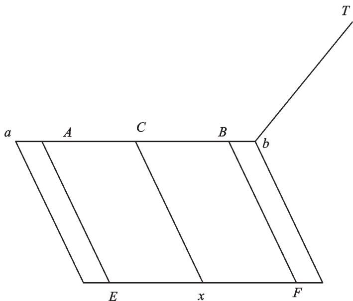
Fig. 274a Piano orizzontale di una volta a botte.
