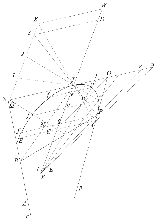
Fig. 134 Ellisse, dati i punti di tangenza.
