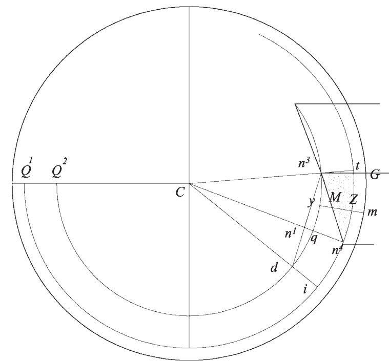
Fig.89b Ingrandimento della Fig.89
