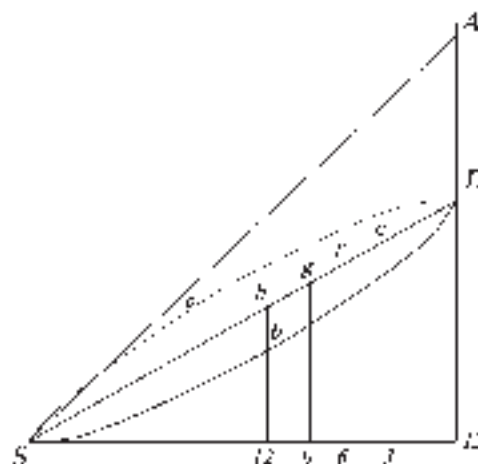
Fig. 139 Tracciare una spirale in un'altra.
