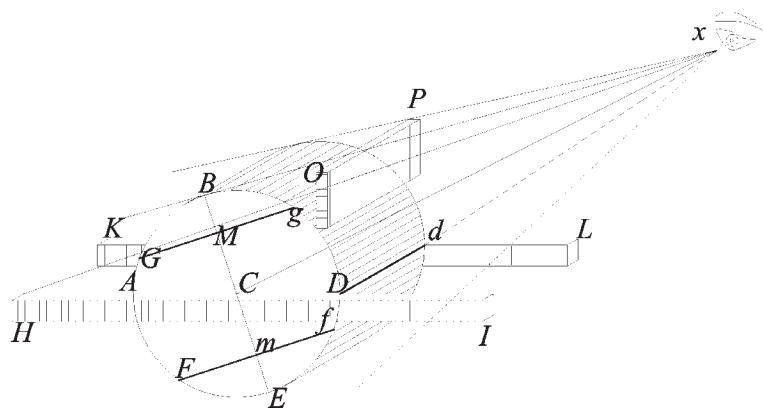
Fig. 177 Primo metodo per tracciare le parallele all'asse che è occupata dall'alto e dal basso, ed obbliga a dovere ricorrere a delle maniere meccaniche per tracciare delle parallele degli assi.
