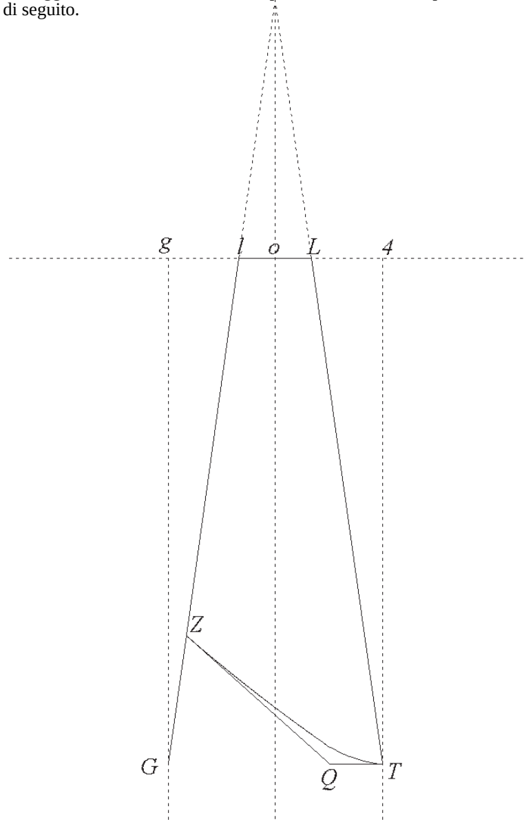
Fig. 135 Concio a piramide retta inscritto nella conoide dal quale si ricaverà, sottraendo pietra, il concio cercato
