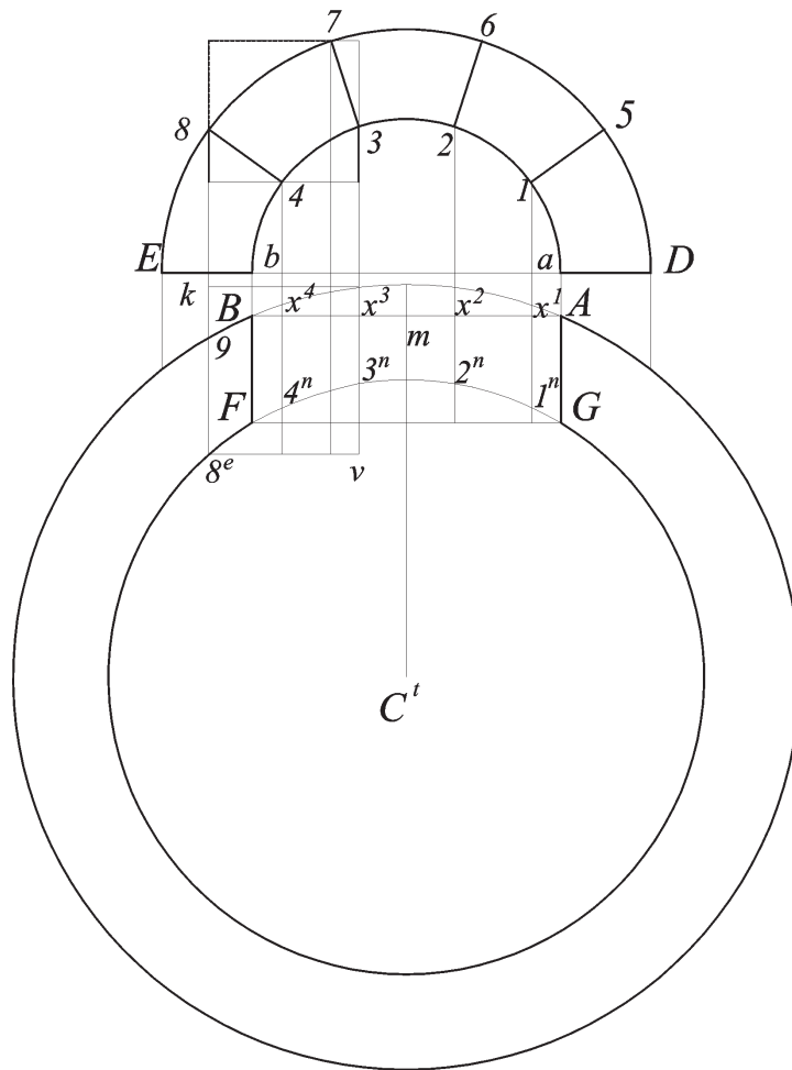
Fig. 33 Il metodo è difficile di questa costruzione, in quanto il resto di essa non differisce in niente da quella delle volte a botte ordinarie.
