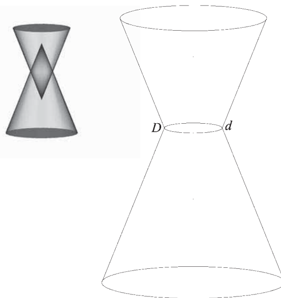
Fig 83. Intersezione di coni con asse coincidente e vertice
