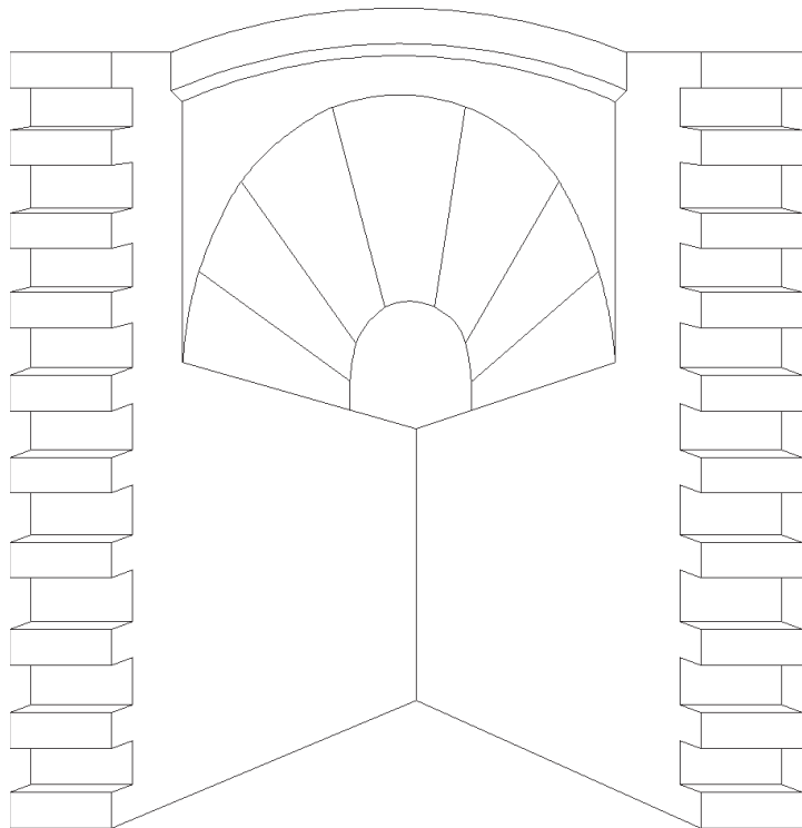
Fig. 137 Costruzione conico-sferoidale, curva alla chiave e retta sulle imposte, raccordante una torre tonda
