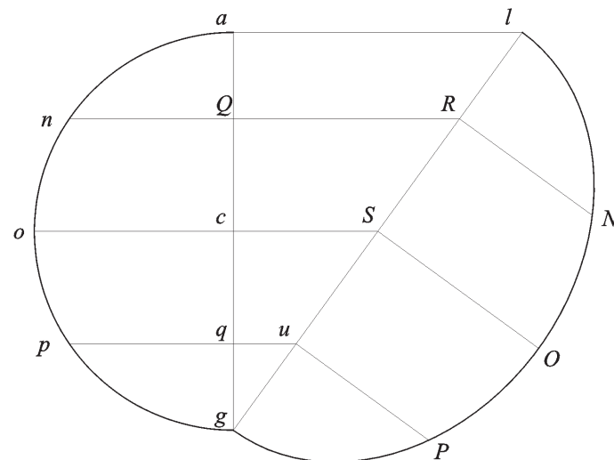
Fig. 178 Costruzione sul piano per la determinazione dell'ellisse sul cilindro.
