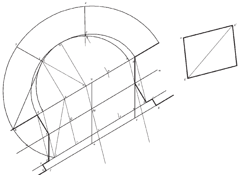
Fig.111: Costruzione del panneau di doele aqri , che stiamo
