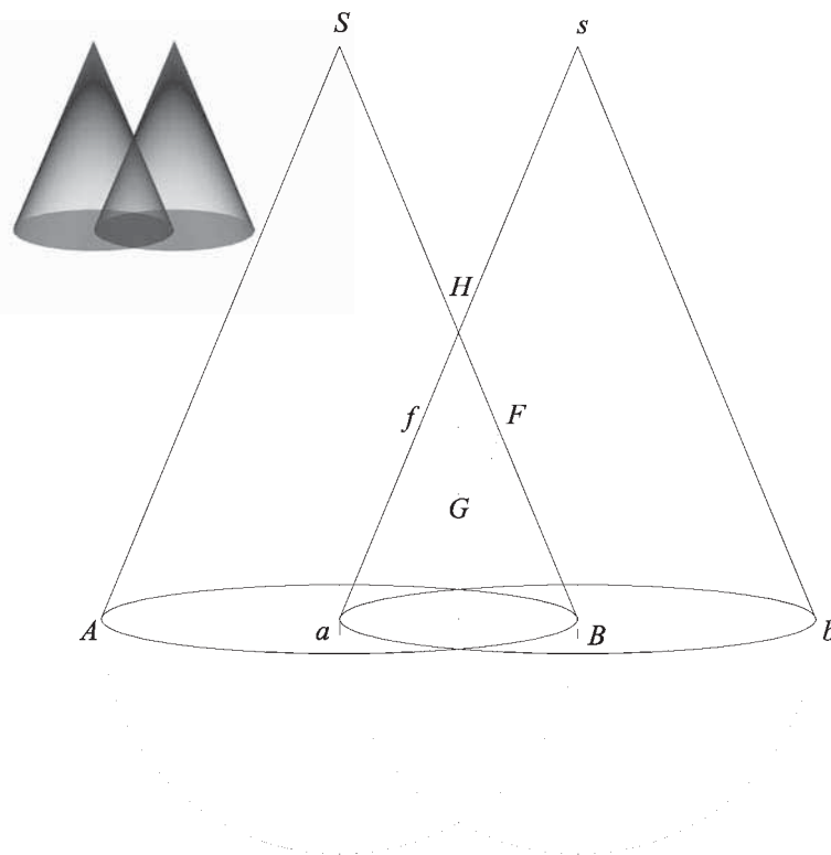
Fig 75. Intersezione di coni ad asse parallelo
