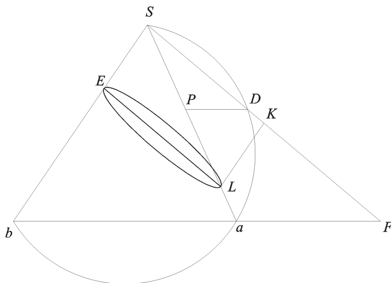
Fig. 181 a Rappresentazione dell'ellisse sulla superficie del cono
