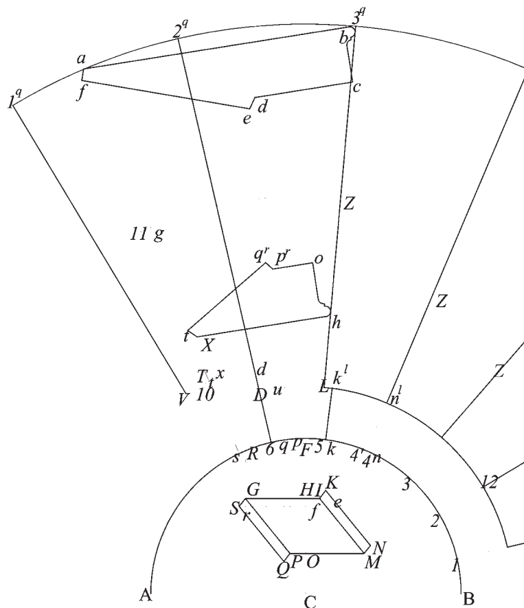
Fig. 188 Pianta di un settore di scala con sezioni del gradino e proiezione della testa del concio.
