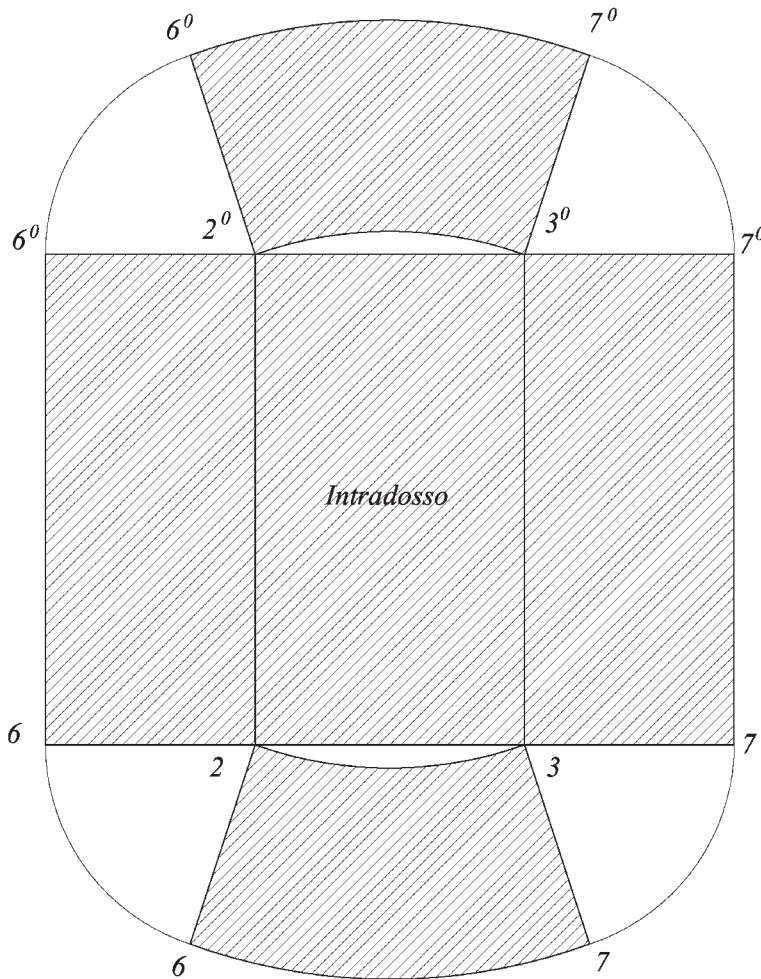
Fig. 59v In figura sono mostrate tutte le superfici formanti il concio 2376 di Fig. 59 ad esclusione della superficie dell'estradosso.
