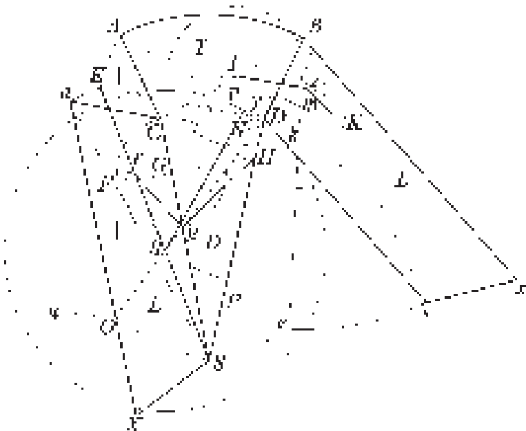
Fig. 309 Applicazione pratica del problema di Fig. 308 ad un mattone per volta conica, angoli che si formano tra loro al fine di poter prendere delle aperture con la fausse equerre , e servirsene per tagliare la pietra che bisogna tagliare
