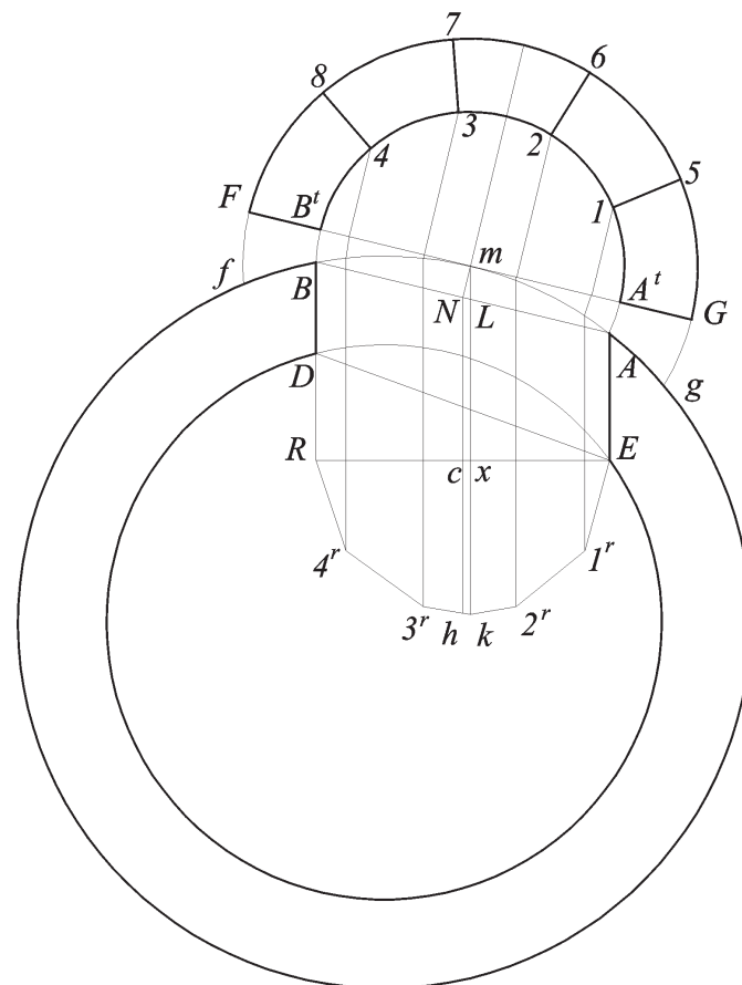
Fig.37b Centina primitiva sullo sviluppo dell'arco AmB
