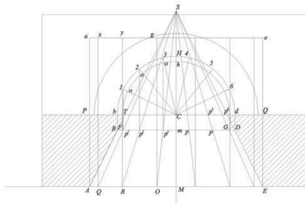
Fig. 261F - Costruzione della volta di Montpellier attraverso il terzo metodo sopradescritto in cui le le direzioni dei giunti delle facce di letto sono fatte su dei piani verticali diretti ad un punto S.
