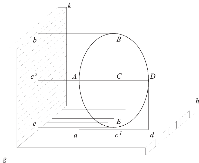
Fig. 170 La proiezione dell'ellisse, sia sul piano orizzontale che su quello verticale, è una linea retta
