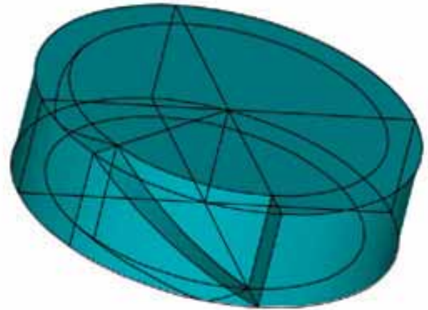
Fig. 226 a Primo taglio della pietra ad angolo retto secondo l'elica De.
