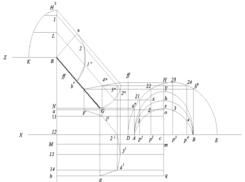
Fig. 56 Costruzione della sezione mediante il piano di riferimento rappresentato dall'asse della volta e il ribaltamento della volta stessa.
