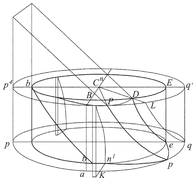
Fig. 226. Proiezione verticale degli spigoli del Cuneo sulla sezione della superficie cilindrica. Per comprendere questa figura, si suppone che il cilindro sia diviso in due parti uguali da un piano orizzontale che passa per i punti C e V. La parte superiore del cilindro, ha occorso supporre dei piani tb e RT, passanti per i punti più elevati c e b, e i più bassi R e 1 1 ; di forza che la superficie del cilindro eccede le eliche che devono essere tracciate sul cilindro, i due triangoli misti, punteggiati alla fig. 228. in cyb 31 , e xi1 1 , i quali devono essere sottratti per un taglio a squadra sulla superficie cilindrica, perché le linee che si devono supporre tirate all'asse, per i punti dell'elica del cilindro, incontrano alla stessa altezza, quella dello spigolo del Cuneo all'intradosso o all'estradosso.
