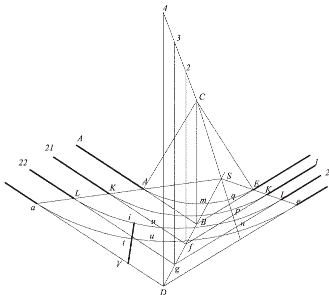
fig.31 diminuzione dell'arrotondamento dato San Michel, secondo l'intenzione dell'ingegnere Direttore (il sig. "glacis" pendenza dolce che parte dalla cima di un camino coperto con il soulo
