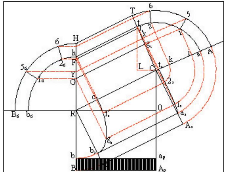
Fig 86. Proiezione del quarto d'ellisse rialzato. Rappresenta la metà della curvatura nel prospetto di salita
