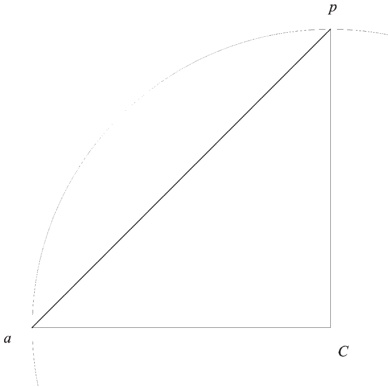
Fig. 174 a Considerando la superficie concava della sfera, la corda ap dell'arco di 90° verrà utilizzata per determinare il polo.
