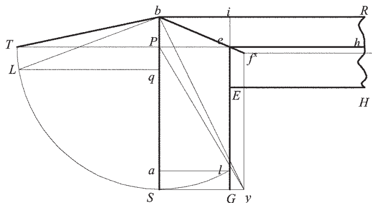
Fig.22 Fare lo spigolo di un'angolo le cui facce hanno pendenza
