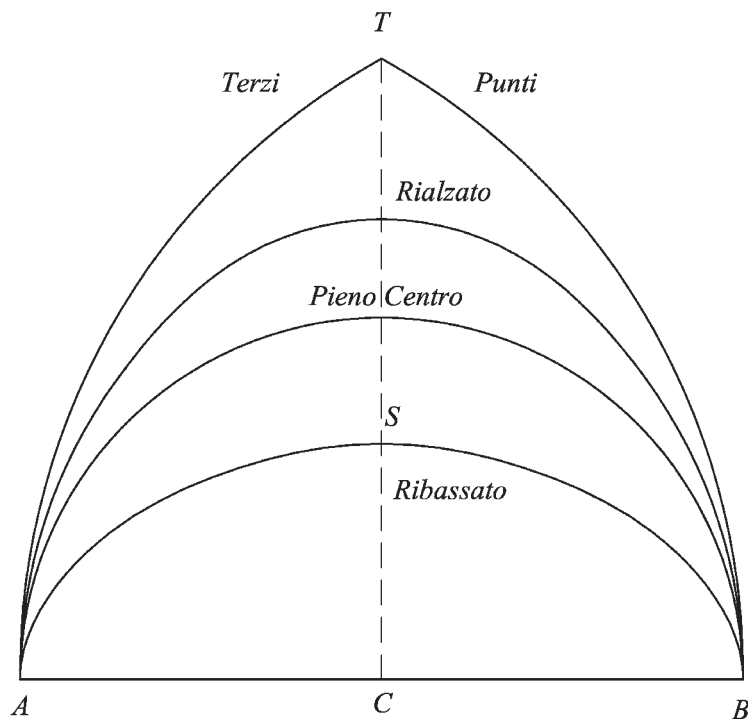
Fig. 57 La figura mostra i quattro tipi di Volta a Botte maggiormente utilizzati: a Sesto Ribassato, in Pieno Centro, a Sesto Rialzato e per Terzi Punti.
