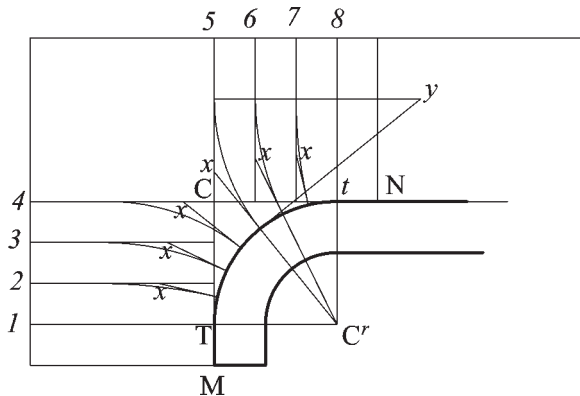
Fig. 175 Costruzione dell'arrotondamento dei gradini per evitare difformità negli aggetti. Confrontando con il disegno della planche possiamo notare una discordanza nella posizione dei centri dell'arrotondamento causati da un'imprecisione della costruzione del disegno originale perché fatti a mano.
