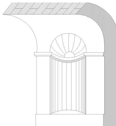
Fig. 102 Incontro di una volta sferica con una volta cilindrica
