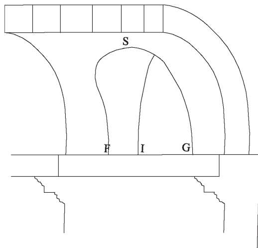
Fig. 28. 2 Incontro di due volte a botte di altezze diverse: lunetta (diritta o di sbieco).
