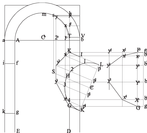
Fig. 30. 2 e 30. 3 Sviluppo dell'intradosso piatto dei conci della volta più alta nella quale viene aperta la lunetta.
