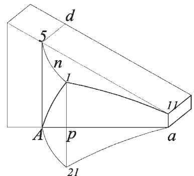
Fig. 129 L'arco AB sembrerebbe diviso in conci di uguale misura, questo porterebbe a un disegno diverso dei giunti di letto in facciata da quello presentato nella Fig.45
