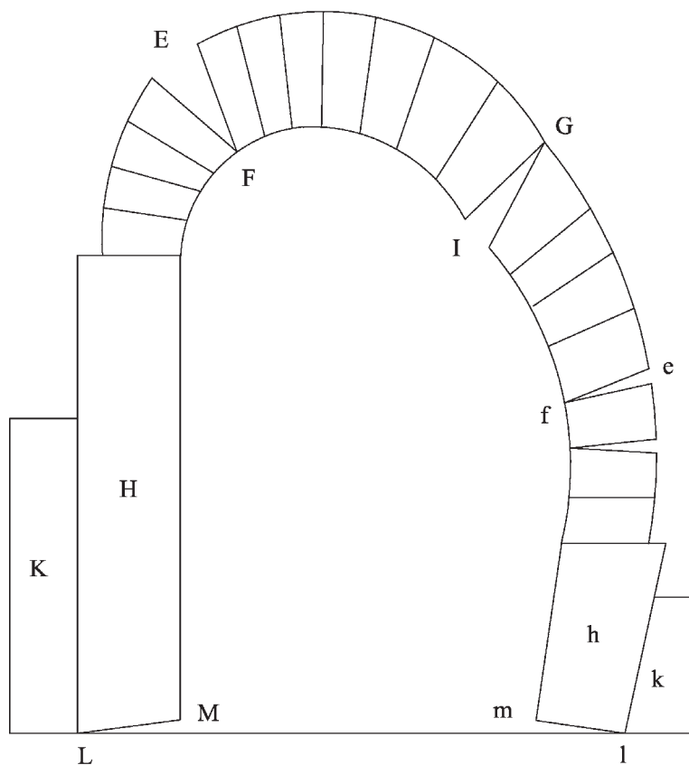
Fig. 239 Rappresentazione di un arco rampante di 18 pietre
