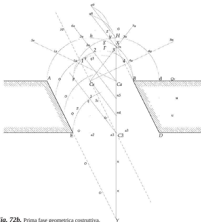
Fig. 72b. Prima fase geometrica costruttiva.
