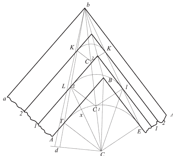
fig.29 arrotondamento conico con pendenze disuguali
