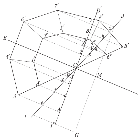
Fig.99 costruzione per tracciare i conci sulla pietra.
