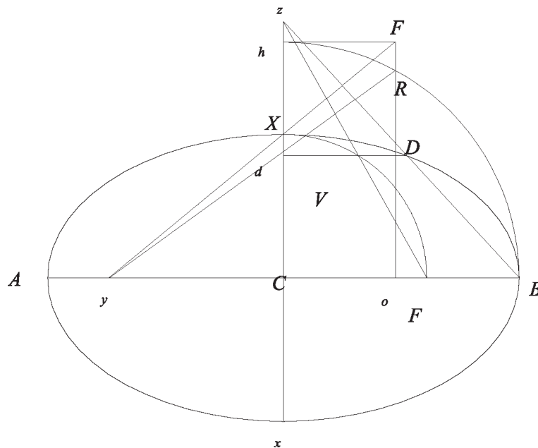
Fig.114 Costruzione di un'ellisse conoscendo solo l'Asse maggiore.
