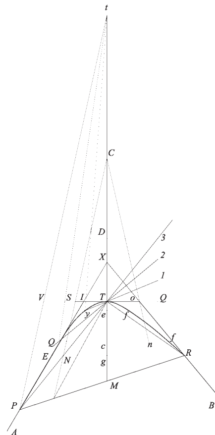
Fig. 135 Iperbole, dati i punti di tangenza.
