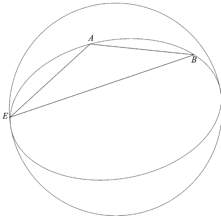
Fig. 173 a Attraverso i punti dati sulla superficie della sfera viene descritto un cerchio
