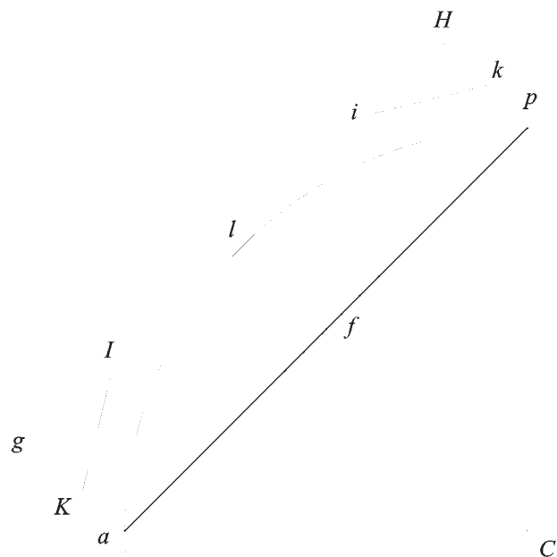
Fig. 174 b Considerando la superficie convessa della sfera, per trovare il polo, verrà utilizzato l'arco aLp
