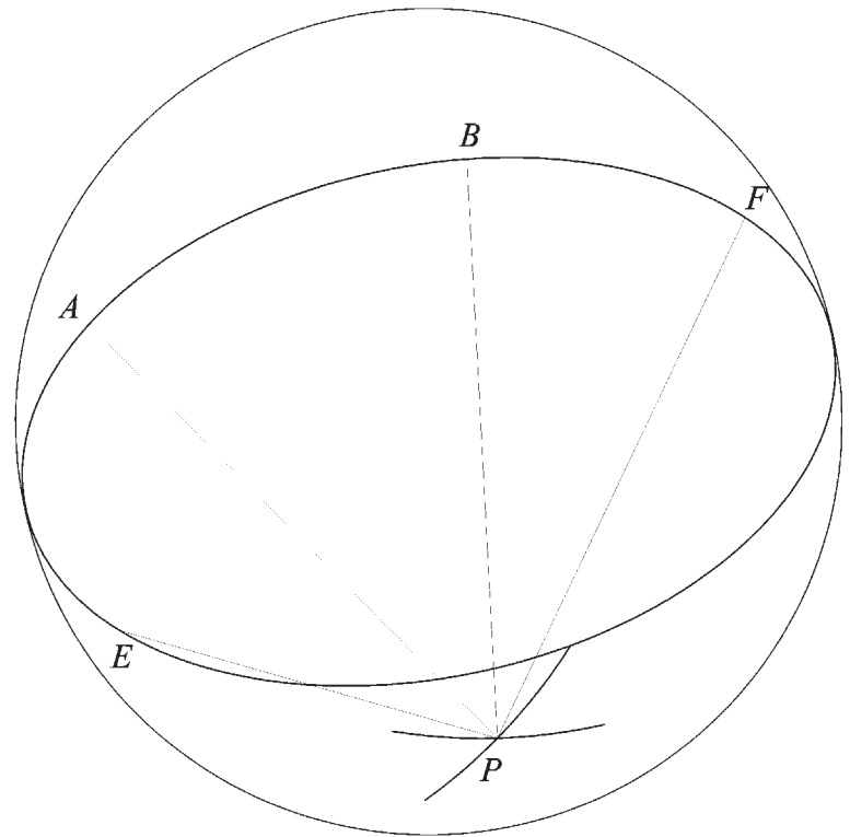
Fig. 173 f attraverso il polo P è stato disegnato il cerchio maggiore EABF
