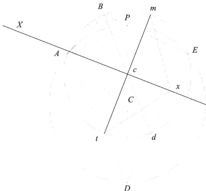
Fig. 175 Metodo per individuare i poli x e X di un cerchio minore
