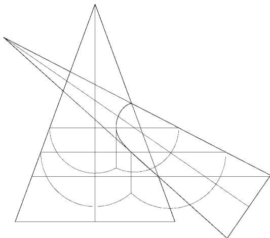
Fig. 207 Ellipsoidimbre composto formato dall'intersezione di due coni
