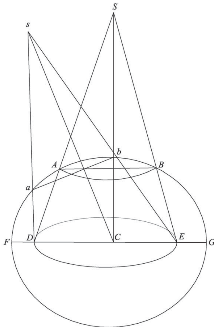
Fig. 102 L'intersezione tra uno sferoide e un cono, sia retto che obliquo, da una ellisse.
