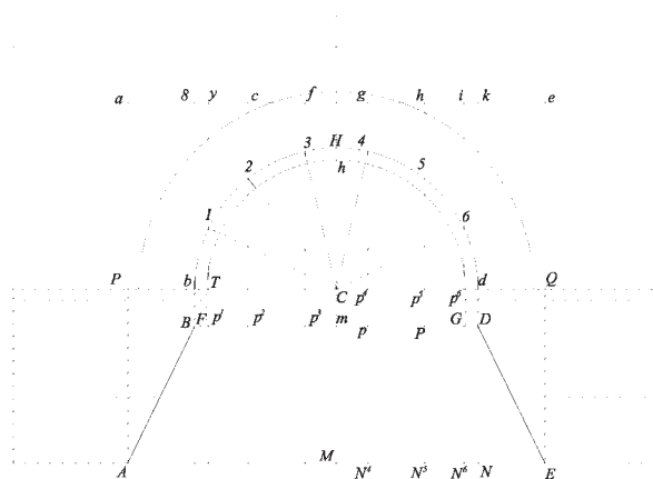
Fig. 261B - Costruzione della volta di Montpellier attraverso il secondo metodo sopradescritto in cui le le direzioni dei giunti delle facce di letto sono parallele alla direzione della volta.
