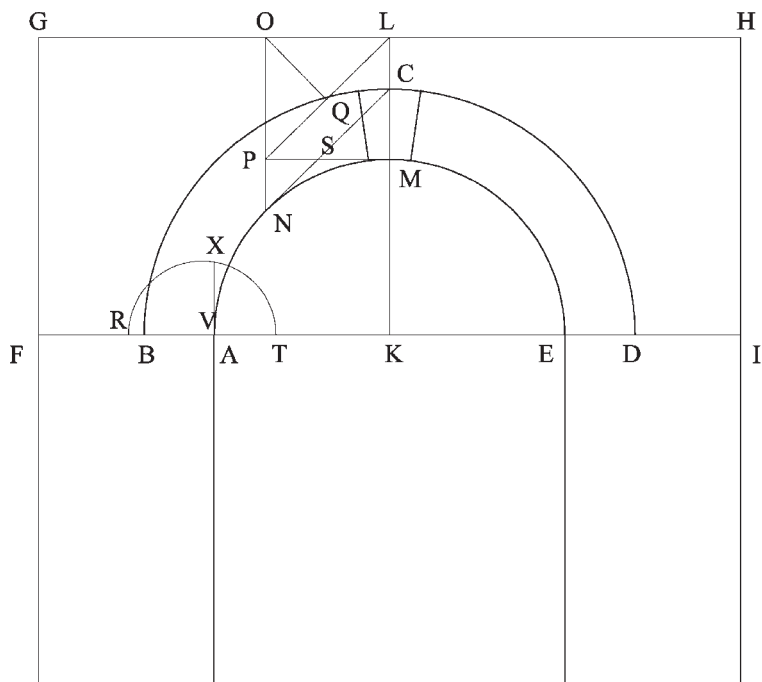
Fig.242 Rappresentazione di un arco di volta.
