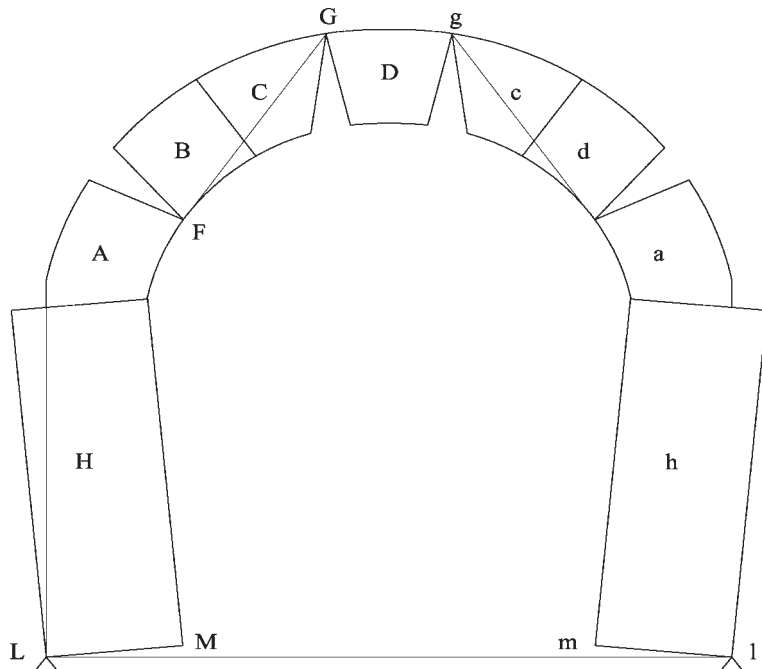
Fig. 235 Rappresentazione di una piccola volta in gesso a tutto sesto composta da sette pietre caricata sulla chiave con un piccolo peso
