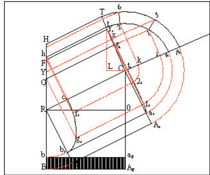
Fig 86. Proiezione del quarto di cerchio. Rappresenta la faccia in discesa della volta a botte
