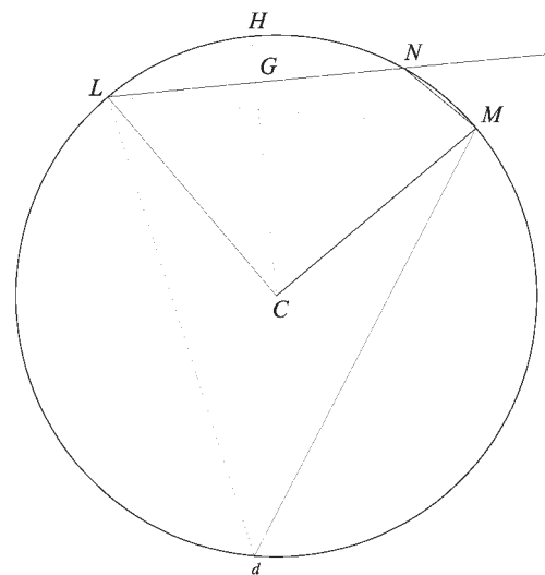
Fig. 108 Individuazione dell'angolo LNM per tracciare un arco di cerchio.
