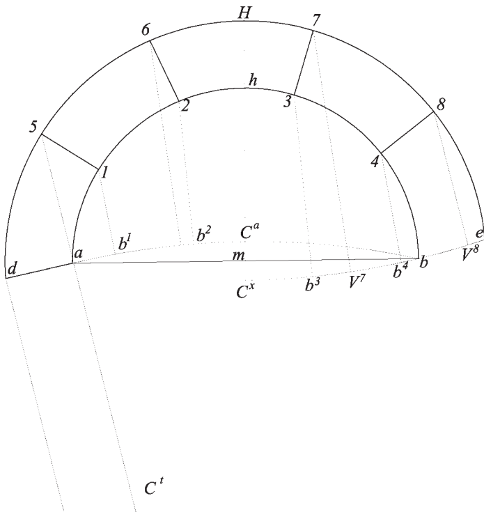
Fig.60 Arco concavo nella torre cava daC^u .
