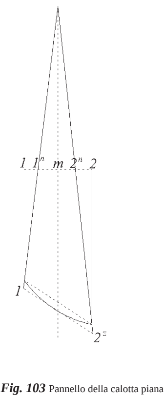
Fig. 103 Pannello della calotta piana
