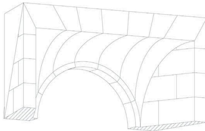
Fig. 263A - Rappresentazione assonometrica della volta di Montpellier attraverso il secondo metodo sopradescritto in cui le direzioni dei giunti delle facce di letto sono parallele alla direzione della volta.
