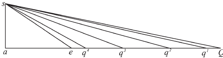
Fig. 230 a Rettificazione degli archi di cerchio della rivoluzione con sviluppi delle eliche dei giunti di letto.
