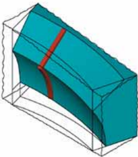
Fig. 228 c Preparazione del letto superiore del cuneo. Si noti che il cuneo ottenuto è lo stesso descritto alla fig. 229.
