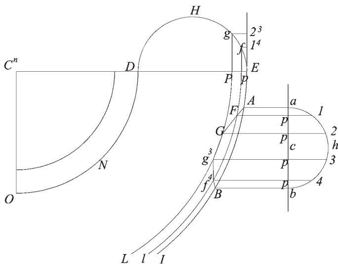
Fig. 122 c Costione completa dell'intersezione della volta a botte con la volta
