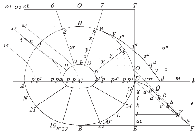
Fig. 126 L'arco AB sembrerebbe diviso in conci di uguale misura, questo porterebbe a un disegno diverso dei giunti di letto in facciata da quello presentato nella Fig.45
