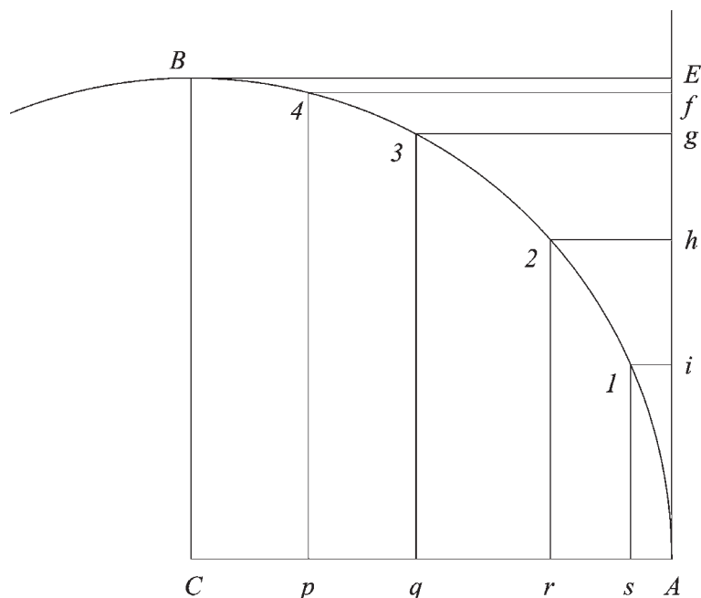
Fig. 243 La figura rappresenta i due possibili metodi per dividere la curva in parti per la divisione del profilo, per la quale si uniscono così tutte le altezze delle divisioni di un centro su una sola linea, è:
