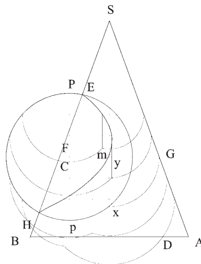
Fig. 206 Ellipsoidimbre composto formato dalla compenetrazione di un cono ed una sfera.
