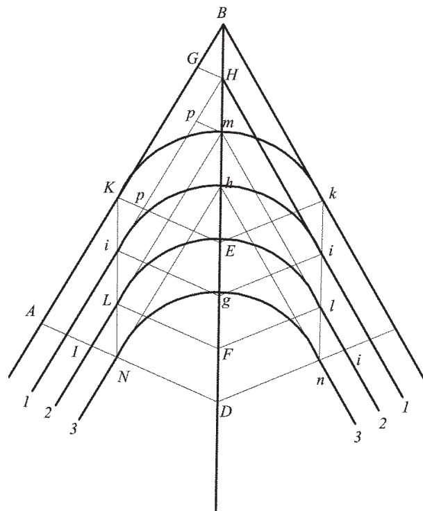
fig.24 ,arrotondamento cilindrico con pendenze uguali in relazione a GH .
