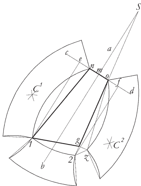
Fig. 98. Rettifica della superficie interna del concio.
