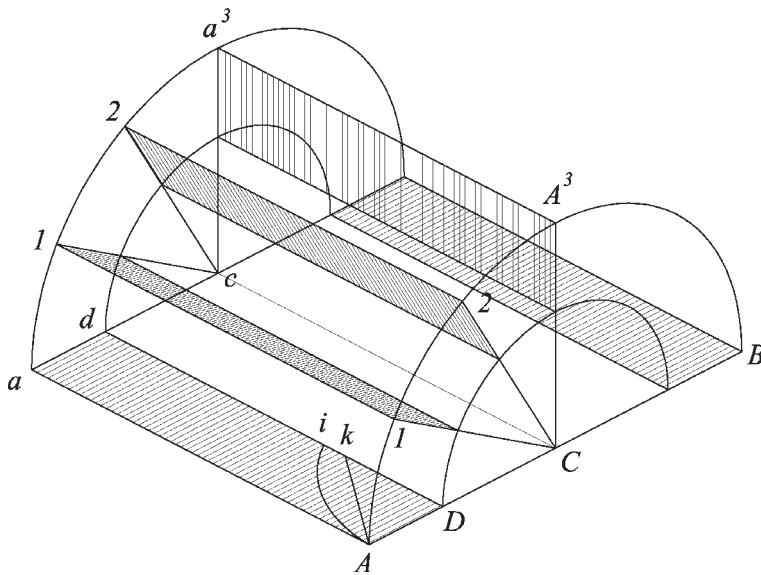
Fig. 55 La Volta a Botte Retta è generata dalla rotazione di una superficie rettangolare ADda attorno ad un'asse Cc.
