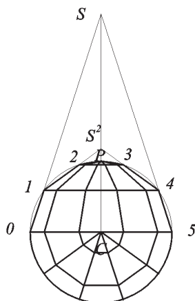
Fig. 276b Il prolungamento dei lati del trapezio ci permette di ricavare il raggio del arco di cerchio su cui stendere le corone circolari per lo sviluppo della sfera.
