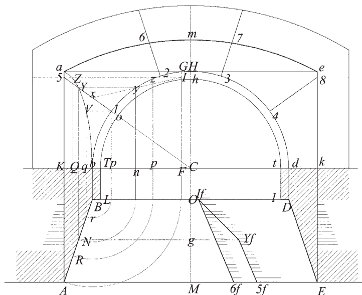
Fig. 235 L'arrière-voussure de Marsiglia ordinaria.
