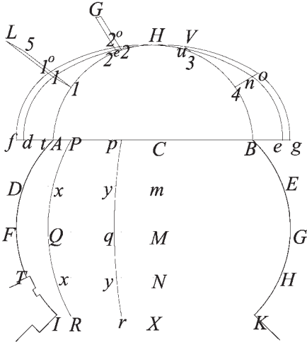
Fig.251a proiezione orizzontale della volta a botte
