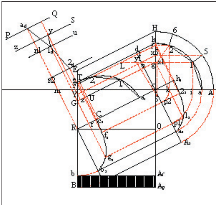
Fig 86. Discesa retta a scarpa sul davanti e a piombo sul di dietro
