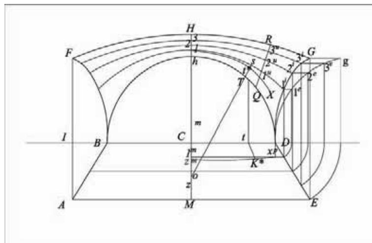
Fig.151b.Nella figura viene riportato il concio della fig.151a precedente indicando le sezioni hH,Ts,QR, attraverso le quali nella fig.152 è stato possibile ricavare alcuni punti della decorazione. Si è inoltre trovato un terzo punto K^* con la proiezione di T, il quale permetterà di tracciare la curva, relativa alla decorazione del concio, z^n K^* x^m
