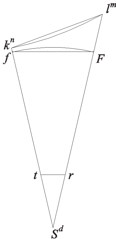
Fig. 68a - Volta conica in torre cava. Sviluppo delle superfici flessibili per il taglio dei conci. Applicazione del tratto sulla pietra.
