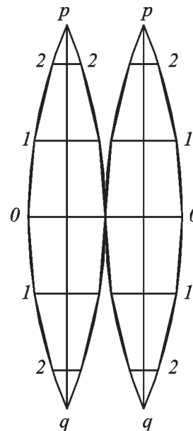
Fig. 277 La sfera può essere sviluppata secondo le meridiane, cioè lo sviluppo in fusi.
