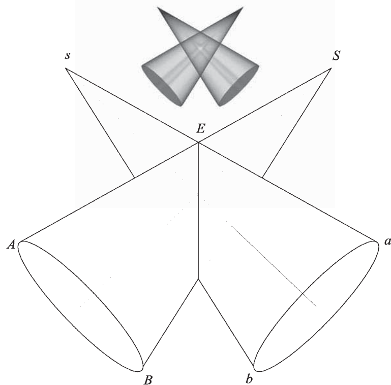
Fig 78. Intersezione di coni con assi che si incontrano in un punto interno.
