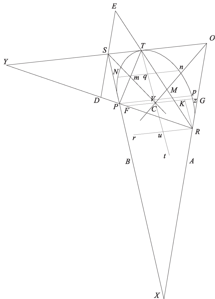
Fig.150 Sezione conica che rappresenta la centina dell'arco, dati i piedritti non paralleli e le linee di Rampa e di Sommità non parallele.
