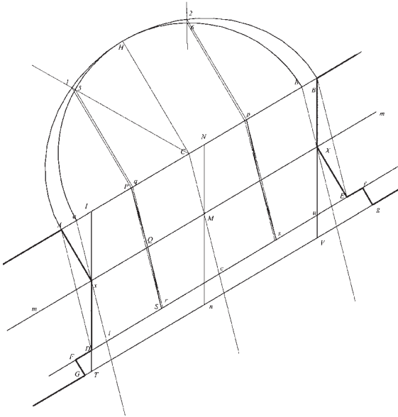
Fig.110b: Costruzione del join de lit PQs di un porta sbieca si formerà il panneau di doele ( Fig.111 ) come è stato detto nel secondo Libro, pag.357 9) , facendo due triangoli uguali, su questa base comune, con la corda di testa a5 , e la proiezione di un join de lit qr , o ai , tali sono
