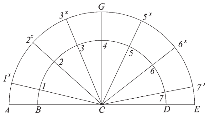
Fig. 193-a Visualizzazione in pianta della staffa AB4DEG
