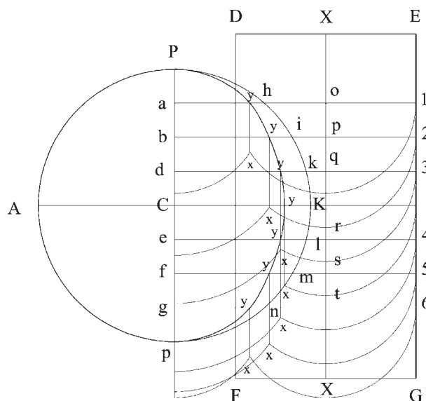
Fig. 202 Ellipsimbre formato dalla compenetrazione parziale di un cilindro con una sfera.
