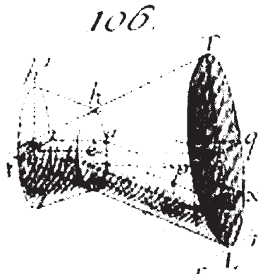
Fig.106: Intersezione di due cono retti con asse comune orizzontale
