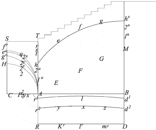
Fig.253a proiezione orizzontale della semivolta a botte retta all'imposta e curva sotto la chiave di volta.
