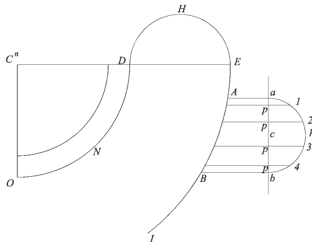
Fig. 122 a Prima costruzione della volta a botte che interseca una volta anulare
