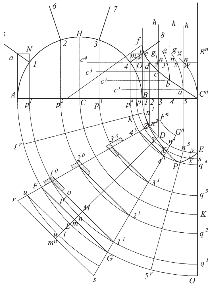
Fig. 224 c Proiezione verticale dell'elica della nascita della Volta a Spirale sul
