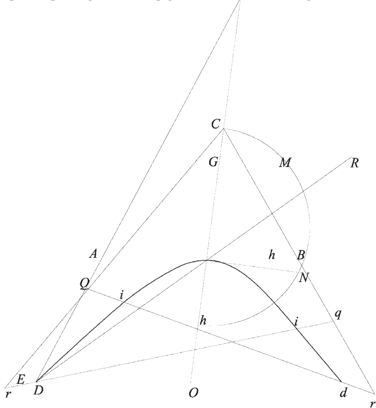
Fig. 125 Iperbole dati il centro C , il vertice S e l'ordinata CO .
