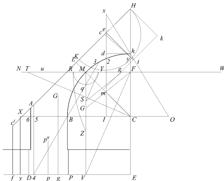
Fig. 214 Metà del profilo di un palazzo voltato a "culla", quale a causa della debolezza dei piedritti crollò ancor prima di essere totalmente disarmato.
