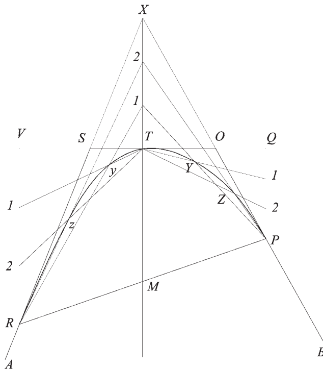
Fig. 132* Sezione conica, data una retta per due punti delle tangenti estreme.
