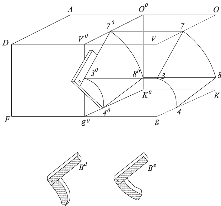
Fig. 62 Sopra è illustrata la parte di materiale che deve essere asportata da una pietra, così come la si ottiene dalla cava, per ottenere un concio tipo che costituisce parte della corona, o di ellisse ABEHD [Fig. 60] o di cerchio [Fig. 59] o di arco rampante [Fig. 61] tagliata dai giunti di testa 51, 62, 73, e 84; così basta tagliare del cartone o un'asse seguendo il contorno misto DA15 , e questo pannello basterà per tutti i conci della faccia se la centinatura è circolare; infatti anche se si facessero dei conci di larghezza ineguale, la direzione dei giunti determinerà sempre lo stesso angolo con la curva dell'intradosso.
