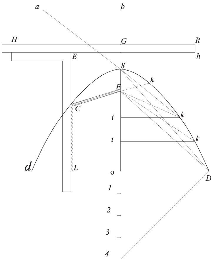
Fig. 122 Parabola per più punti.
