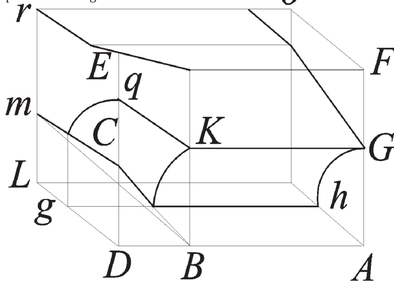
Fig.57 Costruzione dei pannelli per poter tagliare la pietra destinata al concio
