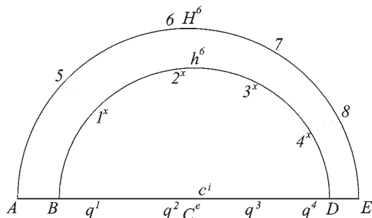
Fig. 107: si vedono con un disegno a parte le divisioni del diametro e le altezze delle ricadute.
