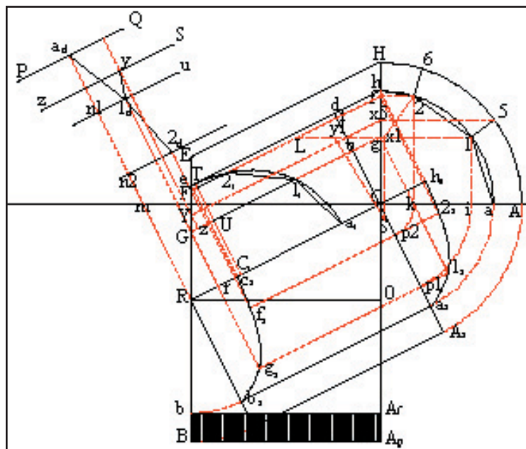
Fig 84. Sviluppo dei pannelli d'intradosso piatto e delle teste
