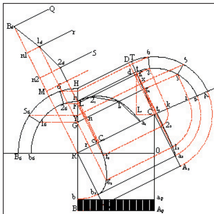
Fig 86. Sviluppo dei pannelli d'intradosso
