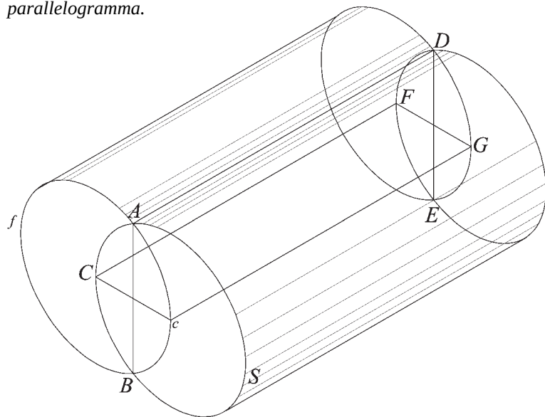
Fig. 55 Il parallelogramma CFGc è comune ai due cilindri.
