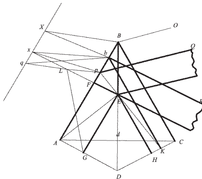
fig.21 Fare lo spigolo di un'angolo le cui facce hanno ugual pendenza
