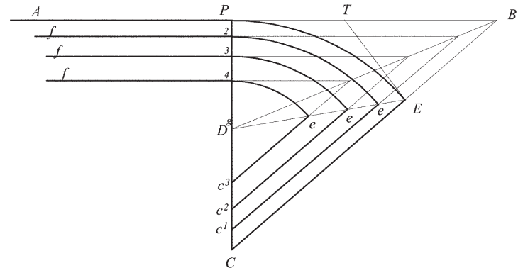
fig. 26 arrotondamento di una sola faccia così le proiezioni orizzontali dei bordi di ogni letto, che si concluderanno in una retta Ee , diversa dalla diagonale BD dell'angolo dato, che sarà la proiezione dell'intersezione dello spigolo delle facce incurvata e retta in pendenza.
