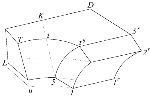
Fig.63 Pietra a taglio ultimato.
