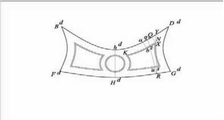
fig 154 nella figura viene rappresentato lo sviluppo dell'intradosso della sezione bombata, dove le due curve BhD, FHG,FB,GD, provengono rispettivamente dalle curve BhG,FHG,FB,GD, della fig.151 con lo stesso sistema si ricava anche il disegno all'interno.
