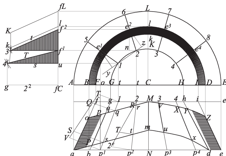
Fig.283 Proiezione verticale e proiezione orizzontale della volta e dei suoi joins de lit
