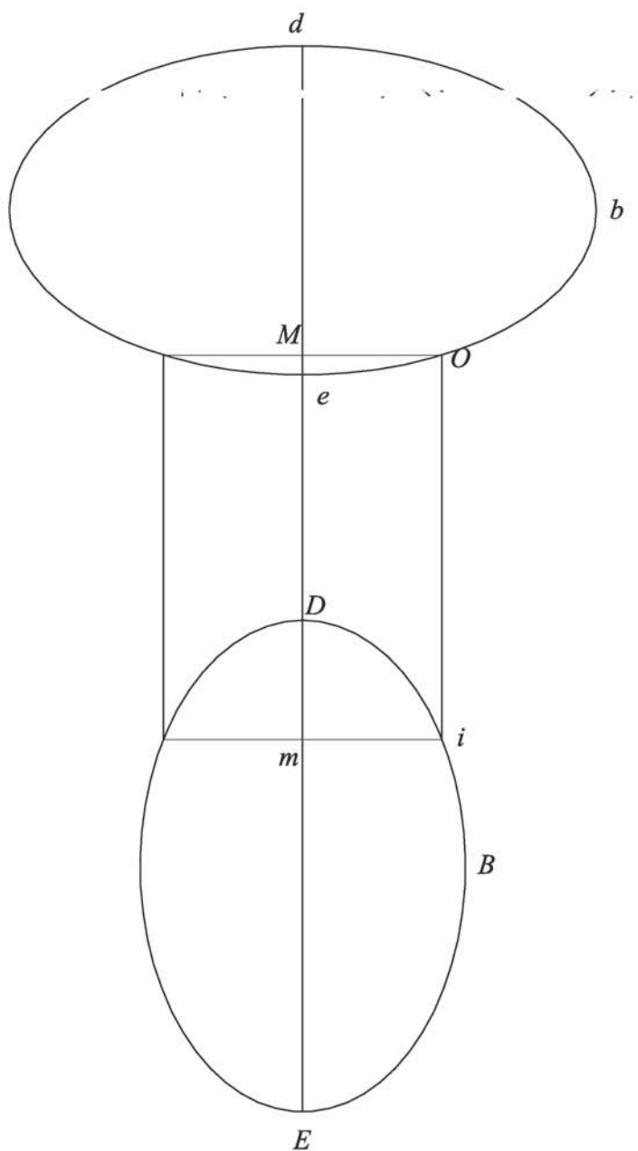
Fig. 96 L'intersezione tra due ellissoidi e uno cilindro retto Fig. 97 e 98 Sarà uguale per l'intersezione tra uno sferoide e un cono
