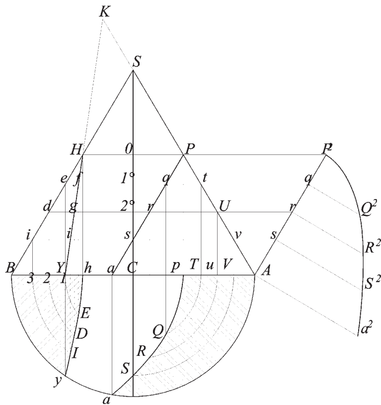
Fig. 184 c Sezione del cono: parabola
