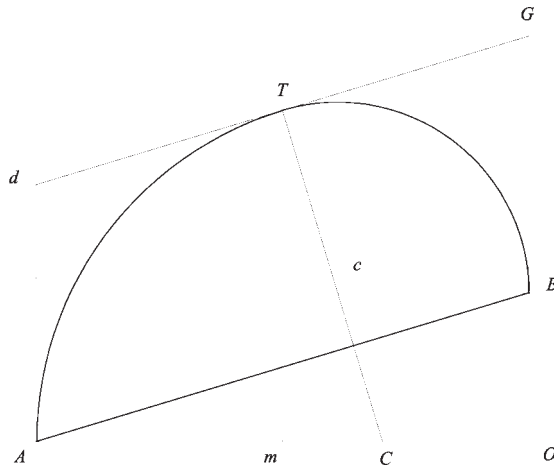
Fig.156: Costruzione di un arco rampante in cui i piedritti sono paralleli e la linea di pendenza è parallela a quella di sommità
