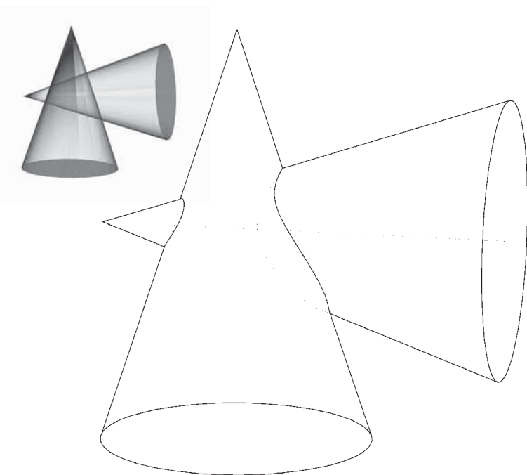
Fig 87. Intersezione di due coni i cui assi si incontrano formando un angolo retto
