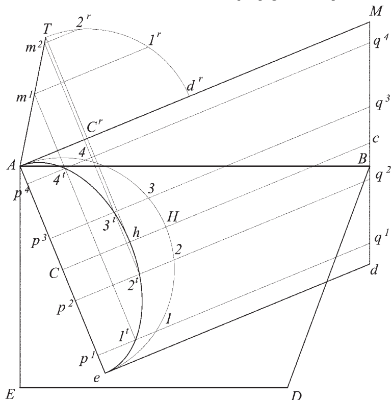
Fig. 92a : Costruzione del piano della volta in discesa obliqua, e di una delle sue
