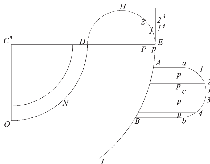
Fig. 122 b Costruzione di 2 perpendicolari sul diametro della volta anulare Dal centro C^n , attraverso i punti P e p della linea DE , si tratteranno degli archi di cerchi concentrici PL , pl che taglieranno le proiezioni delle
