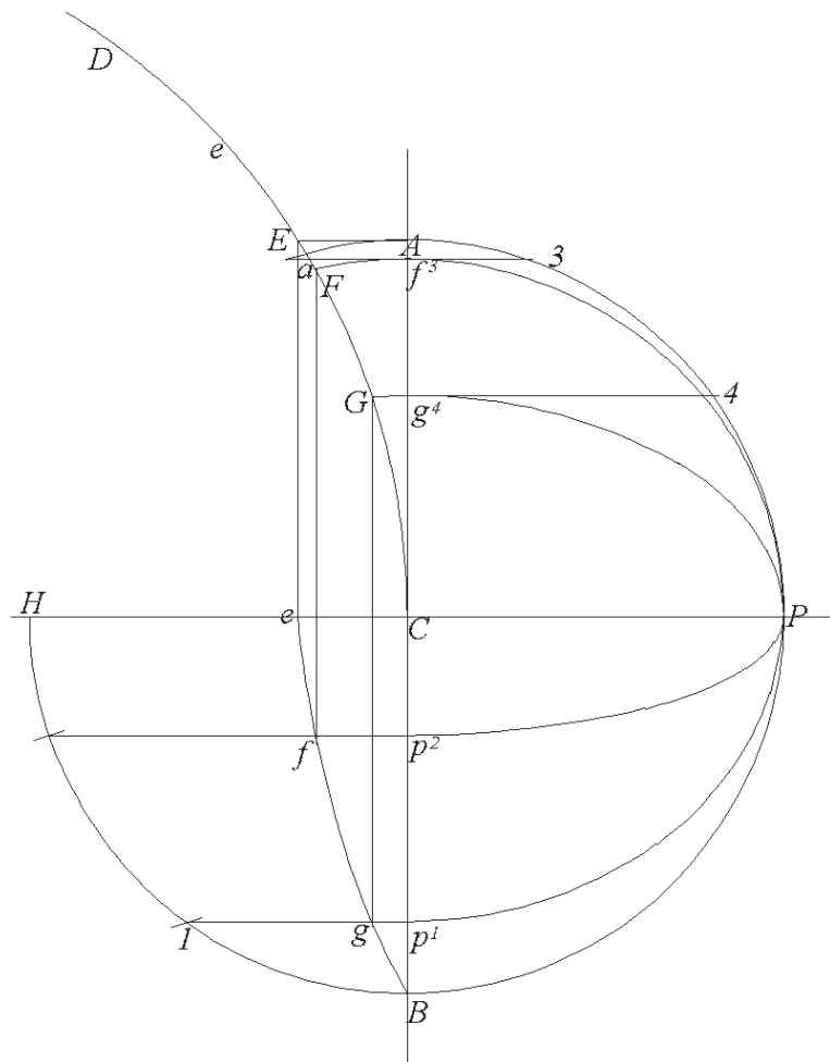
Fig. 101 b Costruzione della proiezione orizzontale della giunzione ( Efg ) della nicchia con la volta a botte
