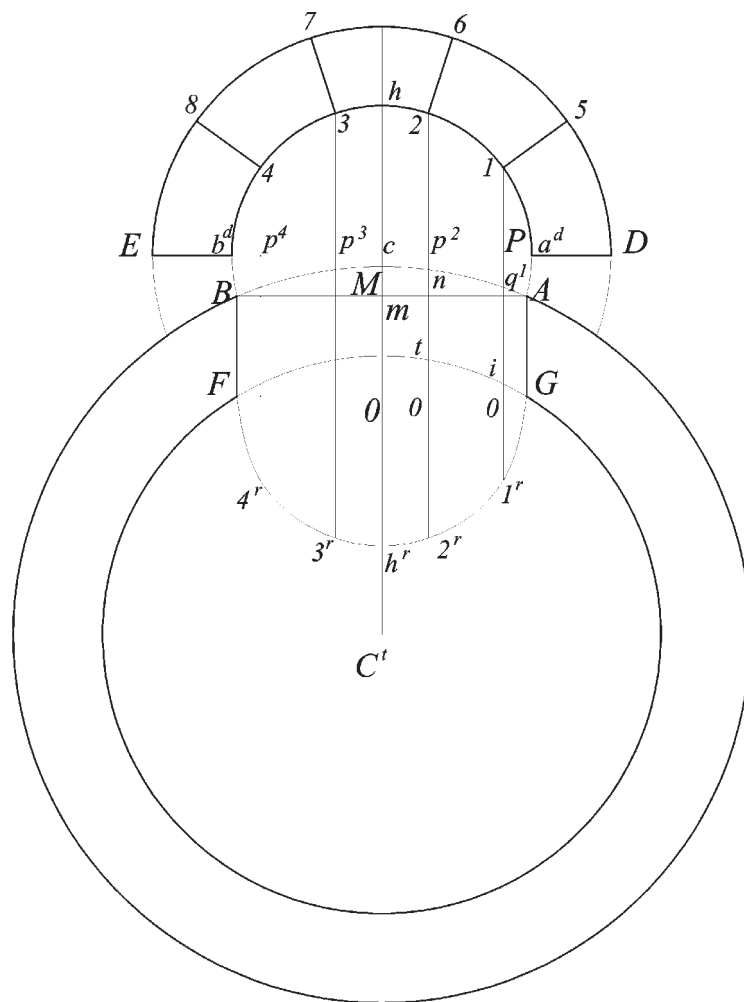
Fig. 33b Secondo metodo: Sesto primitivo a superficie curva
