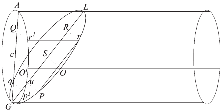
Fig. 176 d Secondo metodo per rappresentare l'ellisse di sezione
