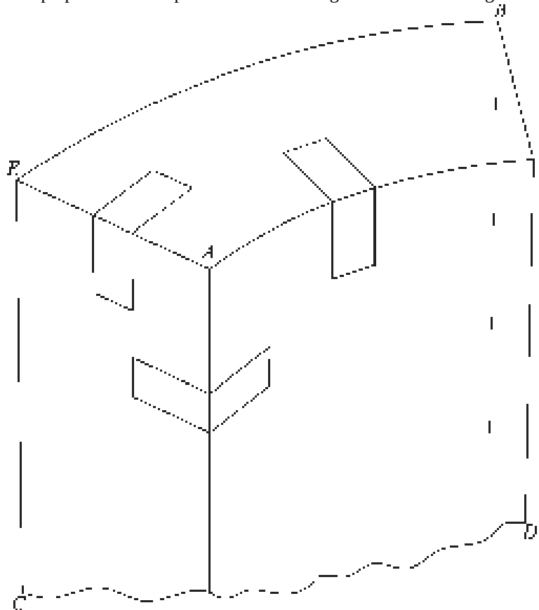
Fig. 307 Applicazione pratica di Fig. 305 ad un'attone per volte a botte rappresentato la linea LM è in aria fuori dal piano della carta.
