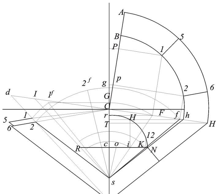
Fig. 110: disegno del pennacchio retto in pendenza come se fosse un pennacchio sbieco senza pendenza; ricerca delle vere lunghezze dei giunti di letto
