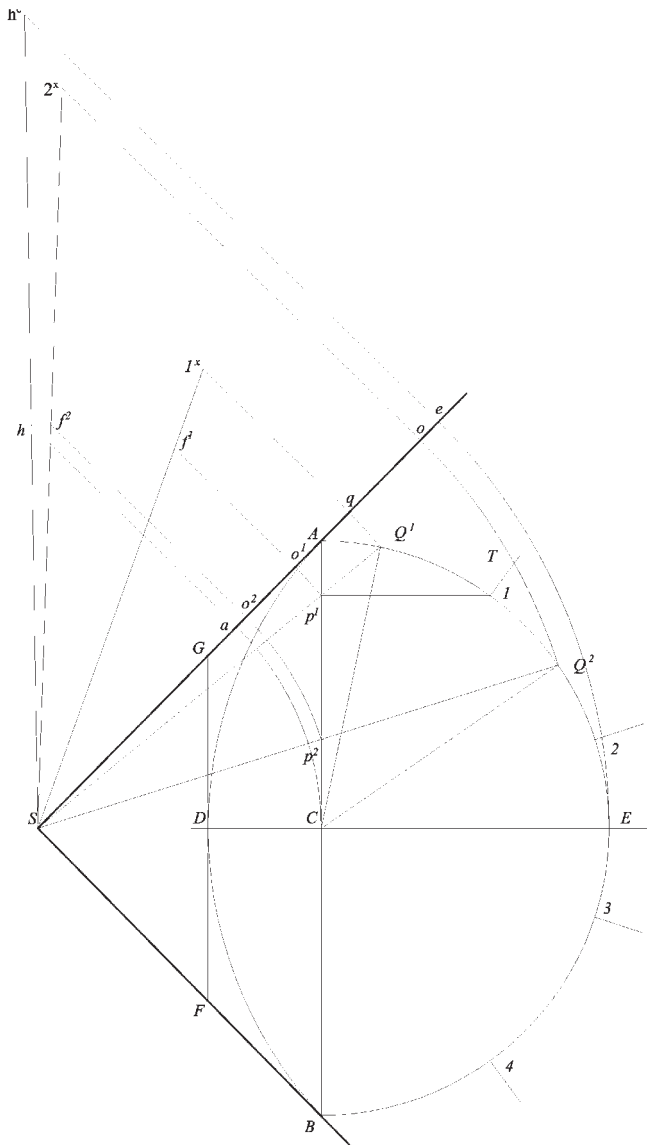
Fig. 67d - Volta conica in torre rotonda. Sviluppo delle superfici flessibili per il taglio dei conci.
