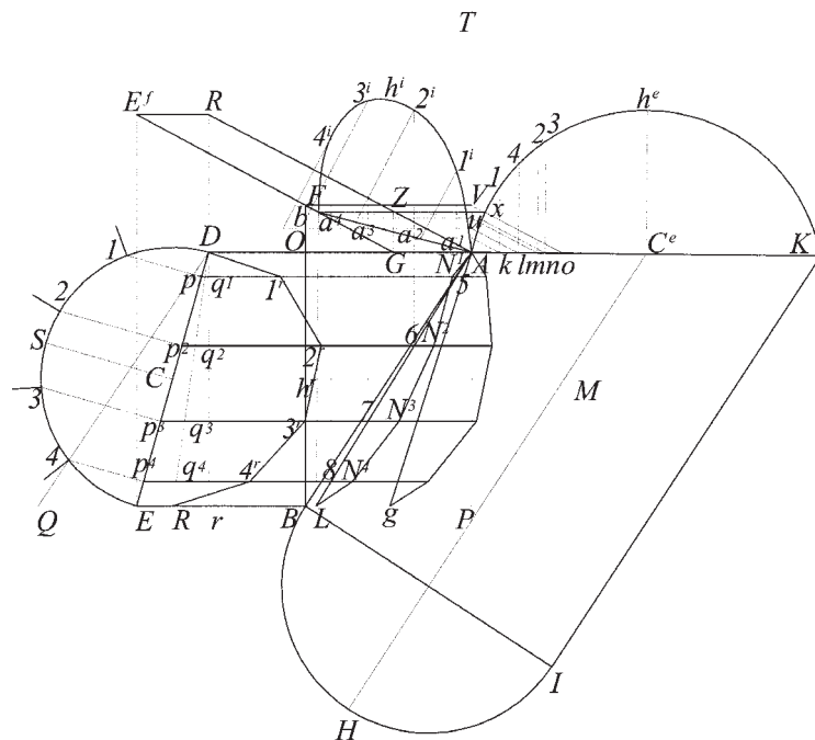
Fig.52.c ricerca delle larghezze dei pannelli per fare lo sviluppo
