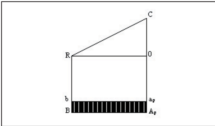
Fig 86. Linea di rampa, metà del piano orizzontale e altezza sull'orizzonte di una volta a botte in discesa
