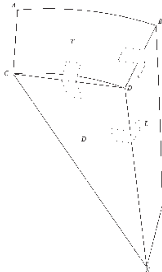
Fig. 310 Applicazione pratica del problema di Fig. 308 ad un mattone per volta conica disegnato in prospettiva.
