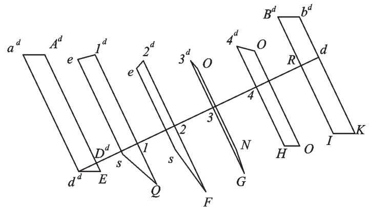
Fig. 280a Il procedimento è lo stesso usato per la costruzione dello sviluppo del cilindro di Fig. 272.
