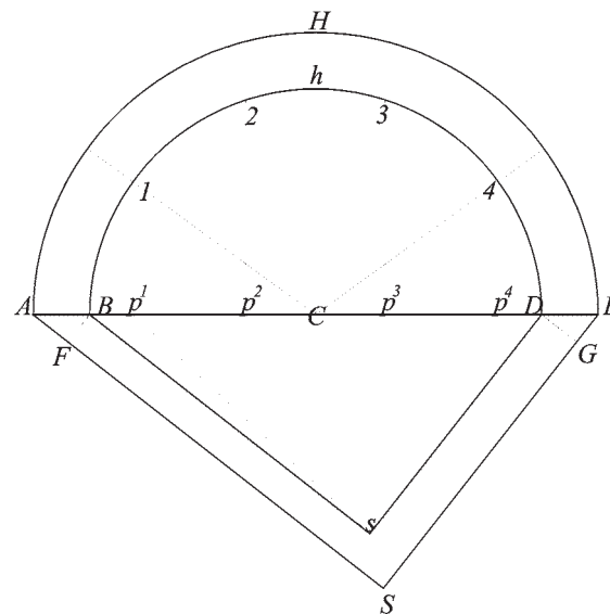
Fig. 104a: la prima disposizione con base triangolare e prospetto circolare, diviso nei suoi conci.
