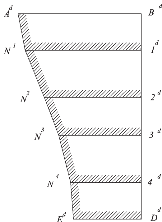
Fig. 89a Proiezione dello spigolo di volta
