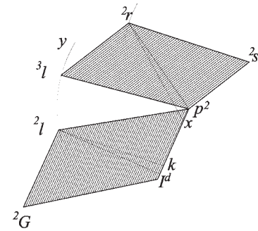
Fig. 289 Costruzione della superficie dell'intradosso piatto del primo concio
