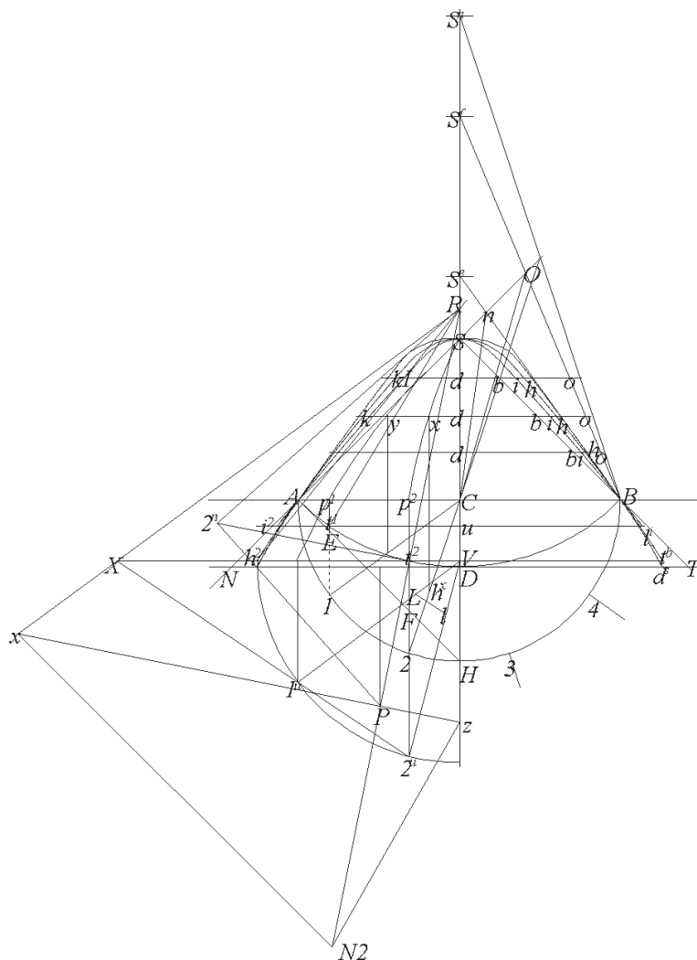
Fig.134 d Applicazioni del taglio sulla pietra
