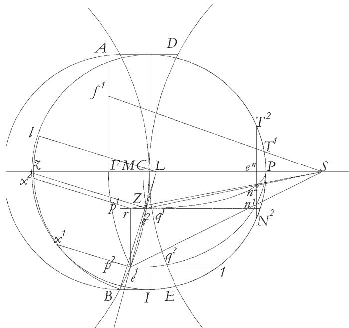
Fig.97a. Il disegno rappresenta il processo di costruzione della base di una torre cava.
