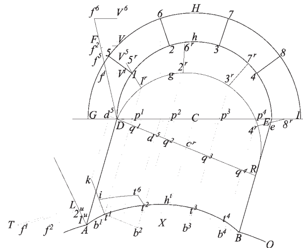
Fig.59 Proiezione sbieca ADEB di una porta a volta a botte su una base orizzontale di una porzione di torre cava a scarpa.
