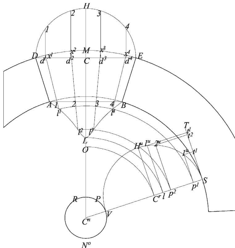
Fig. 170 Lunetta strombata dentro una vite St.Giles rotonda, o volta a crociera tornante e rampante
