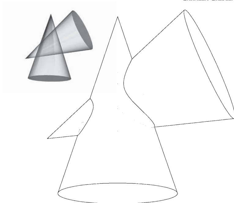
Fig 88. Intersezione di due coni i cui assi si incontrano obliquamente.
