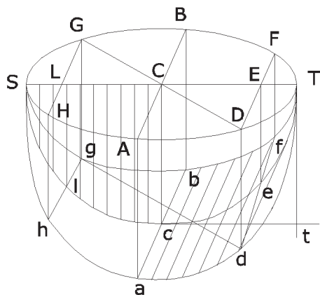
Fig. 27. La figura mostra come è possibile creare un “circulus imbricatus” tramite il cambiamento di posizione delle ordinate dalla quale si otterrà una curva a doppia curvatura.
