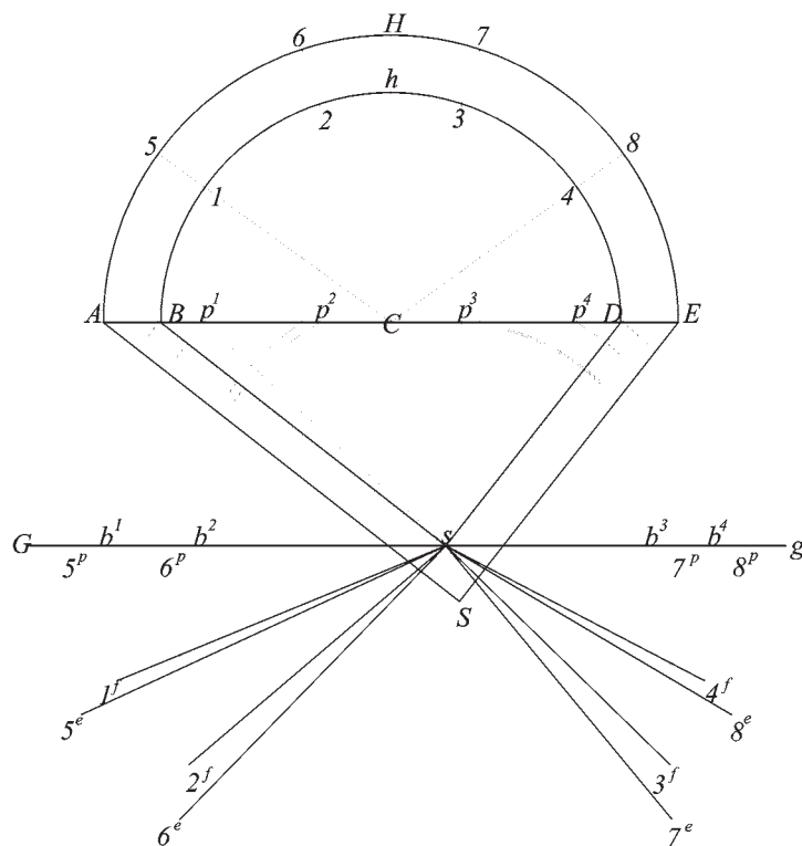
Fig. 104d: terzo metodo per cercare il valore dei giunti di letto tramite la base Gg.
