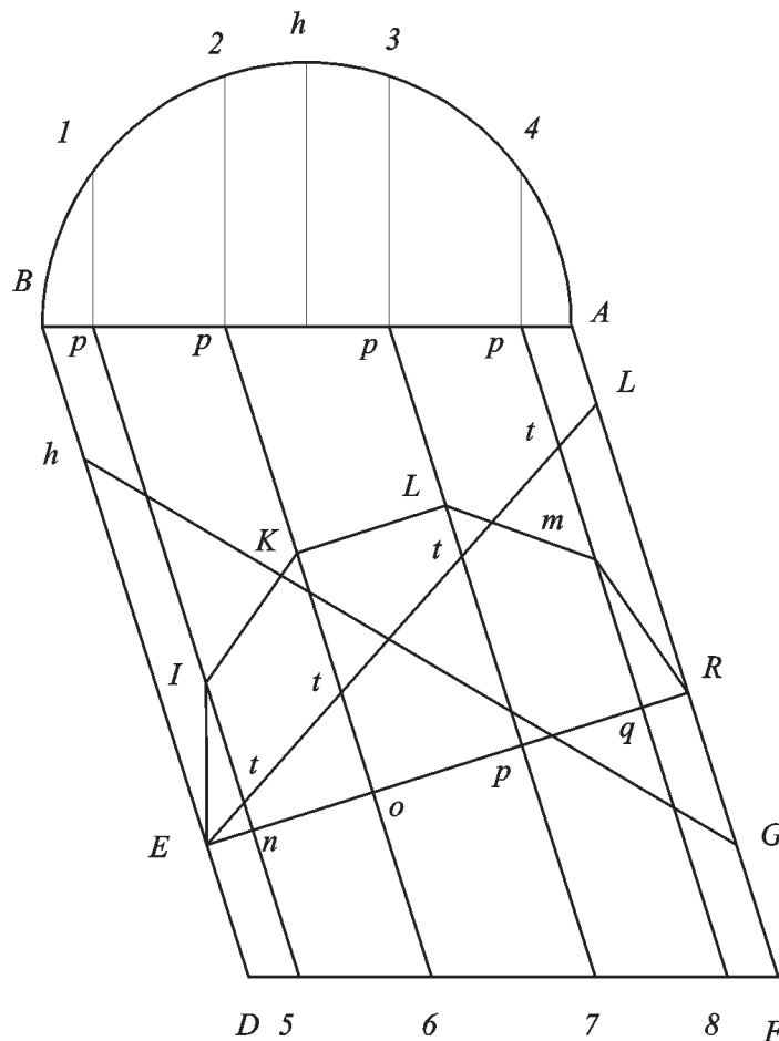
Fig. 270b Le rette EL ed hG non sono altro che le tracce dei piani secanti il cilindro, i quali formano ellissi o circonferenze.
