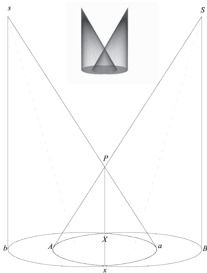
Fig 77. Intersezione di coni scaleni con assi che si incontrano al di sotto dei vertici
