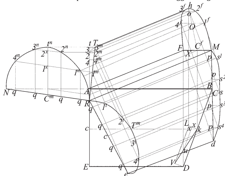
Fig. 93b Rappresentazione come si vede nella Fig. 93b della montata con le linee di livello trovate mediante piccoli archi di cerchio riportati su Rt con le diverse lunghezze dal profilo RT . Non aggiungiamo niente qui per quanto riguarda la formazione degli angoli, lo sviluppo, la formazione dei pannelli e l'applicazione della rappresentazione sulla pietra; in quanto il modo è lo stesso utilizzato per tutte le altre discese.
