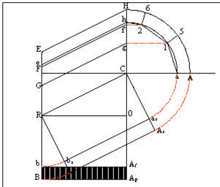
Fig 84. Piano orizzontale trasportato sulla linea di rampa RC
