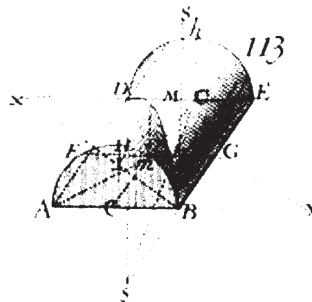
Fig.113: Vista prospettica di un Corne de Vache doppio o di una Volta biaise passé .
