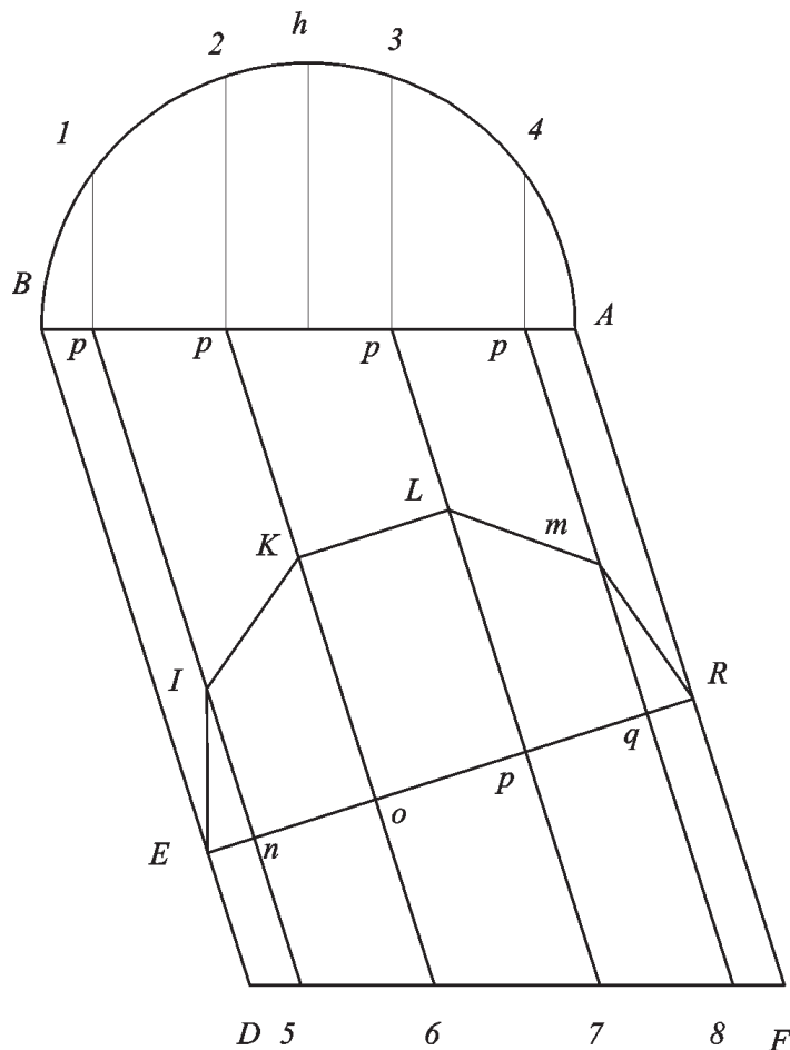
Fig. 270a Lo sviluppo del cilindro scaleno parte dalla figura che si ottiene sezionandolo con un piano passante per il suo asse.
