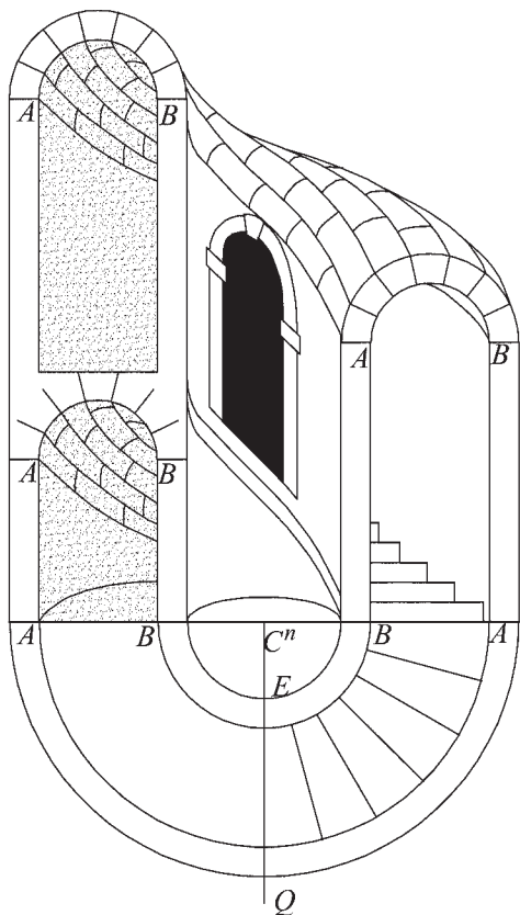
Fig. 225 Botte girante e rampante.
