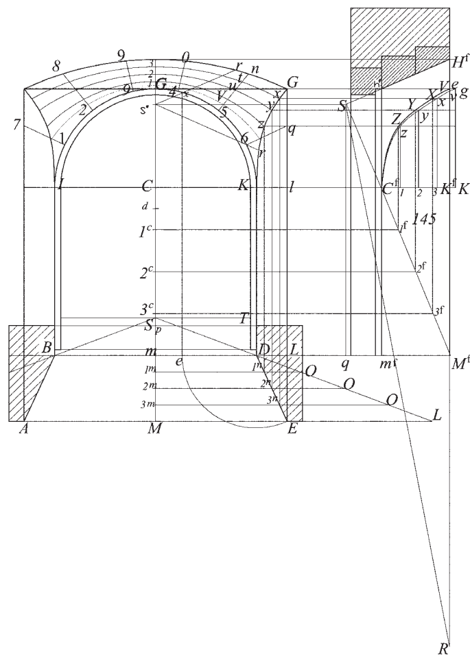
Fig.144-145 costruzione frontale e laterale dell'arriere-vossure
