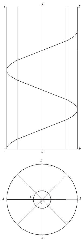
Fig. 184 Schema di costruzione della spirale realizzata dividendo in otto settori la circonferenza di base Sia per esempio un cilindro a b I F Fig. 184 Tavola 105 in cui il piano
