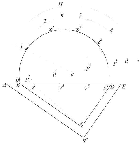
Fig. 106a: il metodo per circoscrizione, supponendo una sezione retta al di fuori del cono dato.
