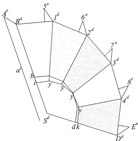
Fig. 105: vengono esplicitate le parti da sottrarre da ogni “doële”.
