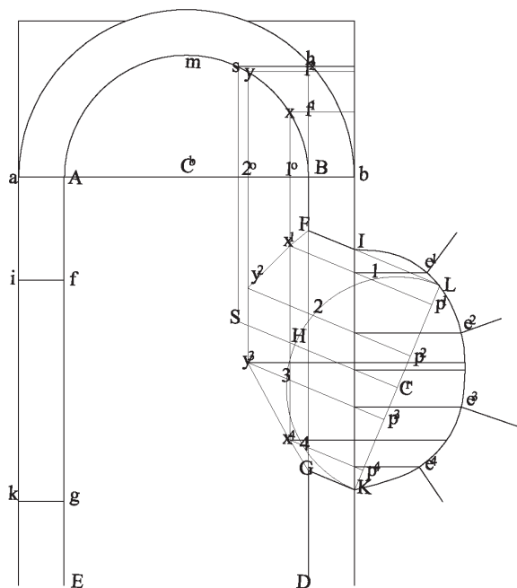
Fig. 30. 2 Sviluppo dell'intradosso ellittico attraverso il Prob. 8 del Secondo Libro : determinazione della faccia della lunetta sul paramento del muro.
