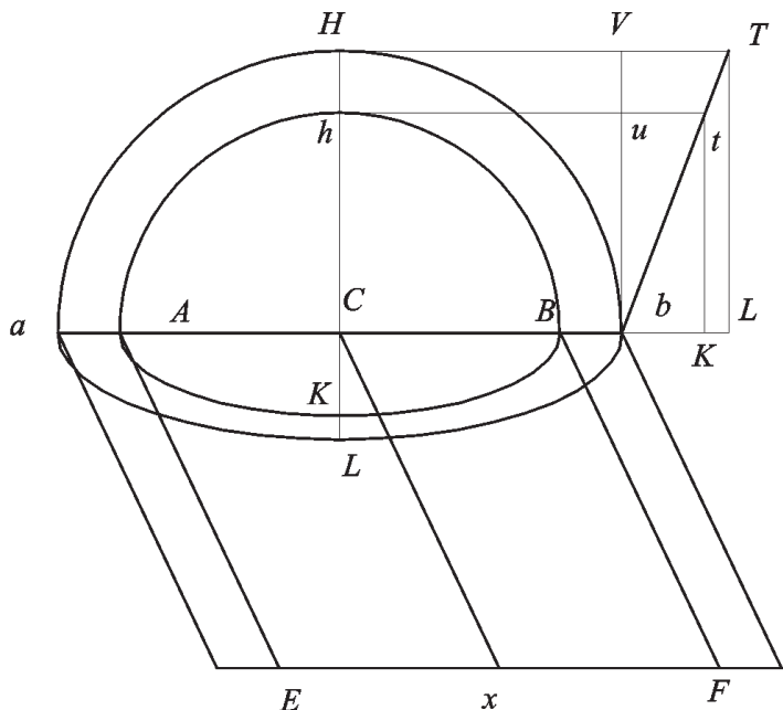
Fig. 274c Proietto dei punti dai semi-archi di intradosso ed estradosso sulle semi-ellissi.
