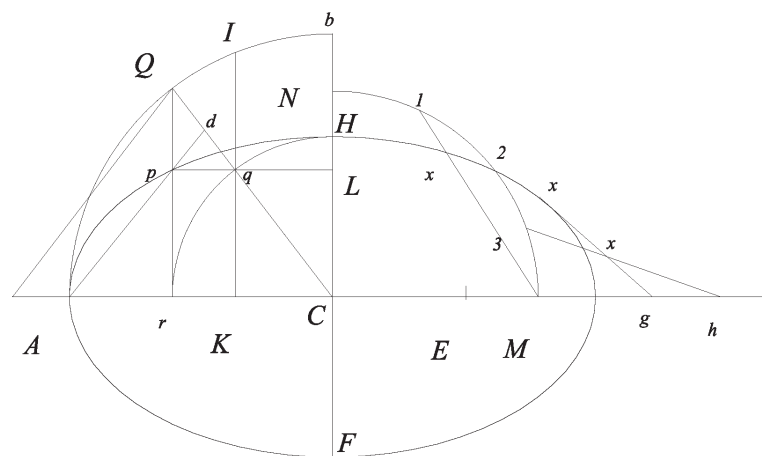
Fig. 116 Costruzione di un' ellisse per più punti.
