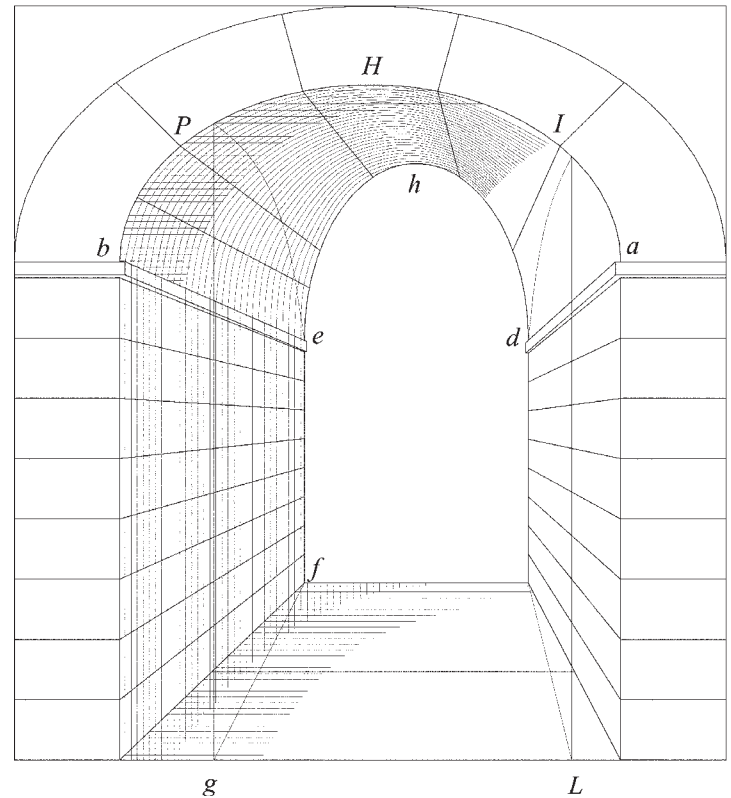
Fig. 231 prospettiva del passage ébrasé.
