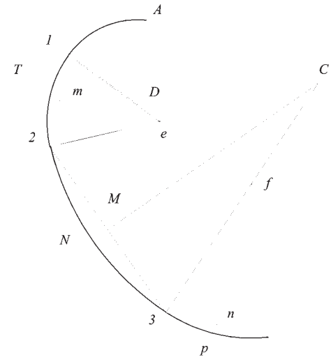
Fig.159: Costruzione di semi-ovali attraverso un numero indefinito di archi di cerchio COROLLARIO.
