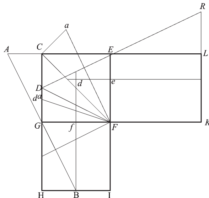
Fig.177 Costruzione di una rampa di scale con piani verticali perpendicolari tra di loro.
