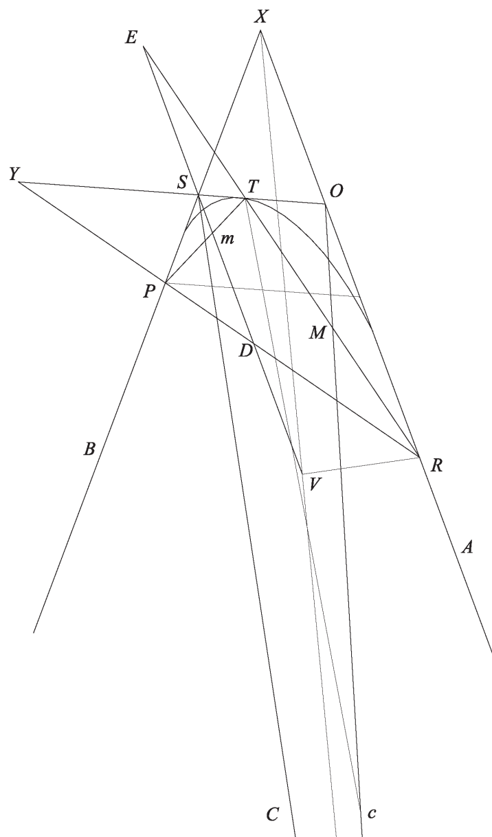
Fig.151 Sezione conica che rappresenta la centina dell'arco, dati i piedritti non paralleli e le linee di Rampa e di Sommità non parallele.
