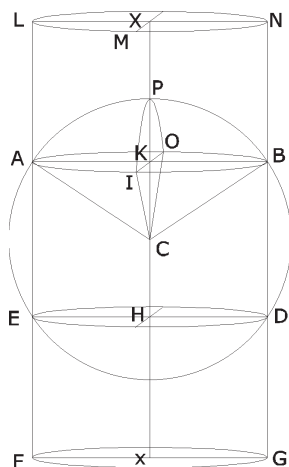
Fig. 32. Di sopra è riportato come un cilindro retto, entrando in una sfera, con il suo asse passante per il centro della stessa, crea nella sua intersezione una circonferenza.
