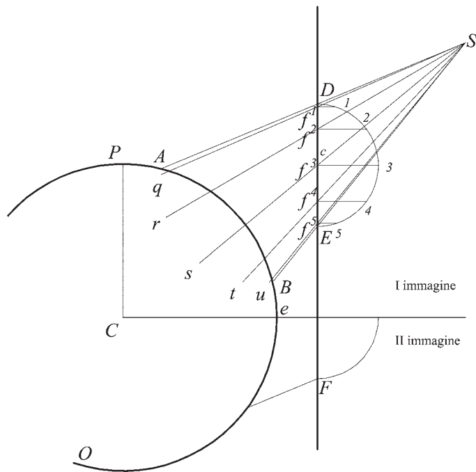
Fig.120a. Determinazione posizione lunotto e individuazione dei giunti di concio.
