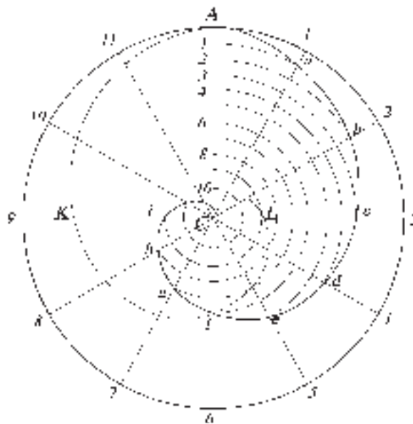
Fig. 136 Spirale d’Archimede.
