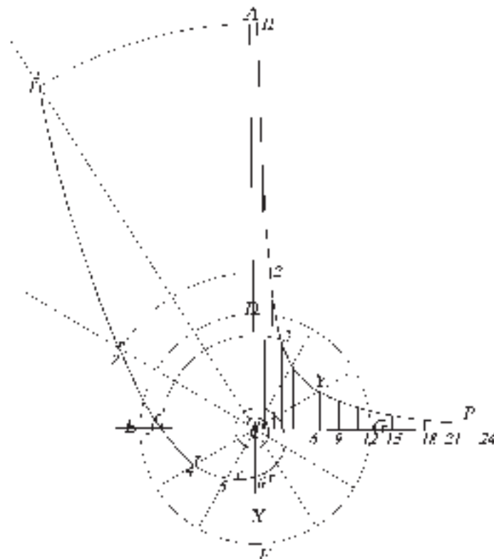
Fig. 141 Spirale avendo la curva generatrice un'iperbole equilatera.
