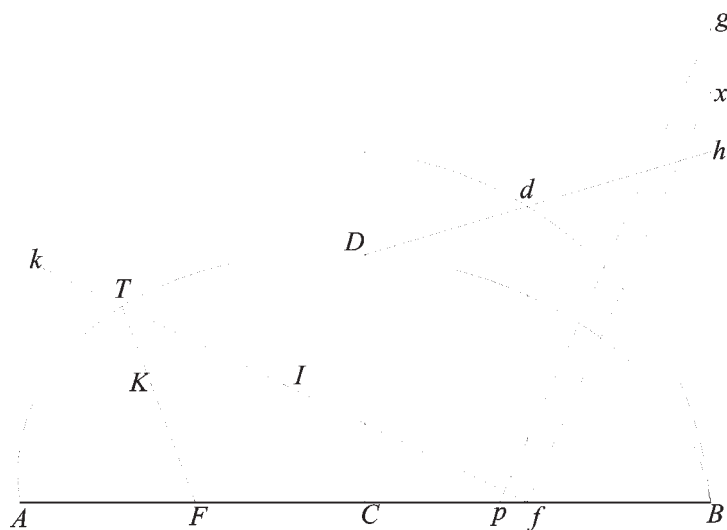
Fig.49. Attraverso l'unione di archi di cerchio otteniamo la circonferenza dell'ovale, da dove si porterà d' parallelo a CH , che taglierà il diametro AB in f ,
