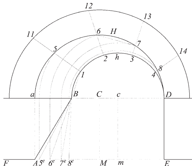
Fig. 132a L'arco aHD e BhD non sono concentrici perciò si avranno delle divisioni dei concii particolari.
