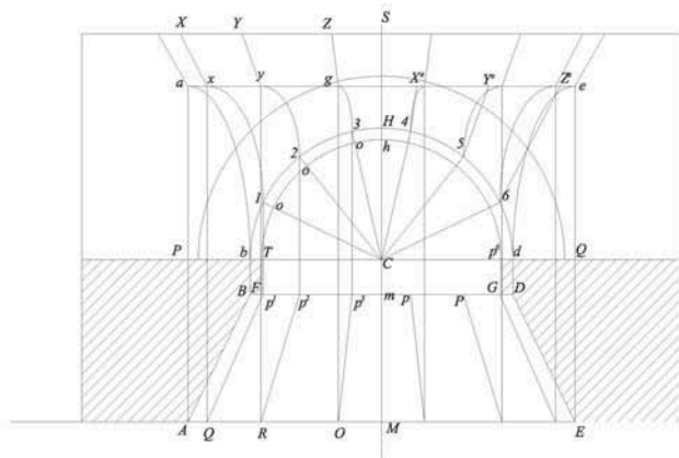
Fig. 261G - Costruzione della volta di Montpellier attraverso il terzo metodo sopradescritto in cui le le direzioni dei giunti delle facce di letto sono fatte su dei piani verticali diretti ad un punto S.
