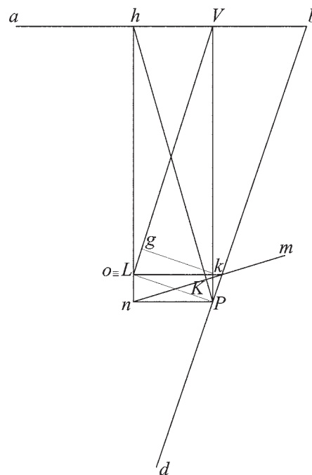
Fig. + : Figura supplementare utile per trovare il semidiametro dell'arco di faccia. Si dividerà quindi, nella Fig. 92b , FM in due parti uguali in K e si porterà la lunghezza Kn della preparazione di K in X , ove passerà Xh
