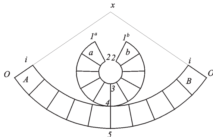
Fig. 278a Sviluppo della prima e seconda corona.
