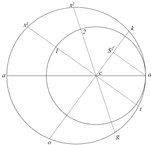
Fig. 134 Sezione verticale del cono, in cui si trova il vertice dell'iperbole di profilo.
