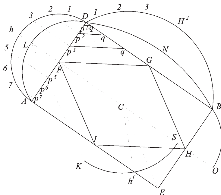
Fig. 213c Sviluppo della porzione di ellisse ALDNBO in cui LDNBO rappresenta il profilo o sezione verticale della volta.
