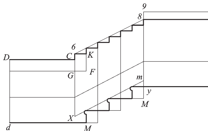
Fig. 176 Profilo della fig. 173
