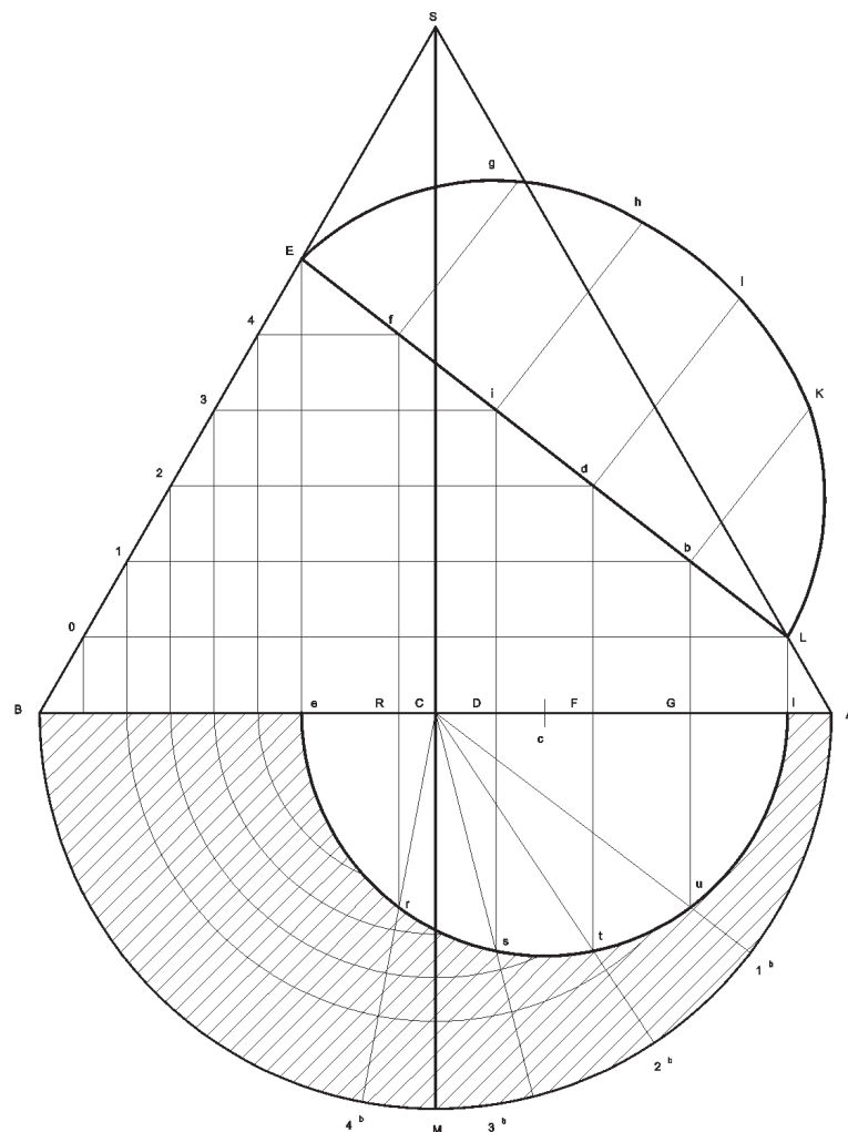
Fig. 183 b Sezione del cono: ellisse
