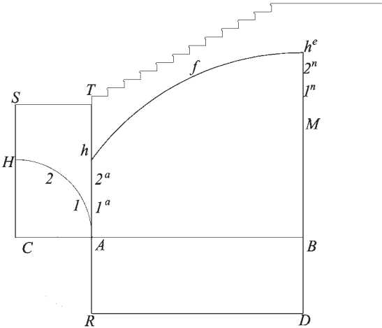
Fig.253a proiezione orizzontale della semivolta a botte retta all'imposta e curva sotto la chiave di volta.
