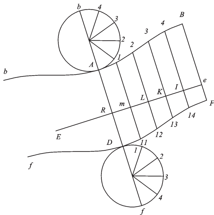
Fig. 272c Lo sviluppo del cilindro è completo.
