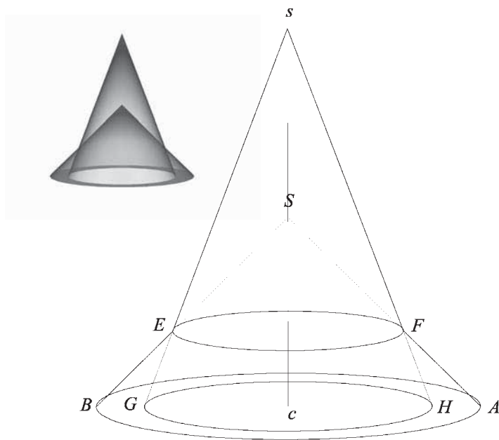
Fig 81. Intersezione di coni in cui si confondono le basi e gli assi.
