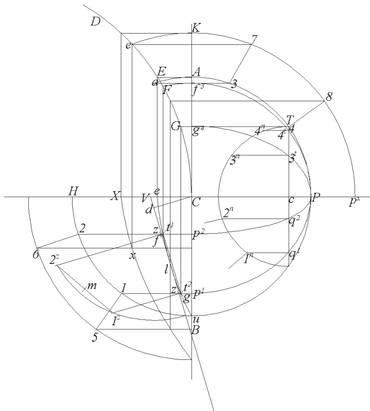
Fig. 101 d Costruzione delle divisioni dei concii di cui P^n e 2^n sono le proiezioni orizzontali attraverso il ribaltamento dell'arco di giunzione passante per il punto 4
