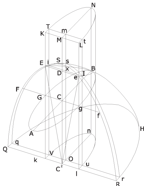
Fig. 40. Esempificazione della fig. 38 tramite sezione sull'asse del cilindro retto.
