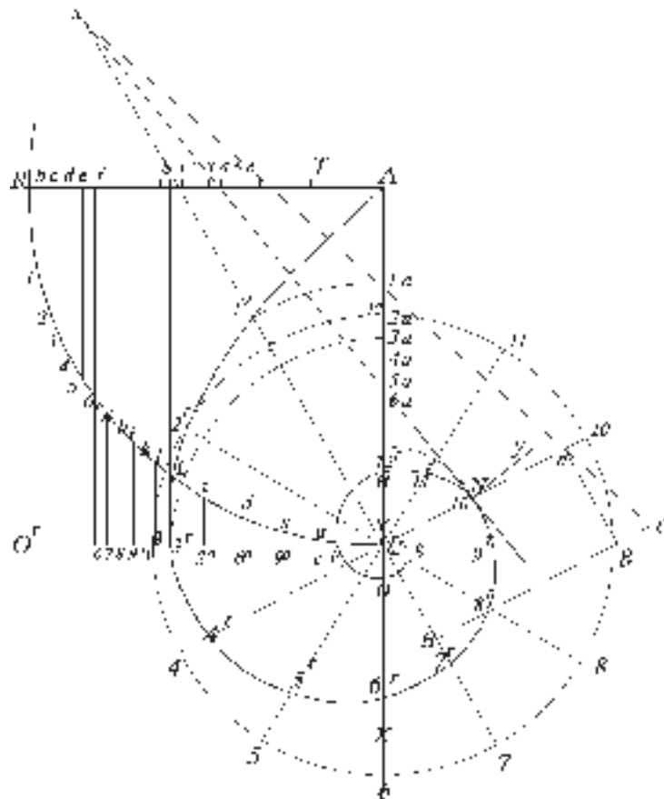
Fig. 140 Spirale circolare o ellittica o parabolica.
