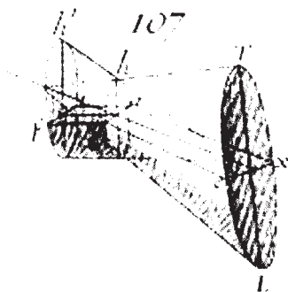
Fig.107: Intersezione di due coni retti con asse comune inclinato. Invece di avere gli assi sulla stessa linea, hanno un lato in comune Cc sotto il mezzo della chiave, nella linea s^o s^e , che si suppone retta, cosa che mostra la necessità di una rappresentazione di piano e una di profilo per restituire bene la posizione dei due coni scaleni.
