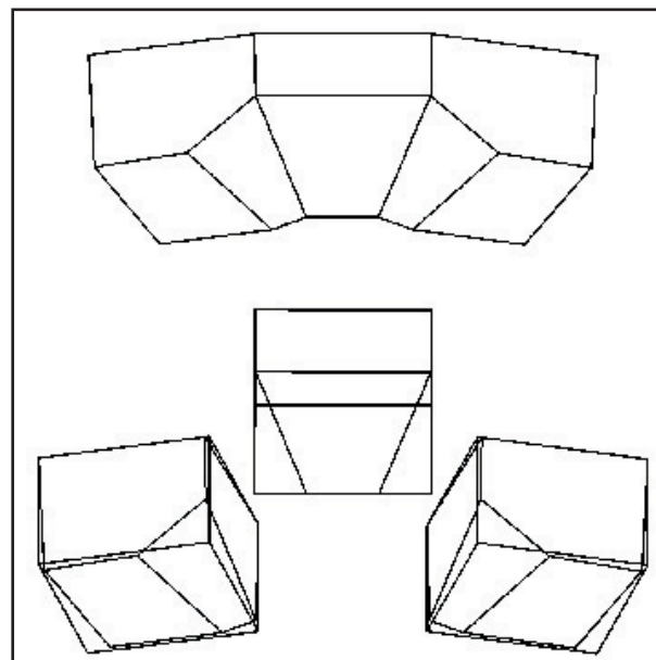
Fig.115d In questa figura gli stessi elementi regolari in pietra della fig.5 sono stati sbizzati, invece che sagomati. Notare come le linee curvilinee della figura precedente si sono tradotte in spezzate rettilinee (sicuramente di più facile realizzazione).
