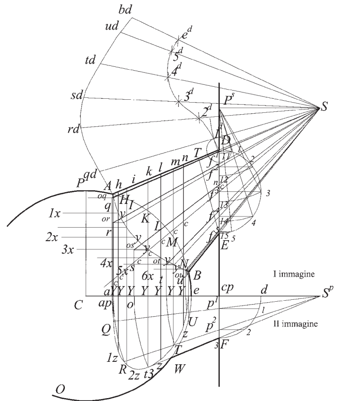
Fig.120e. Rettifica della superficie interna del lunotto.
