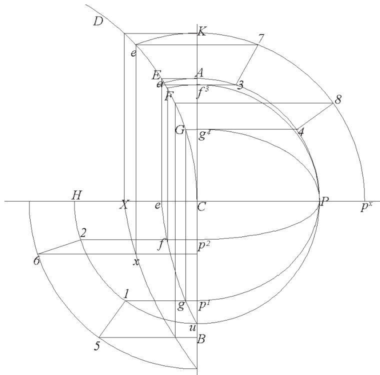
Fig.101 c Costruzione della proiezione del secondo arco di giunzione ( Xx ) della nicchia con la volta a botte
