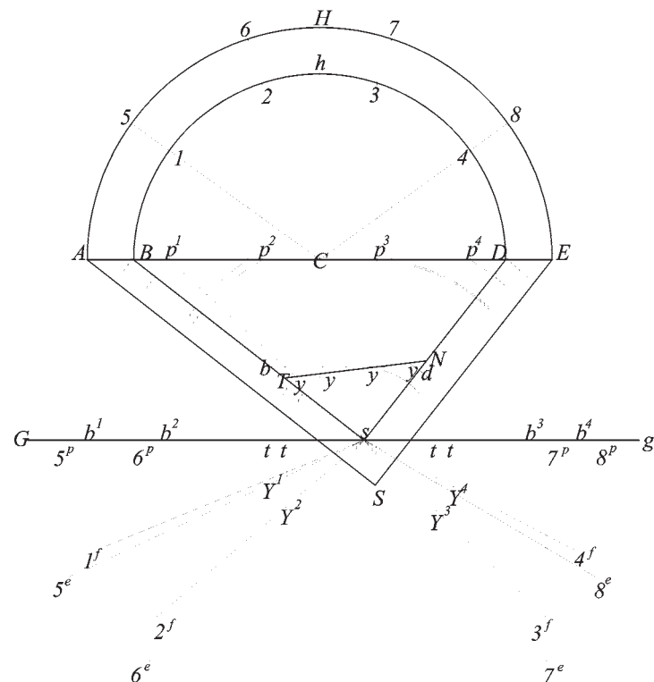
Fig. 104e: si ottiene la lunghezza che deve essere sottratta da ogni giunto.
