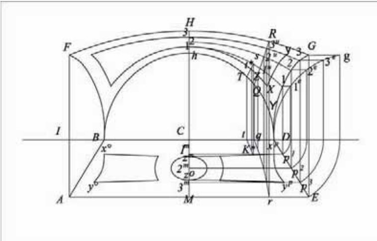
fig 151c nella figura viene tracciato il disegno della decorazione unendo i punti delle curve trovati in precedenza
