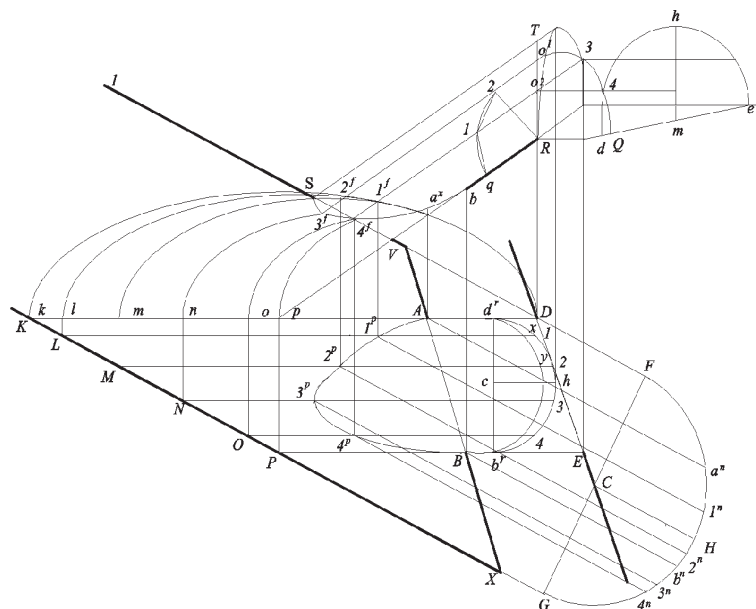
Fig.55 Costruzione in P.O. dell'incrocio della volta a botte sbiega e con la lunetta sbiega e in discente.
