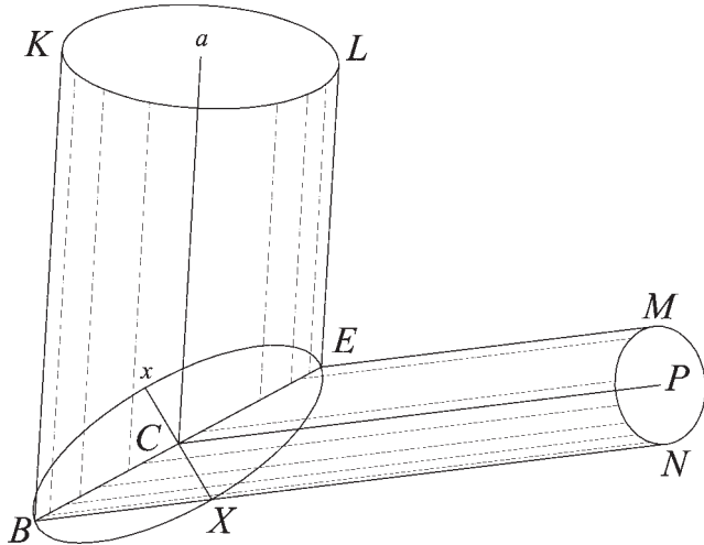
Fig. W L'ellisse BXCx è comune ai due cilindri scaleni KLEB e EMNB .
