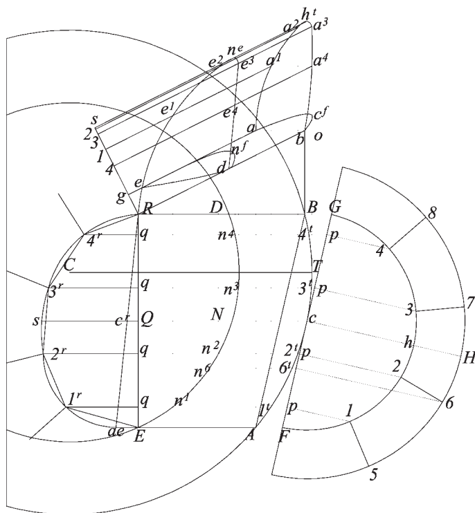
Fig. 38 Visualizzazione dell'arco retto nel caso il piano di sviluppo sia orizzontale alla direzione del piano verticale e dell'arco rampante nel caso del piano inclinato.
