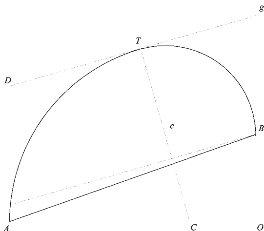
Fig.157: Costruzione di un arco rampante in cui i piedritti sono paralleli e la linea di pendenza non è parallela a quella di sommità Terzo caso dove la linea di sommità Dg [Fig.157.] non è parallela alla
