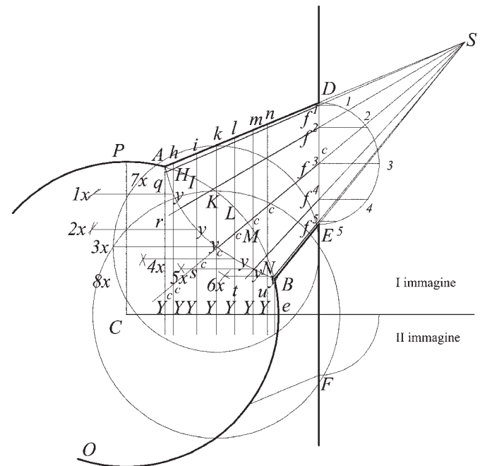
Fig.120b. Determinazione della proiezione verticale dello spigolo interno superiore di intersezione tra lunotto e volta sferica.
