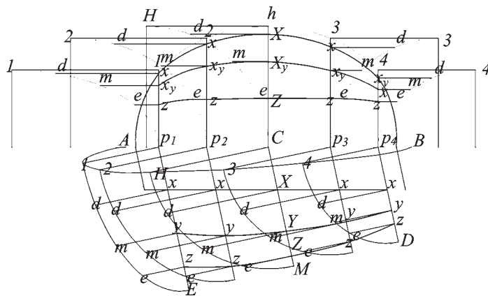
Fig.251. Sezioni di una volta irregolare.
