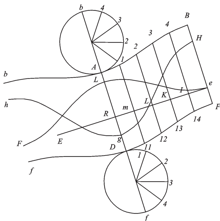
Fig. 272d Con lo stesso procedimento possiamo ottenere anche lo sviluppo dell'ellissi e delle circonferenze.
