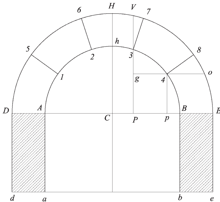
Fig. 59 In Figura sono mostrati i rapporti geometrici in una Volta a Botte in Pieno Centro.
