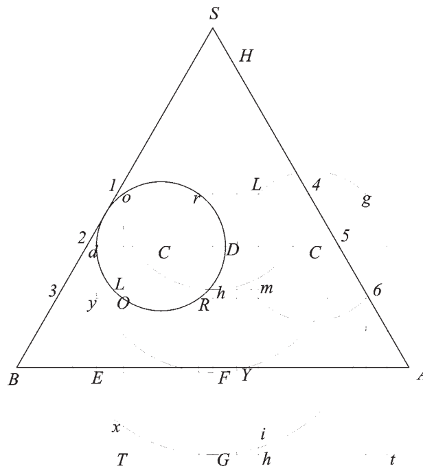
Fig.200. Intersezione tra un cilindro ed un cono con gli assi perpendicolari.
