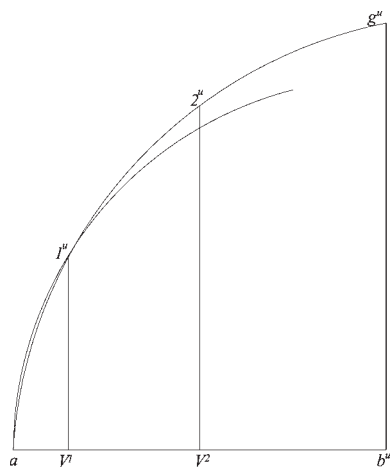
Fig.254 costruzione per la sagomatura dei conci
