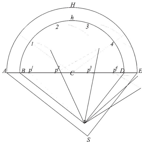
Fig. 104b: primo metodo per cercare il valore dei giunti di letto considerando le proiezioni come basi di profilo.
