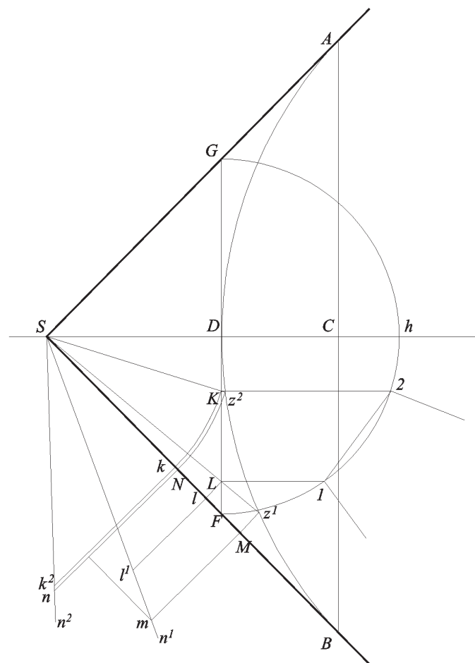
Fig. 67c - Volta conica in torre cava. Sviluppo delle superfici flessibili per il taglio dei conci.
