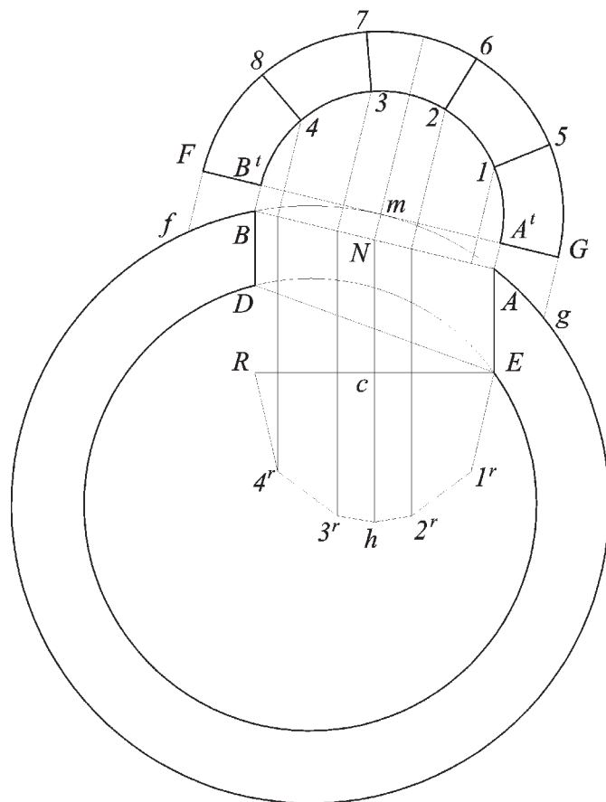
Fig.37a Primo metodo: Centina primitiva sulla corda AB
