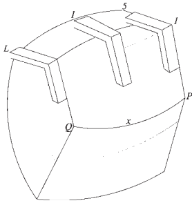
Fig.252 realizzazione del concio in pietra all'intradosso della volta
