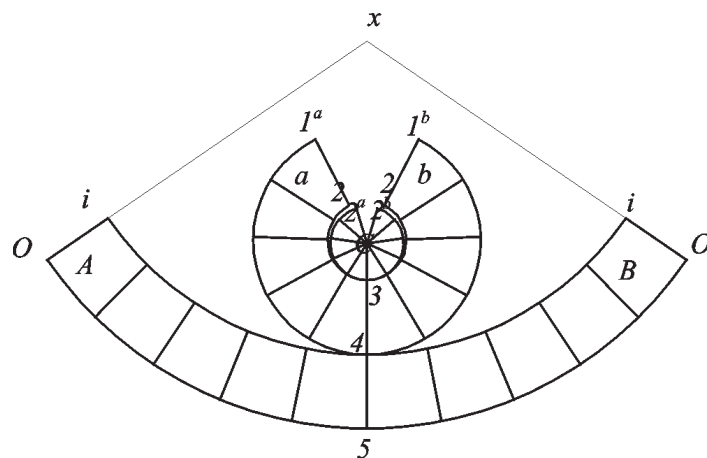
Fig. 278b Sviluppo completo dell'emisfero superiore della sfera.
