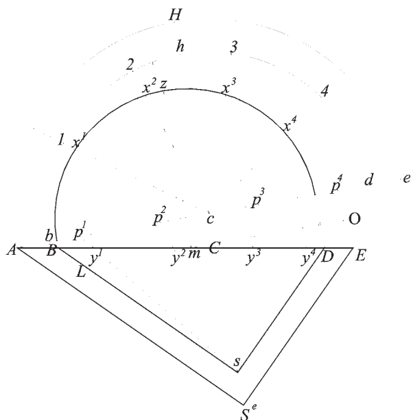
Fig. 106b: individuazione del semiasse coniugato a quello dato.
