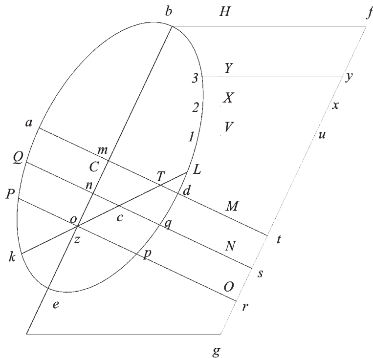
Fig. 170 La proiezione dell'ellisse, sia sul piano orizzontale che su quello verticale, è una linea retta
