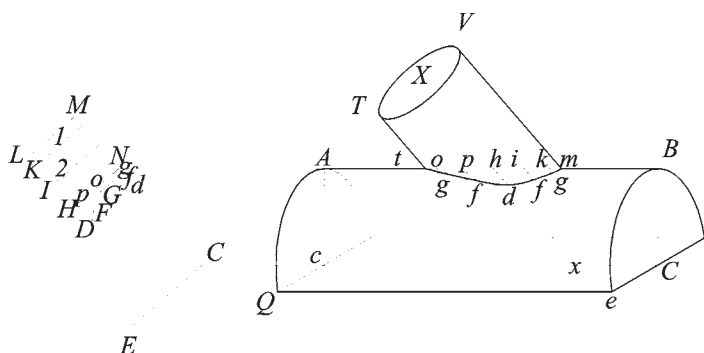
Fig.190. Intersezione tra cilindri con assi inclinati.
