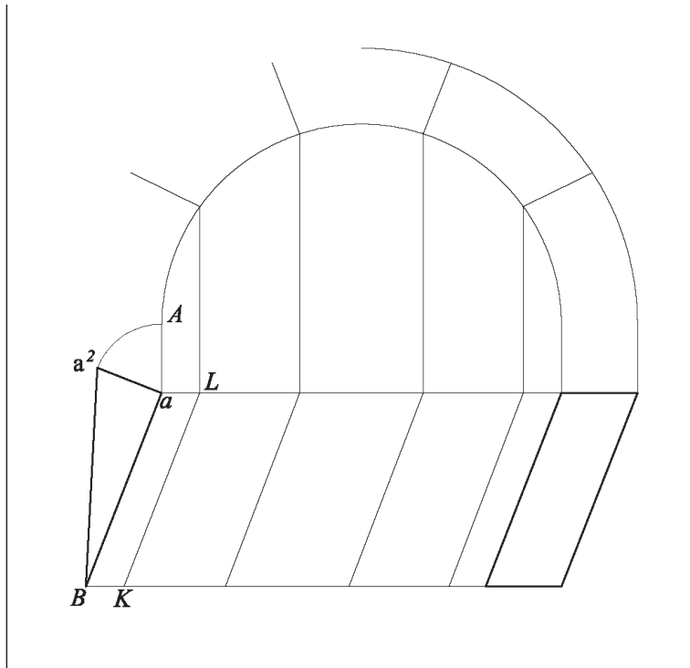
Fig.296 Faccia inclinata verso i giunti di letto.
