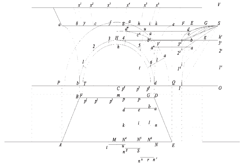
Fig. 261D e 262 - Costruzione della volta di Montpellier attraverso il secondo metodo sopradescritto in cui le le direzioni dei giunti delle facce di letto sono parallele alla direzione della volta.
