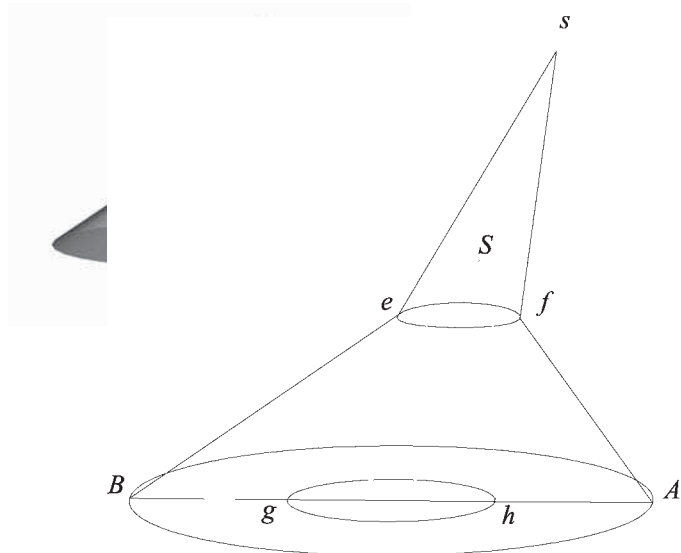
Fig 82. Intersezione di coni scaleni in cui si confondono le basi e gli assi.
