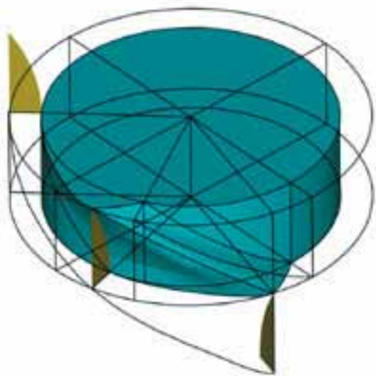
Fig. 226 C Completamento del taglio della pietra attraverso l'uso della sagoma convessa che riproduce l'intradosso del cuneo.
