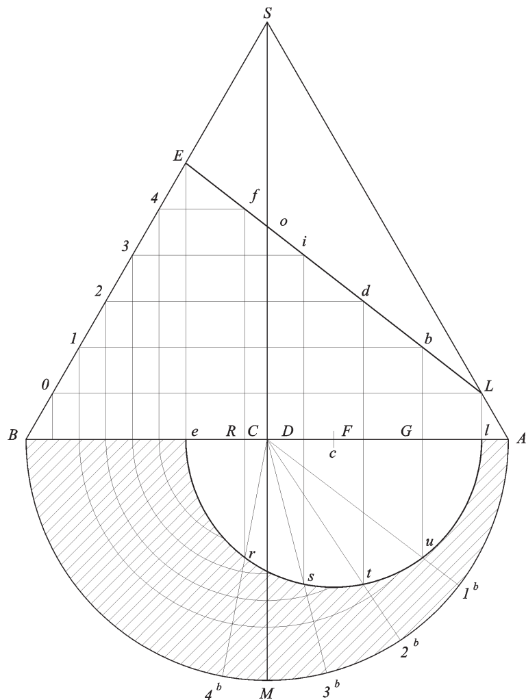
Fig. 183 a Rappresentazione della base in ellittica in proiezione ortogonale: porteranno delle perpendicolari a BA , come 4^l , 3^l , 2^l , 1^l , 0^l , fino all'incontro dell'asse EL , e attraverso i punti fi , db , si caleranno delle perpendicolari alla base BA prolungate fino al cerchio esl , come bu , dt , is , fr che taglieranno la sua circonferenza ai punti r , s , t , u , attraverso i quali e attraverso il centro C si traceranno le linee Cr4^b , Cs3^b , Ct2^b , Cu1^b , che daranno sulla base del Cono i punti 4^b , 3^b , 2^b , 1^b , attraverso i quali e attraverso il vertice S si traceranno delle linee rette sulla superficie che non è stata segnata nella Figura 183 , ma bensì nella Figura 185 , che
