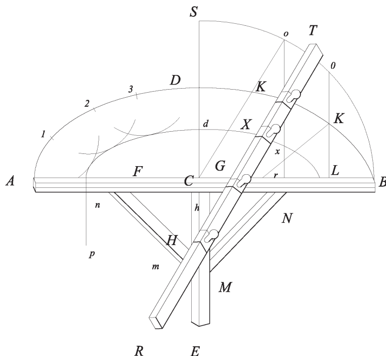
Fig. 117 Costruzione di un'ellisse con uno strumento chiamato Compasso.
