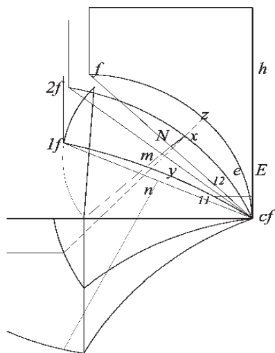
Fig. 129 L'arco AB sembrerebbe diviso in conci di uguale misura, questo porterebbe a un disegno diverso dei giunti di letto in facciata da quello presentato nella Fig.45
