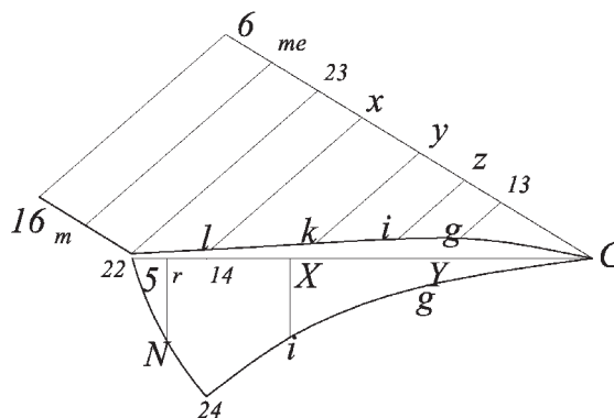
Fig. 128 L'arco AB sembrerebbe diviso in conci di uguale misura, questo porterebbe a un disegno diverso dei giunti di letto in facciata da quello presentato nella Fig.45
