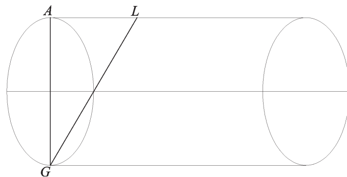
Fig. 176a Costruzione dell'ellisse sulla superficie del cilindro, il cerchio mediante linee diritte parallele all'asse si sarà su una superficie piana a parte ( Fig. 178 ) un angolo ga , uguale a quello dell'asse del cilindro sulla base, retto se il cilindro è retto ed
