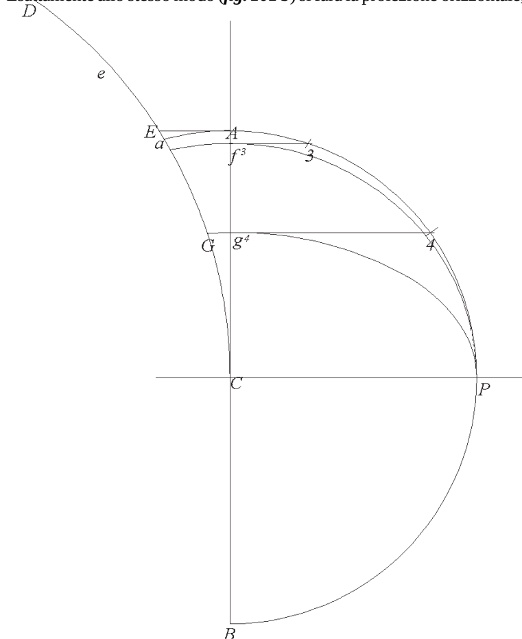
Fig. 101 a Immagine di profilo della nicchia a porzione di sfera nel suo incontro con la volta a botte
