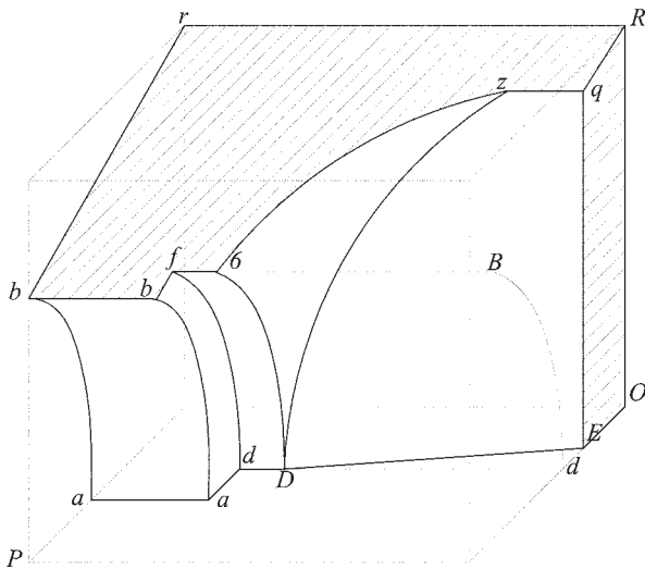
Fig. 148 settimo concio della doele.
