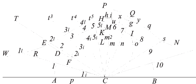
Fig.47 Costruzione per ottenere i conci dell'arco
