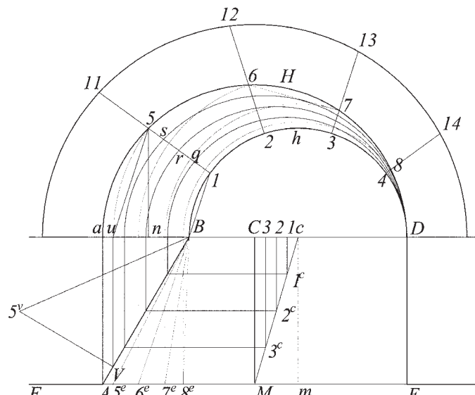
Fig. 132b Sia l’arco più piccolo e quello più grande vengono creati dei semicerchi ausiliari.
