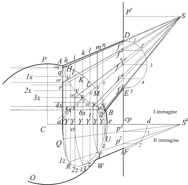
Fig.120d. Determinazione della vera lunghezza dei giunti dei concii inferiori del lunotto.
