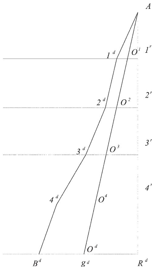
Fig.53 sviluppo degli intradossi
