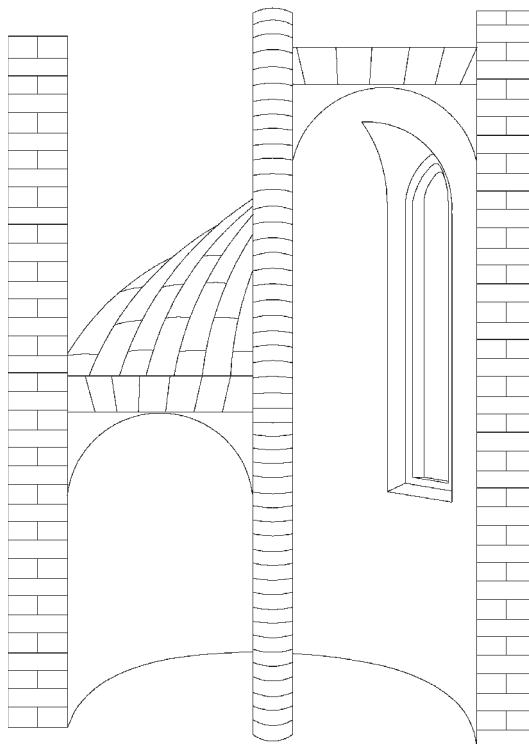
Fig. 170 Lunetta strombata dentro una vite St.Giles rotonda, o volta a crociera tornante e rampante
