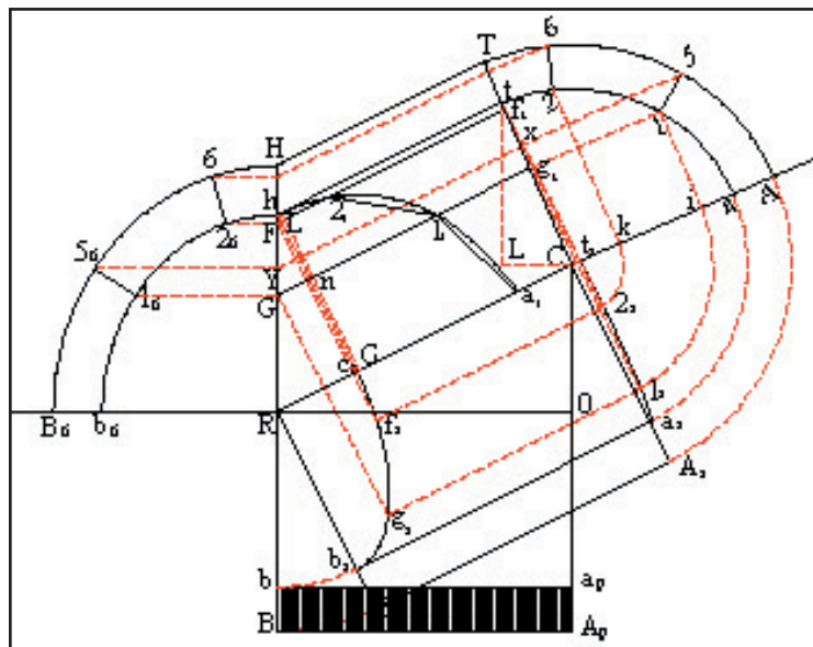
Fig 86. Proiezione dell'arco-retto ribassato
