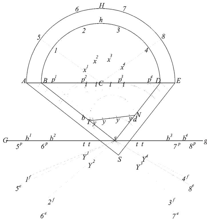
Fig. 104i: la costruzione precedente cambia se si ipotizza che la faccia sia rialzata o ribassata.
