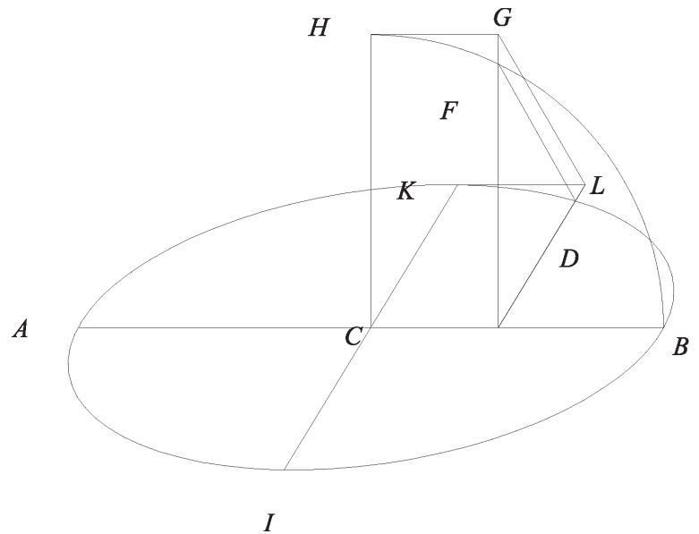
Fig. 113 Impiego di un Ellisse per trovare uno dei diametri coniugati avendo almeno un diametro e la sua ordinata.
