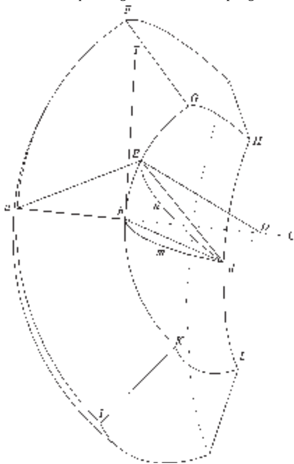
Fig. 304. L'angolo d'insolazione di due piani di curvatura, misurate per le linee oblique alla loro comune sezione, è più acuto di quello che misurano le loro perpendicolari su queste alla comune sezione.
