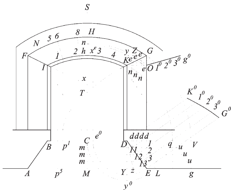
Fig. 138b Volta posteriore bombata con centro O della chiave dell'arco di battuta e di battamento della curva KG per ottenere la vera grandezza
