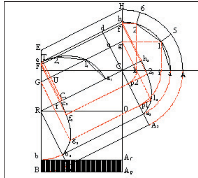
Fig 84. Proiezione dell'arco-retto ribassato
