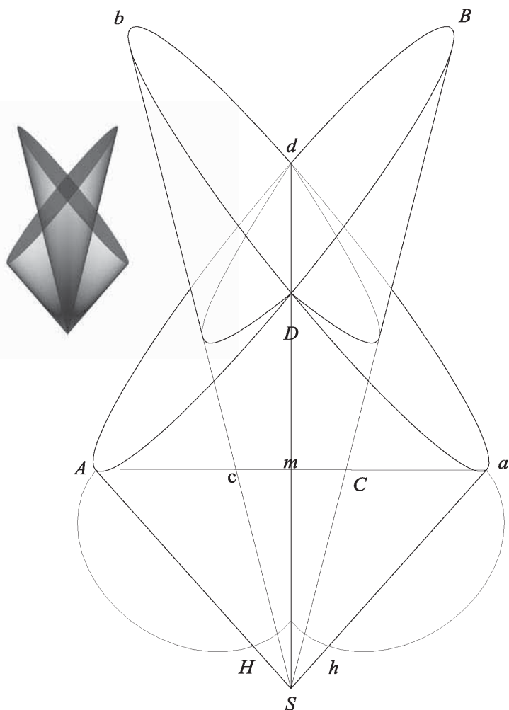
Fig 80. Intersezione di coni scaleni in cui l'asse di uno coincide con il lato dell'altro e viceversa
