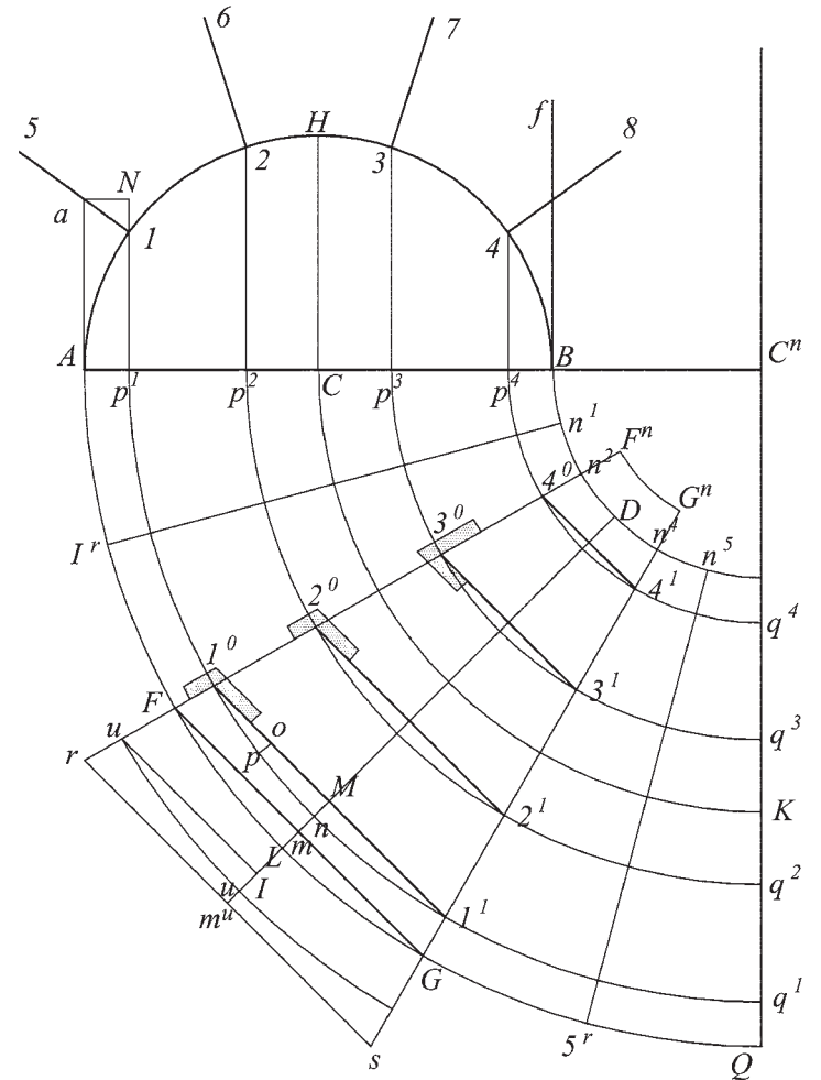
Fig. 224 b Determinazione delle lunghezze dei Cunei. Si notano i calandrini per la sagomatura delle pietre agli intradossi 1^01^1 , 2^02^1 , 3^03^1 .
