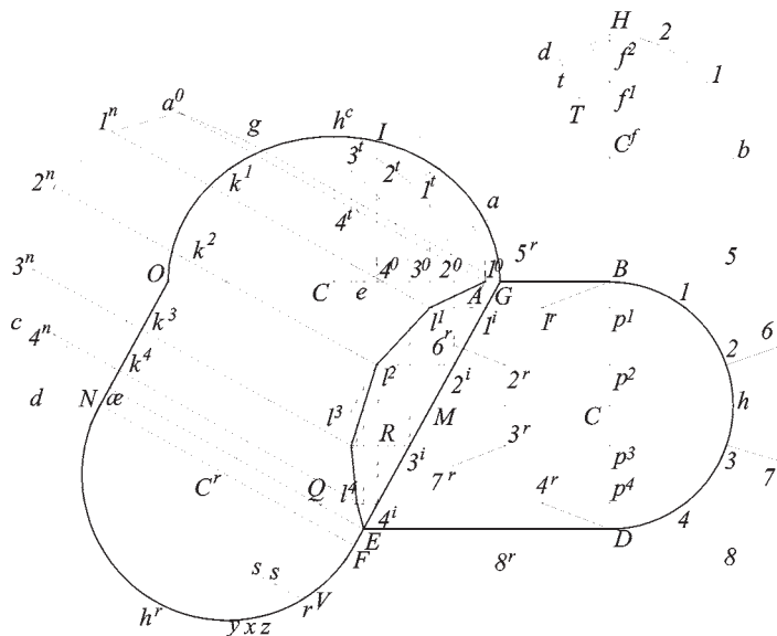
Fig. 50 Il disegno rappresenta la proiezione orizzontale dell'incontro di due volte a botte, una discendente e l'altra di livello, in cui il poligono A^r E è la proiezione della lunetta generata dall'incontro di queste due volte.
