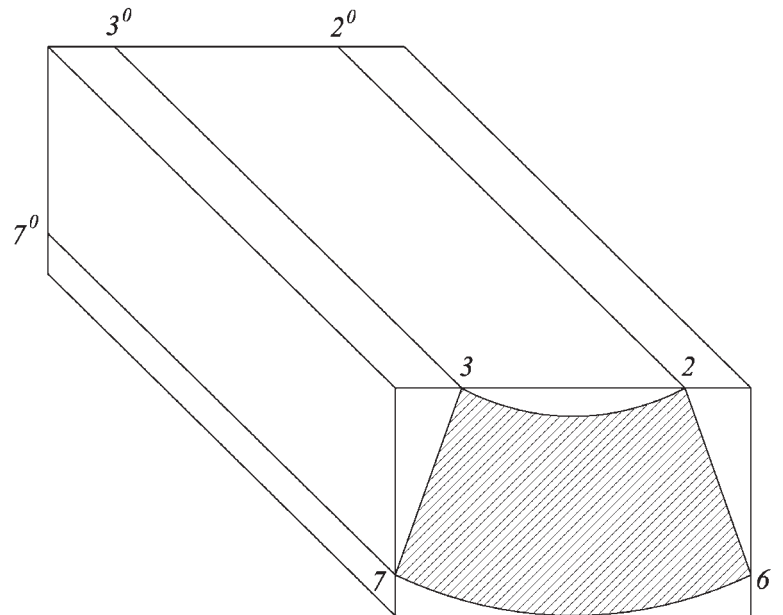
Fig. 59q Assonometria del concio 3487 di Fig. 59 .
