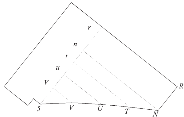
Fig. 146 costruzione del giunto della doele quinto concio.
