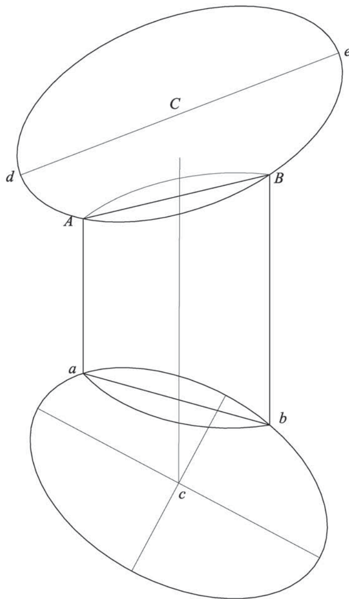
Fig. 100 La sezione fatta dall'incontro di un cilindro e di uno sferoide, i cui assi non si incontrano, è una specie di "ellissoimbre"
