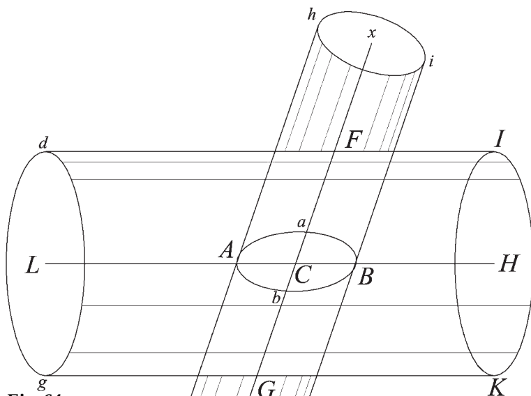
Fig. 64 Se il piccolo cilindro fosse scaleno allora la sua sezione solida non sarà più un Ellipsimbre ma sarà un Cicloimbre.
