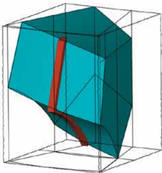
Fig. 227 b Cuneo concavo convesso sul lato del Nocciolo. Si noti come la differenza con il cuneo della fig. 229 consista nell'angolazione delle teste opposte verso l'interno. Vista assonometrica.
