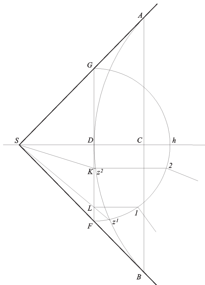
Fig. 67b - Volta conica in torre cava. Sviluppo delle superfici flessibili per il taglio dei
