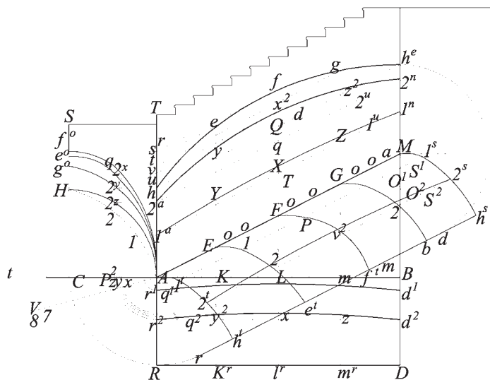
Fig 253c semivolta a botte retta all'imposta e curva sotto mla chiave di volta.
