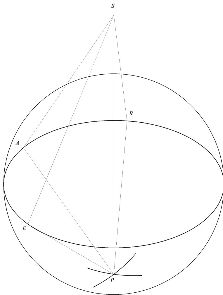
Fig. 173 g Altro metodo per l'individuazione di un cerchio maggiore
