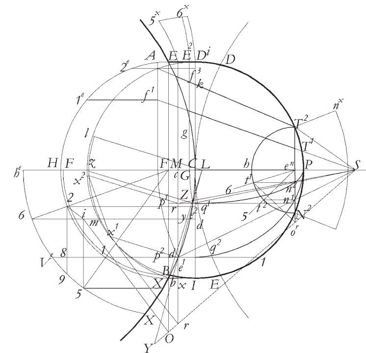
Fig.97b Il disegno rappresenta il processo di costruzione della base di una torre cava nella quale si vuole creare una nicchia, il cui sviluppo della porzione cilindrica taglia la torre.
