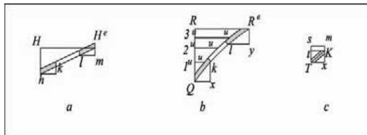
Fig.152: Nelle tre figure, sono riportate le tre sezioni( Hh, RQ, Ts ) attraverso le quali è possibile ricavare la vera grandezza del disegno dell'infisso.Nella fig.152a l'altezza hH viene riportata in vera grandezza, perpendicolarmente ad essa in h viene inserita la misura di CM, che è l'altezza del trapezio dato ABDE, così da formare un triangolo rettangolo, sul quale porterò le tracce del disegno della figura, attraverso k l, che nella fig 151 b indico con z" e z'. fig.152b sempre con il solito sistema di prima individuo una sezione generica dell'infisso QR che rappresento nella figura 151b, RR' corrispondente di nuovo a CM, con i punti kl indico due generici punti del fregio che nella figura successiva vado ad indicare con le lettere 3"4"fig.152c qui sono riportati due punti il punto T e il punto s, i quali sono stati trovati unendo la curva di altezza centrale con l'arco dell'intradosso. T è un punto generico, la direzione corretta Ts viene data come proseguo della retta che unisce o a T, dove o rappresenta il centro delle due circonferenze che hanno come centro l'una il punto C e l'altra il punto I.
