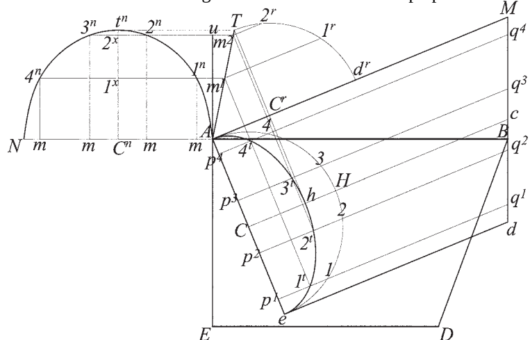
Fig. 92c : Innalzamento della faccia della montata, effettuato mediante le divisioni del profilo di faccia inclinata, innalzamento in vera grandezza, per avere la posizione della base Lk , se si crea l'angolo del pendio fuori dalla posizione ove è stato messo, si deve solo aggiungere all'angolo retto VLk l'angolo NDB , oppure creare subito questo angolo uguale a EDB .
