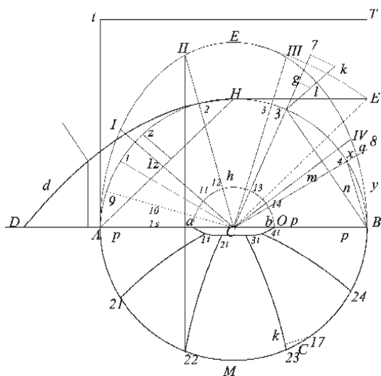
Fig. 129 L'arco AB sembrerebbe diviso in conci di uguale misura, questo porterebbe a un disegno diverso dei giunti di letto in facciata da quello presentato nella Fig.45
