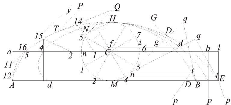
Fig.51. Costruzione di una Cicloide, orizzontale AB , e la sua altezza sotto chiave MH , dal punto C , centro di MH per centro si descriverà un cerchio MNHG , di cui si dividerà la circonferenza in altrettante parti uguali che si vorrebbero avere di punti
