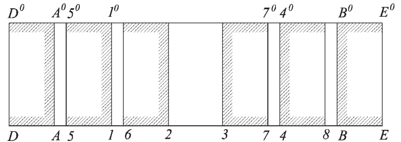
Fig. 59d Aree determinate dai giunti dei concios che compongono la Volta a Botte.
