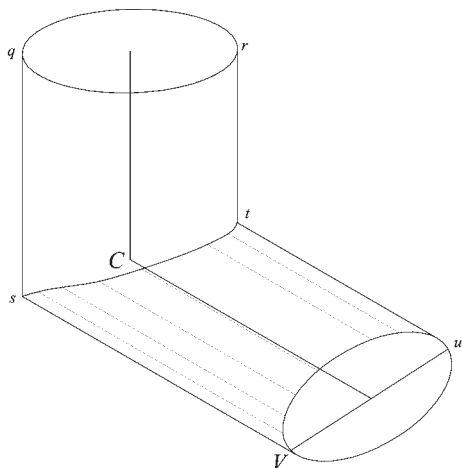
Fig. 57 Differentemente dalla figura W si ha un cilindro retto qt e uno scaleno su .
