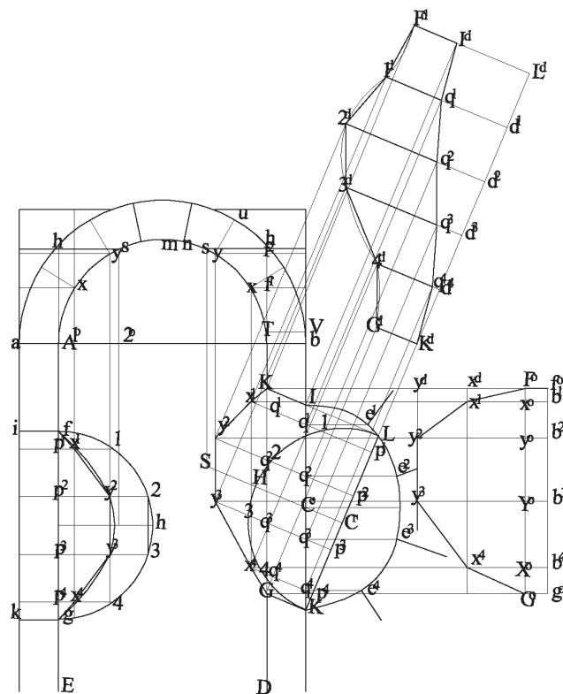
Fig. 30. 2 , 29. 2 e 30. 3 Lunette dritta e di sbieco in una volta a botte il cui piano orizzontale è BmA.
