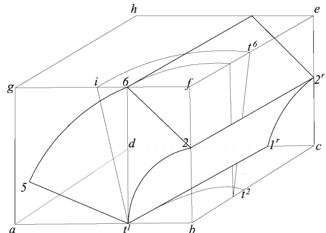
Fig.62 Costruzione del concio.
