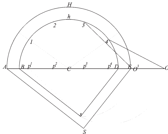
Fig. 104c: secondo metodo per cercare il valore dei giunti di letto tramite i lati degli appiombi e le lunghezze delle proiezioni.
