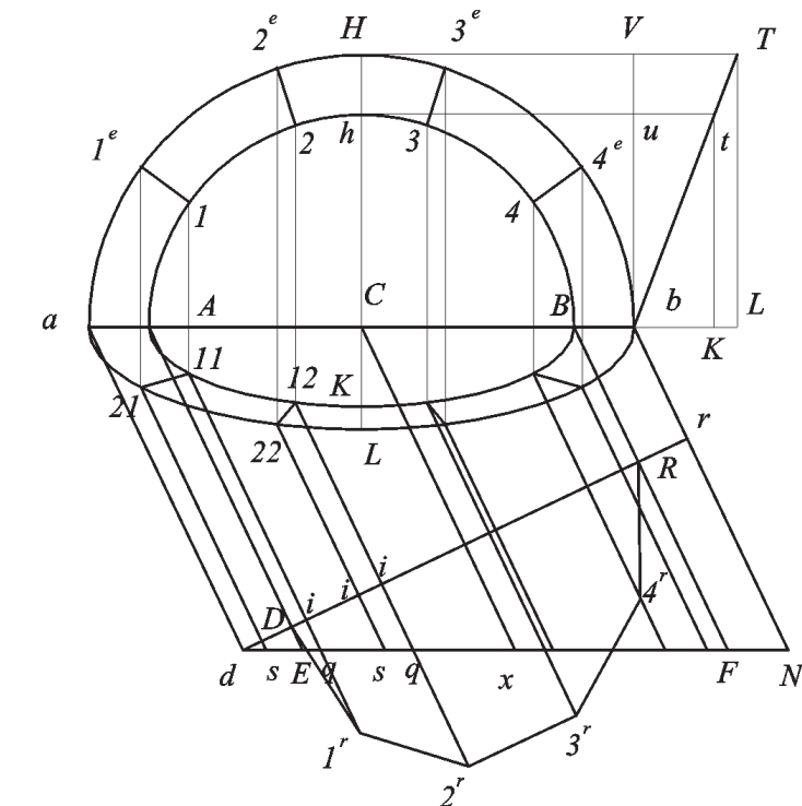
Fig. 274d Il procedimento è uguale a quello utilizzato per lo sviluppo del prisma e del cilindro.
