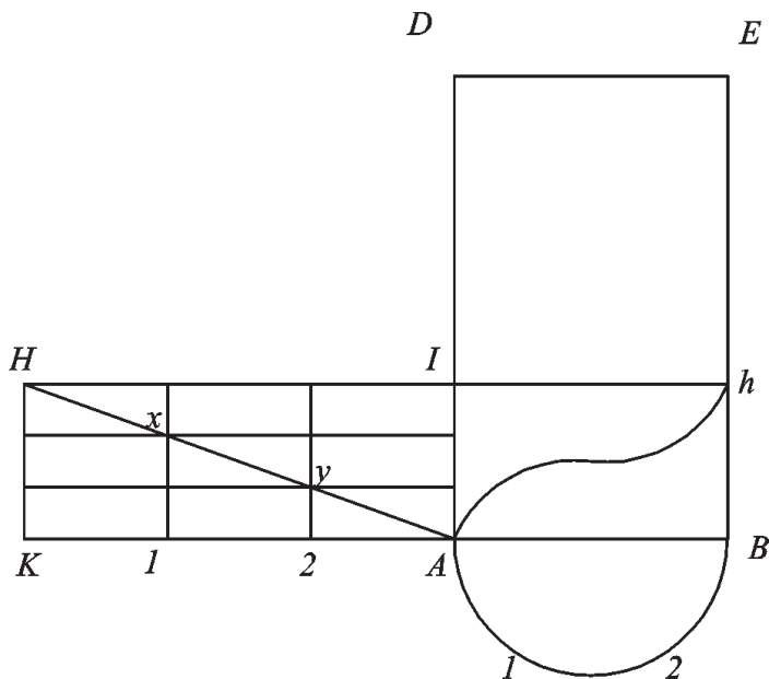
Fig. 281a Il cilindro viene suddiviso in più parti. possono diminuire o aumentare in altezza, secondo quella progressione
