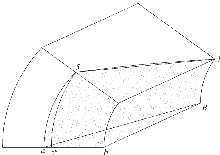
Fig. 137 Secondo questo metodo tutta la parte tratteggiata dovrà essere scolpita dal concio di pietra.
