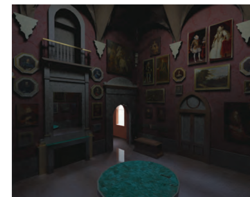
Fotografia 9 Restituzione fotorealistica dell'interno della Sala, ottenuta con simulazione transitoria di luce naturale senza schermatura per il mese di dicembre alle ore 10 - Vista sulle pareti Sud ed Est - Stato attuale.
