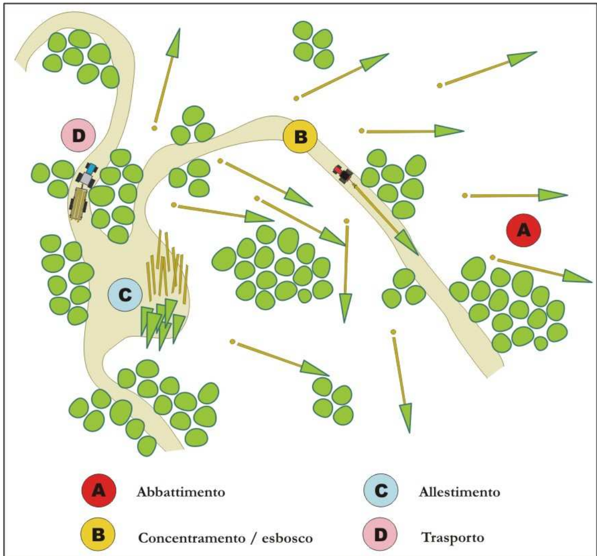
Figura 17. Rappresentazione schematica del metodo di lavoro convenzionalmente denominato “FTS” – Full Tree System.
