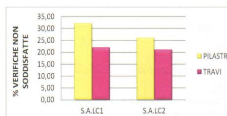
Figura 23 – Percentuali di verifiche non soddisfatte risultanti dall'analisi dinamica al passo condotta allo stato attuale
