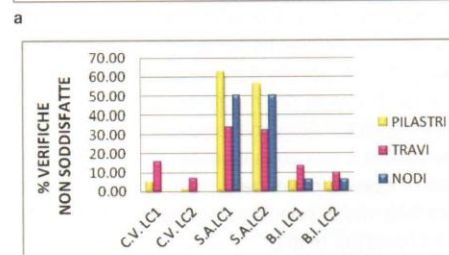
Figura 32 – Confronto dei risultati delle tre analisi, in termini generali (a) e di elementi (b)
