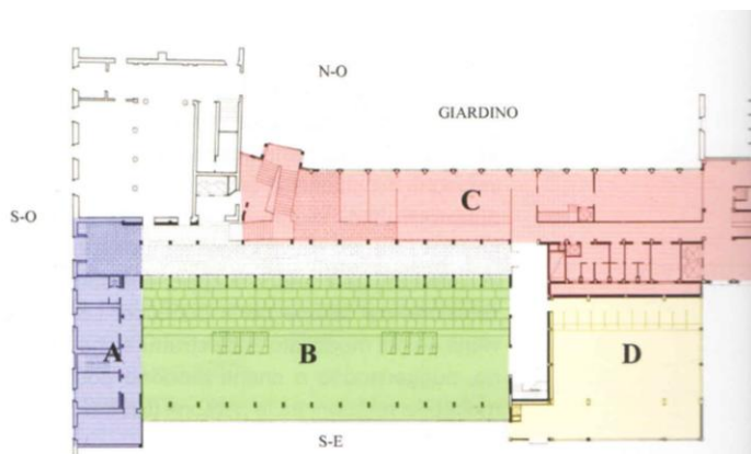
Figura 5 - Pianta del piano terra con individuazione dei differenti blocchi
