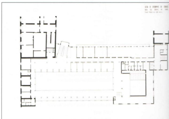
Figura 6 - Pianta del piano primo (Archivio CRF)
