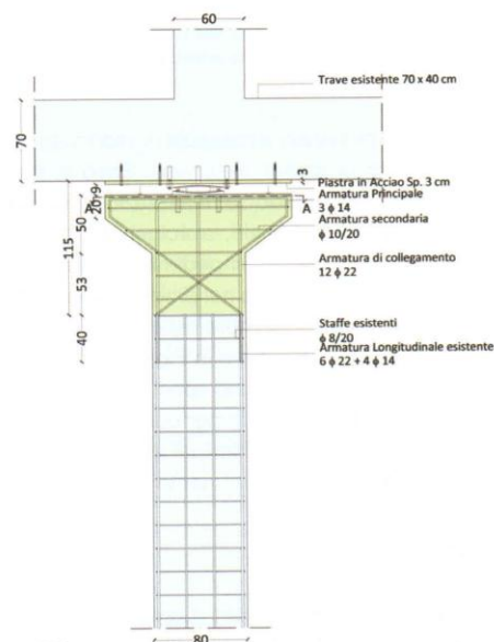
Figura 31 – Dettaglio di un baggiolo tipo
