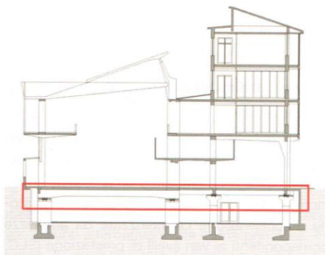
Figura 24 - Sezione trasversale dell'edificio isolato
