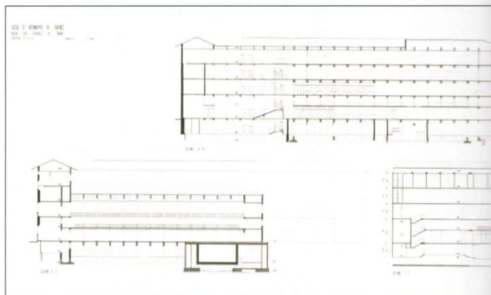
Figura 7 - Sezioni longitudinali coinvolgenti i vari blocchi (Archivio CRF)
