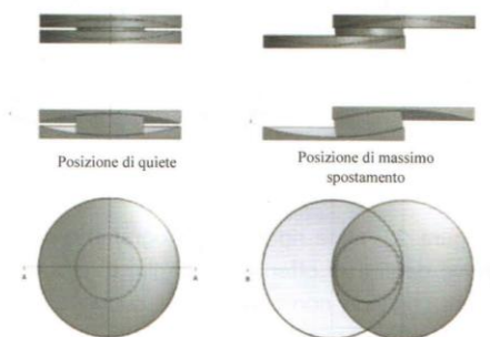
Figura 26 - Vista in prospettiva ed in pianta di un isolatore DFP nella condizione di quiete e di massimo spostamento
