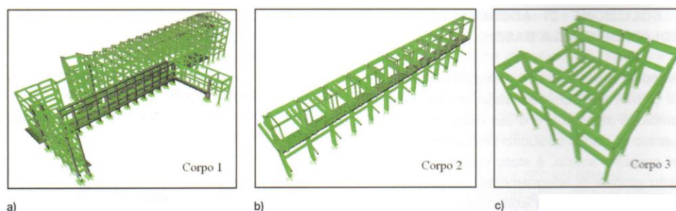
Figura 21 – Modelli agli elementi finiti relativi ai Corpi 1 (a), 2 (b), 3 (c)
