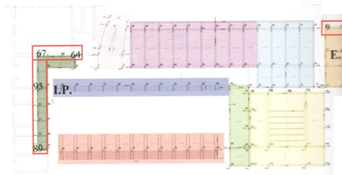
Figura 30 – Indicazione delle zone di martellamento
