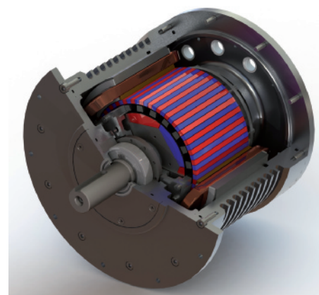
Fig. 19 – Esempio di moto-riduttore integrato (motore elettrico e riduttore magnetico radiale integrati in unica soluzione), immagine tratta da documentazione tecnica magnomatics ( www.magnomatics.com ).
