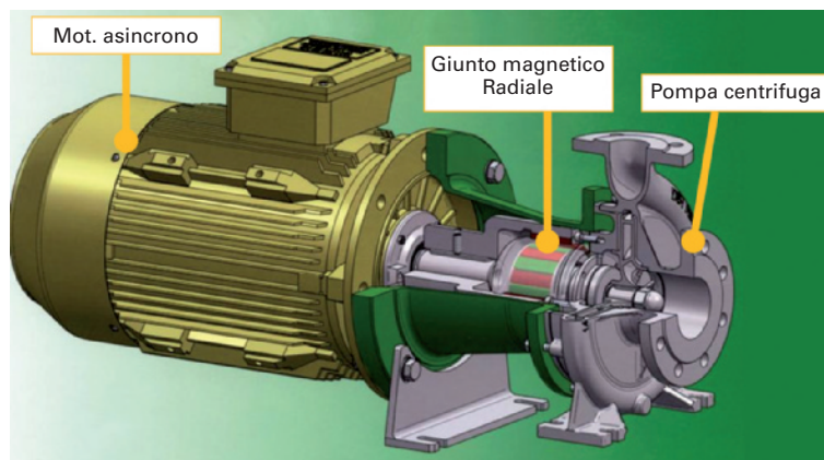
Fig. 5 - Pompa centrifuga con trasmissione magnetica radiale (tratto da doc. tecnica DST Dauermagnet-SystemTechnik GmbH).
