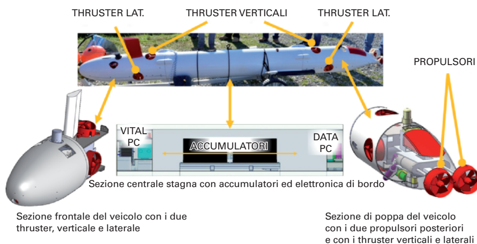
Fig. 1 – Il veicolo sottomarino Tifone e il relativo sistema di propulsione.
