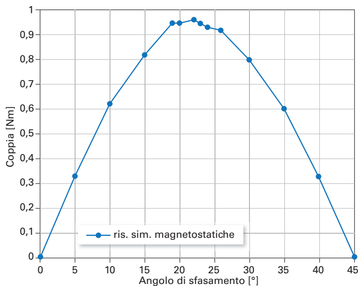
Fig. 13 – Andamento della coppia trasmessa dal giunto in funzione dello sfasamento angolare
