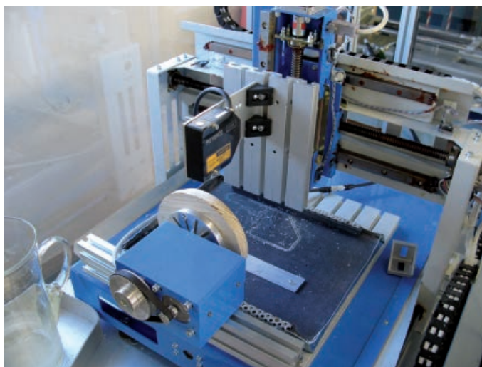
Photo 2a. Banc d'essai du test de la qualité de surface. a) Position du disque sur l'axe tournant. Photo H. Aknouche.
