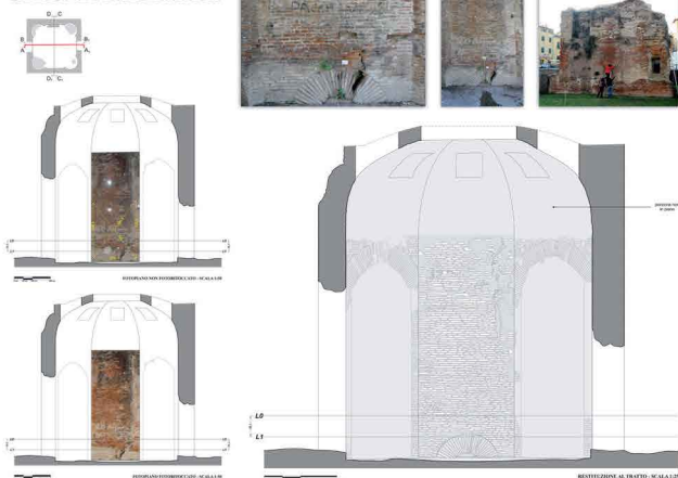
SEZIONE INTERNA A-A1
