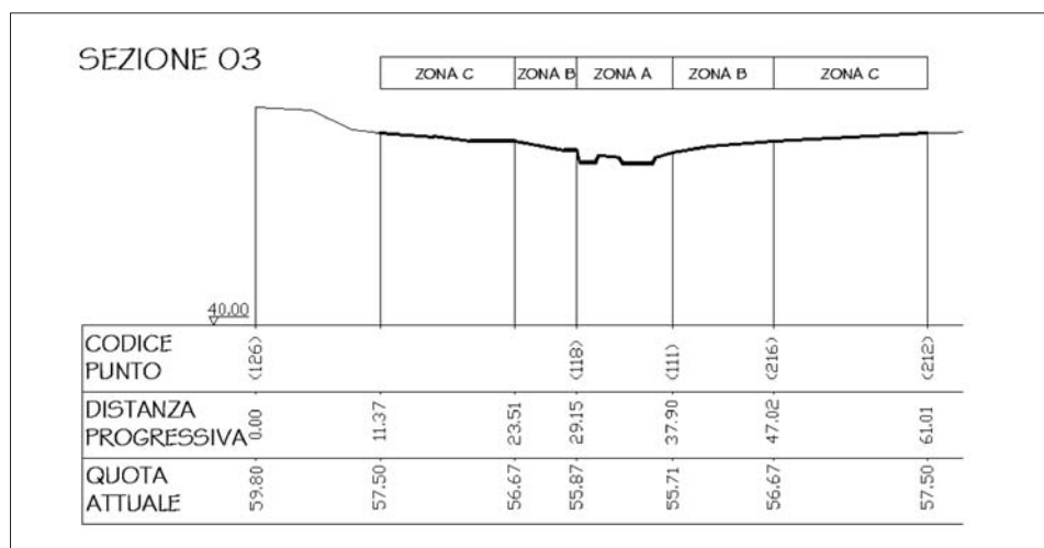
Figura 1 – Estratto esemplificativo della sezione trasversale numero 03 con sviluppo complessivo di 142,89 m, in evidenza di spessore zona A, B, C.
