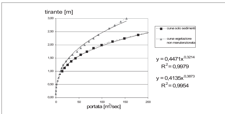
Figura 2 – Curve di deflusso con correlazione tra tiranti idrici e portate transitabili nel transect T2, confronto tra presenza di vegetazione e assenza di vegetazione (solo sedimenti) con modello Hmodel.
