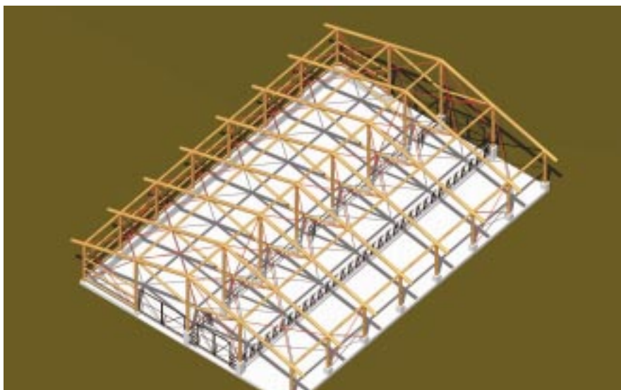
Fig. 8 - Progetto A: schema strutturale assonometrico.
