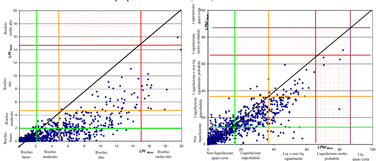
Figura 2. Confronto tra i valori dell'indice del potenziale di liquefazione LPI (a) e di probabilità di liquefazione LPbI (b) calcolati partendo dal metodo di Robertson e Wride e dal metodo di Moss.
