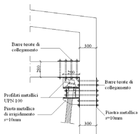
Particolare 3 Ancoraggio del cavo in sommità Scala 1:20 - Quote in mm
