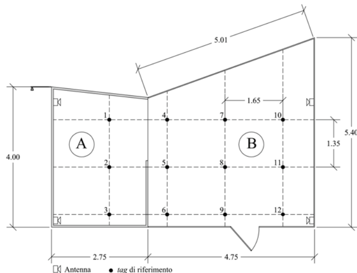
Figura 2. Schema planimetrico del box per suini e della maglia dei tag di riferimento disposti nelle due aree analizzate: A) area di riposo, B) area di esercizio. La figura mostra anche la collocazione delle quattro antenne dei nodi ricevitori.
