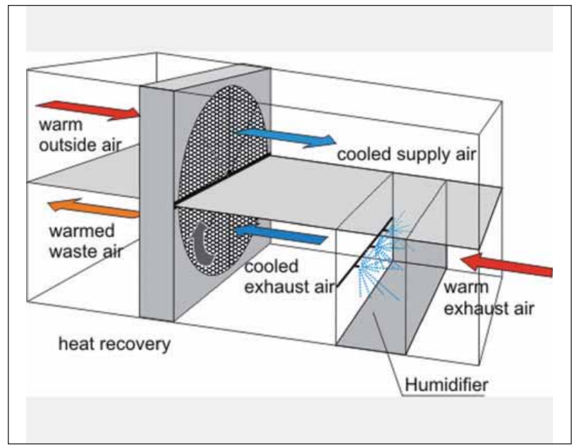
Raffrescamento ad evaporazione.
