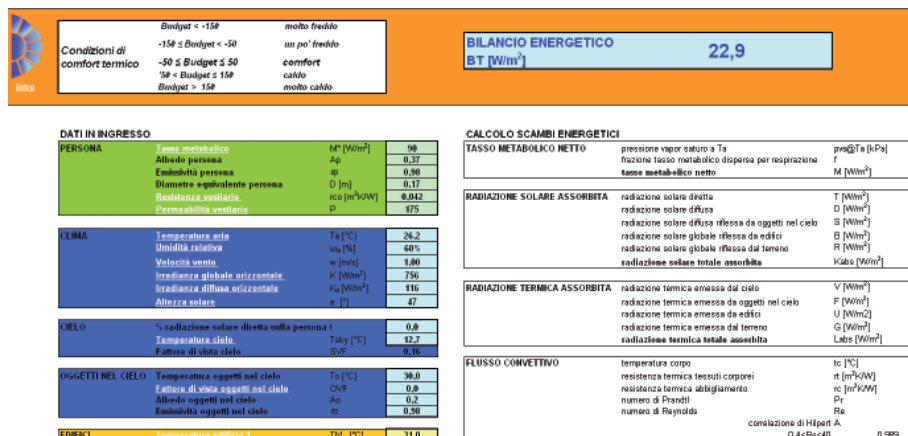
Fig. 2.27 Schermata principale con i dati di input richiesti dal foglio di calcolo Comfa+.
