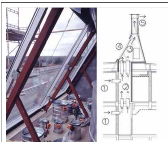
Camino solare.
