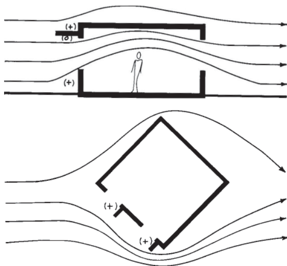
Fig. 3.44 Esempi di deviazione del flusso d'aria dovuto alla presenza degli aggetti orizzontali e verticali.
