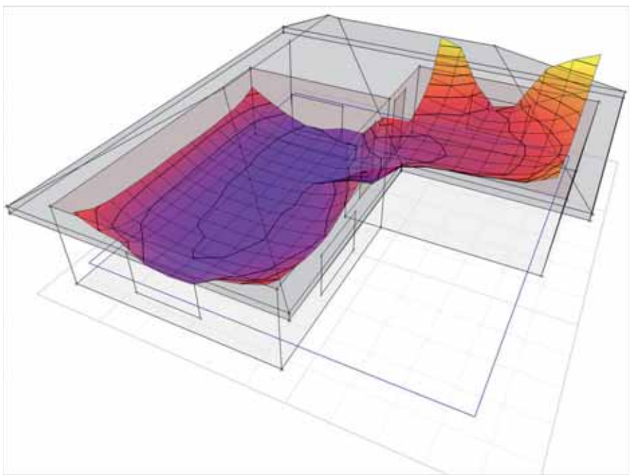
Fig. 17 Prestazioni termiche: calcolo dei carichi di riscaldamento e raffreddamento per modelli con qualsiasi numero di zone o tipo di geometria. (Fonte Autodesk).
