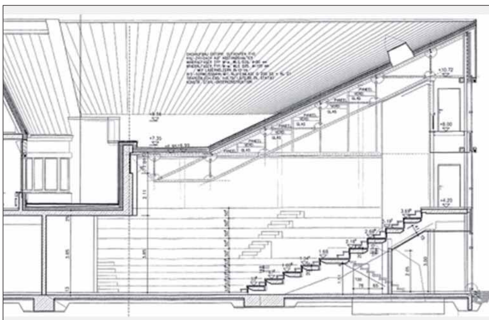
Sezione est-ovest.
