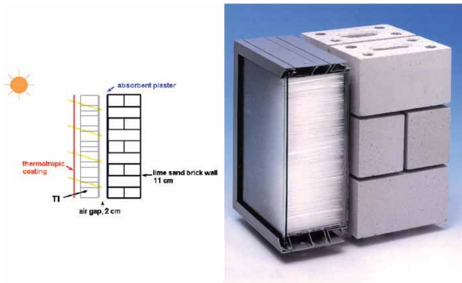
Fig. 3.26a – 3.26b Sistema traslucido TIM con elevate prestazioni di isolamento termico.
