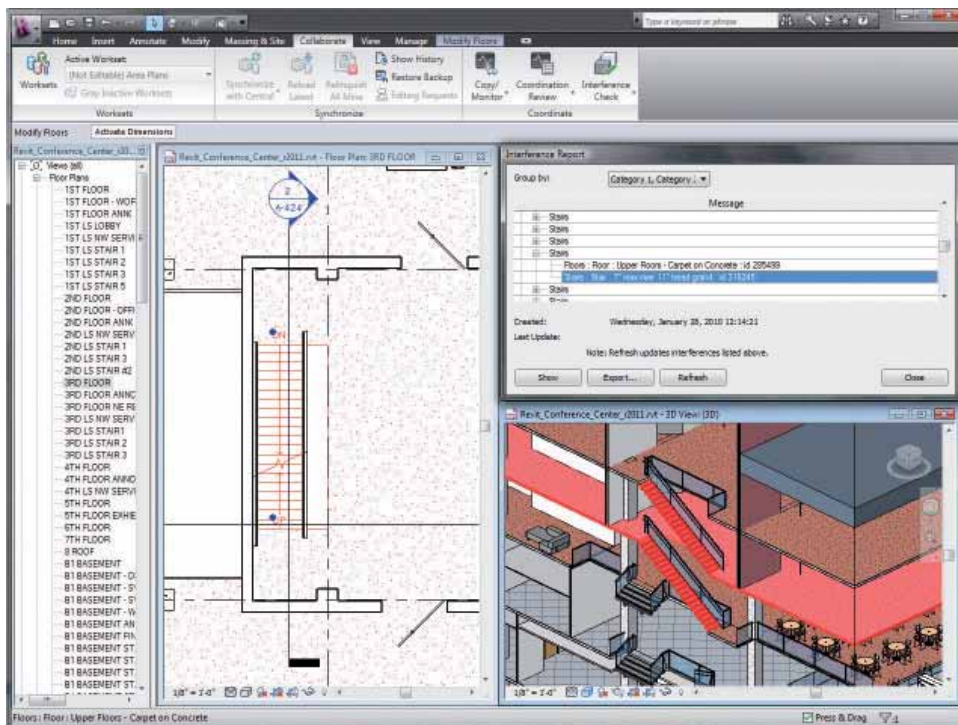
Fig. 25 Il controllo delle incongruenze progettuali è utile per rilevare nel modello eventuali anomalie tra gli elementi. (Fonte Autodesk).
