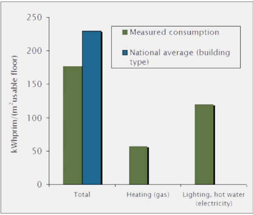
Istogramma energia primaria consumata per m 2 di superficie utile. Fonte: EULEB.
