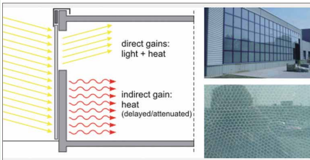
Isolamento termico trasparente – salone attrezzature.
