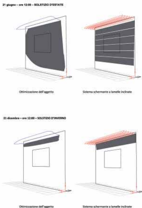
Fig. 3.33 Studi per la scelta del sistema di ombreggiatura ottimale.
