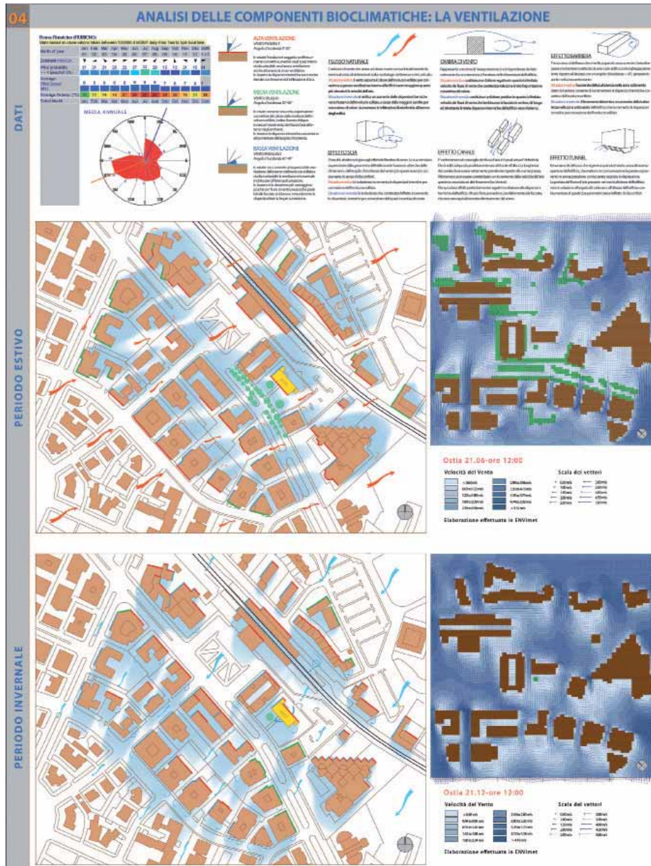
Fig. 1.10 Master di II Livello, Architettura Bioecologica e Tecnologie Sostenibili per l'Ambiente, 2007. Analisi e valutazione delle condizioni di Ventilazione (Software Envimet) nell'ambito del progetto di recupero dell'Asilo nido "Il Sagittario", Roma. Arch. Mario Piccirillo.
