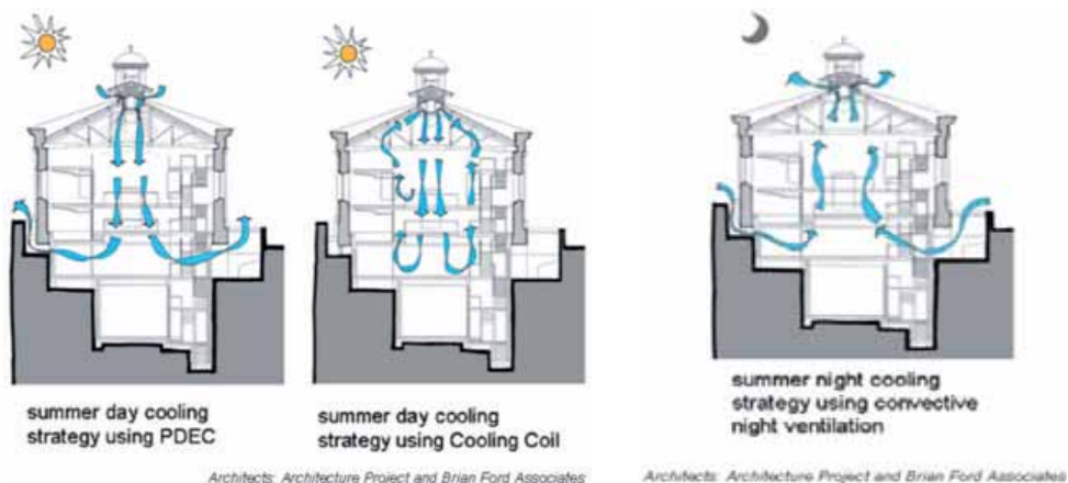
Strategia mista di raffrescamento.
