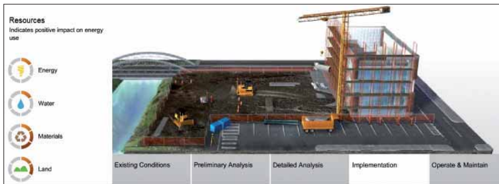
Fig. 24 Attraverso l'uso di sistemi BIM, si può valutare l'impatto ambientale sui consumi energetici della fase costruttiva. (Fonte Autodesk - http://usa.autodesk.com/ ).
