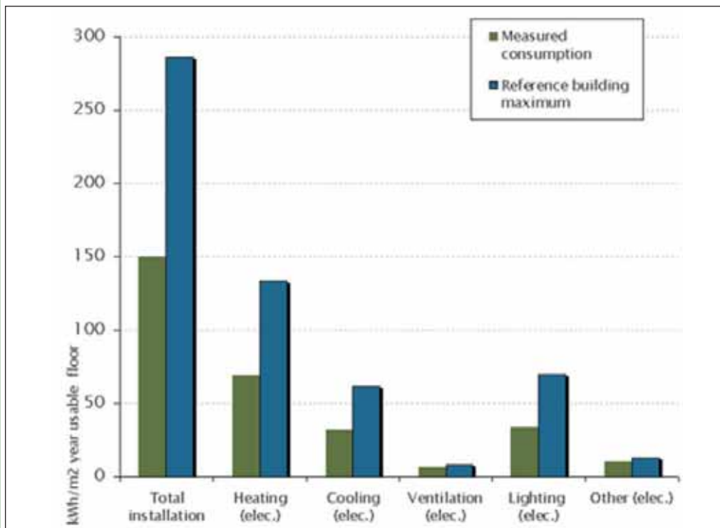
Istogramma energia primaria annuale consumata per m 2 di superficie utile. Fonte: EULEB.
