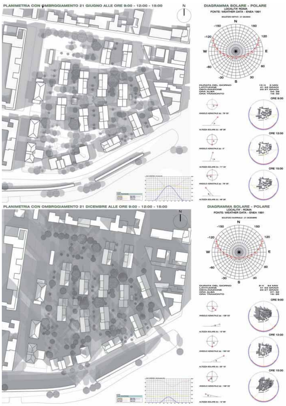
Fig. 1.11 Master di Il Livello, Architettura Bioecologica e Tecnologie sostenibili per l'Ambiente, 2008. Valutazione della dinamica del soleggiamento a livello insediativo nell'ambito del progetto di recupero del quartiere ATER "Casilino II", Roma. Arch.tti Elia Chalarambos, Angela Recchi, Silvia Vagni.
