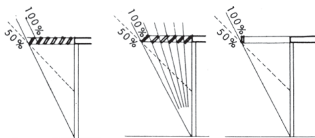
Fig. 3.34 Dimensionamento della schermatura esterna fissa.
