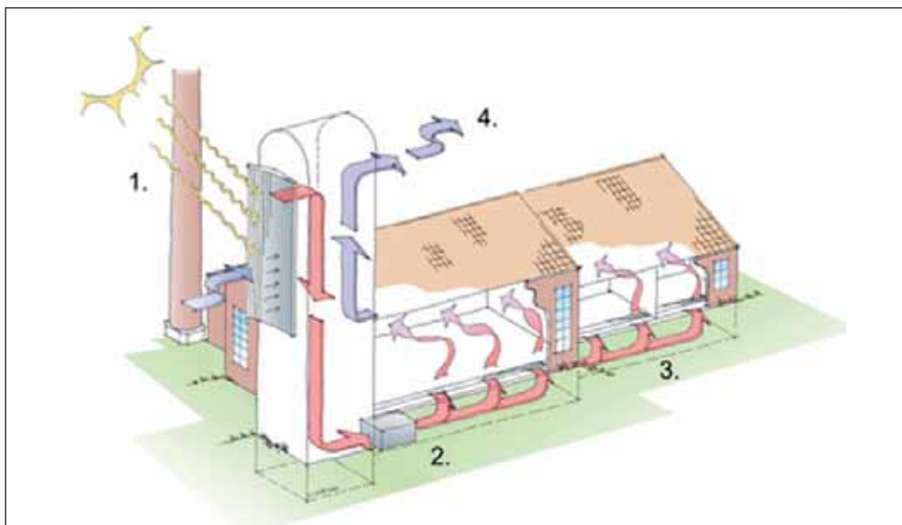
Schema ventilazione.
