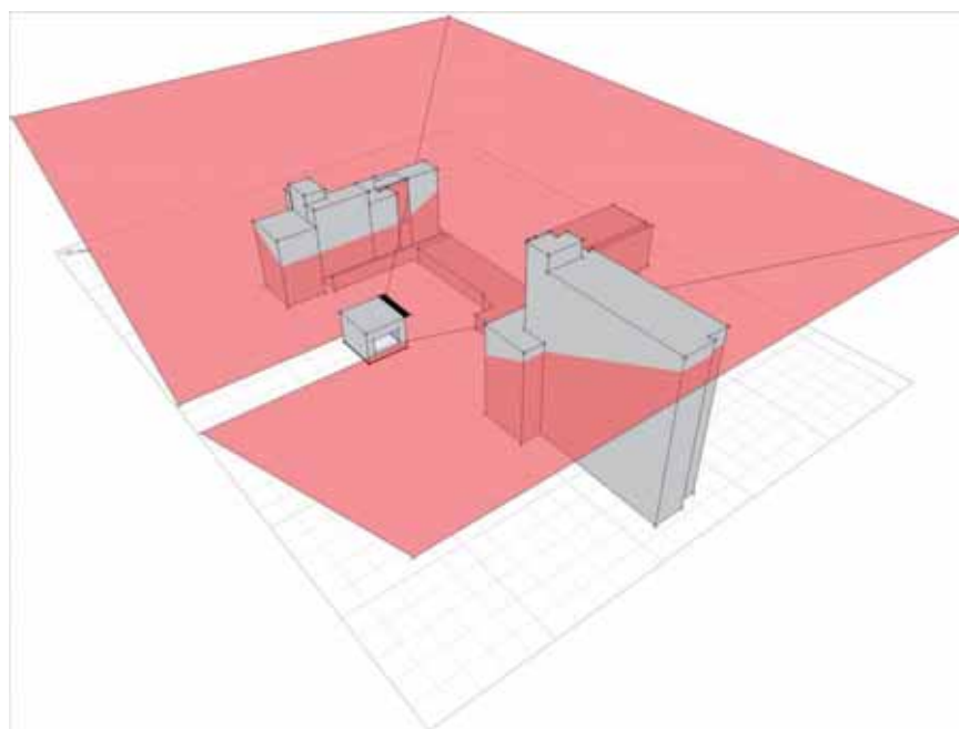
Fig. 14 Accesso alla luce: analisi degli angoli di proiezione del sito e valutazione delle ostruzioni, calcolo delle ombre. (Fonte Autodesk).
