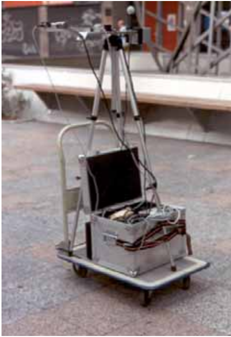
Fig. 2.23 Rilievo microclimatico di uno spazio urbano con l'utilizzo di un set di strumenti di rilievo di fattori microclimatici.
