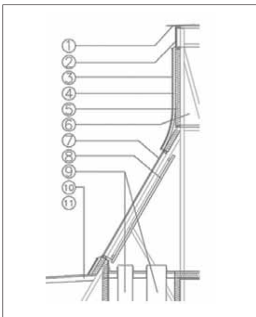
Sezione su camino solare.
