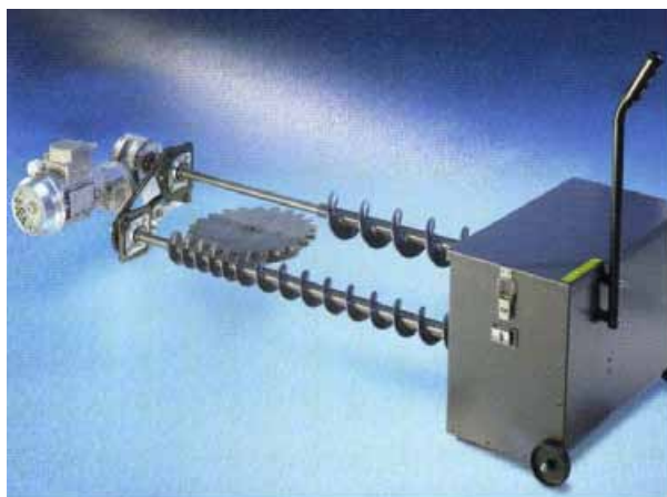
Sistema di estrazione delle ceneri
