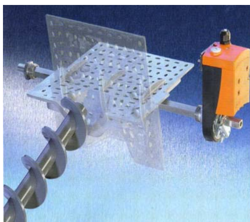
Particolare della griglia
