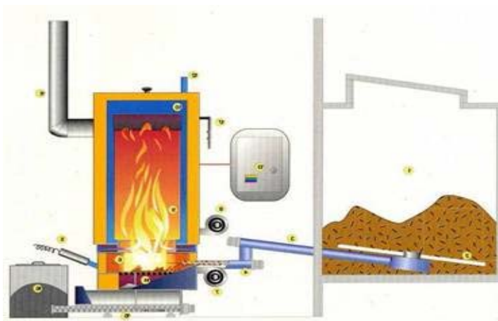
Schematizzazione del generatore di calore con sistema di trasporto del combustibile dal silo di stoccaggio.
