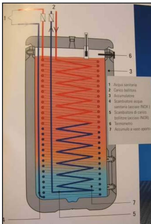
Accumulatore inerziale in sezione.
