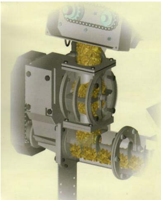
Saracinesca stellare contro il ritorno di fiamma
