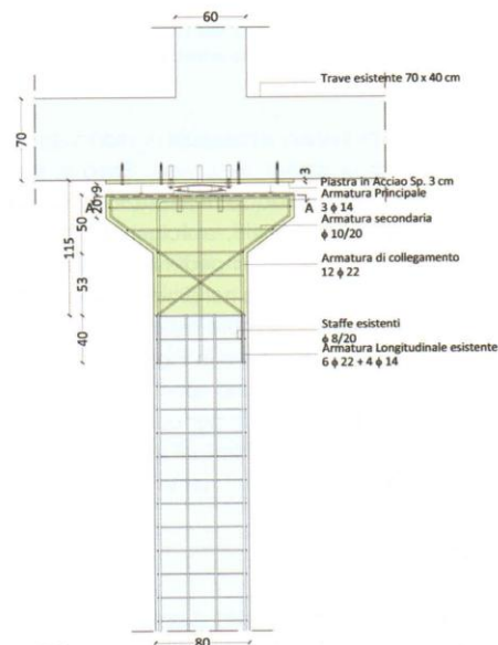
Figura 31 – Dettaglio di un baggiolo tipo
