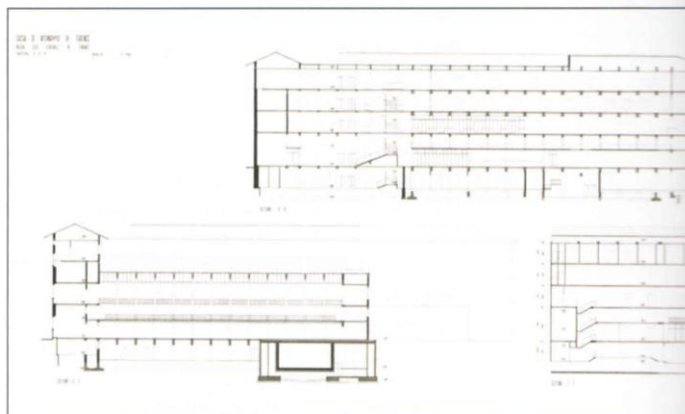
Figura 7 - Sezioni longitudinali coinvolgente i vari blocchi (Archivio CRF)
