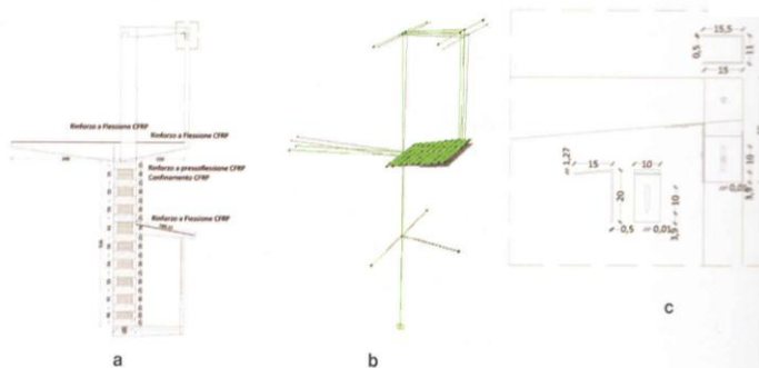
Figura 34 - a) Vista prospettica dell'intervento nel telaio lato ospedale; b) schema deformativo telaio lato ospedale; c) dettaglio costruttivo del giunto elastico
