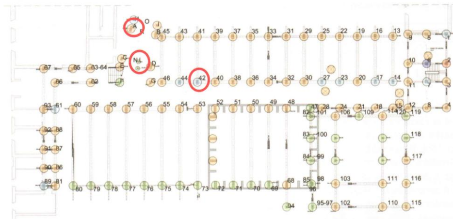
Figura 28 - Disposizione in pianta degli isolatori
