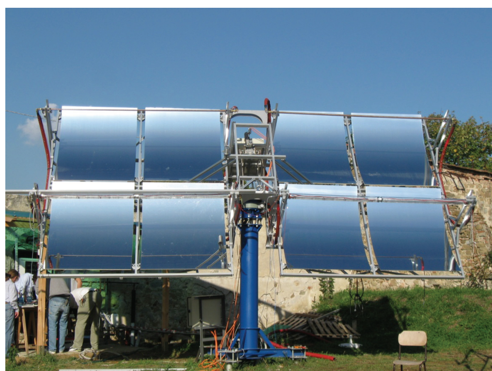
Fig. 1: The Cesare System
