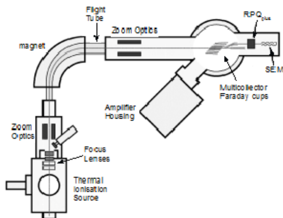
Figura 2.8 - Schema della Spettrometro di massa ThermoFischer.
