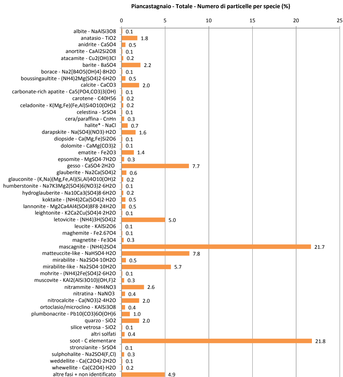
Figura 3.28 - Istogramma della concentrazione relativa delle fasi, calcolata sul numero di particelle individuate, espresso come percentuale, sul totale dei giorni di campionamento analizzati per Piancastagnaio.
