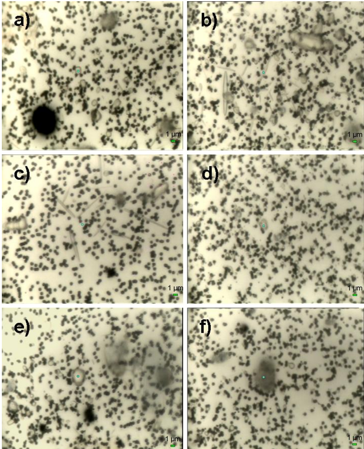
Figura A.4 - Immagini acquisite con il microscopio ottico (1000 \times ) in cui è visibile la morfologia delle particelle delle fasi più comuni: a) cristalli di forma rettangolare e arrotondata di mascagnite, b) cristalli aciculari di letovicite, c) cristalli aciculari di matteuccite-like, d) cristallo anedrale di gesso, e) cristallo di forma arrotondata di nitrammite, f) particella di soot. Gli spot neri di forma circolare sono i pori di 0.8 \mu\text{m} di diametro nel policarbonato.
