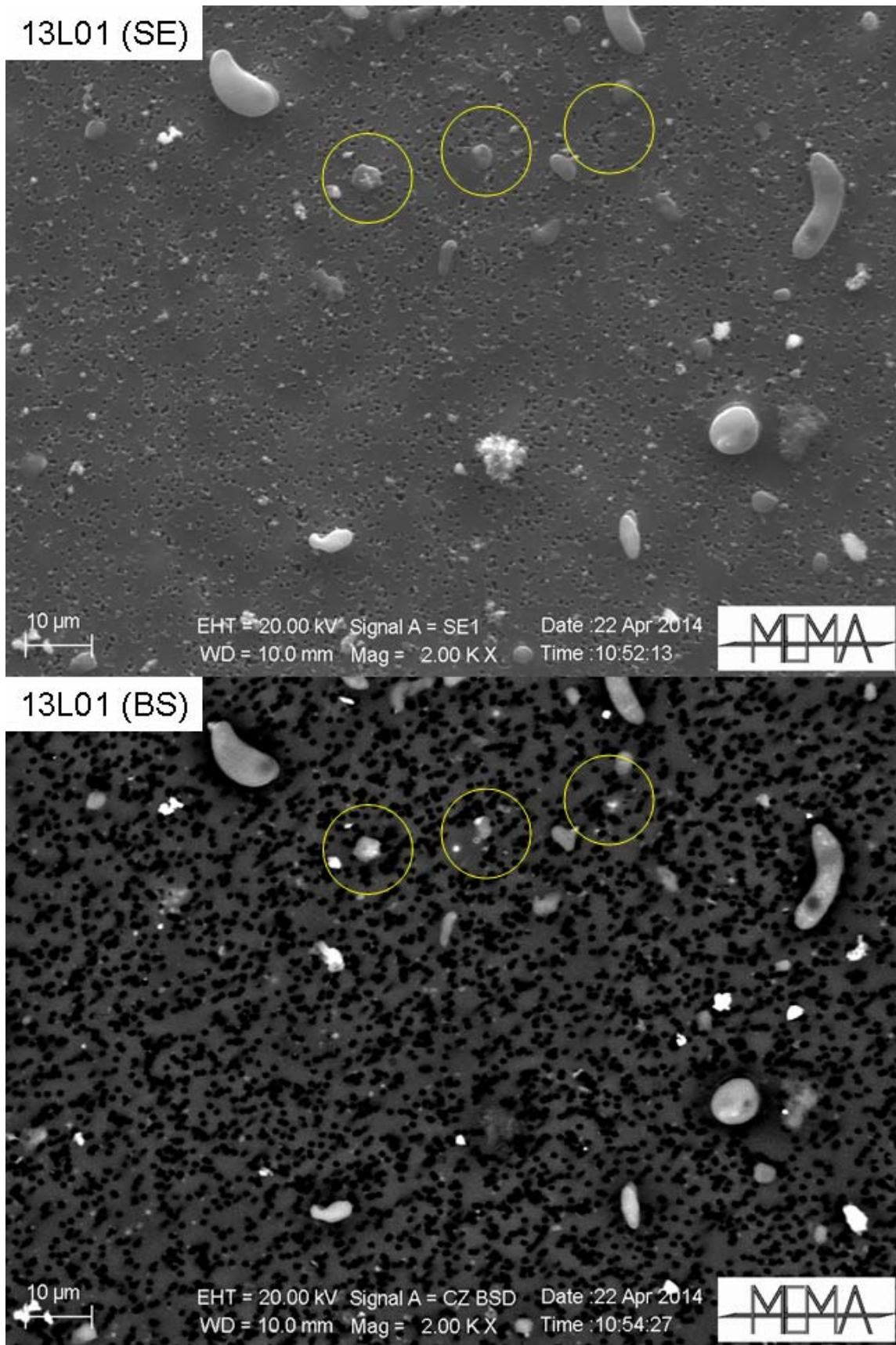
Figura A.8 - Immagine di un'area del filtro 13L01 in elettroni secondari (SE) e primari (BS) a confronto. Le particelle evidenziate mostrano zone a differente contrasto di grigio in elettroni primari che significa presenza di zone di diversa natura chimica.
