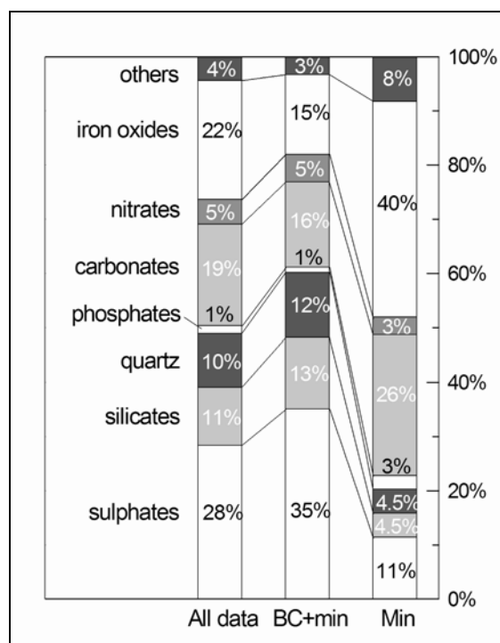
Figura 4.6 - Percentuali di particelle appartenenti alle fasi rilevate nella città di Roma (Catelani et al. 2014). All data = dati cumulativi; BC+min = black carbon + minerali; Min = particelle di minerali.
