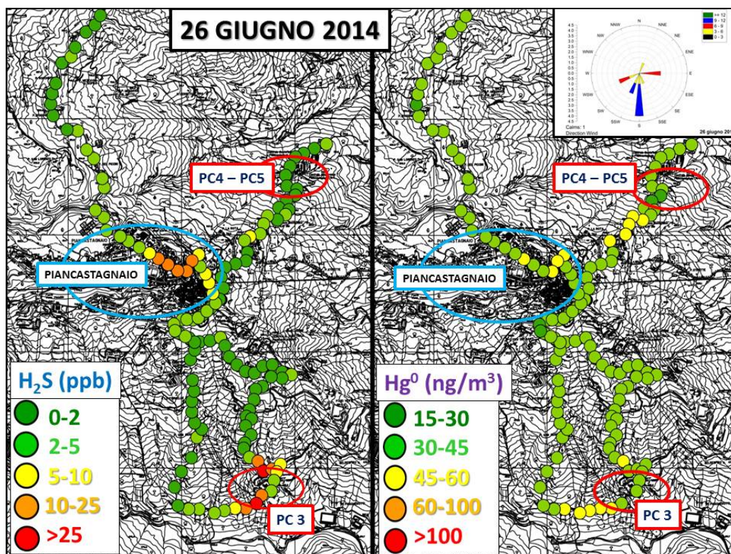
Figura 3.15 - Distribuzione delle concentrazioni di H 2 S (parte sinistra) e Hg 0 (parte destra) lungo il percorso prestabilito nel giorno 26 giugno 2014. In alto a destra è riportata la rosa dei venti, ottenuta con le media giornaliera dei dati acquisiti. Le zone cerchiare rappresentano: a) abitato di Piancastagnaio (cerchio azzurro); b) centrali geotermoelettriche (cerchi rossi).
