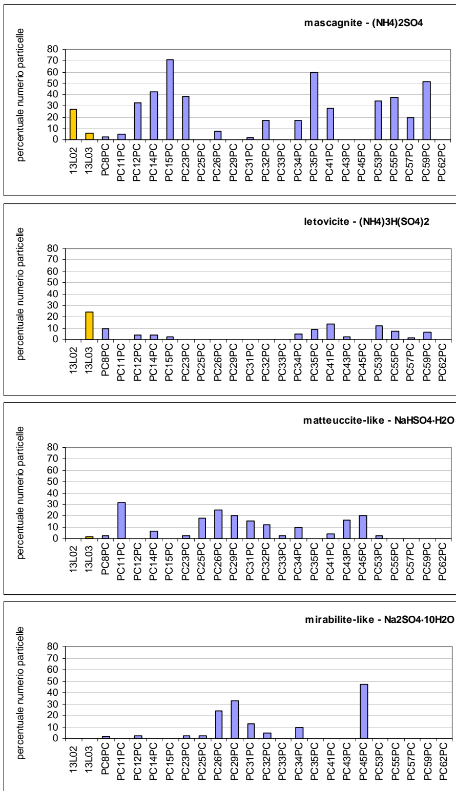
Figura 3.31 - Concentrazione relativa (in %) dei minerali del gruppo dei solfati maggiormente abbondanti nel PM10 raccolto a Piancastagnaio per i campioni analizzati, espressa come percentuale sul numero di particelle. Gli istogrammi mostrano lo stesso intervallo nella scala verticale. In arancio i campioni raccolti nel sito urbano di Piancastagnaio. Il campione PC26PC è stato raccolto a Gallina.
