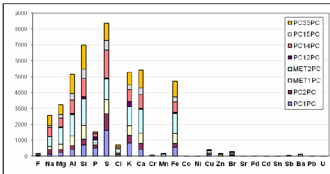
Figura 3.34 - Numero cumulativo delle particelle che contengono gli elementi rilevati per i giorni di campionamento analizzati (Piancastagnaio).
