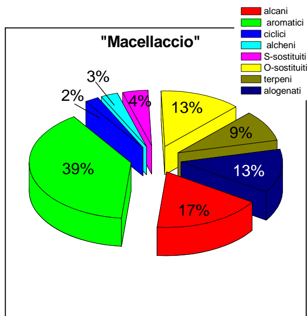
Figura 3.10 - Distribuzione in % delle famiglie di COV in aria nei campioni di Piancastagnaio "Stazione Macellaccio" (M)
