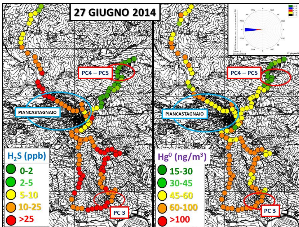
Figura 3.18 - Distribuzione delle concentrazioni di H_2S (parte sinistra) e Hg^0 (parte destra) lungo il percorso prestabilito nel giorno 27 giugno 2014. In alto a destra è riportata la rosa dei venti, ottenuta con le media giornaliera dei dati acquisiti. Le zone cerchiare rappresentano: a) abitato di Piancastagnaio (cerchio azzurro); b) centrali geotermoelettriche (cerchi rossi).
