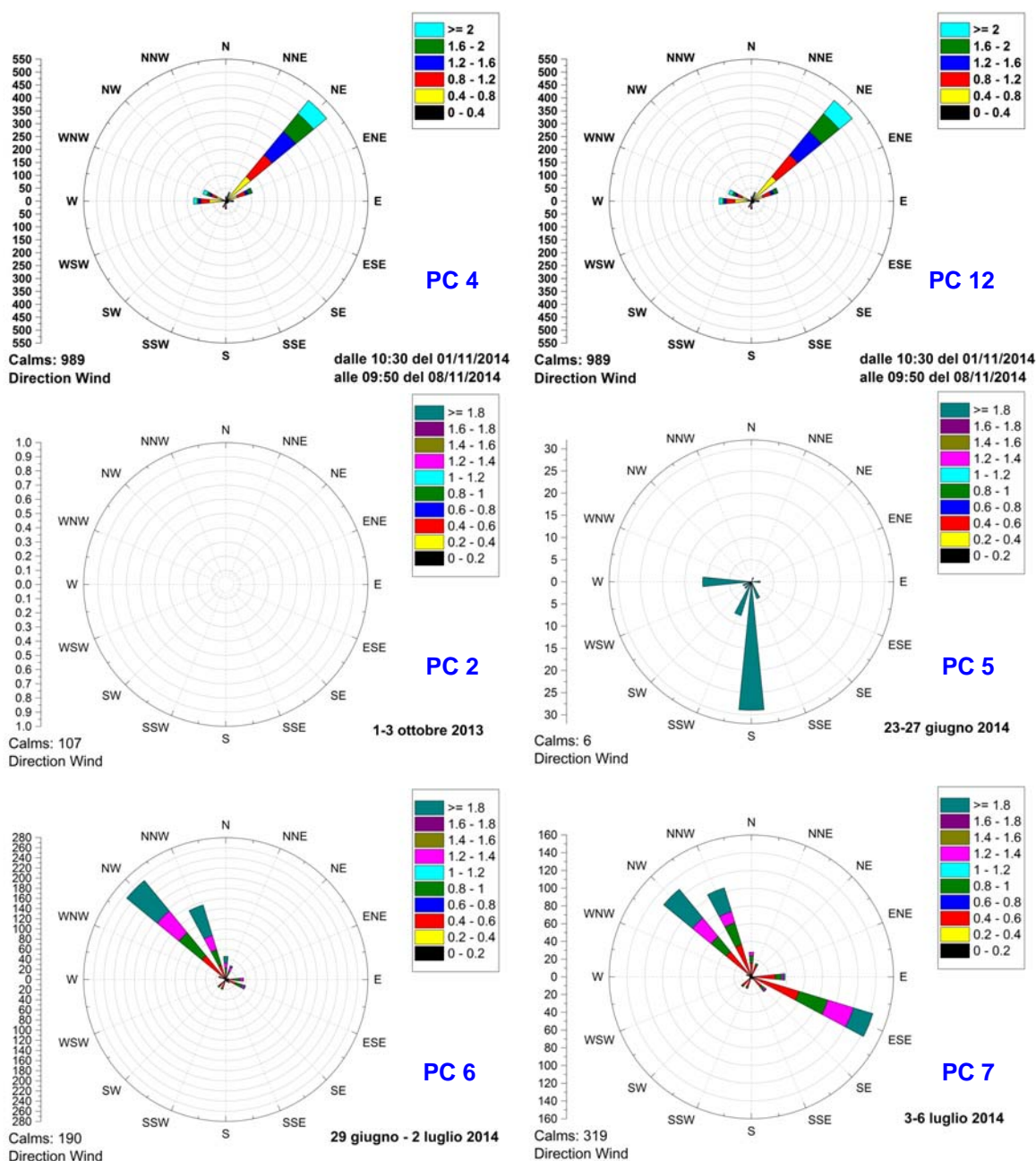
Figura 3.8 - Direzione media dei venti in alcune settimane di campionamento con indicati i rispettivi campioni di PM10 analizzati.
