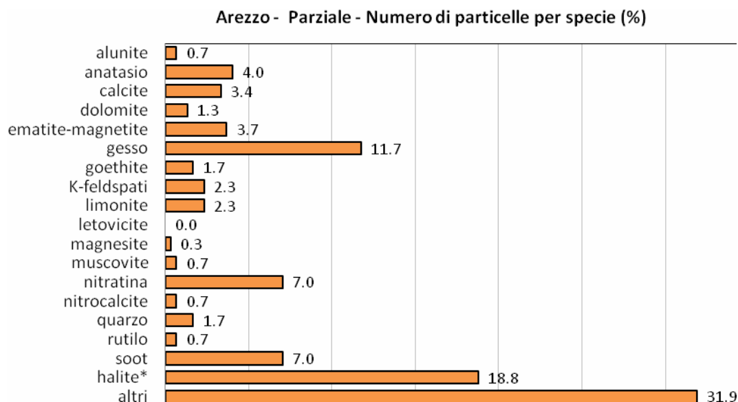
Figura 3.37 - Istogramma della concentrazione relativa delle fasi, calcolata sul numero di particelle individuate, espresso come percentuale, sul totale dei campioni PC-AR12, PC-AR13 e PC-AR14.
