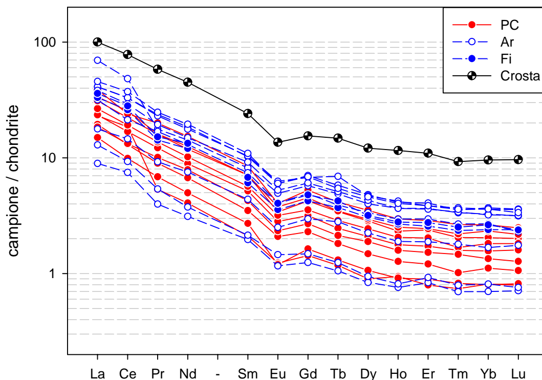
Figura 3.4 - Pattern Terre Rare dei campioni di PM10 di Piancastagnaio, Arezzo e Firenze e della Crosta Superiore (Rudnick & Gao, 2003).
