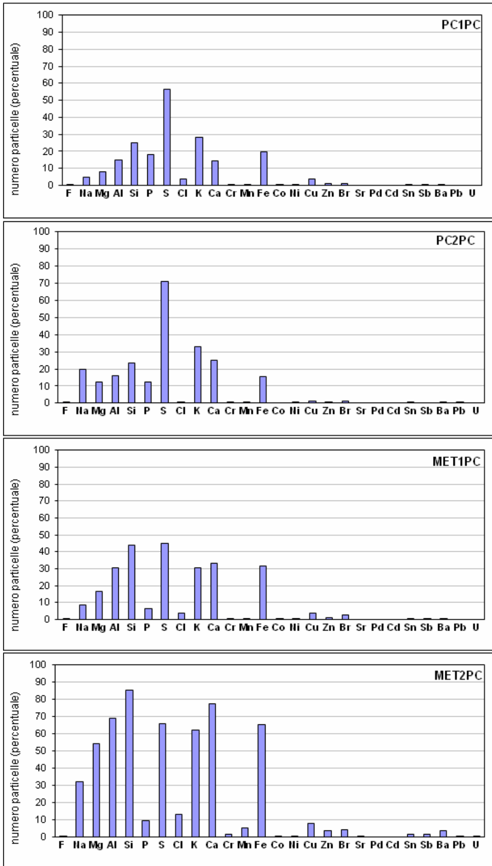
Figura A.5 - Frequenza di particelle contenenti gli elementi chimici rilevati, espressa come percentuale in numero, per ogni campione analizzato.
