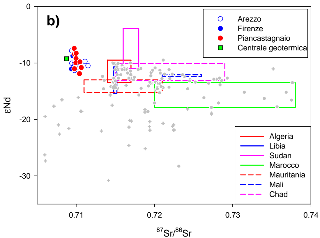
Figura 3.5 – (a) Mappa schematica delle composizioni isotopiche di Sr e Nd delle potenziali sorgenti di aerosol dell’Africa centro settentrionale. (b) Rapporti isotopici di Sr e Nd nei campioni di PM10 di Piancastagnaio, Arezzo e Firenze, nonché nel fluido geotermico della centrale PC5. I campi riportano la variazione isotopica di vari campioni di aerosol provenienti dalla regione Africana; i cerchi grigi rappresentano campioni di sedimenti e aerosol di provenienza africana, mentre le croci grigie rappresentano le composizioni isotopiche estreme di rocce Archeane della Mauritania e del Senegal (database da: Boher et al., 1992; Grousset et al., 1998; Grousset & Biscaye 2005; Pawlig et al., 2006; Abouchami et al., 2013; Scheuven et al., 2013; Kumar et al., 2014).
