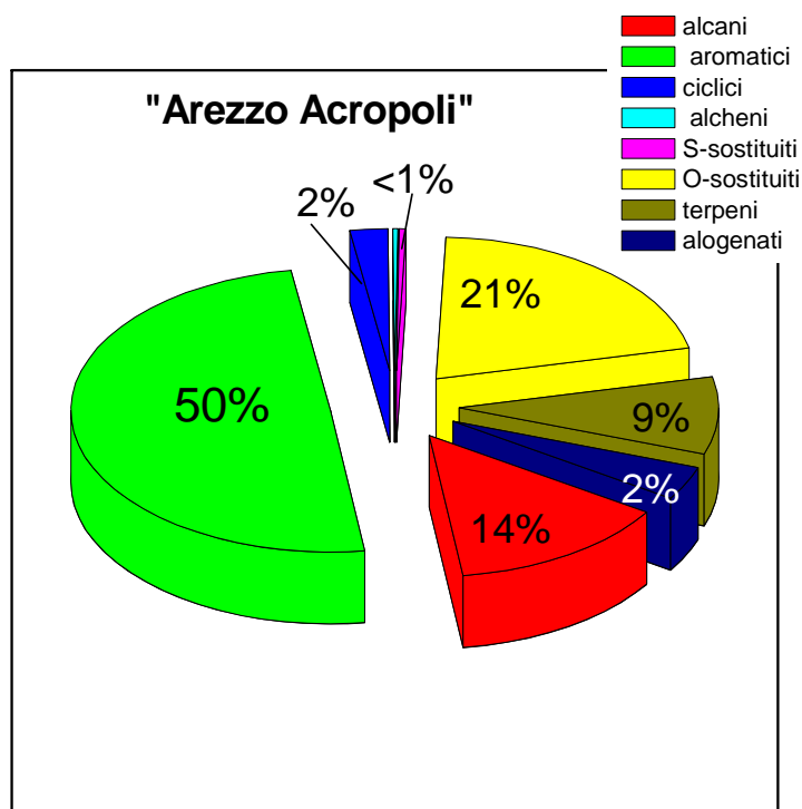
Figura 3.12 - Distribuzione in % delle famiglie di COV in aria nei campioni di Arezzo "Acropoli" (AR)
