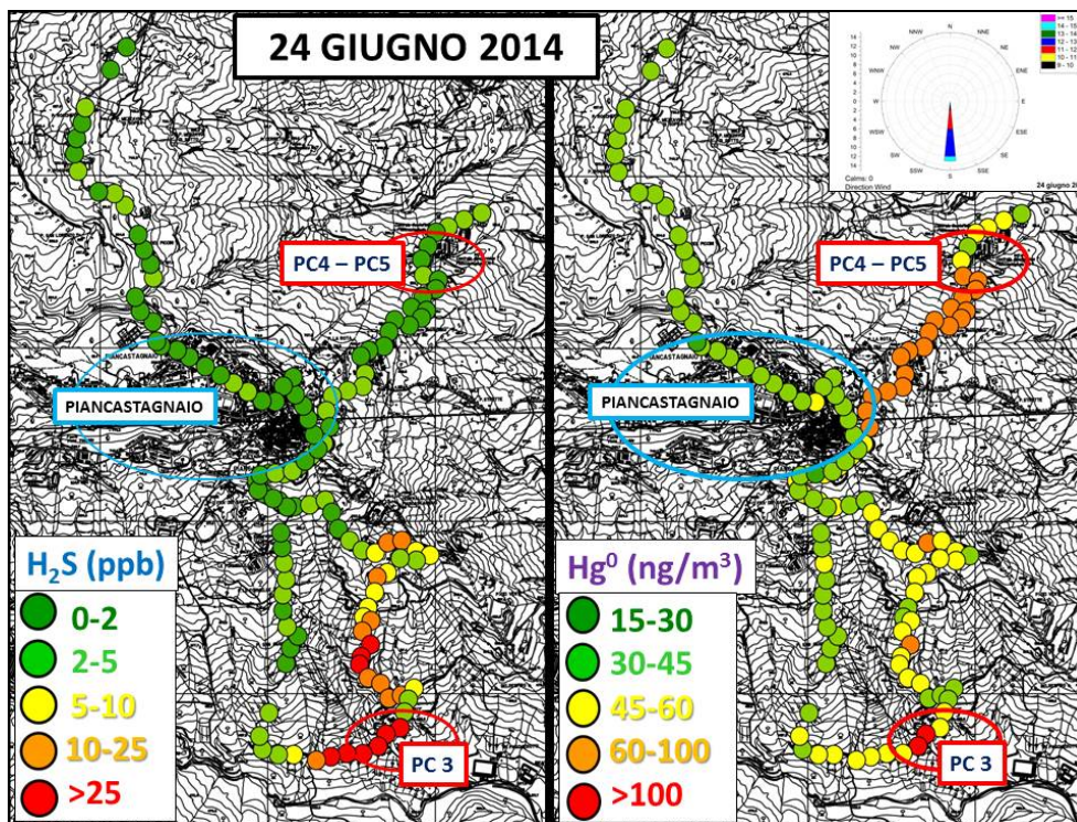
Figura 3.13 - Distribuzione delle concentrazioni di H_2S (parte sinistra) e Hg^0 (parte destra) lungo il percorso prestabilito nel giorno 24 giugno 2014. In alto a destra è riportata la rosa dei venti, ottenuta con le media giornaliera dei dati acquisiti. Le zone cerchiata rappresentano: a) abitato di Piancastagnaio (cerchio azzurro); b) centrali geotermoelettriche (cerchi rossi).
