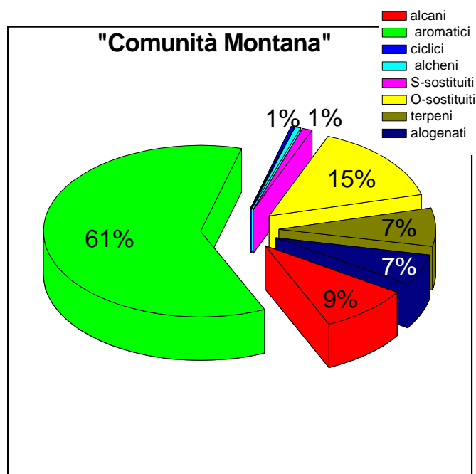
Figura 3.11 - Distribuzione in % delle famiglie di COV in aria nei campioni di Piancastagnaio "Comunità Montana" (CM)
