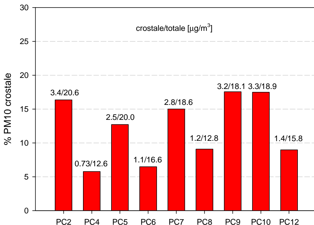
Fig. 3.2 – Contributo crostale nel PM10 di Piancastagnaio.
