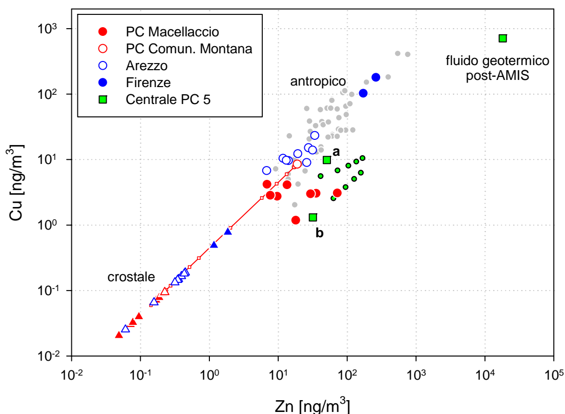
Figura 4.1 - Concentrazioni di Zn versus Cu nei campioni di PM10 di Piancastagnaio, Arezzo e Firenze. Sono riportate anche le concentrazioni del fluido geotermico post-AMIS, a più alta concentrazione di Zn e Cu, e quelle del fluido geotermico diluito (a e b) unitamente a quelle di una serie di fluidi geotermici autodiluiti (rombi rossi e verdi) e ad una linea di mescolamento tra la sorgente antropica e quella crostale (vedi testo per ulteriori spiegazioni). Il database dei campioni di aerosol europeo (cerchi grigi) è come in Fig. 3.7.
