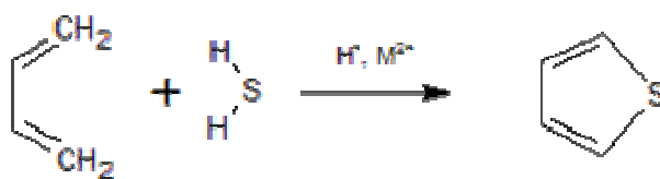
Figura 4.3 - Sintesi del C 4 H 4 S dal butadiene
