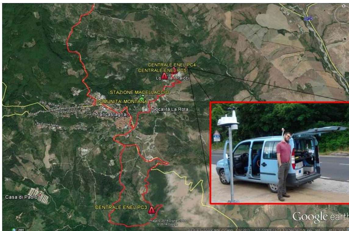
Figura 2.15 - misurazioni simultanee H_2S , SO_2 ed Hg^0 , con posizionamento GPS e acquisizione dati meteo.
