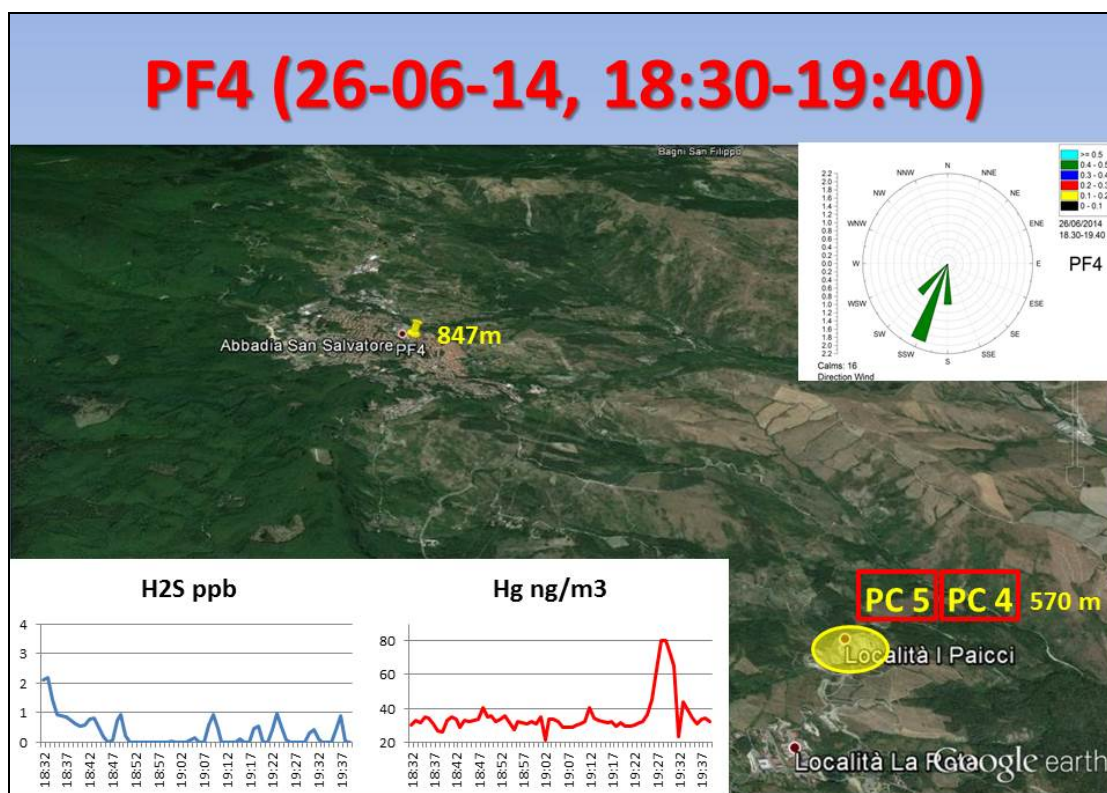
Figura 3.17 - Ubicazione e quota del punto fisso PF4 rispetto alle centrali geotermoelettriche con relativi andamenti delle concentrazioni di H 2 S e Hg 0 rispetto al tempo. In alto a destra la rosa dei venti relativa alle due ore di misura.
