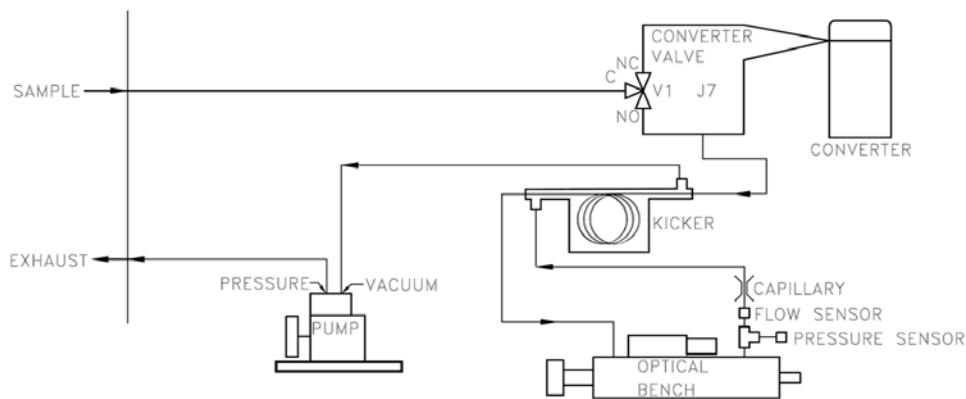
Figura 2.13 - Rappresentazione schematica del THERMO 450i.
