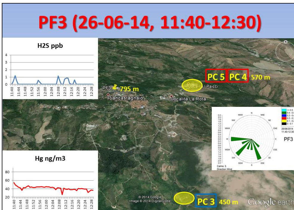
Figura 3.16 - Ubicazione e quota del punto fisso PF3 rispetto alle centrali geotermoelettriche con relativi andamenti delle concentrazioni di H 2 S e Hg 0 rispetto al tempo. In alto a destra la rosa dei venti relativa alle due ore di misura.
