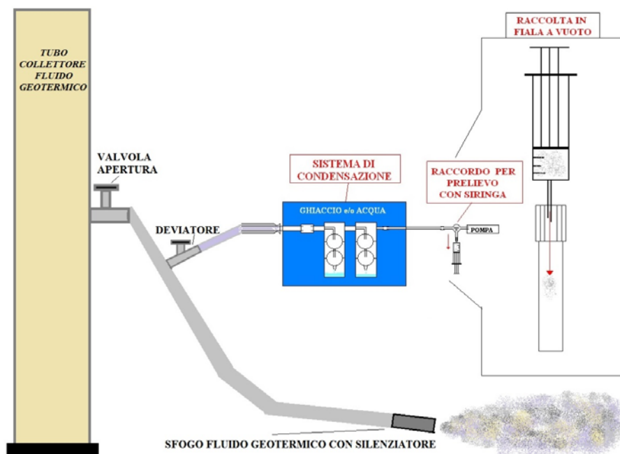
Figura 2.16 - Schema del sistema di condensazione per il prelievo del fluido geotermico dal collettore.
