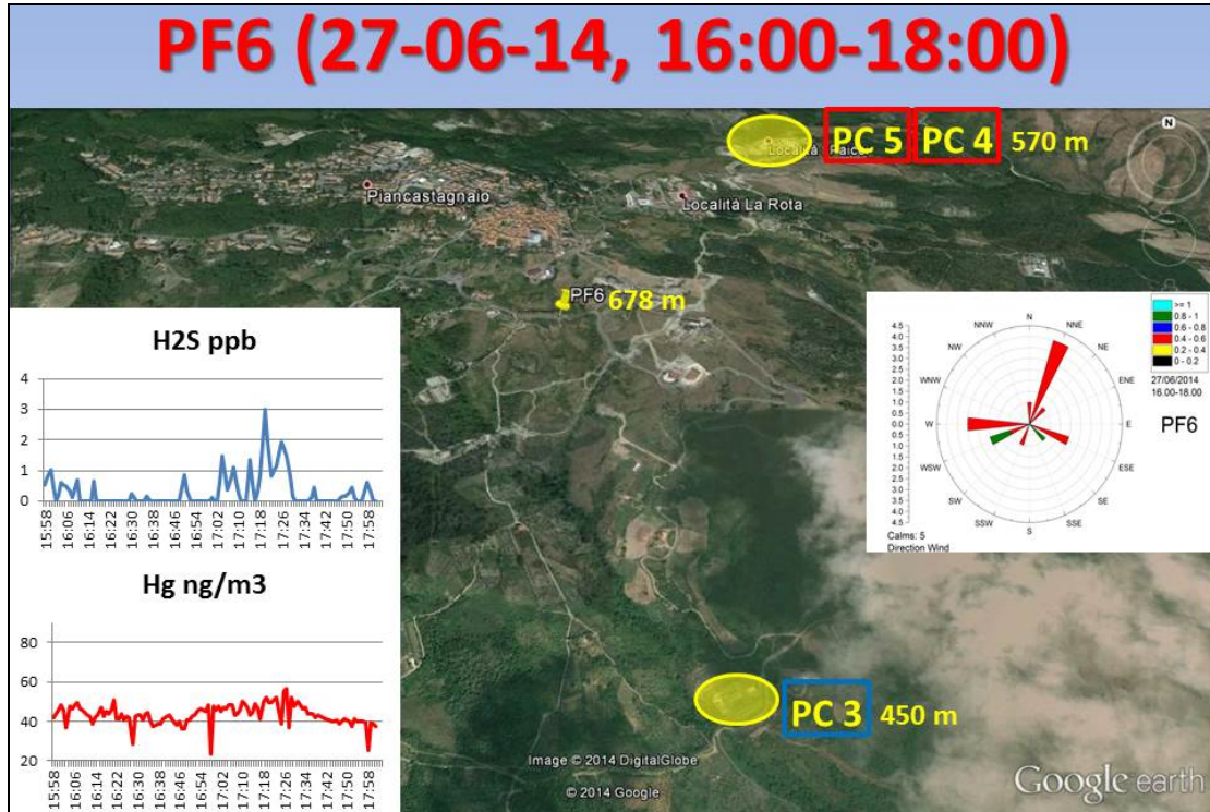
Figura 3.20 - Ubicazione e quota del punto fisso PF6 rispetto alle centrali geotermoelettriche con relativi andamenti delle concentrazioni di H_2S e Hg^0 rispetto al tempo. In alto a destra la rosa dei venti relativa alle due ore di misura.
