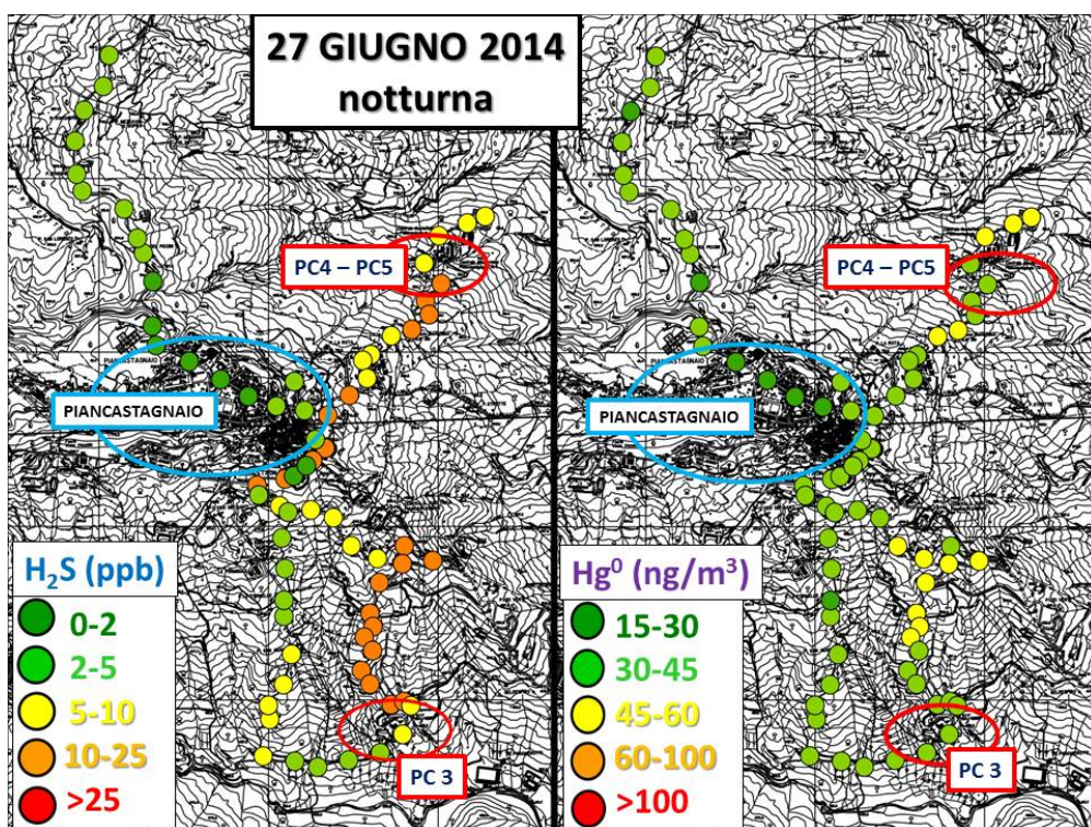
Figura 3.21 - Distribuzione delle concentrazioni di H_2S (parte sinistra) e Hg^0 (parte destra) lungo il percorso prestabilito nella notte tra il 27 ed il 28 giugno 2014. Le zone cerchiato rappresentano: a) abitato di Piancastagnaio (cerchio azzurro); b) centrali geotermoelettriche (cerchi rossi).
