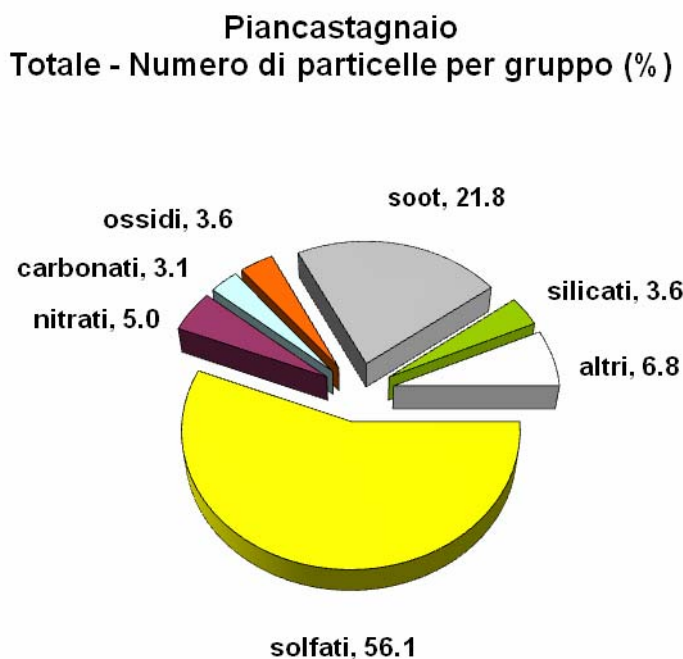
Figura 3.29 - Concentrazione relativa dei principali gruppi di minerali, e altre fasi, che compongono il PM10 raccolto a Piancastagnaio, espressa come percentuale sul numero di particelle, del totale analizzato.
