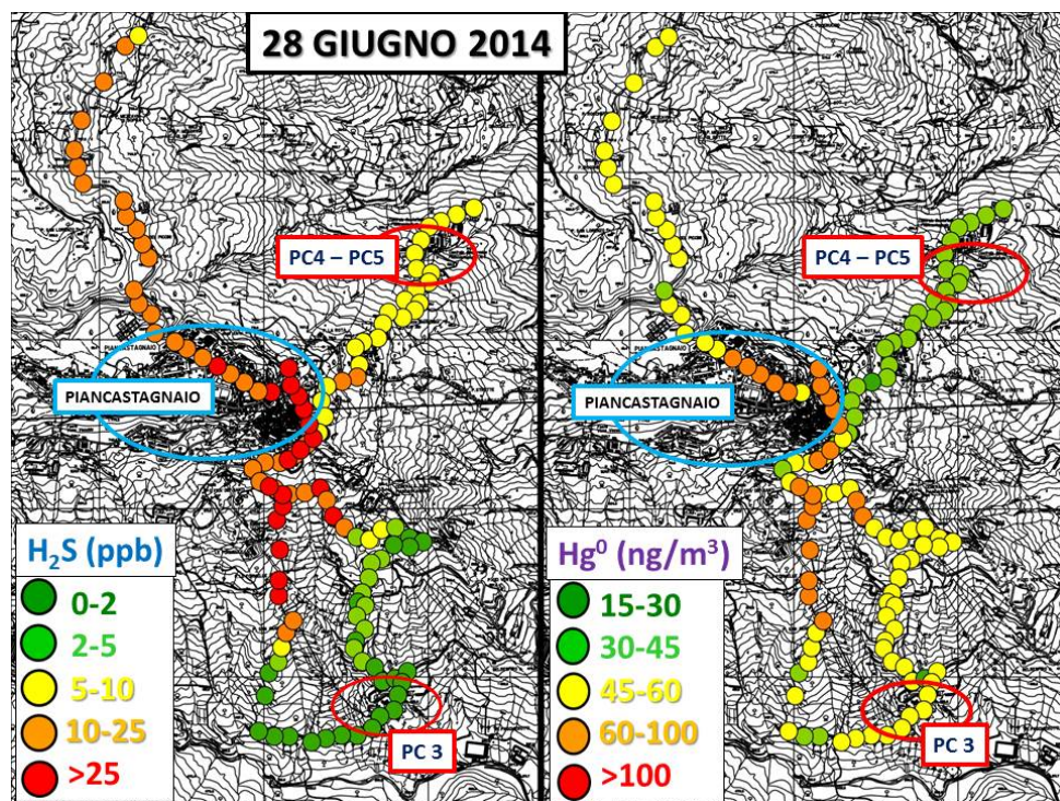
Figura 3.22 - Distribuzione delle concentrazioni di H_2S (parte sinistra) e Hg^0 (parte destra) lungo il percorso prestabilito nel giorno 28 giugno 2014. Le zone cerchiato rappresentano: a) abitato di Piancastagnaio (cerchio azzurro); b) centrali geotermoelettriche (cerchi rossi).
