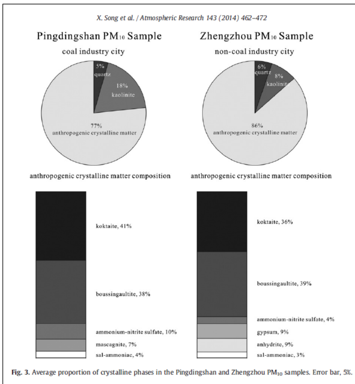
Figura 4.5 - Quantità medie delle specie cristalline rilevate nel PM10 delle città di Zhengzhou and Pingdingshan (Song et al. 2014).
