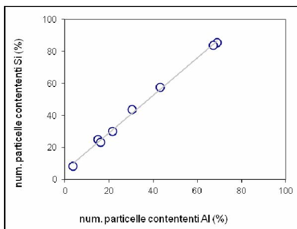
Figura 3.35 - Numero di particelle contenenti Si e contenenti Al per i campioni analizzati, espresso come percentuale.
