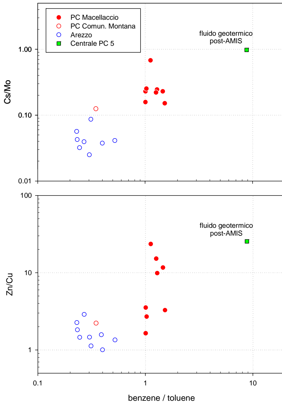
Fig. 4.8 Diagrammi binari relativi ai rapporti Zn/Cu e Cs/Mo versus benzene/toluene dei campioni prelevati a Piancastagnaio e Arezzo.
