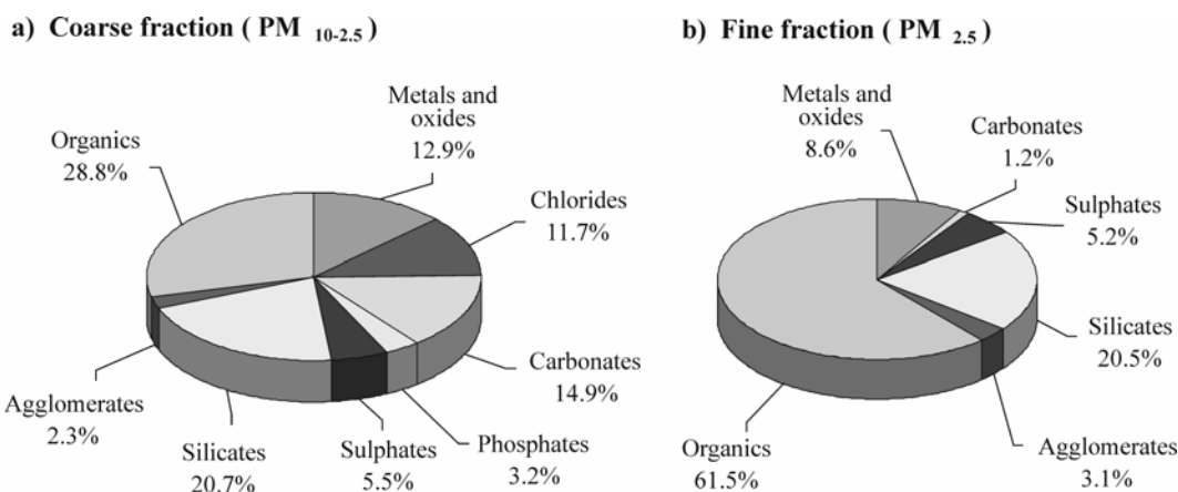
Figura 4.7 - Percentuali di particelle appartenenti alle fasi rilevate nella città di Prato, nelle frazioni PM 10-2.5 e PM 2.5 , tramite la tecnica di microanalisi SEM-EDS (Pratesi et al. 2007).
