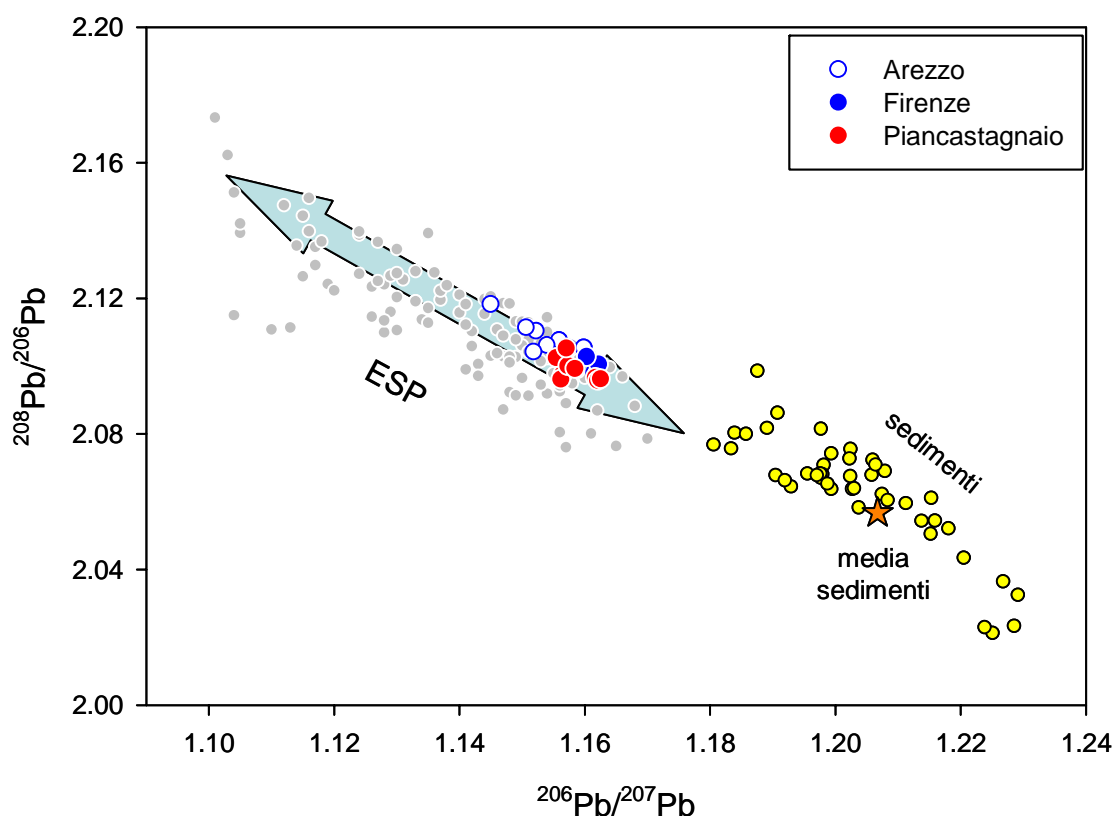
Figura 3.6 - Rapporti ^{206}\text{Pb}/^{207}\text{Pb} versus ^{208}\text{Pb}/^{206}\text{Pb} nei campioni di PM10 di Piancastagnaio, Arezzo e Firenze. Sono riportati anche valori dei rapporti isotopici misurati in sedimenti (cerchi gialli) e in campioni di aerosol europei (cerchi grigi). ESP: European Standard Pollution line (database da: Elbaz-Poulichet et al., 1984; Maring et al., 1987; Hopper et al., 1991; Erel et al., 1997; Veron et al., 1999; Tommasini et al., 2000; Bollhofer & Rosman 2001; Haack et al., 2002; Tommasini 2007).
