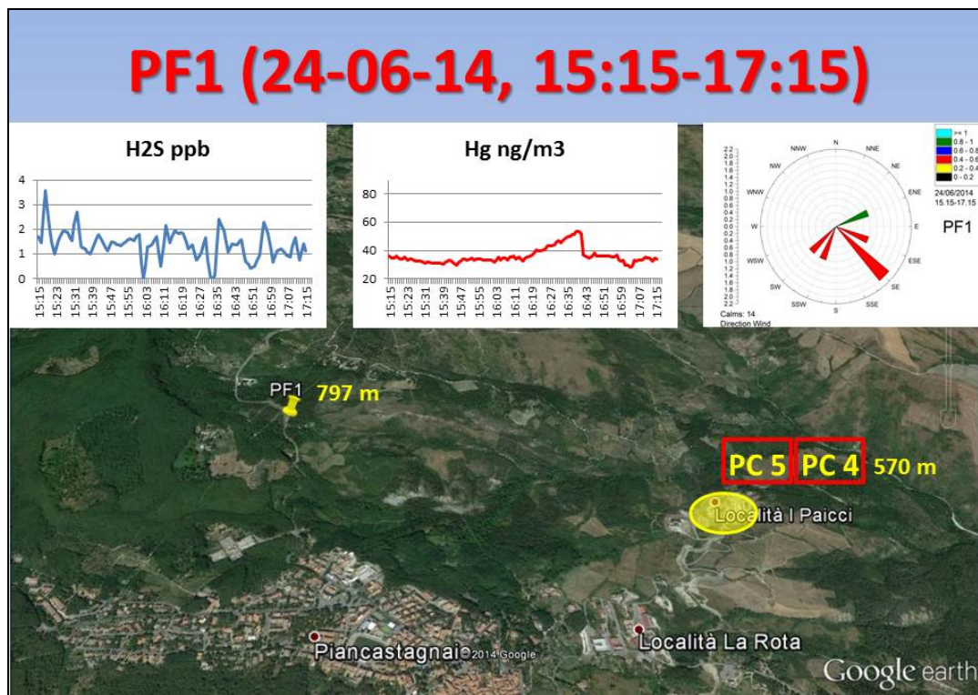
Figura 3.14 - Ubicazione e quota del punto fisso PF1 rispetto alle centrali geotermoelettriche con relativi andamenti delle concentrazioni di H_2S e Hg^0 rispetto al tempo. In alto a destra la rosa dei venti relativa alle due ore di misura.
