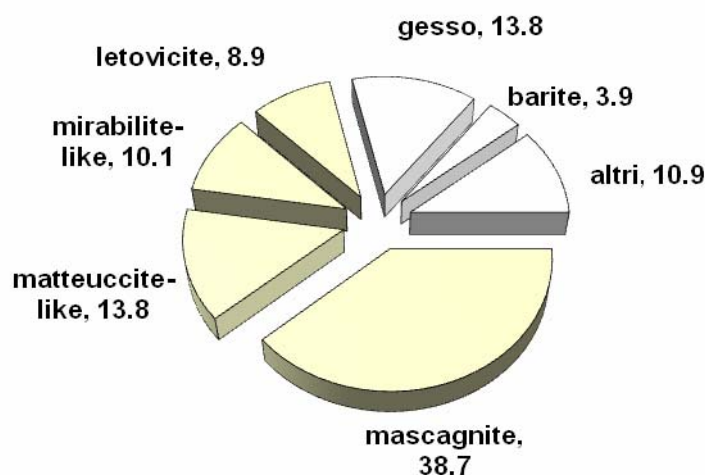
Figura 3.30 - Concentrazione relativa delle specie appartenenti al solo gruppo dei solfati che compongono il PM10 raccolto a Piancastagnaio, espressa come percentuale sul numero di particelle, del totale analizzato.
