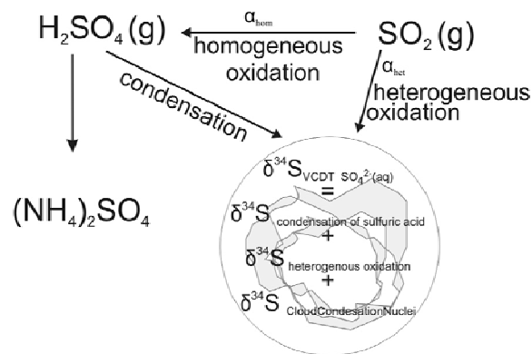
Figura 3.24 – Caratterizzazione isotopica della sorgente di \text{SO}_2 durante il processo di ossidazione omogeneo (fase gassosa) ed eterogeneo (fase acquosa). Assumendo che la composizione isotopica della sorgente di \text{SO}_2 sia nota e che nessun solfato primario solubile in acqua abbia agito come nucleo di condensazione di nuvole, è possibile calcolare il contributo relativo della condensazione dell'acido solforico gassoso su di una goccia e l'ossidazione eterogenea nella goccia d'acqua. La composizione isotopica può essere stimata dalle particelle che derivano dalla conversione gas-particella come, ad esempio, il solfato di ammonio.
