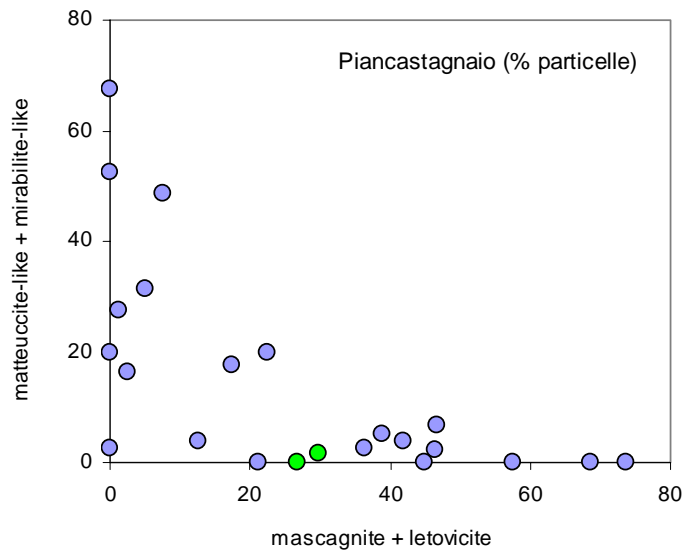
Figura 3.32 – Somma delle concentrazioni relative (%) di particelle di mascagnite e letovicite contro la somma delle concentrazioni di matteuccite-like e mirabilite-like nei campioni analizzati del PM10 raccolto a Piancastagnaio. In verde i campioni raccolti nel sito urbano di Piancastagnaio.
