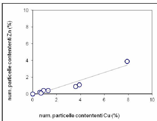
Figura 3.36 - Numero di particelle contenenti Zn e Cu per i campioni analizzati, espresso come percentuale.
