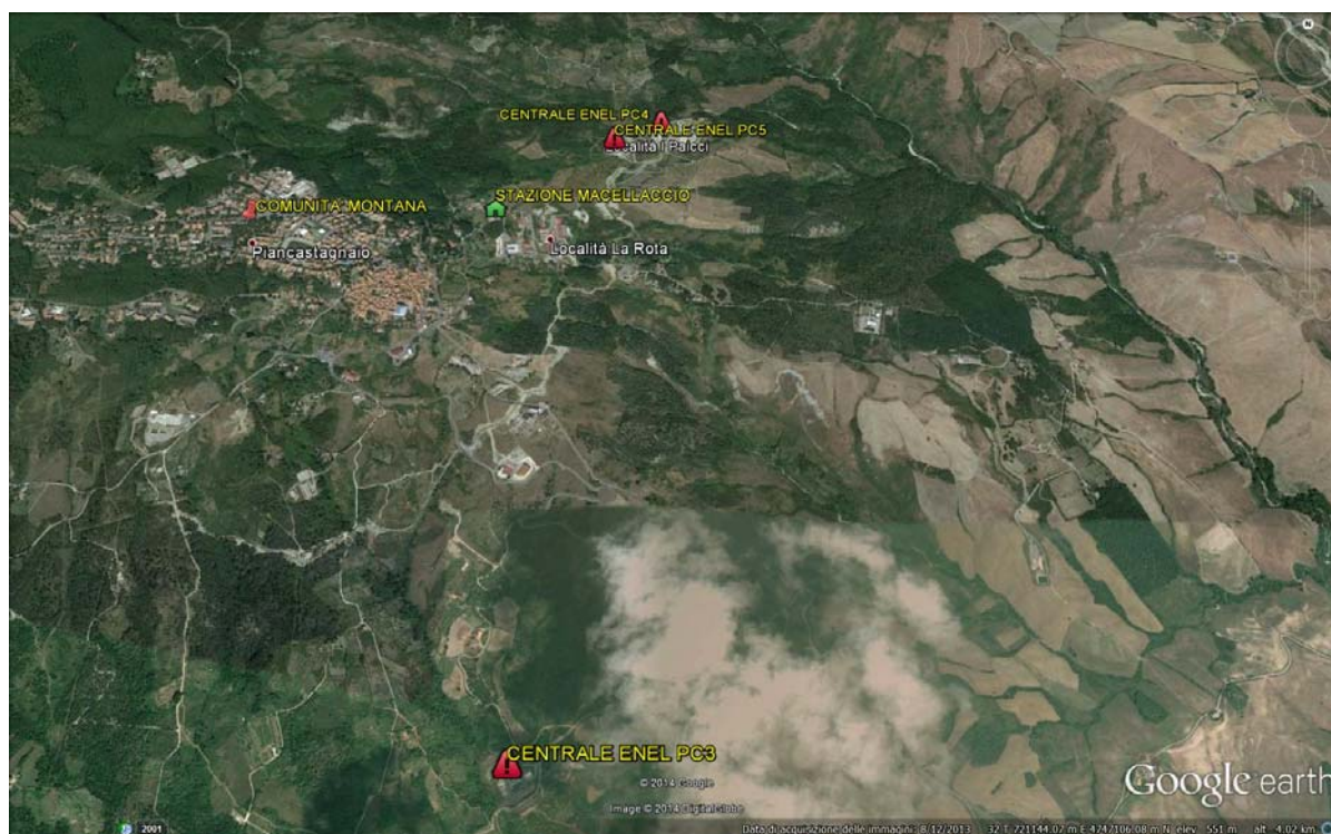
Figura 2.1 - Mappa dell'area di Piancastagnaio con l'ubicazione delle tre centrali geotermoelettriche di Enel e delle postazioni di misura.
