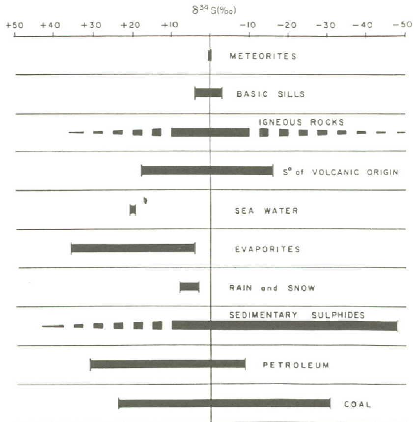
Figura 3.23 – Variazione degli isotopi dello zolfo nei principali reservoir terrestri.
