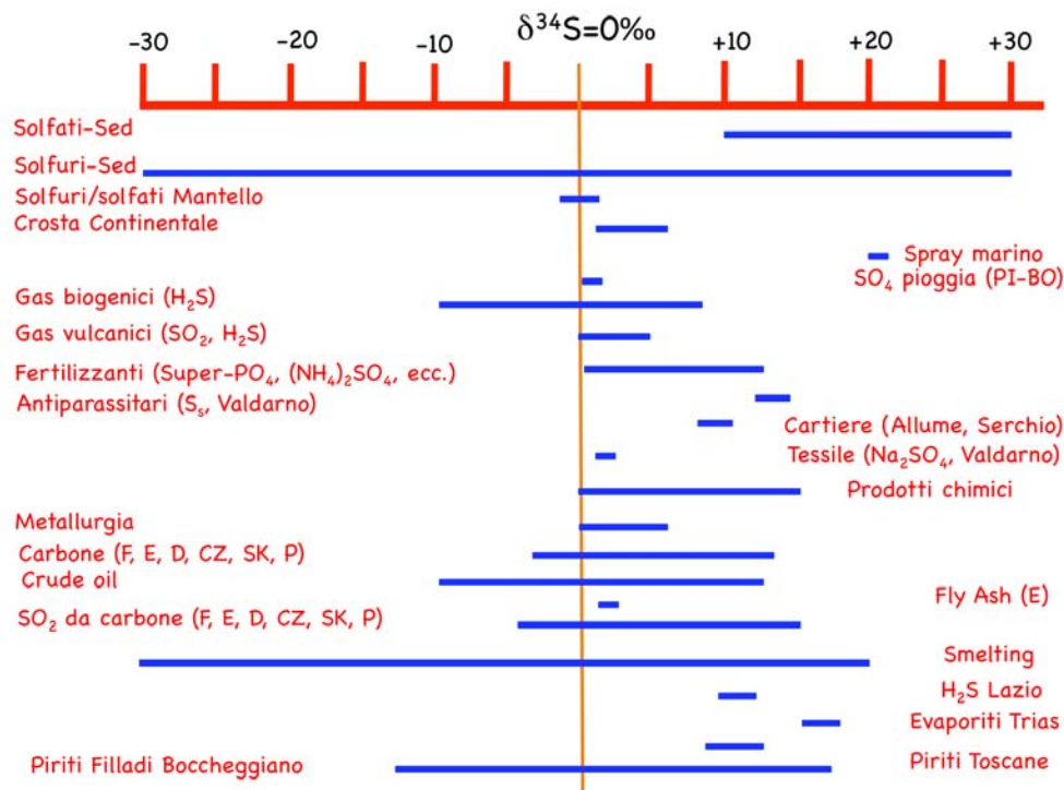
Figura 3.25 – Intervalli isotopici dello zolfo relativi ai potenziali apporti naturali ed antropici in atmosfera.
