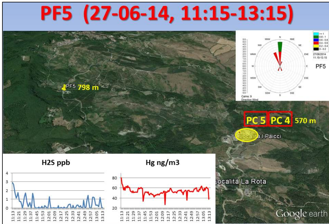
Figura 3.19 - Ubicazione e quota del punto fisso PF5 rispetto alle centrali geotermoelettriche con relativi andamenti delle concentrazioni di H_2S e Hg^0 rispetto al tempo. In alto a destra la rosa dei venti relativa alle due ore di misura.
