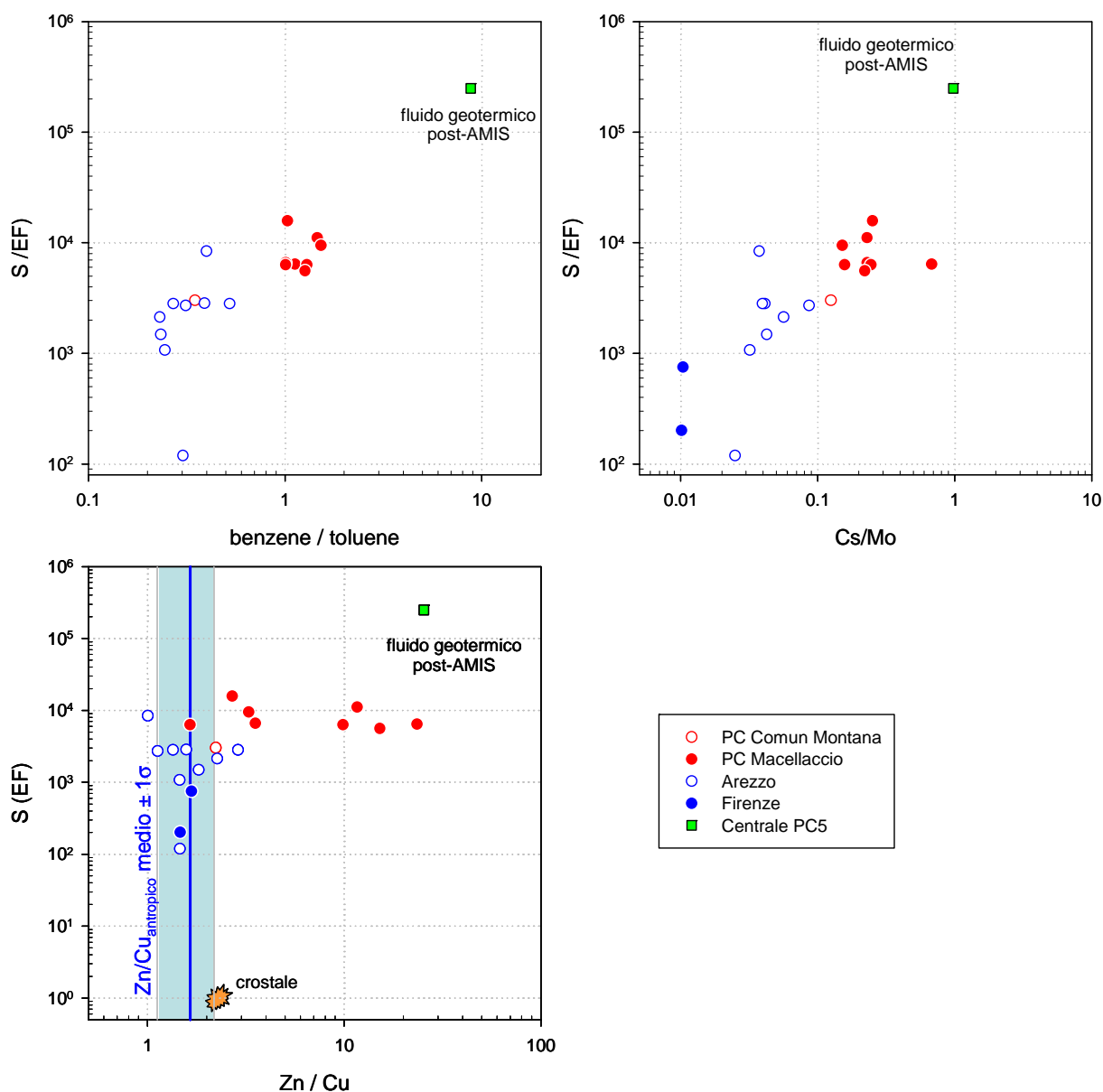
Figura 4.9 - Fattore di arricchimento di Zolfo versus il rapporto benzene/toluene, Cs/Mo e Zn/Cu nei campioni di PM10 di Piancastagnaio, Arezzo e Firenze, nonché nel fluido geotermico della centrale PC5.
