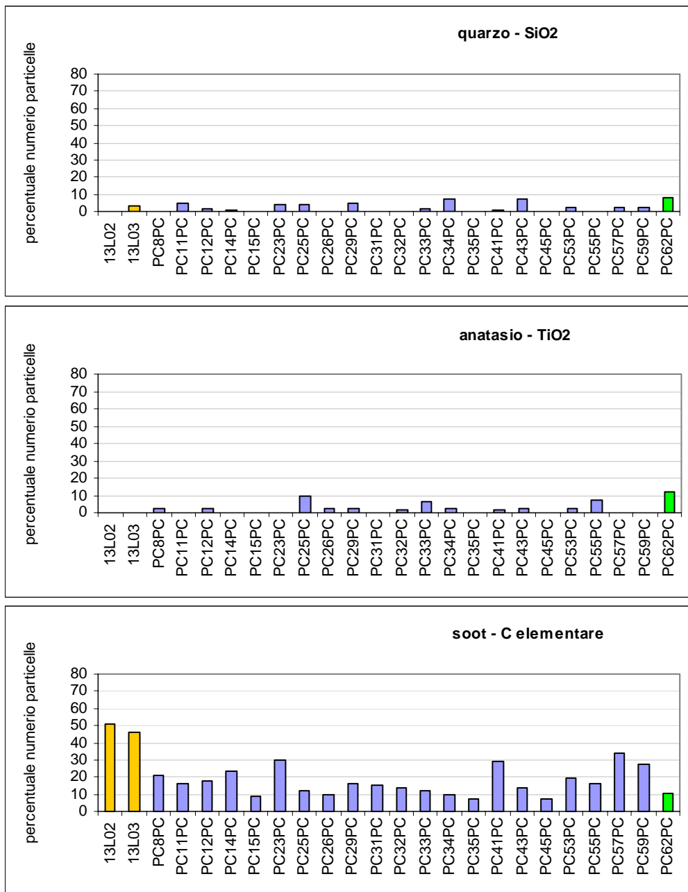
Figura A.2 - Concentrazione relativa dei minerali maggiormente abbondanti nel PM 10 raccolto a Piancastagnaio per i campioni analizzati, espressa come percentuale sul numero di particelle. Gli istogrammi mostrano lo stesso intervallo nella scala verticale. In arancio i campioni raccolti nel sito urbano di Piancastagnaio. Il campione PC26PC è stato raccolto nella località di Gallina.
