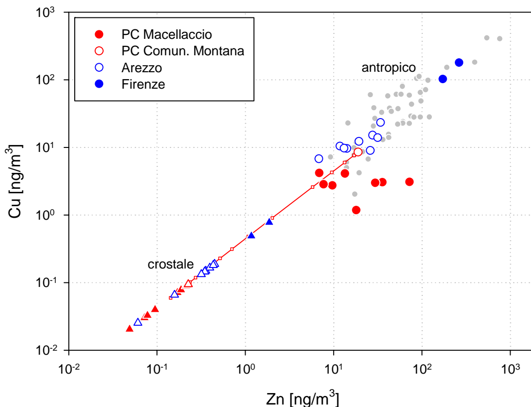
Figura 3.7 - Concentrazioni di Zn versus Cu nei campioni di PM10 di Piancastagnaio, Arezzo e Firenze (vedi testo). Sono riportate anche le concentrazioni in campioni di aerosol europei (cerchi grigi), (database da: Sternbeck et al., 2002; Johansson et al., 2009; Dongarrà et al., 2010; Pey et al., 2010; Terzi et al., 2010; Albade et al., 2011; Amato et al., 2011; Muranszky et al., 2011; Gianini et al., 2012; Tecer et al., 2012; Avino et al., 2014; Balcilar 2014; Ivosevic et al., 2014)
