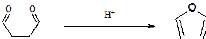
Figura 4.4: Sintesi Paal-Knorr del C 4 H 4 O.
