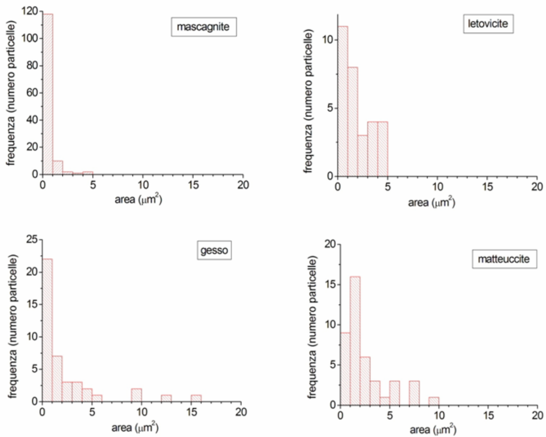
Figura 3.33 - Istogramma della distribuzione di frequenza dei valori dell'area delle particelle misurate, per le fasi maggiormente abbondanti: mascagnite, letovicite, gesso e matteuccite-like.
