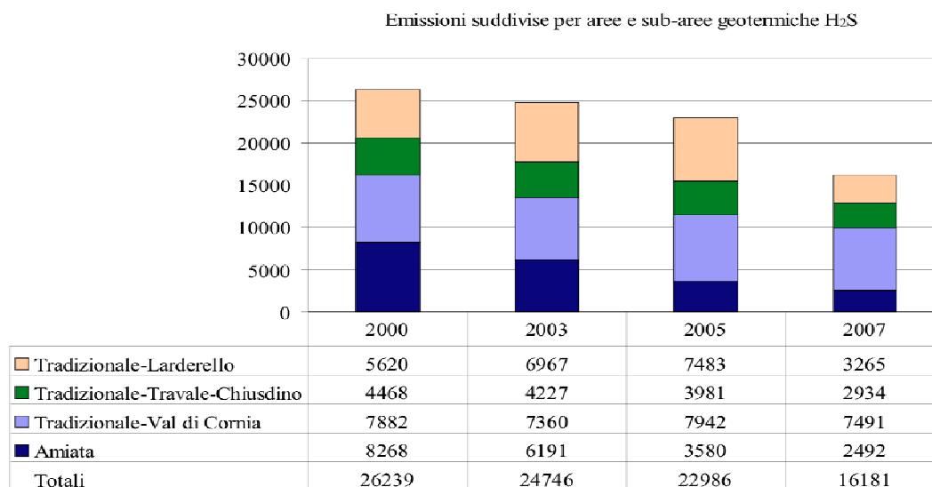
Figura 3.26 – Emissioni di H 2 S (ton/anno) dalle centrali geotermoelettriche toscane.
