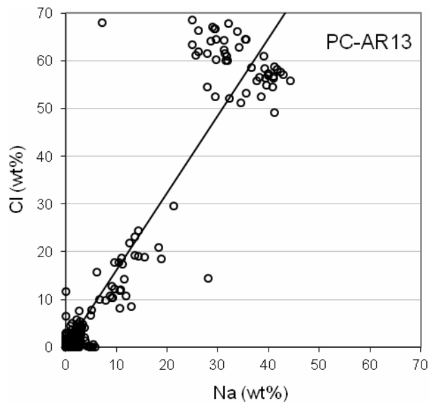
Figura 3.39 – Valori della concentrazione, come percentuale in peso in atomi, del Na e Cl misurato nelle particelle analizzate (SEM-EDS) nel campione PC-AR13.
