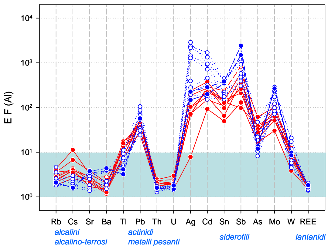
Fig. 3.3 – Fattori di arricchimento (EF) dei campioni di PM10 di Piancastagnaio, Arezzo e Firenze.
