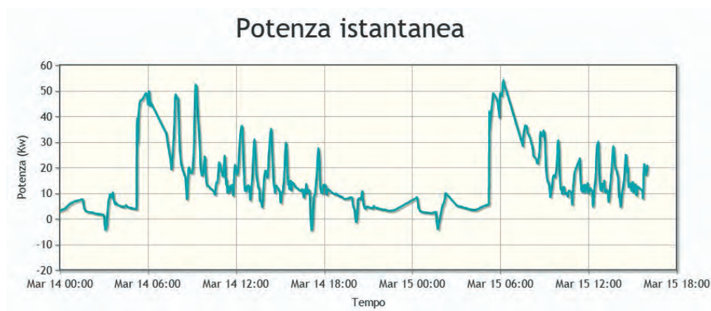
Figura 7.7. Esempio di grafico in tempo reale della potenza istantanea di un impianto monitorato.
