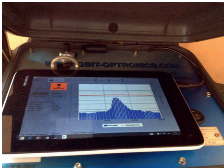
Figura 7.6. Modulo qualità dell'aria, sistema di rilevazione delle polveri ( PM_{2,5} ).
