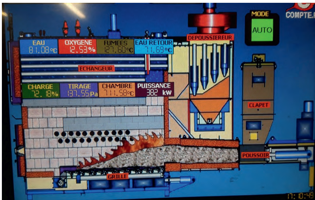
Figura 5.1. Monitor di controllo dell'impianto di Cité Aurore - Bastia (Corsica). La caldaia è in modulazione ad una potenza di 382 kw, rispetto ad una potenza nominale di 550 kw. La camera di combustione supera di poco i 700°C ed il livello di O 2 è al 12,53%.
