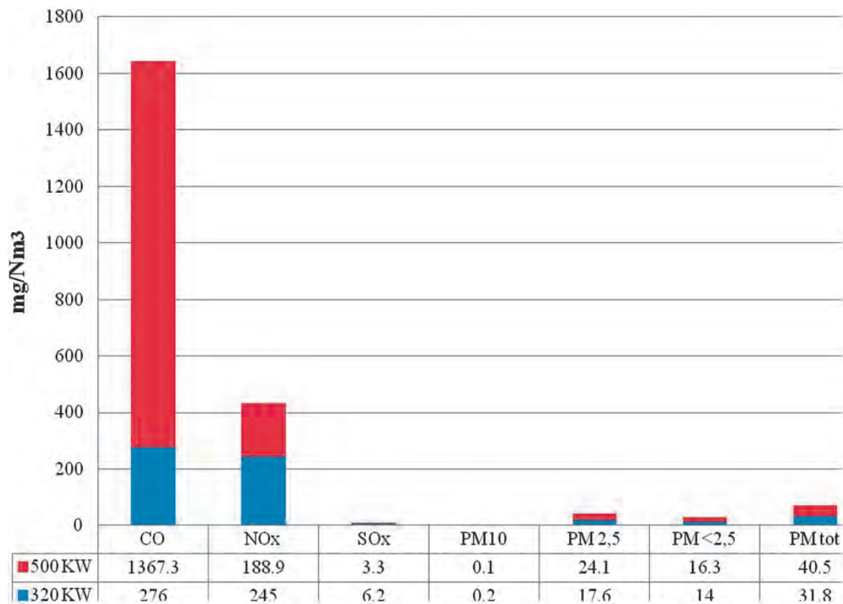
Figura 5.10. Emissioni della centrale di TLR di San Romano in Garfagnana (mg/Nm 3 ).
