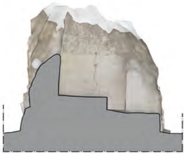
Sezione LL'
