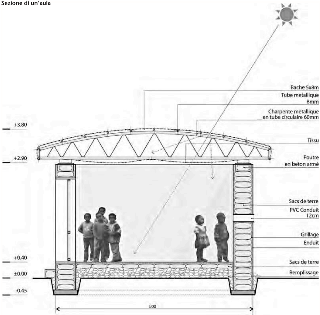
Sezione di un'aula
