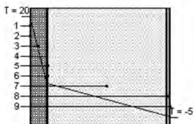
Stratigrafia struttura
