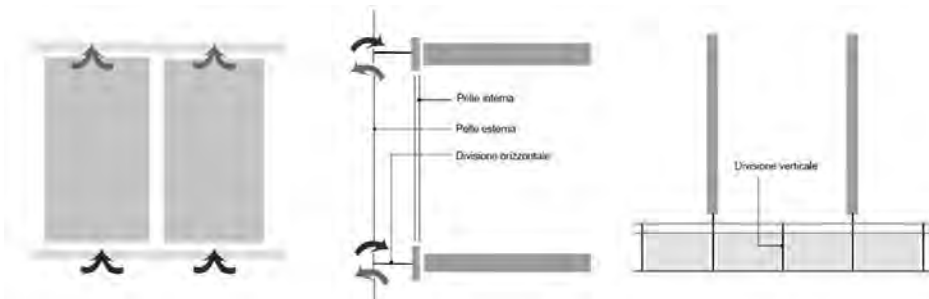
Fig. 3.6 – Schema del sistema di ventilazione nelle facciate “box windows”
