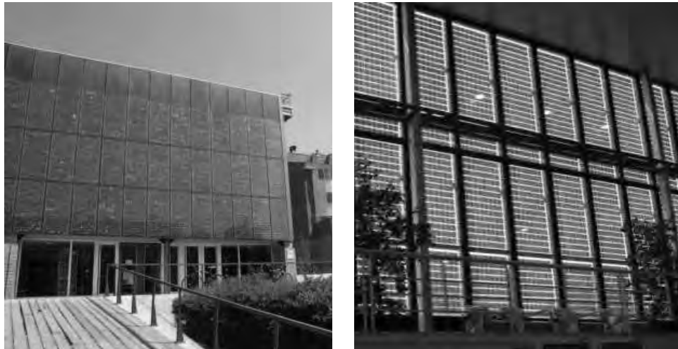
Fig. 2.10: Biblioteca Pública Pompeu Fabra, Miquel Brullet Matarò, Barcellona, Spagna, 1998. Si tratta di uno dei primi edifici d'Europa in cui è realizzata una facciata fotovoltaica in pannelli di silicio policristallino semitrasparente. Il fotovoltaico contribuisce alla produzione di energia elettrica per l'edificio e funziona come sistema di ombreggiatura per la sala lettura.
