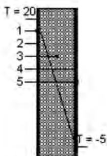
Stratigrafia struttura
