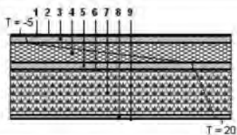
Stratigrafia struttura
