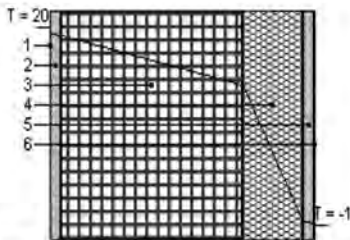
Stratigrafia struttura
