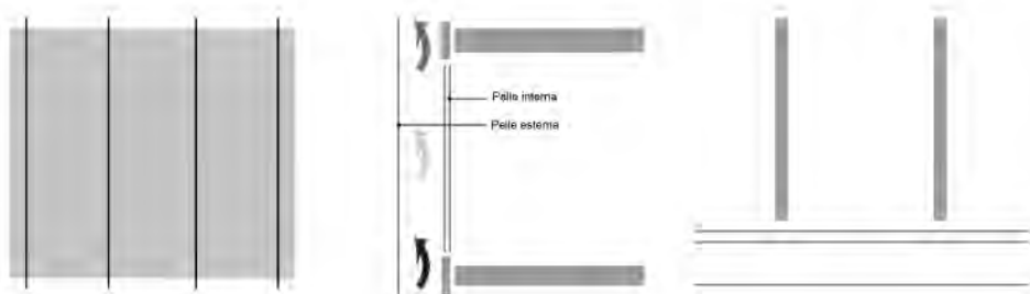
Figura 3.9: Sistema di ventilazione nelle "multistory facades"
