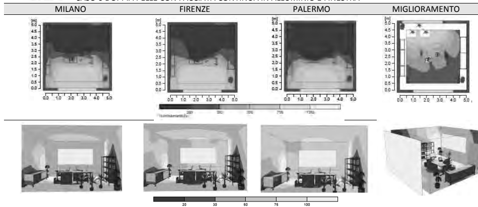
CASO 6 DOPPIA PELLE CON FACCIAIA CONTINUA IN ALLUMINIO E FINESTRA
