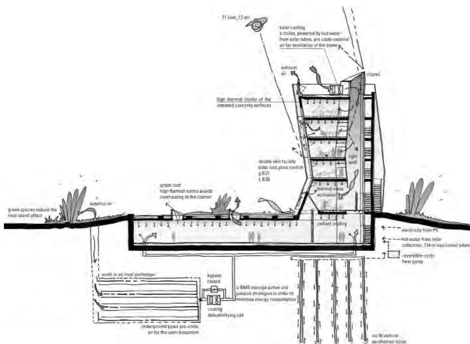
Fig. 1.6: CSET, Centre for Sustainable Energy Technologies, Mario Cucinella Architects, Ningbo, China, 2009. Sezione Bioclimatica con analisi del funzionamento nei mesi estivi.
