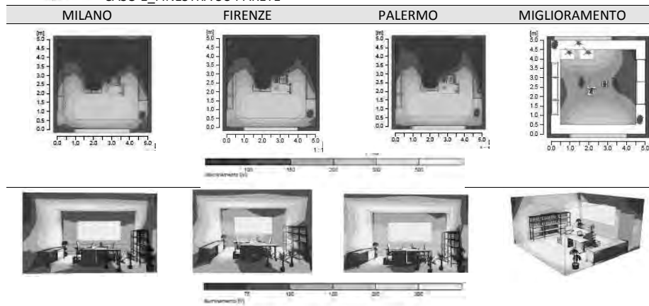
CASO 1_FINESTRA SU PARETE
