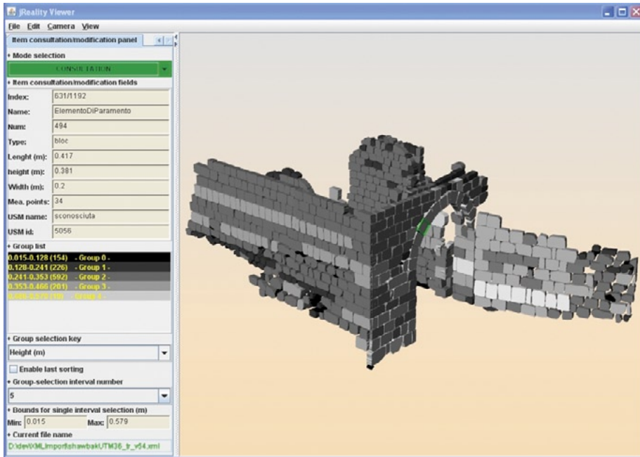
Fig. 10 – Visualisation 3D avec affectation de couleur en fonction de l'appartenance à une classe basée sur la hauteur des blocs.
