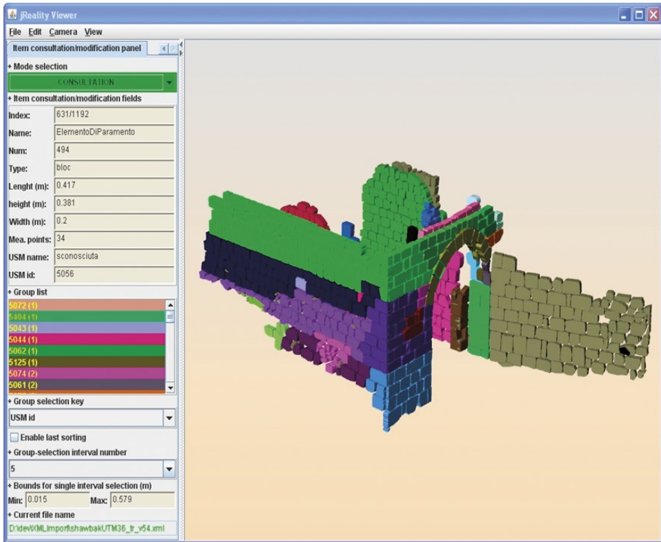
Fig. 9 – Visualisation 3D des blocs avec une couleur en fonction de leur USM. Le panneau de gauche permet la consultation/modification du bloc sélectionné.
