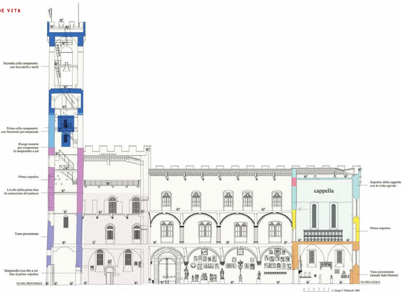
Sezione longitudinale sull'ala settentrionale del cortile e la cappella della Maddalena Longitudinal section of the courtyard's northern wing and the Maddalena chapel
