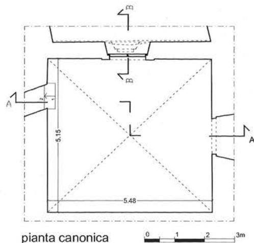
pianta canonica
