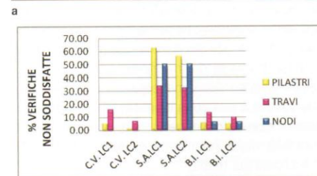
Figura 32 – Confronto dei risultati delle tre analisi, in termini generali (a) e di elementi (b)
