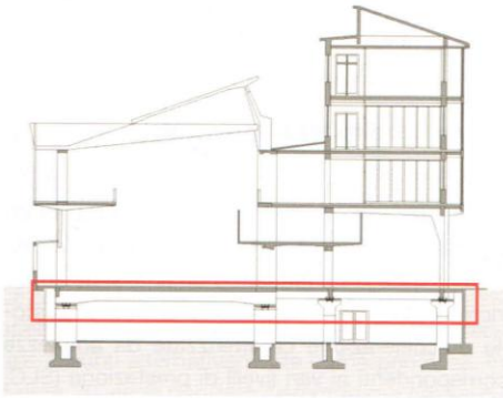
Figura 24 - Sezione trasversale dell'edificio isolato
