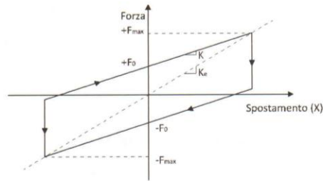
Figura 27 - Ciclo d'isteresi caratterizzante un dispositivo del tipo DFP
